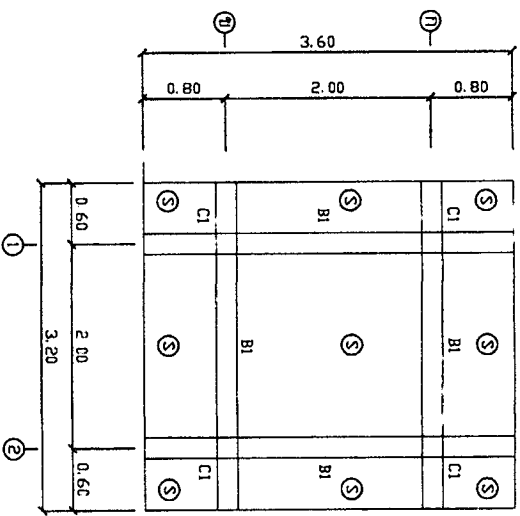
แปลนฐาน B1 1:50
