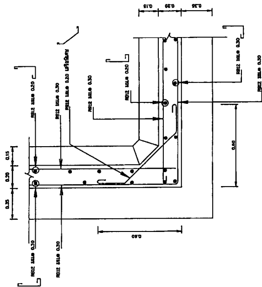
รูปขยายการเสริมเหล็กมุงถึง
