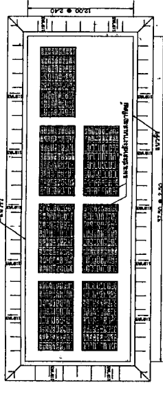
แบบแปลนอาคารพาณิชย์ 10 ชั้น 1 : 125
