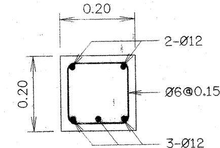
การเสริมเหล็กคานฟาบดบ่อ
