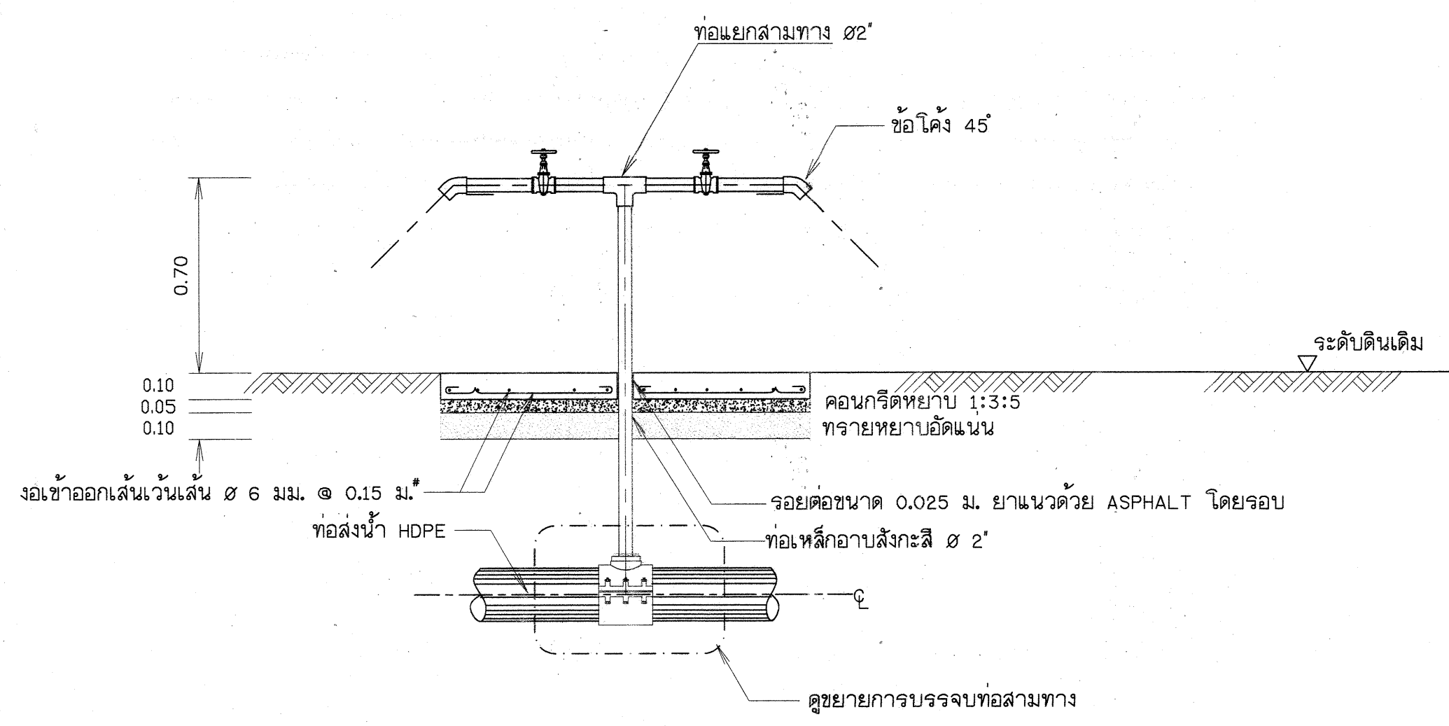
รูปตัด ก - ก
