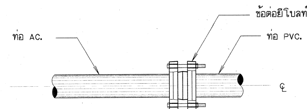
การบรรจุท่อ AC. กับท่อ PVC.
