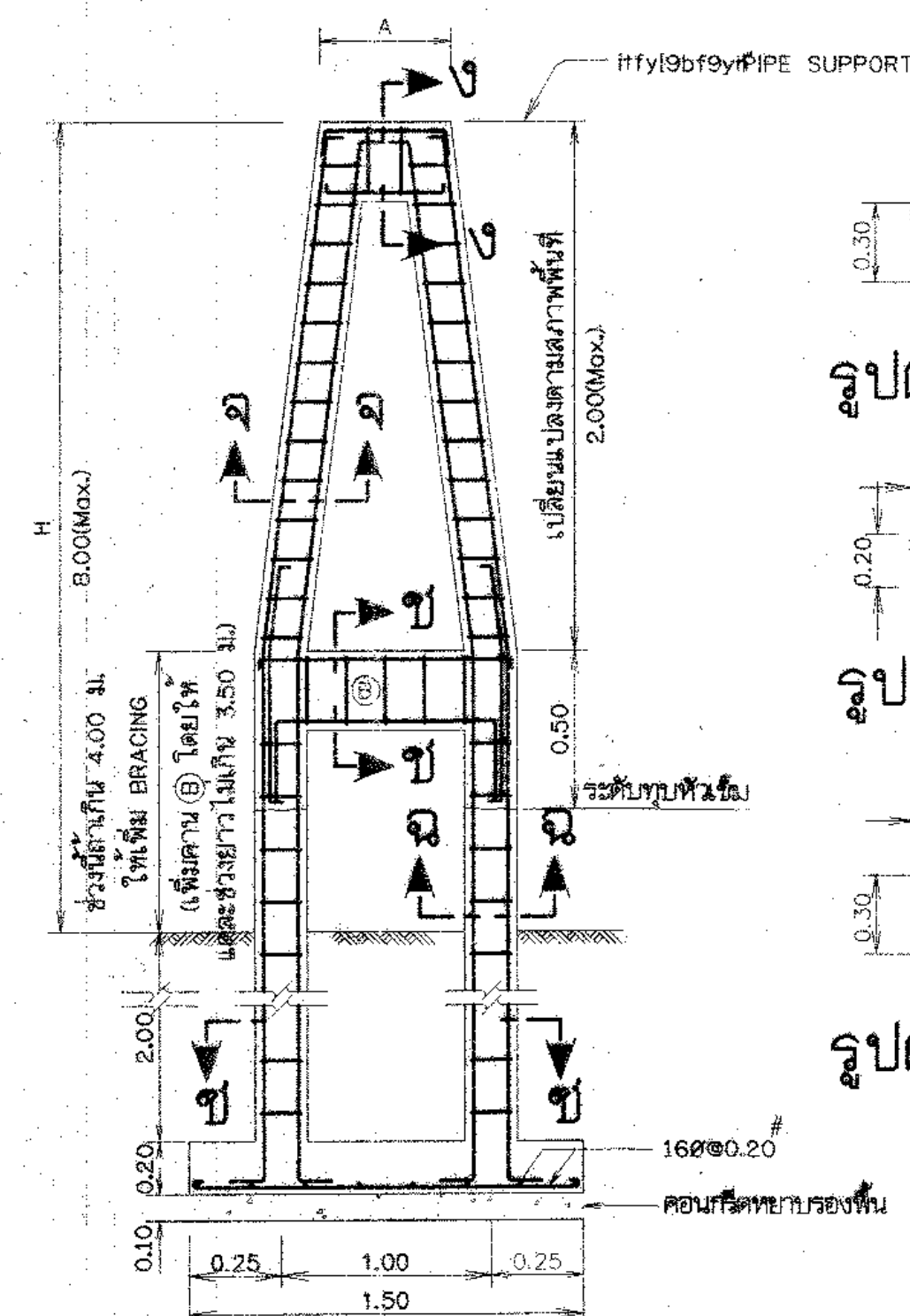
การเสริมเหล็ก ดอม่อบทที่ 2
