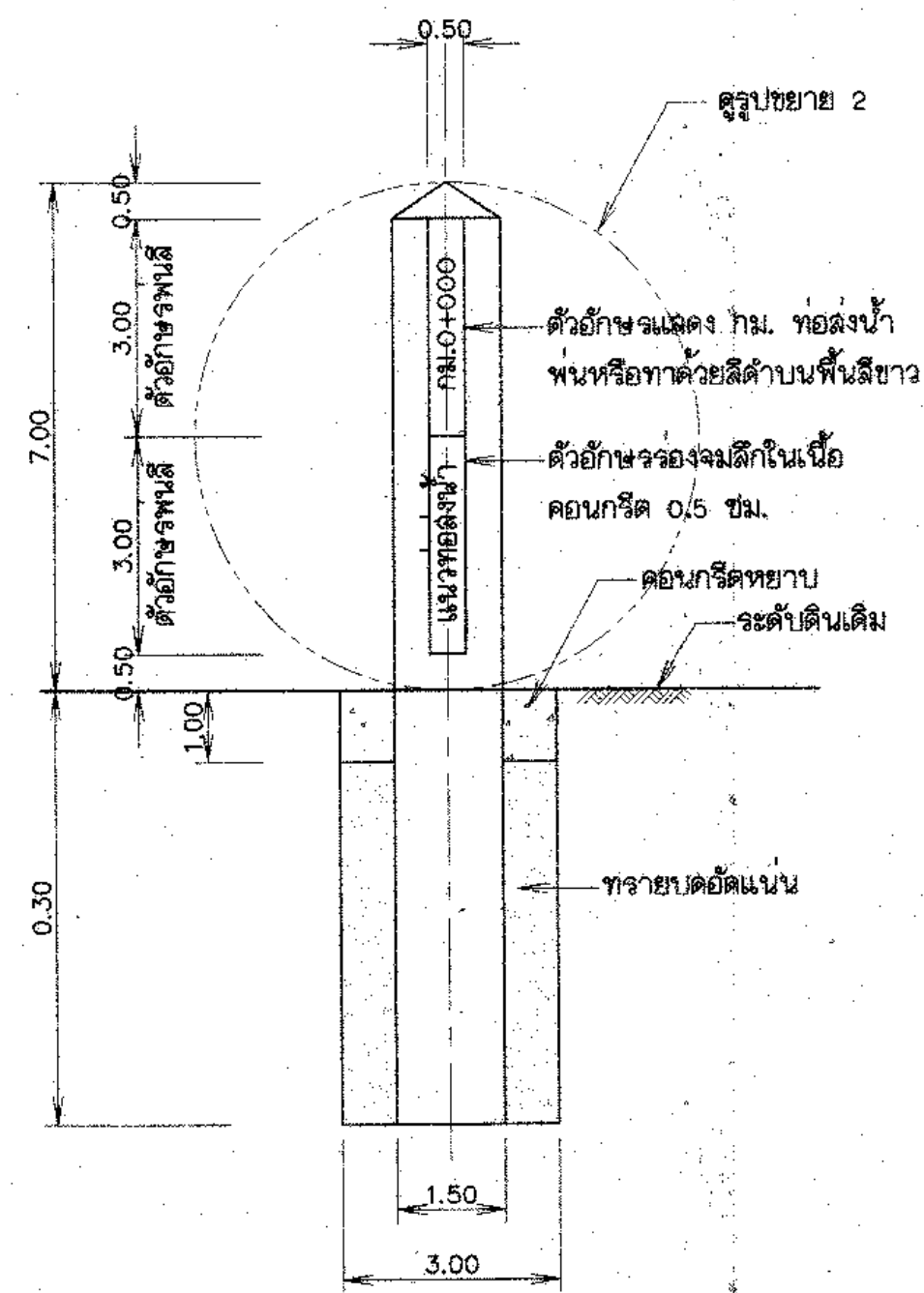
รูปตัด ก-ก แบบที่ 1 แสดง กม.ท่อดังน้ำ ไม่แสดงมาตราส่วน
