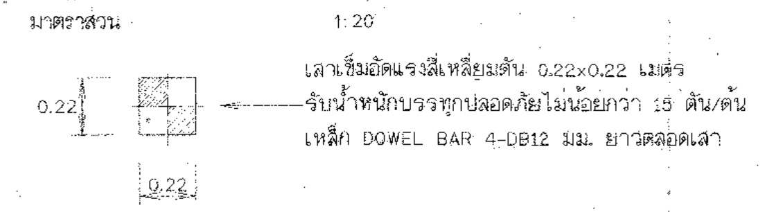
แบบขยายเสาเข็ม P2
