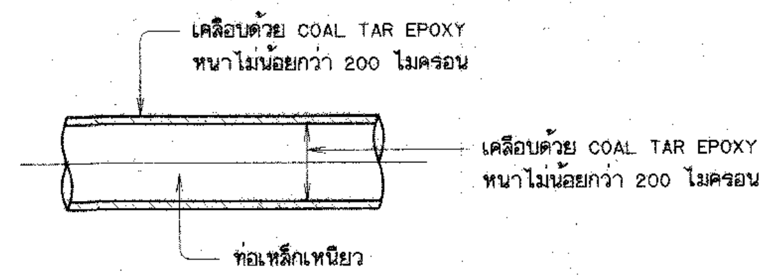
การเคลือบผิวท่อเหล็ก
