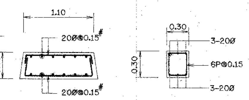
รูปตัด ก-ก ข-ข ค-ค
