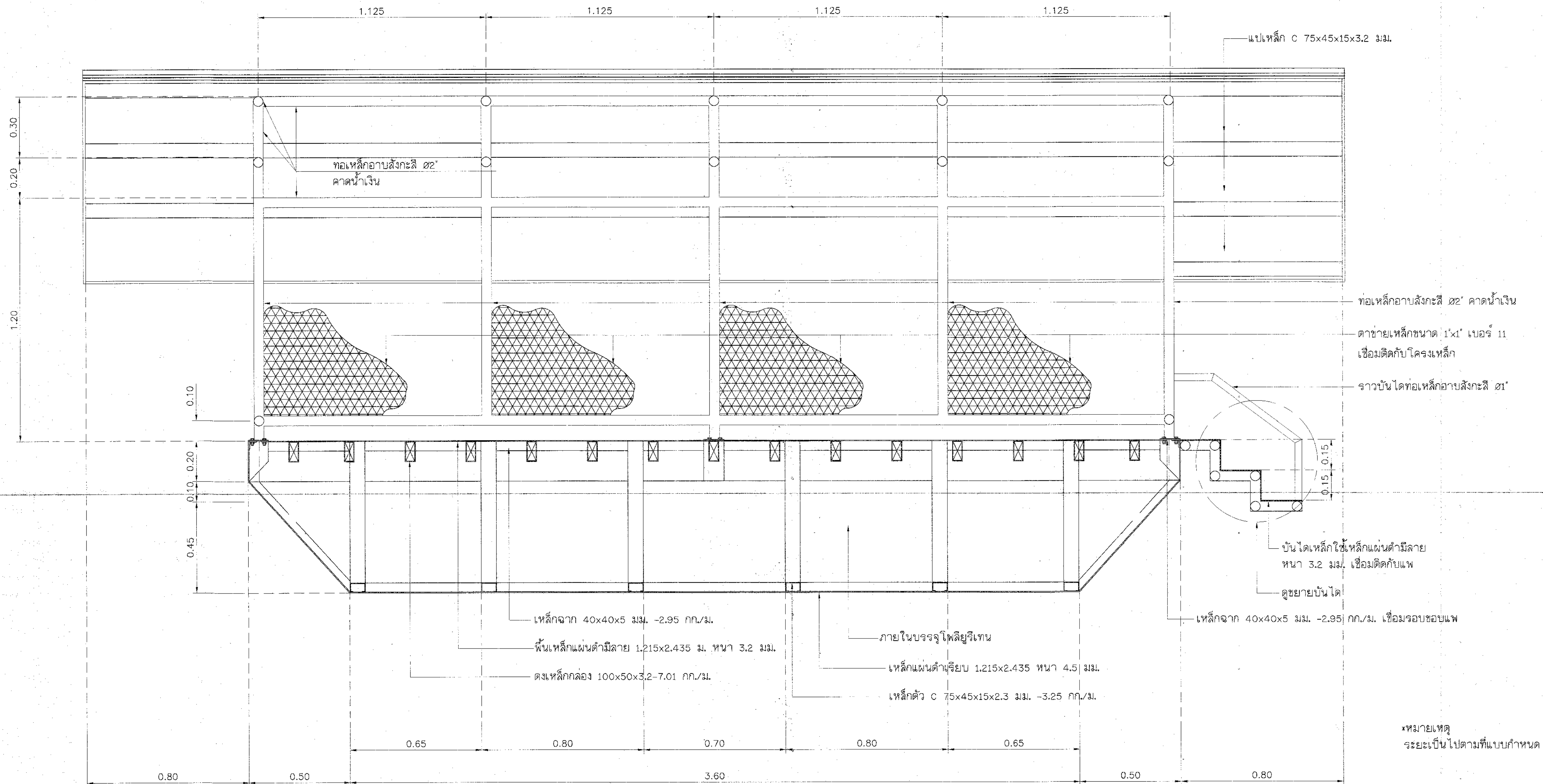
รูปตัด B-B ไม่แสดงมอดูลส่วน
