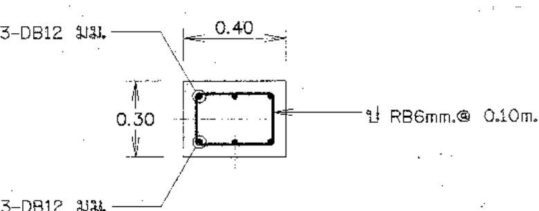
แบบขยายคาน B3
