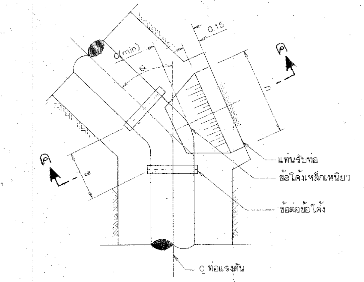
แปลน มาตราส่วน 1:10
