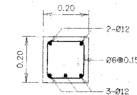
การเสริมเหล็กคานฟาดบ่อ มาตราส่วน 1:10
