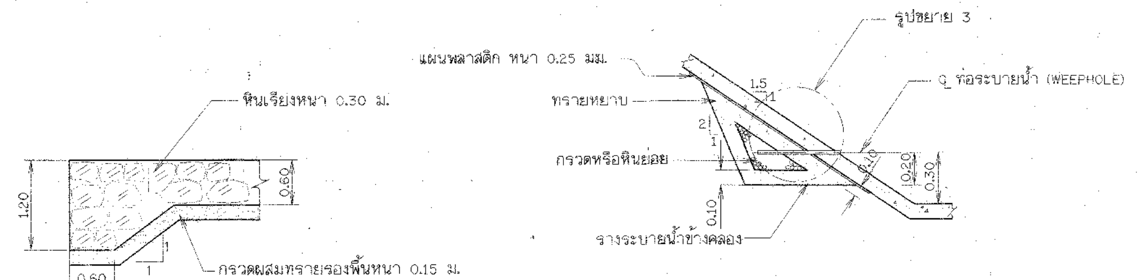
รูปขยาย 2
