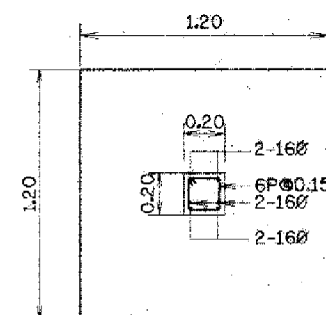
รูปตัด ก-ก ข-ข ค-ค
