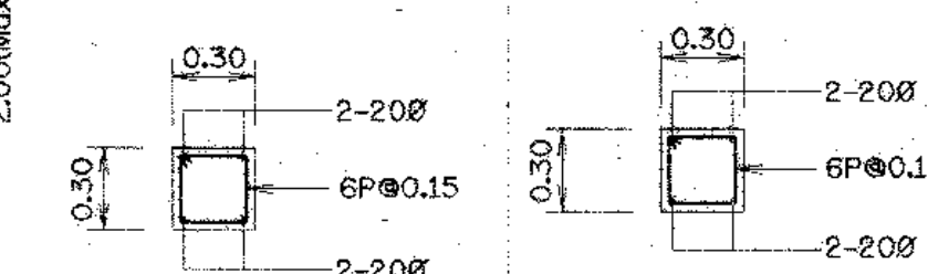
รูปตัด ก-ก ข-ข ค-ค
