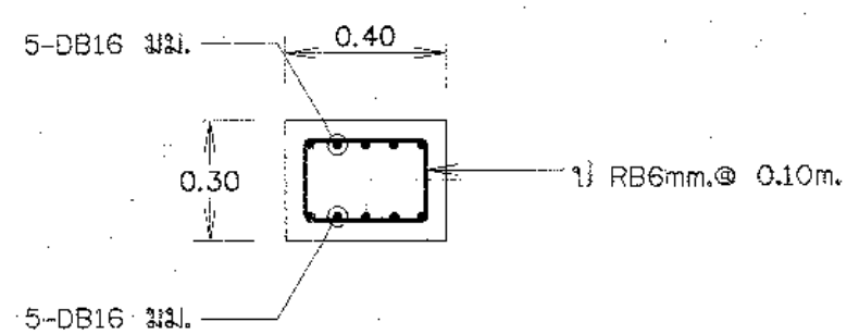
แบบขยายคาน B2
