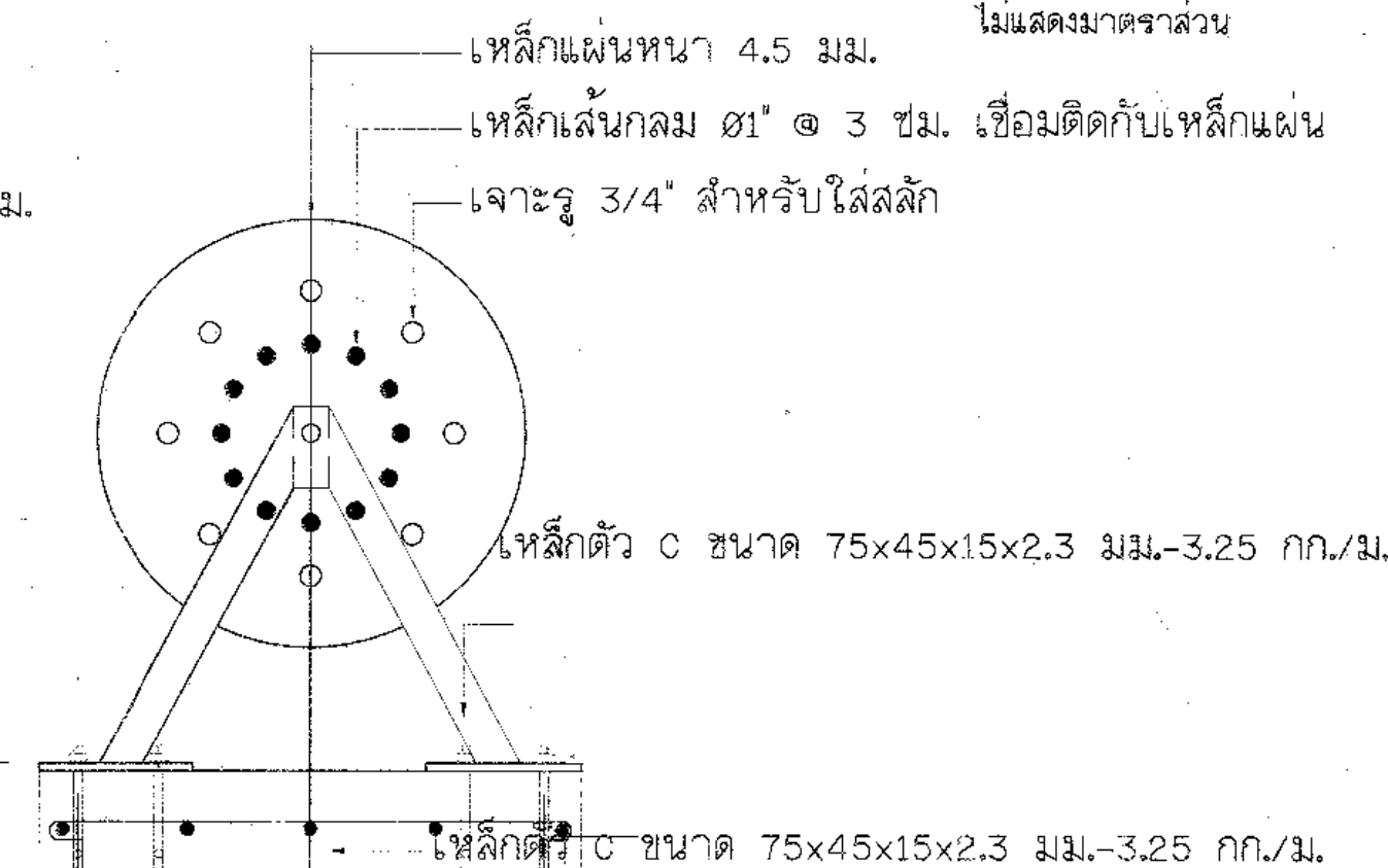
แบบขยาย "ด"
