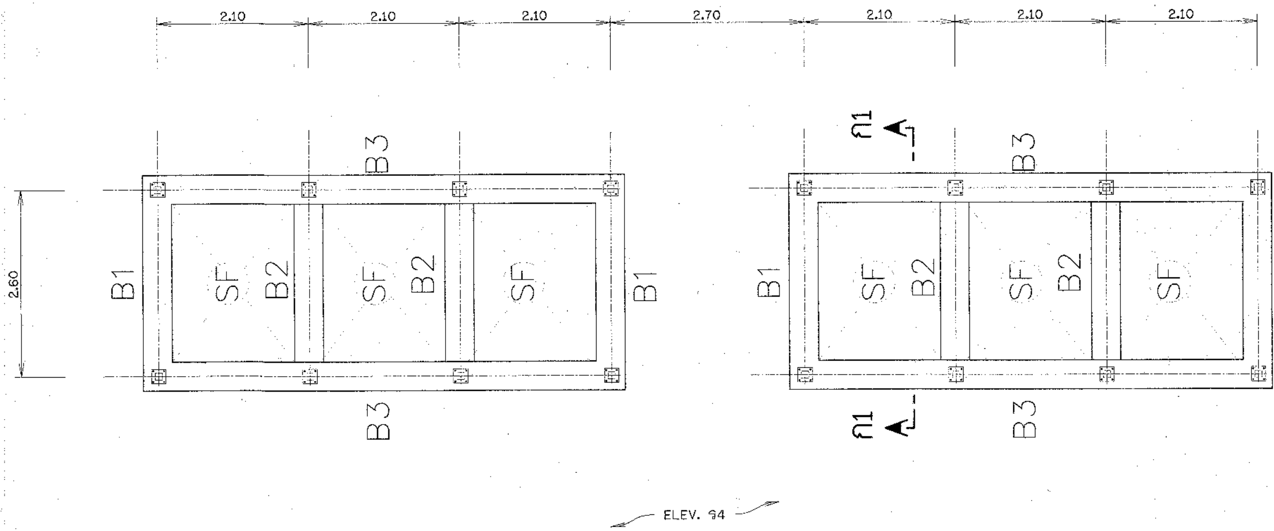
แปลนคานาคอนกรีตเสริมเหล็กชั้นวางแสงอาทิตย์
