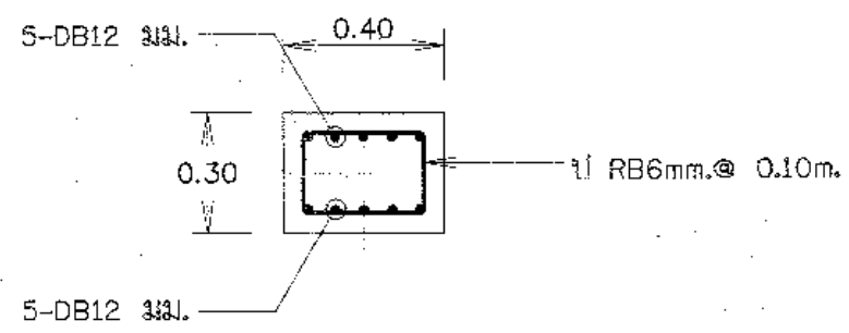
แบบขยายคาน B1
