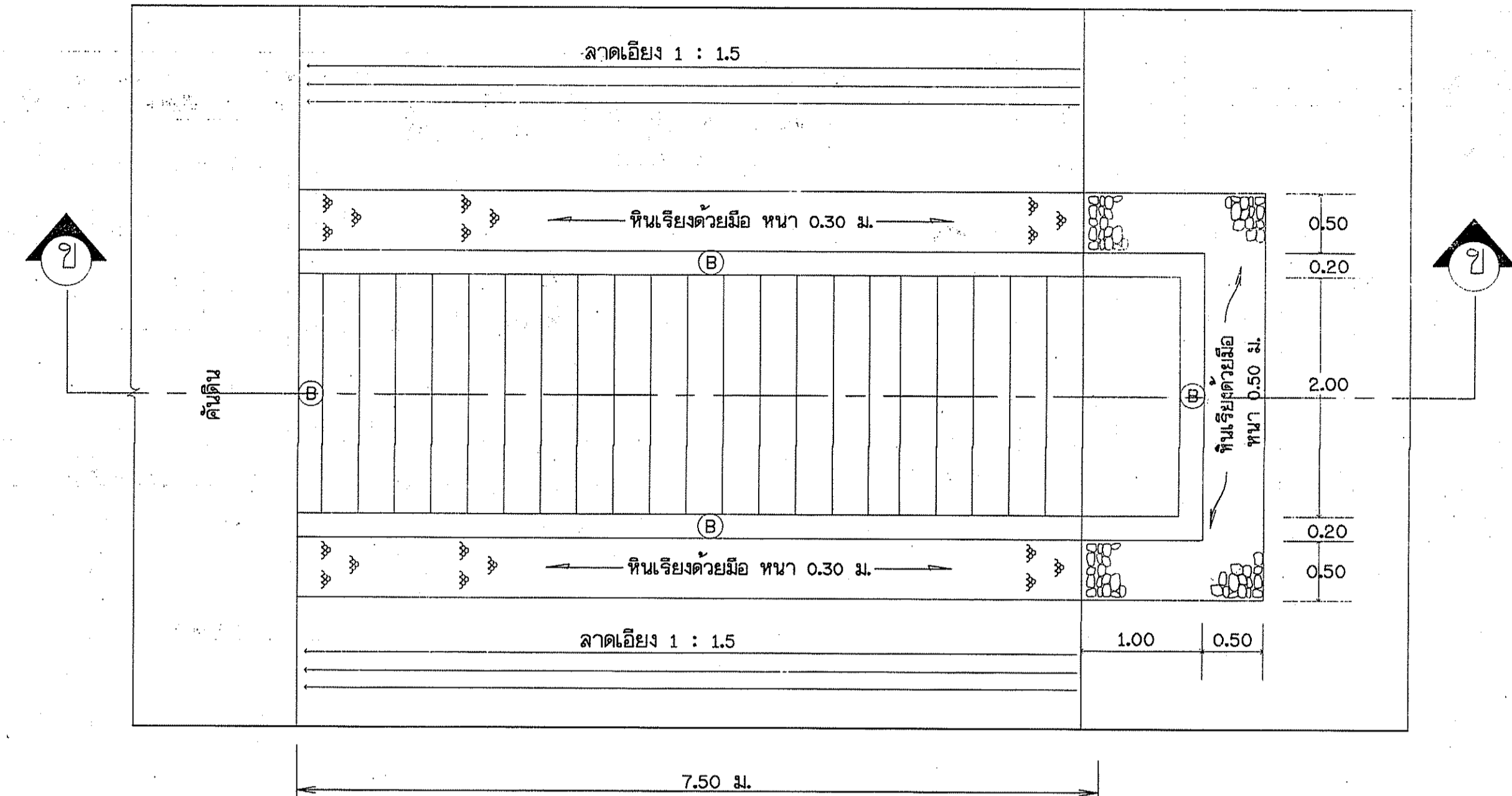
แปลนบันได คสล. แบบไม่มีช่องทาง
