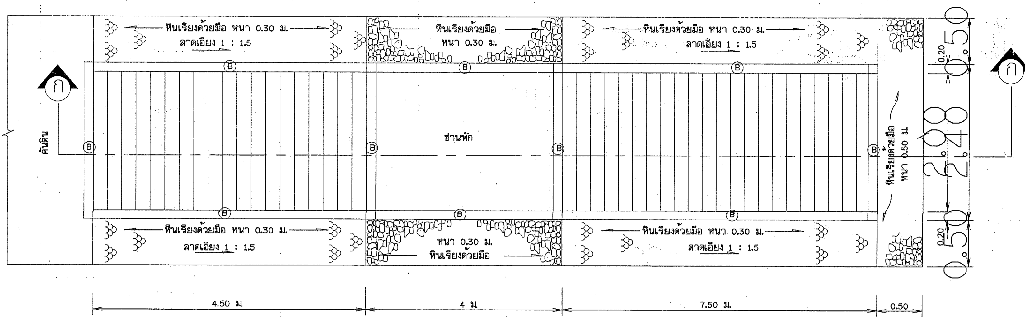
แปลนบันได คสล. แบบมีช่องทาง
