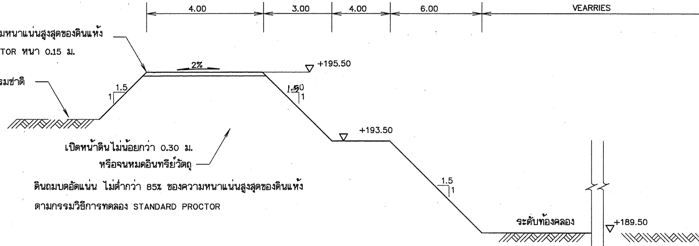
รูปตัดทั่วไป
