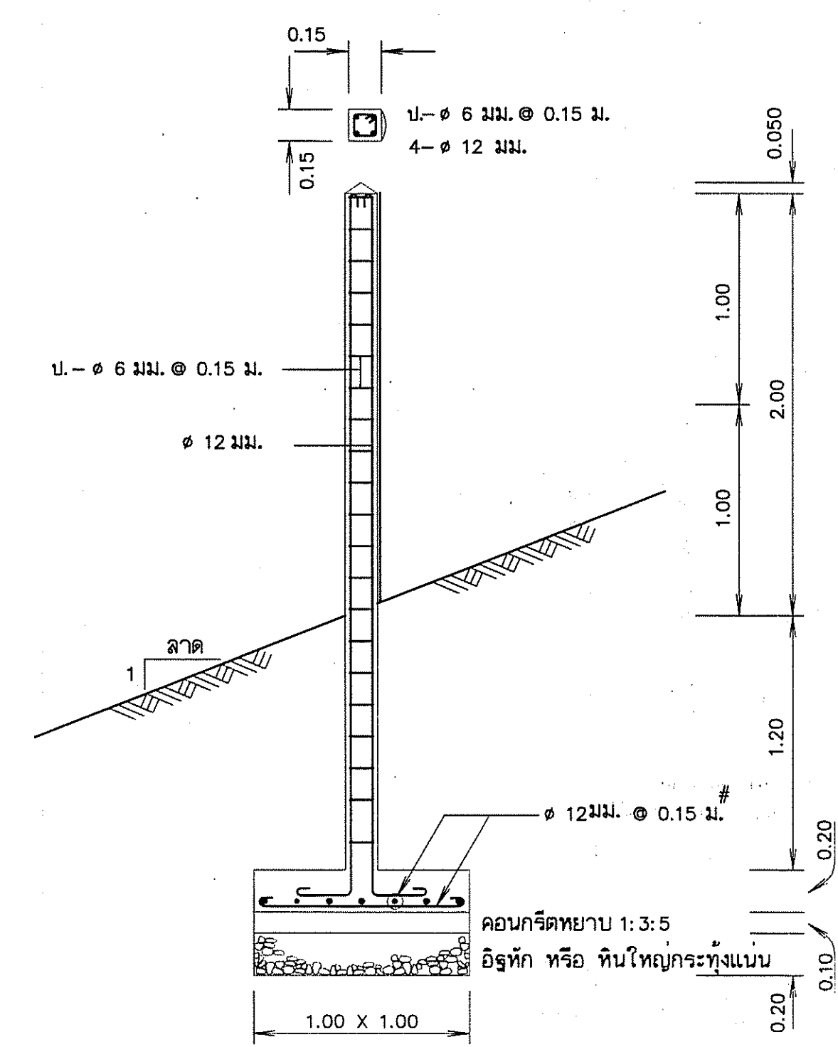
ขยายหลัก คสล.บอการค้าระดับ มาตรฐาน 1:25
