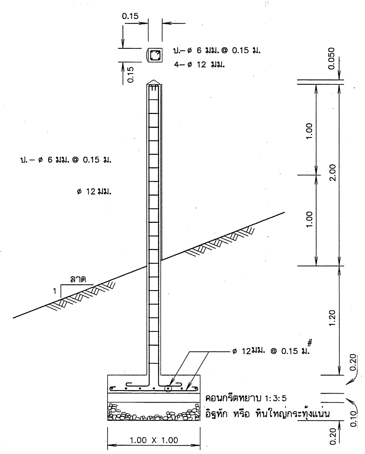
ขยายหลัก คสล.บอกระดับ มาตราส่วน 1:25
