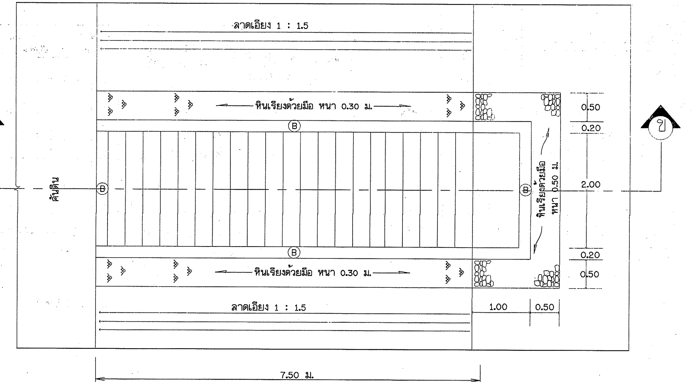
แปลนบ้านใด คสล. แบบไม่มีชานพัก
