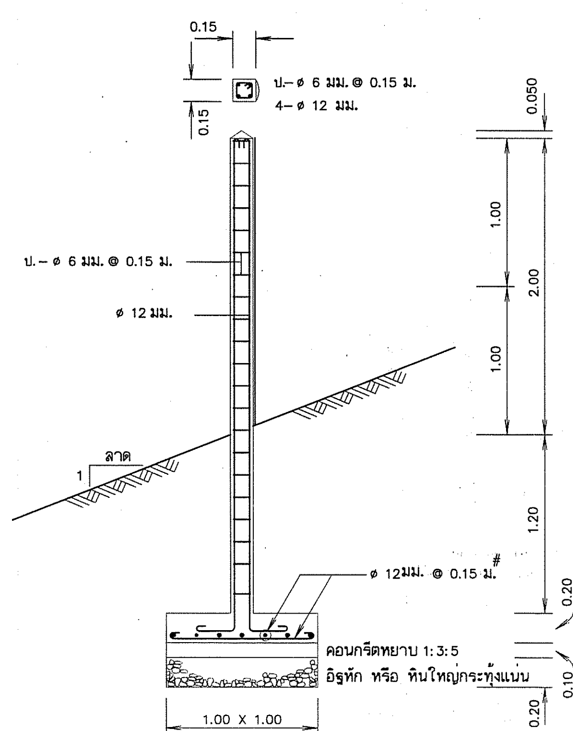
ขยายหลัก คสล.บอกระดับน้ำ มาตราส่วน 1:25
