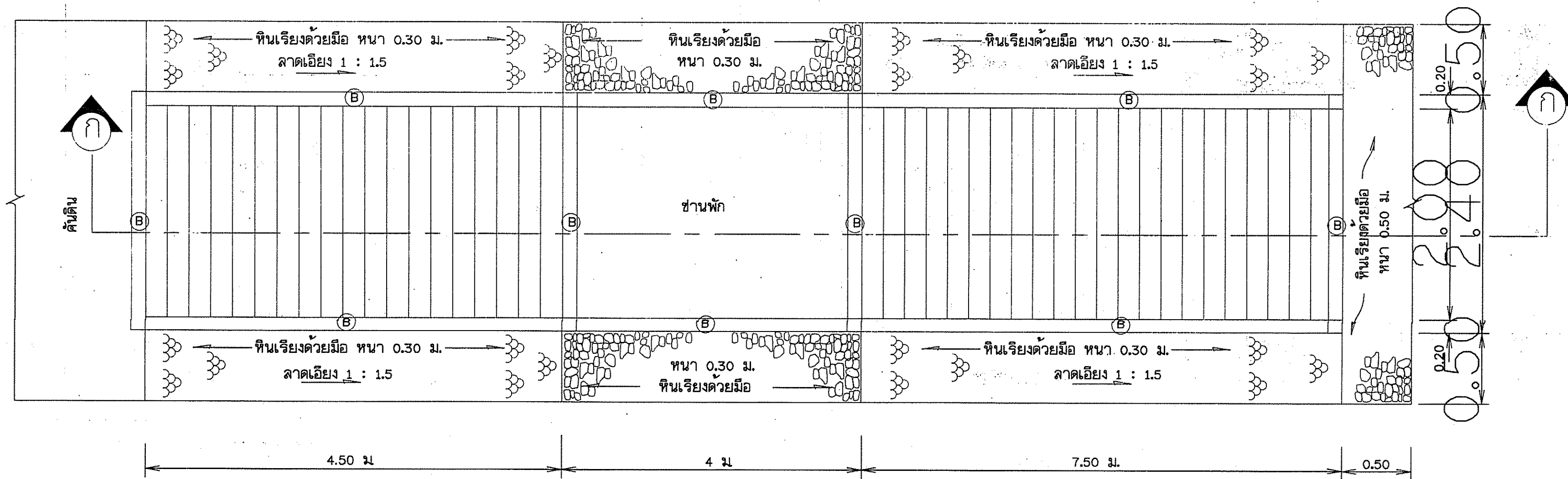
แปลนบ้านใด คสล. แบบมีชานพัก
