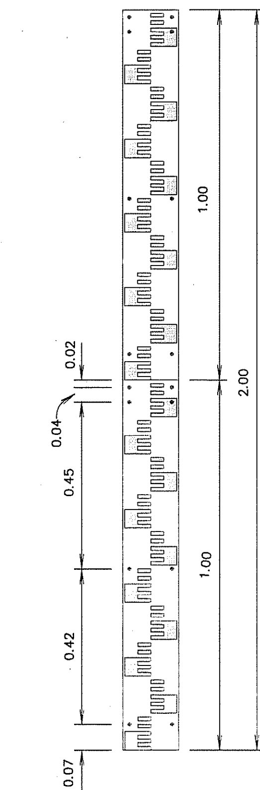
แผ่นเหล็กบอกระดับน้ำ มาตราส่วน 1:10
