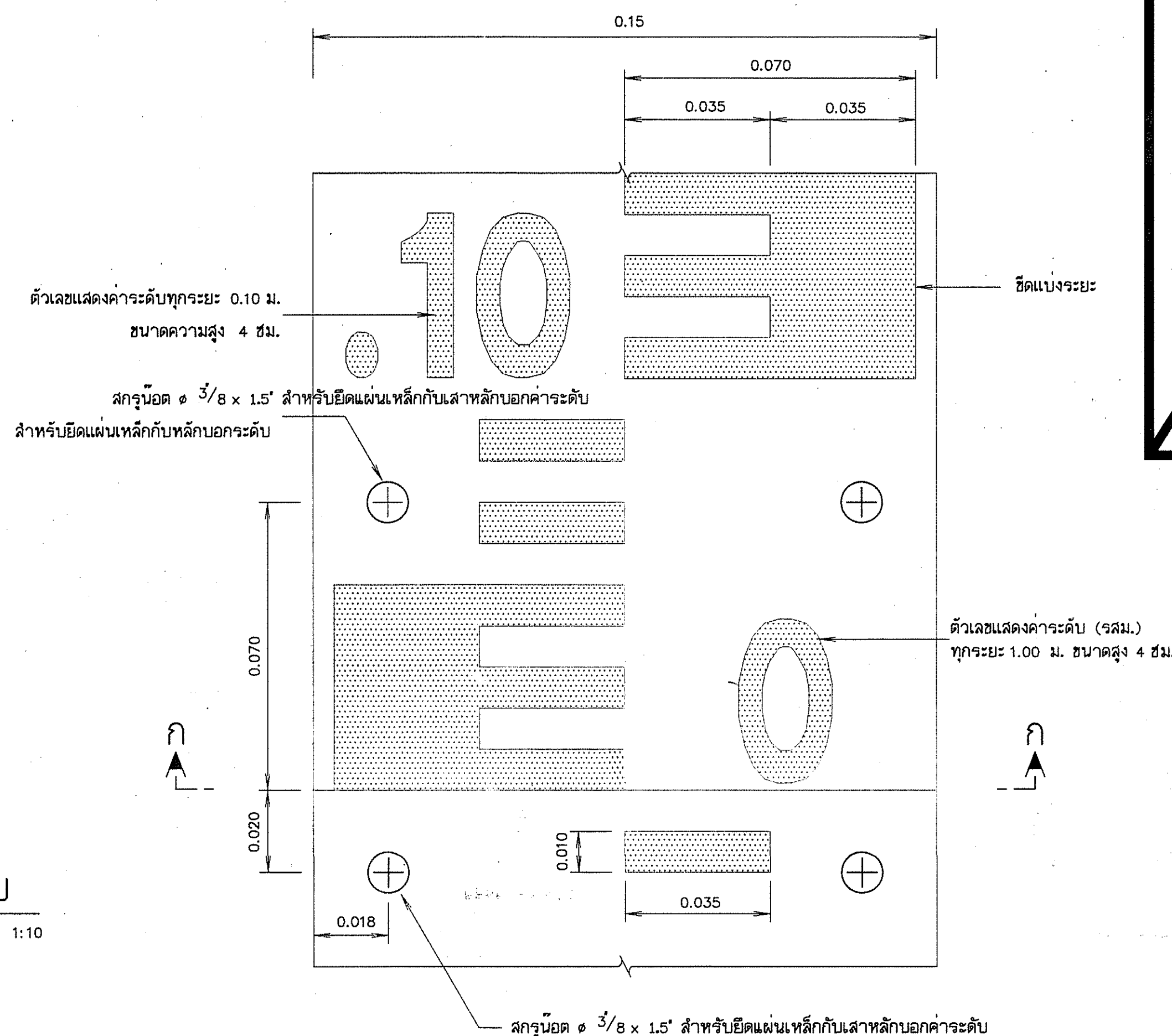
ขยายแผ่นเหล็กบอกระดับน้ำ มาตราส่วน 1:1
