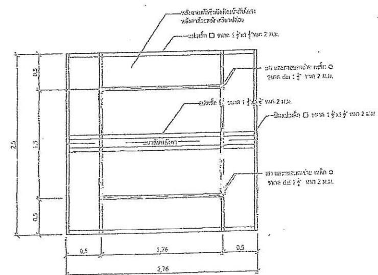
แปลนพื้น 1:25
