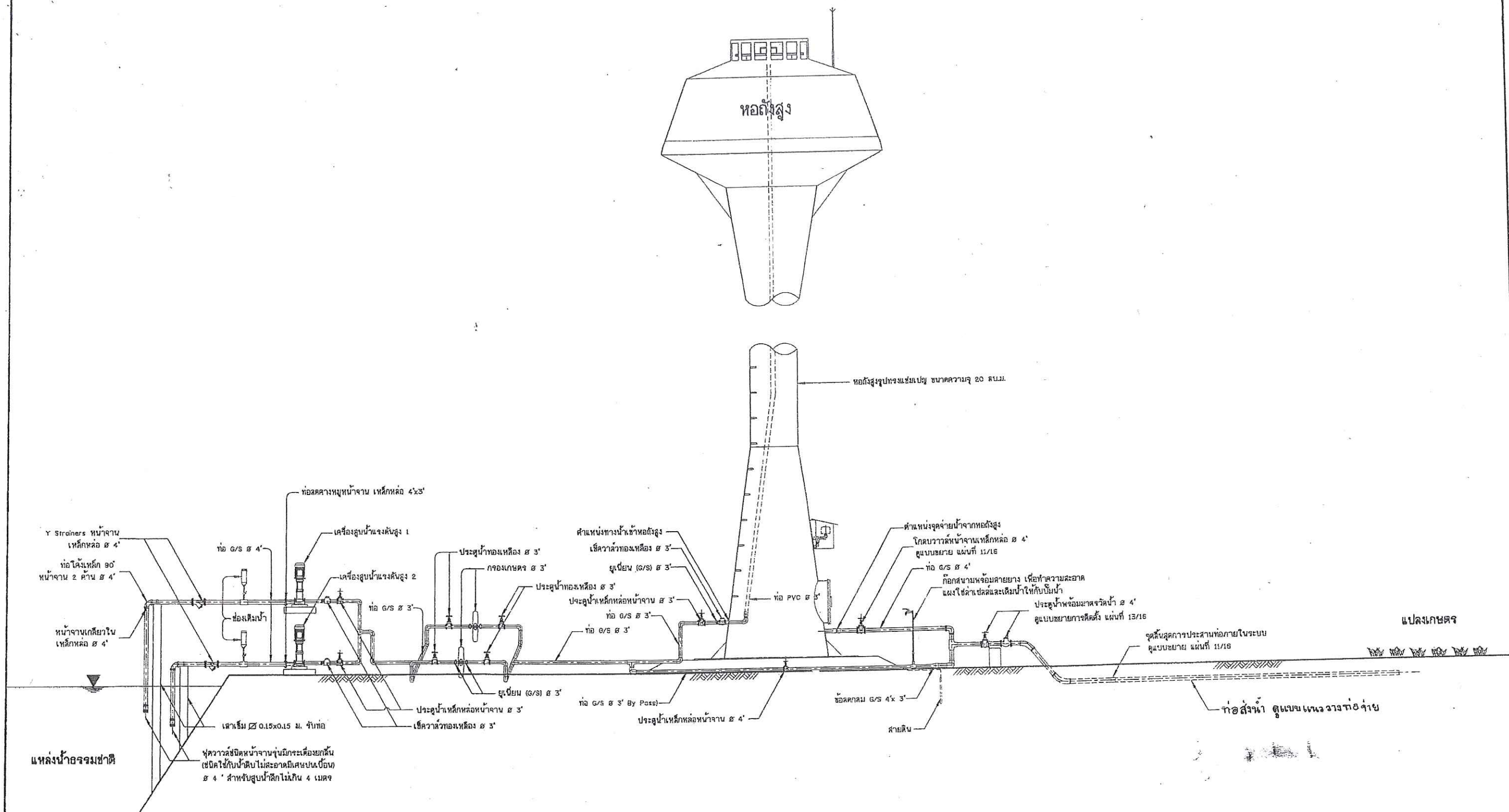
รูปแสดงรายละเอียดท่อและอุปกรณ์ระบบสูบน้ำพลังงานแสงอาทิตย์ ไม่แสดงขนาดส่วน
