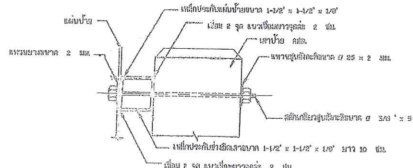
รูปทัศนียภาพการยึดแผ่นป้ายและเสา
