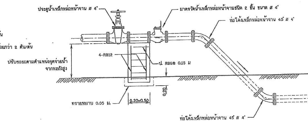
14. การติดตั้งมาตรวัดน้ำบนพื้นดิน ๕ 4"
