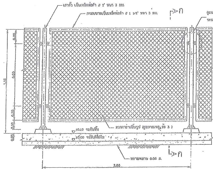
แบบขยายรั้วลดตายาย ไม่แสดงขนาดส่วน
