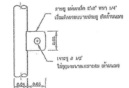
แบบขยายสายรัด ไม่แสดงขนาดส่วน
