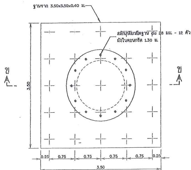
แปลน ฐานรากหล่อสูง (แบบเสาเข็ม)
