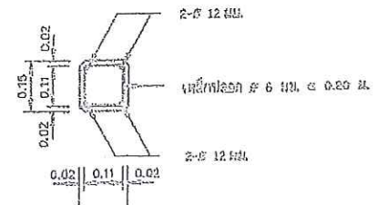
รูปตัด ก-ข โหนด และรอยร้าว
