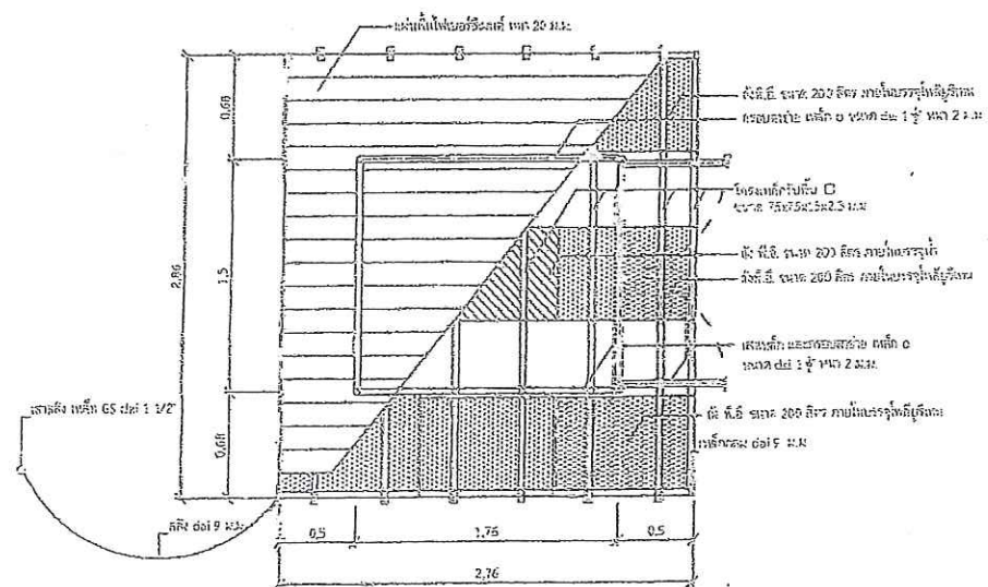
รูปด้านข้าง 1:25
