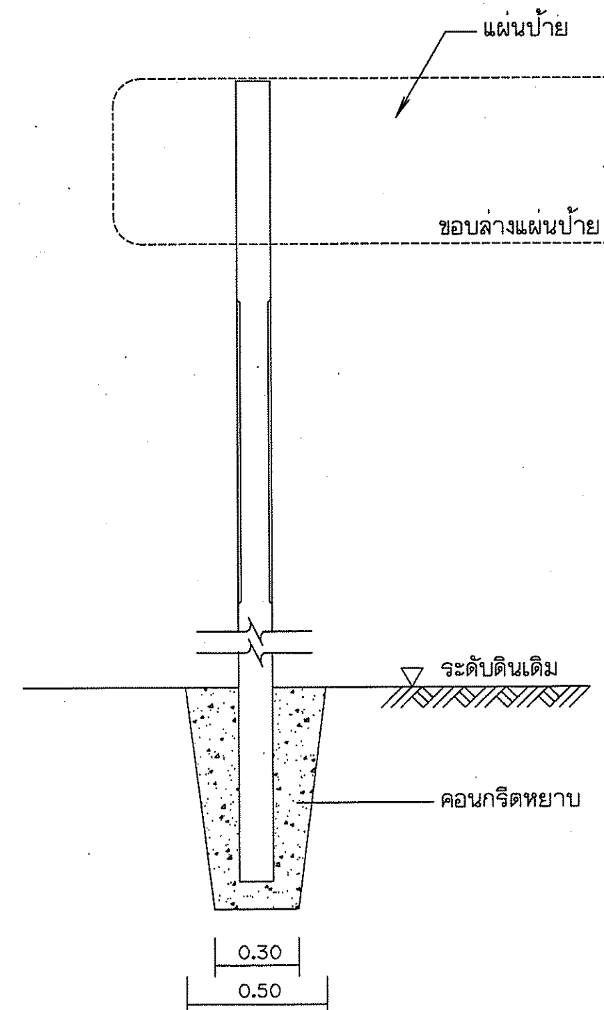
รายละเอียดการติดตั้งเสาป้าย มาตราส่วน 1:20
