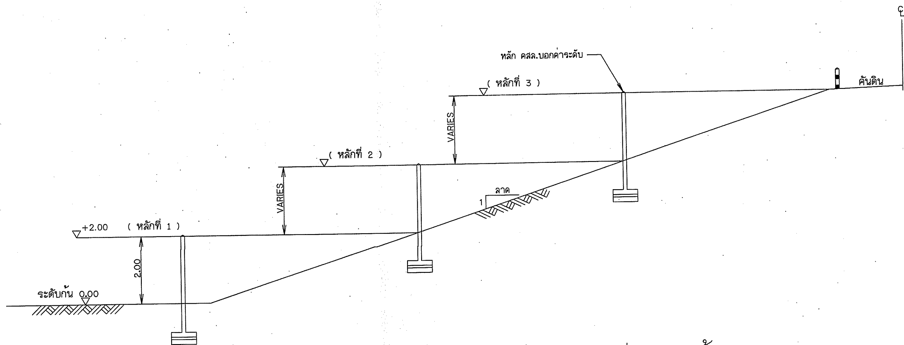
รูปตัดทั่วไปแสดงตำแหน่งหลักบอกระดับน้ำ
