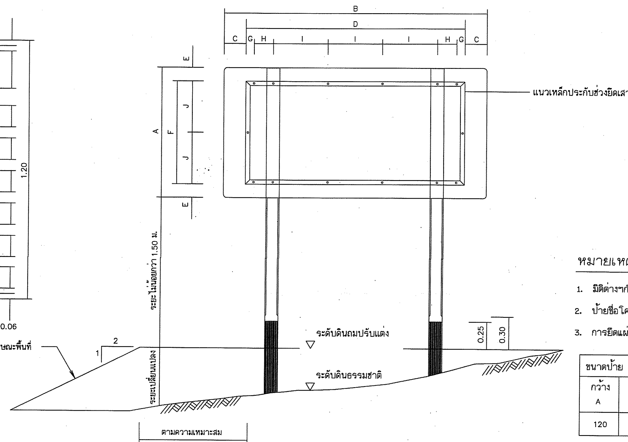
รูปแสดงการประกอบแผ่นป้าย มาตรฐาน 1:20
