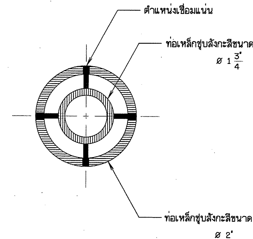
รูปตัด ข-ข
