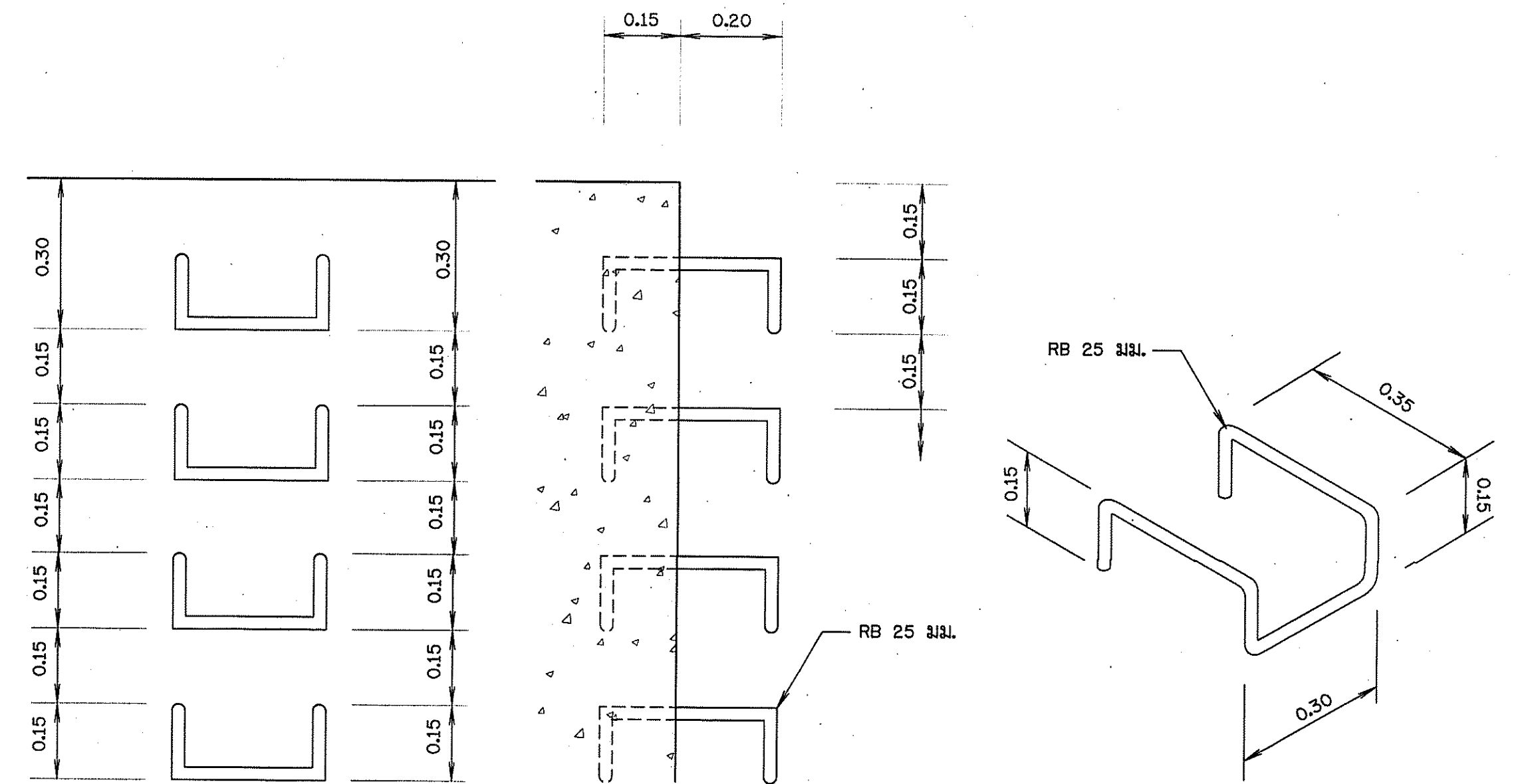
รูปขยายบันไดลิง
