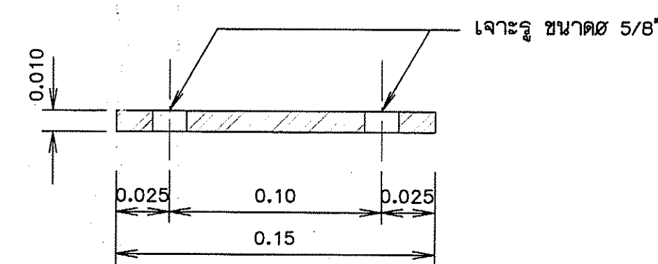
รูปตัด ค-ค
