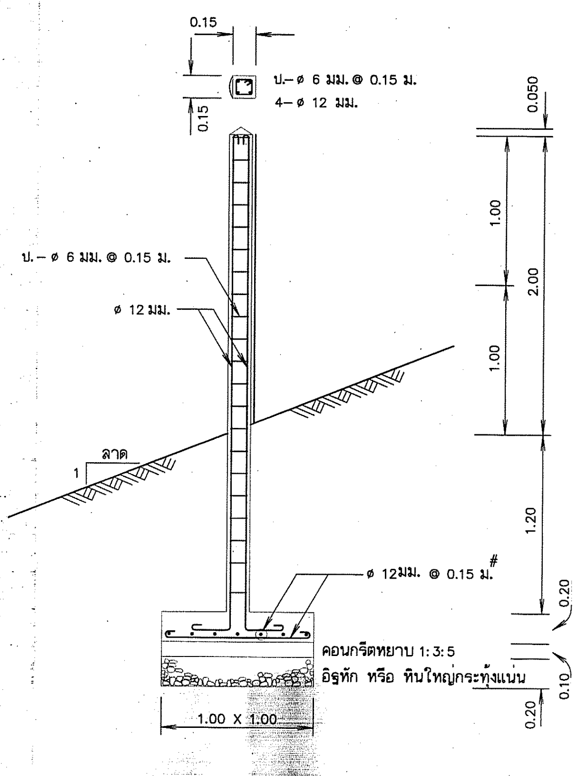
ขยายหลัก คสล.บอกระดับ
