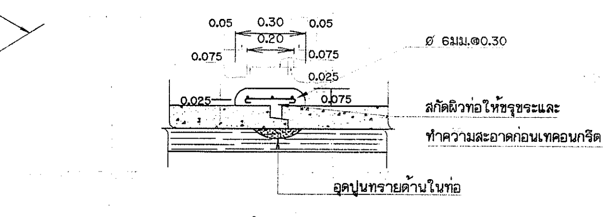
รูปตัด ข-ข ไม่แสดงมาตราส่วน
