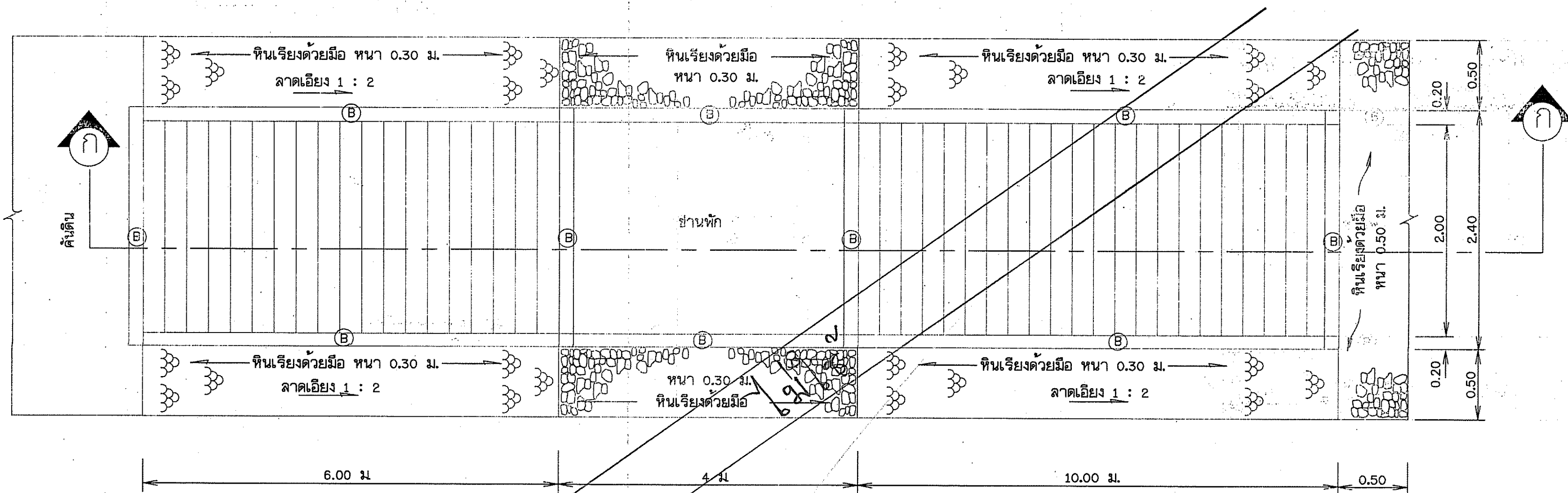
แบบบันได คสล. แบบมีชานพัก
