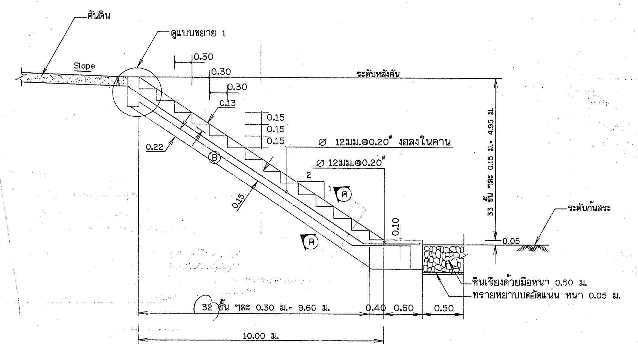
รูปตัด ข - ข
