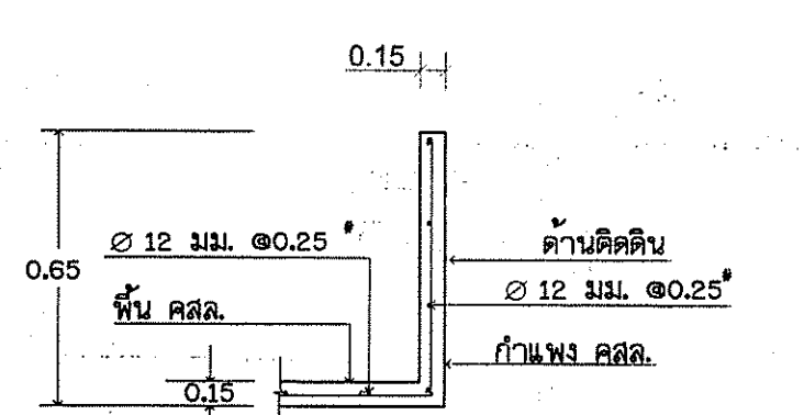
รูปตัด ค-ค (ความหนาพื้น 0.15 ม.) ไม่แสดงมาตราส่วน
