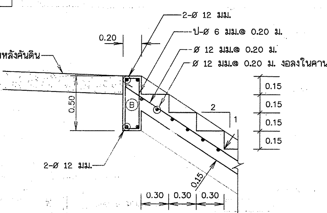
รูปขยาย 1
