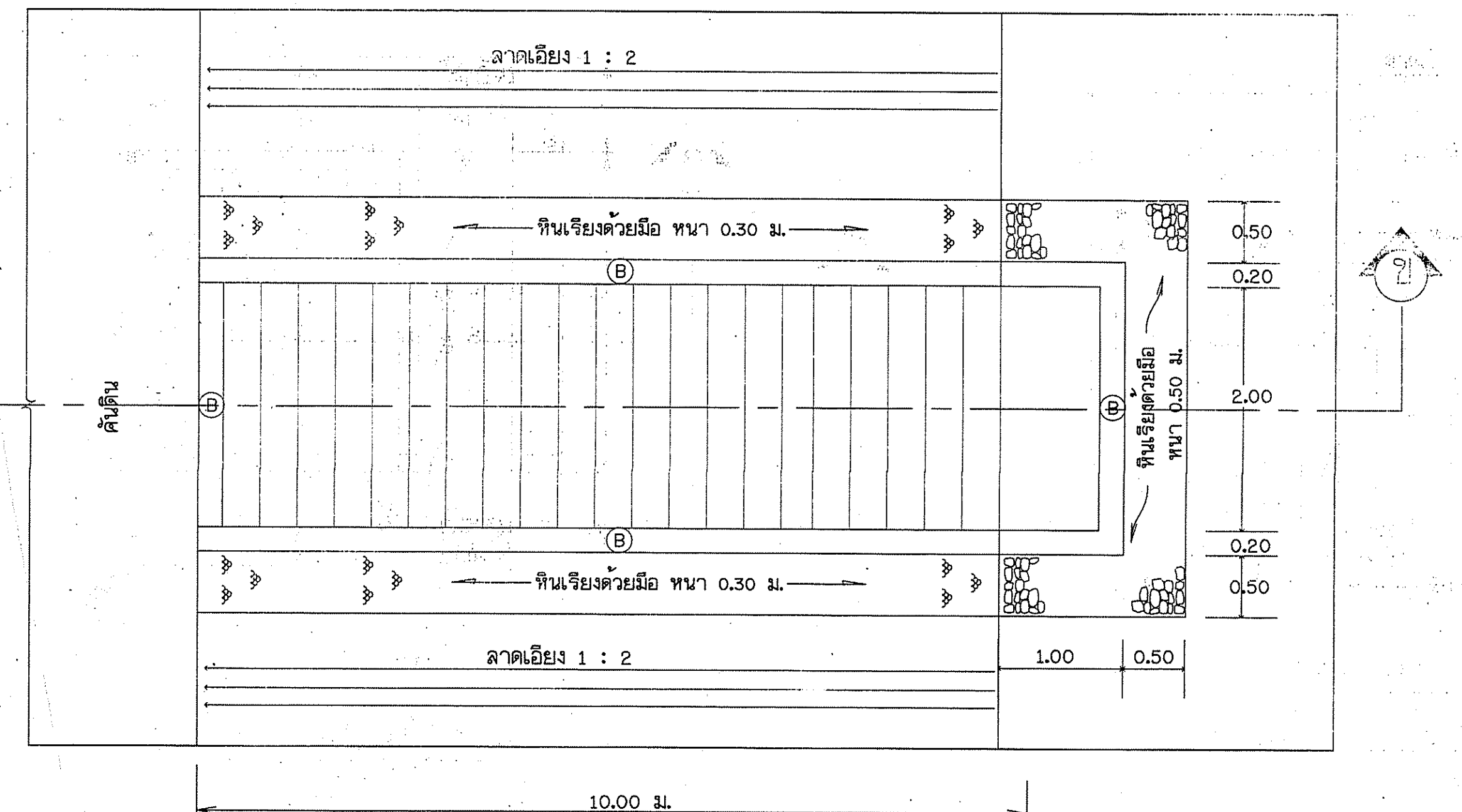
แบบบันได คสล. แบบไม่มีชานพัก
