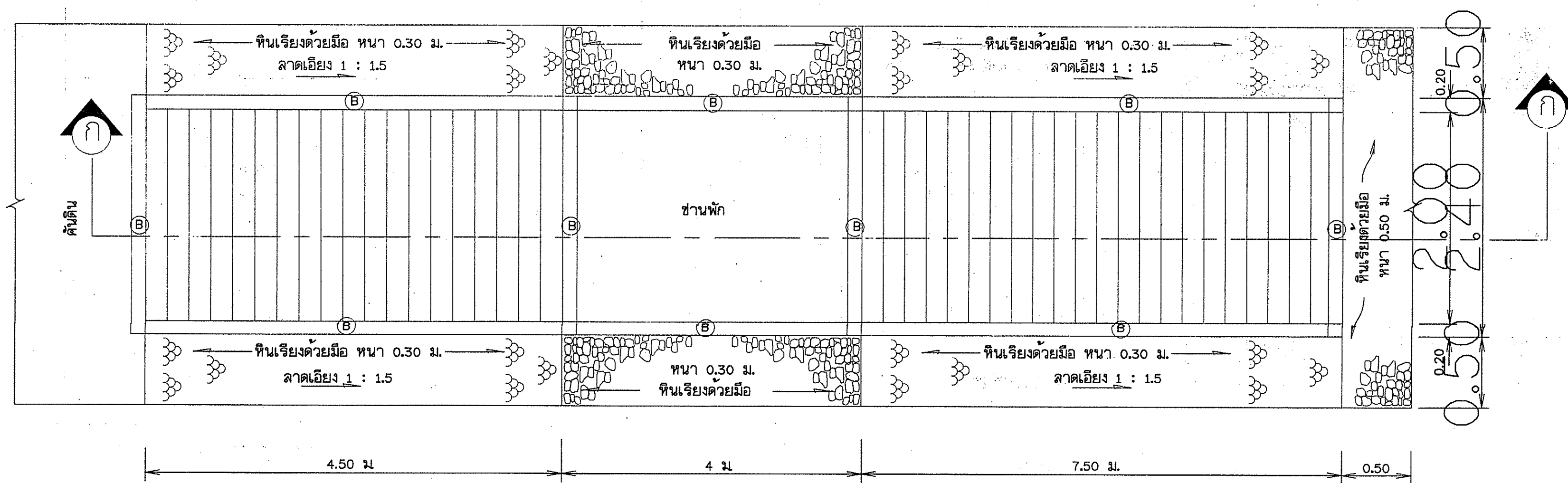
แปลนบ้านโต คสล. แบบมีชันพัก
