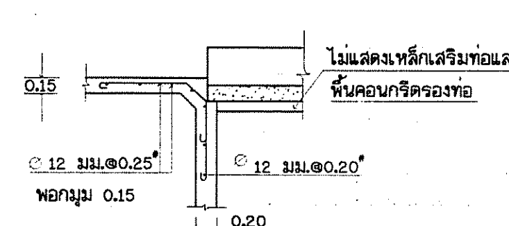
ขยาย ๔ ไม่แสดงมาตราส่วน
