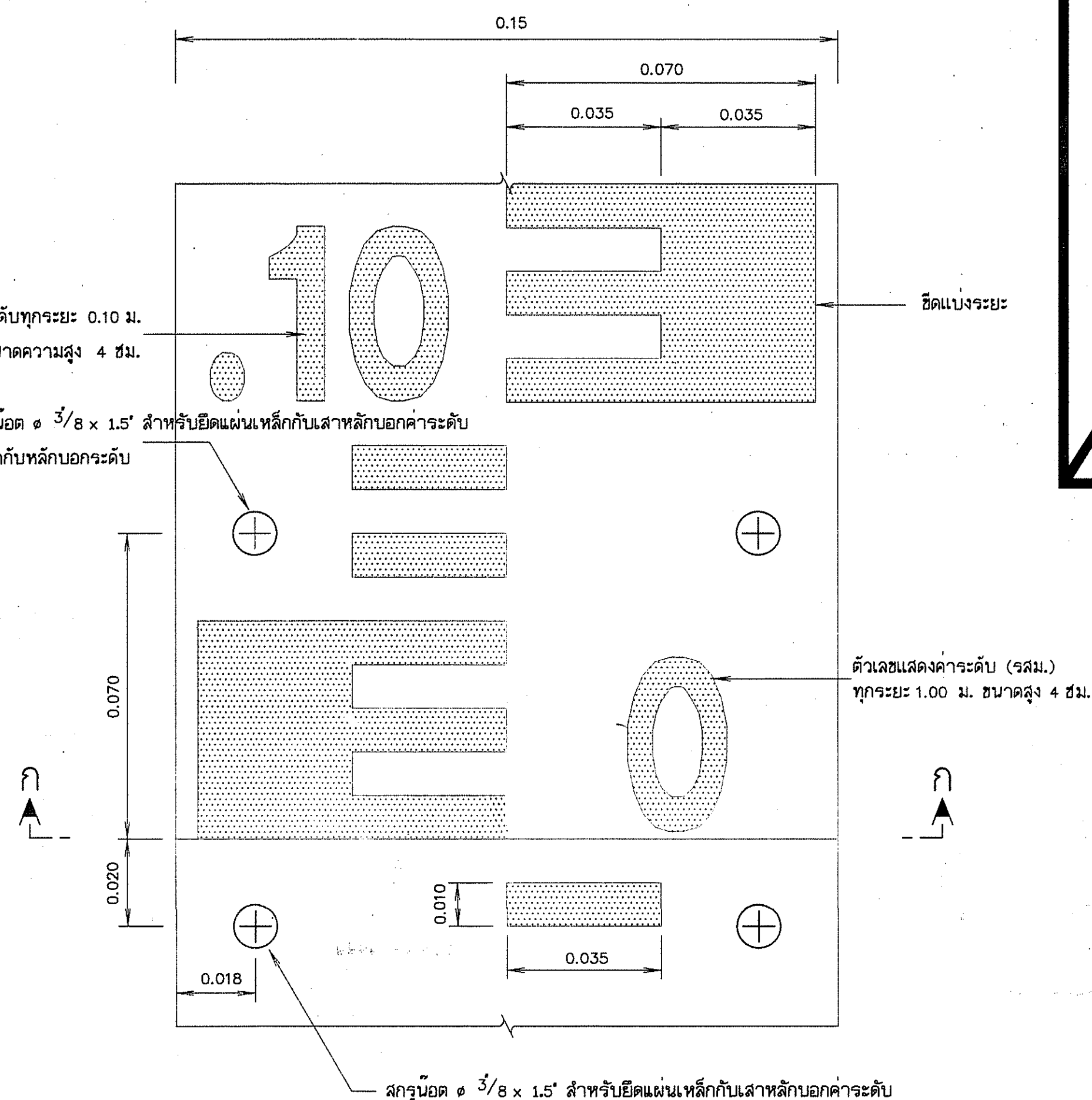
ขยายแผ่นเหล็กบอการค้าระดับ มาตราส่วน 1:1
