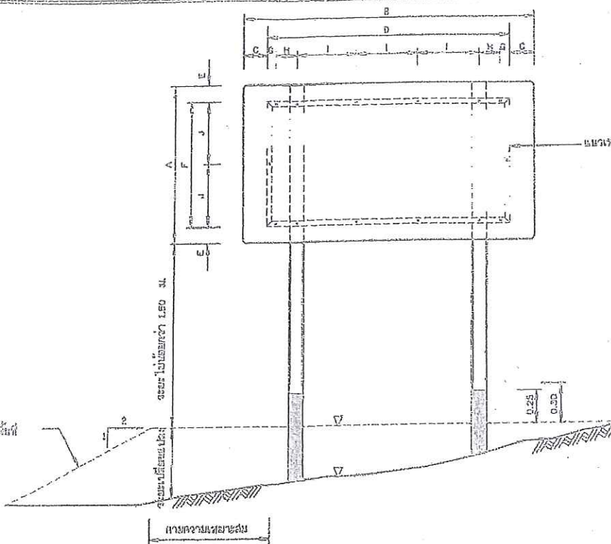
รูปแสดงการประกอบแผ่นป้าย ไม่แสดงขนาดส่วน
