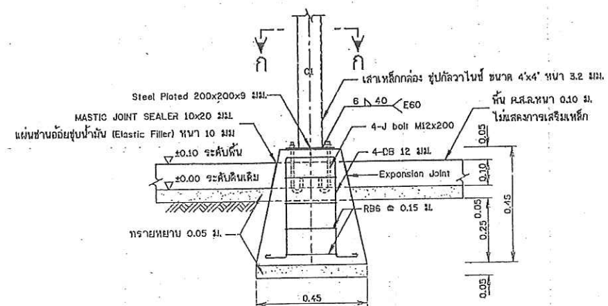
รูปขยายฐานรากโครงสร้างรับแผง F1 (ต่อเนื่อง คสล. หล่อสำเร็จรูปพร้อมติดตั้ง)
