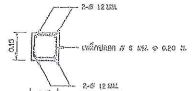
รูปตัด ก-ก ไม่แสดงขนาดส่วน
