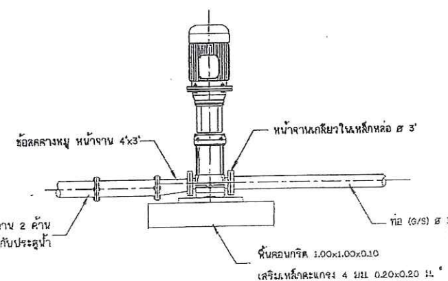
15. การต่อท่อเครื่องสูบน้ำ
