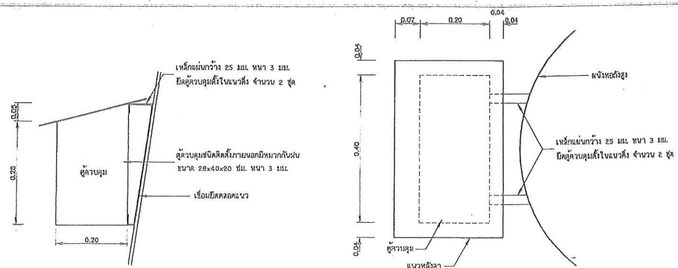
แบบขยายตัววัด ไม่แสดงมาตราส่วน
