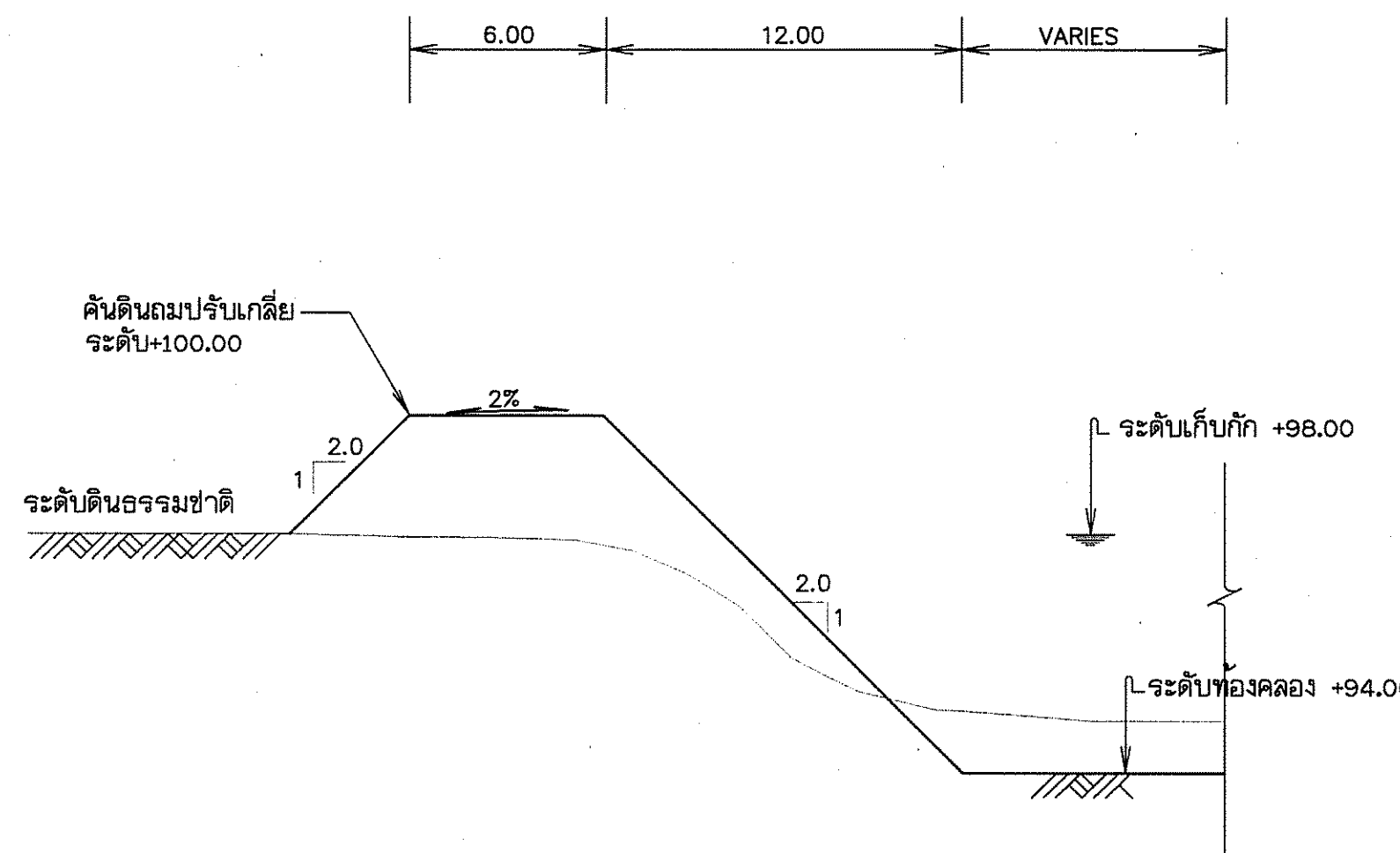
รูปตัดทั่วไป
