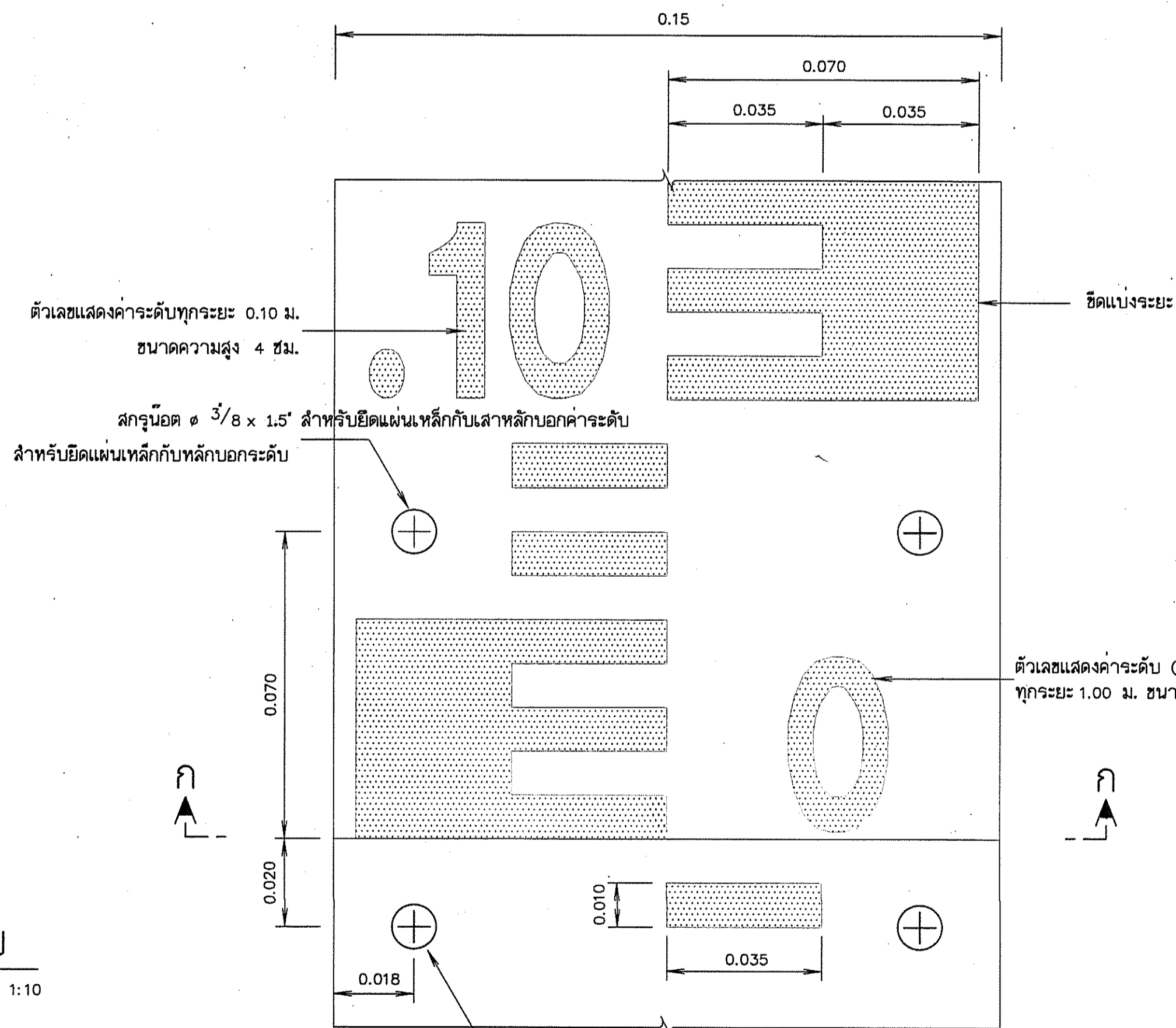
แผ่นเหล็กบอกระดับ
