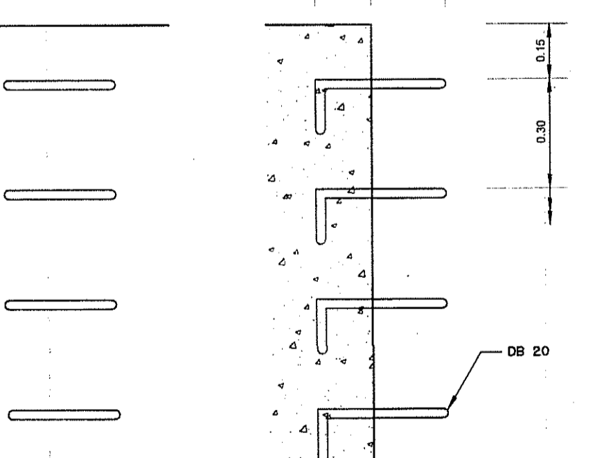
รูปขยายบันไดลิง ไม่แสดงมาตราส่วน
