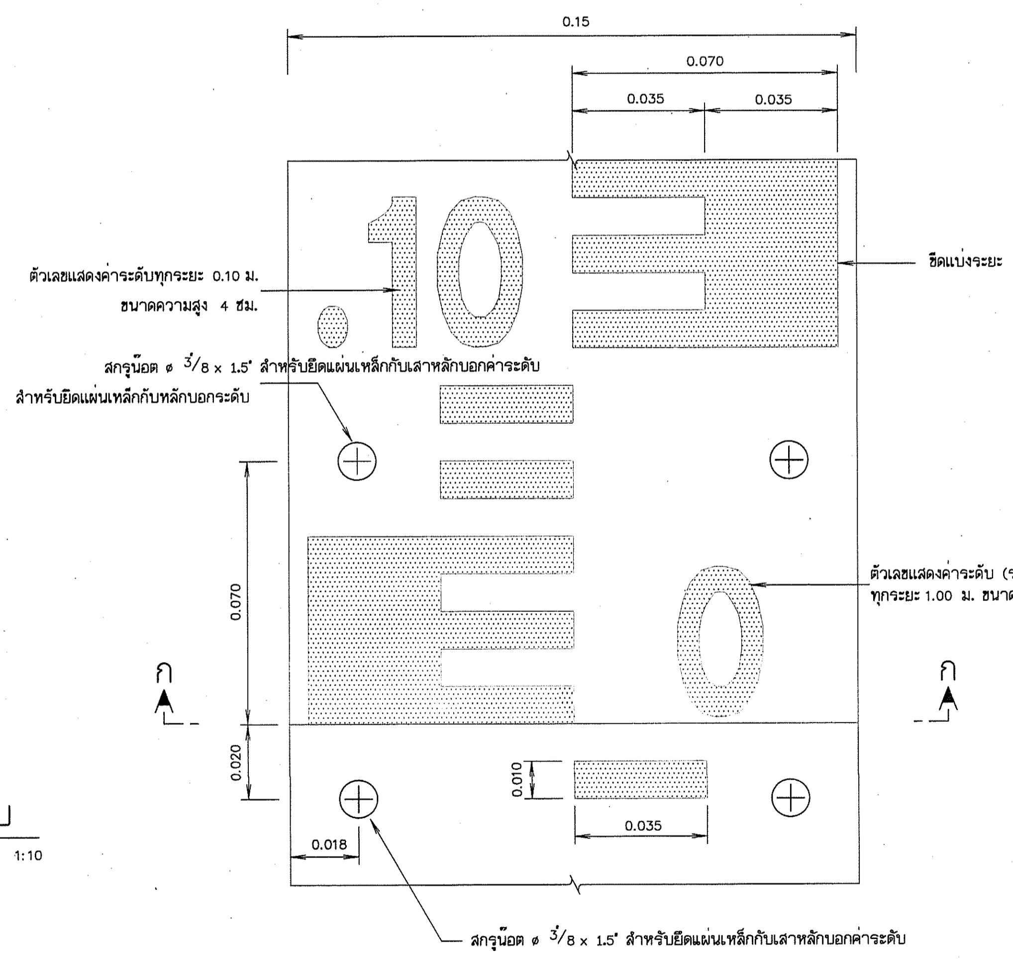
ขยายแผนเหล็กบอการค้าระดับ มาตรฐาน 1:1
