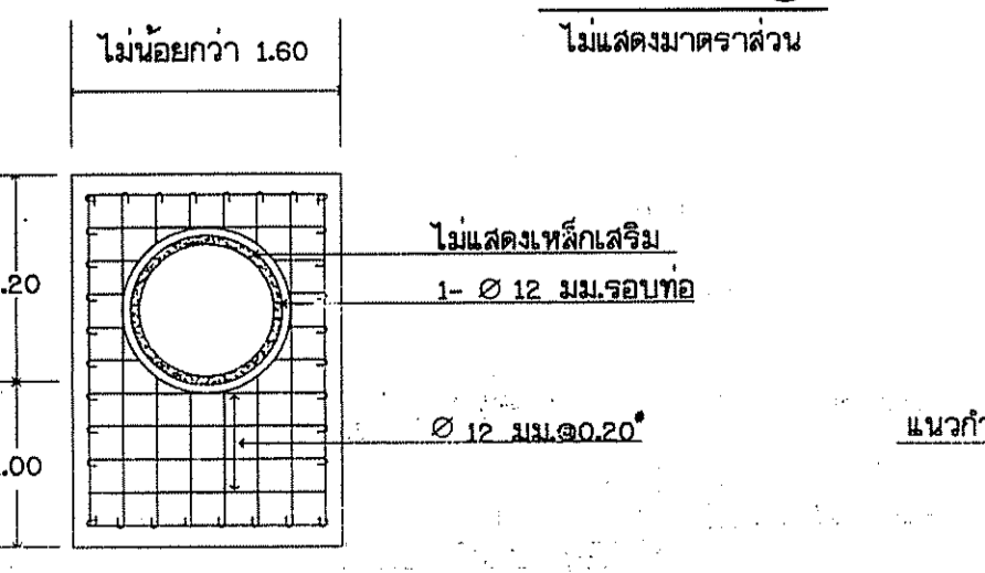
ขยายการเสริมเหล็กกำแพงปากท่อและท้ายท่อ (HEAD WALLS) ไม่แสดงมาตราส่วน
