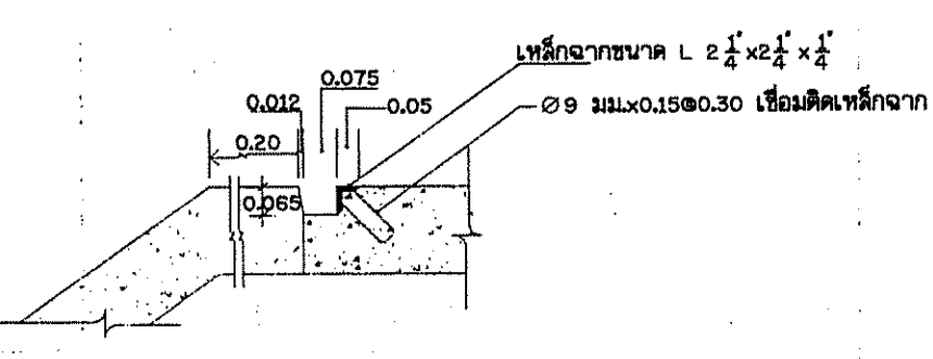
รูปขยายร่องใส่บานประตูไม้ ไม่แสดงมาตราส่วน
