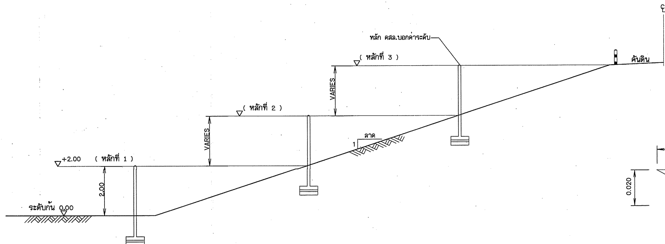
รูปตัดทั่วไปแสดงตำแหน่งหลักบอการค้าระดับน้ำ มาตรฐาน 1:100
