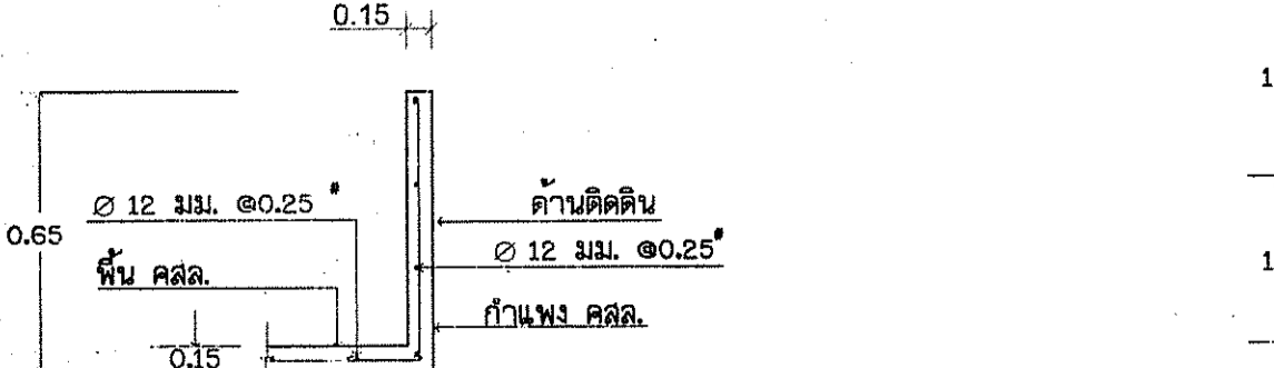
รูปตัด ค-ค (ความหนาพื้น 0.15 ม.) ไม่แสดงมาตราส่วน
