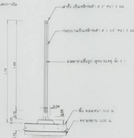
รูปตัด ก-ก โมเดลมาตรฐาน
