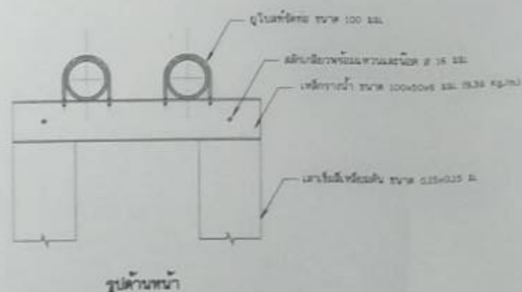
13. เสาติดอม่อรับท่อนุด และแบบขยายอุปกรณ์รัดท่อ
