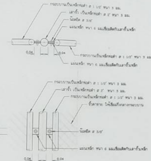
แบบขยายรายละเอียดแสดงการยึดระหว่างรั้วกับเสา โมเดลมาตรฐาน
