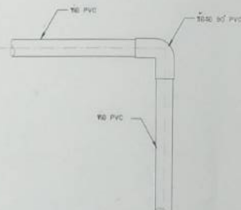
7. แบบการต่อข้ออ 90° PVC ในเขตมาตรฐาน
