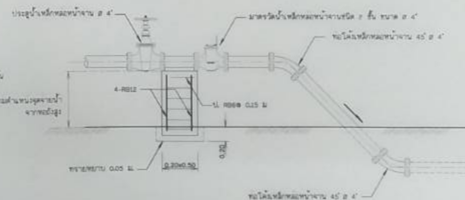
14. การติดตั้งมาตรวัดน้ำบนพื้นดิน ๕ 4'
