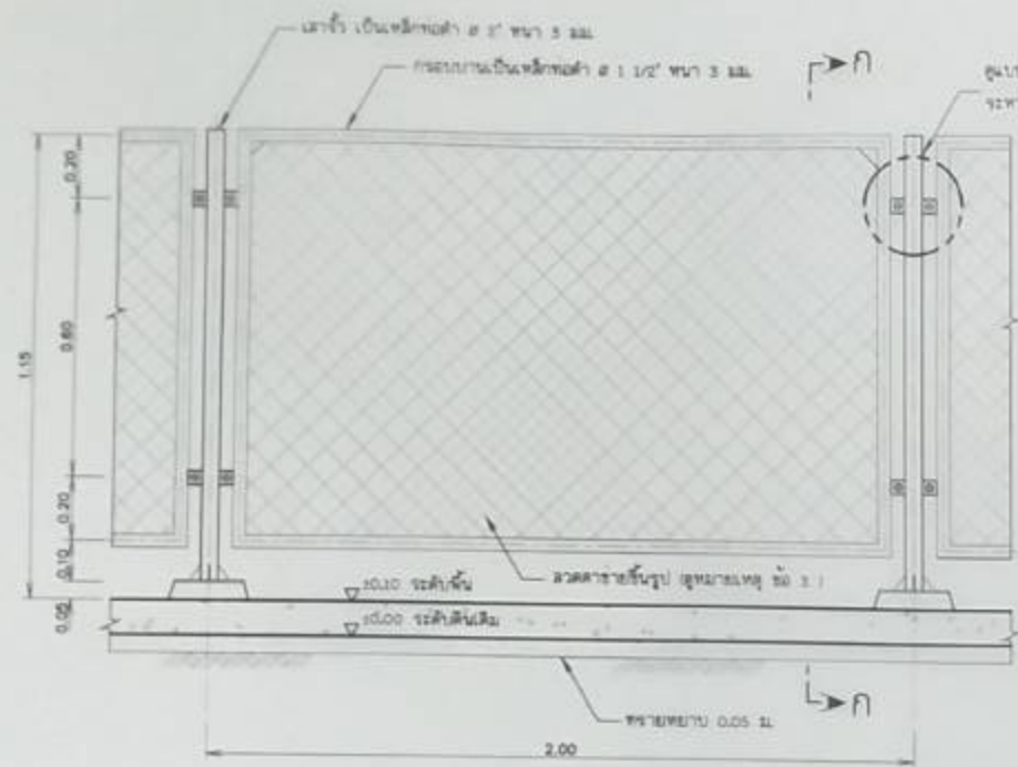
แบบขยายรั้วลวดตาข่าย โมเดลมาตรฐาน
