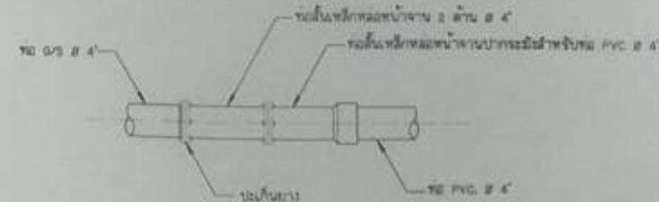
8. การบรรจุท่อเหล็กอาบสังกะสี G/S กับท่อ PVC. ในเขตมาตรฐาน
