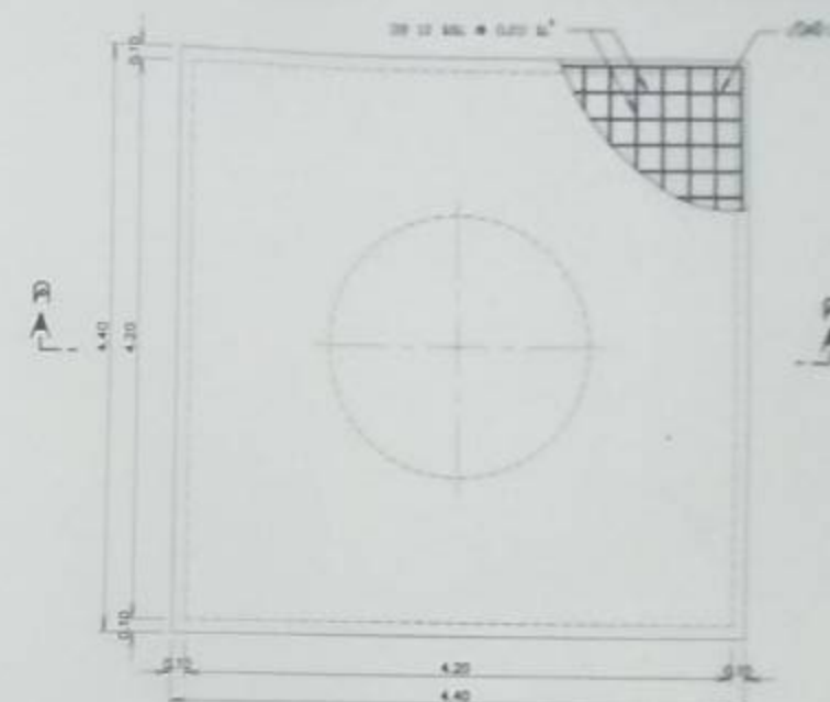
แป้นพื้นคอนกรีตเสริมเหล็ก
