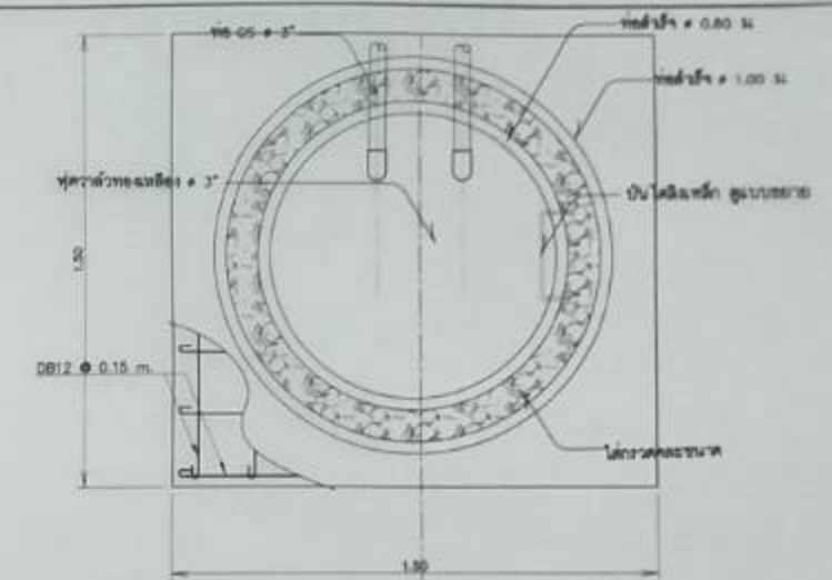
แปดนอาคารบอกรองน้ำดิบ คสล
