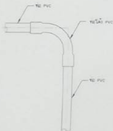
6. แบบการต่อข้อโค้ง 90° PVC ในเขตมาตรฐาน
