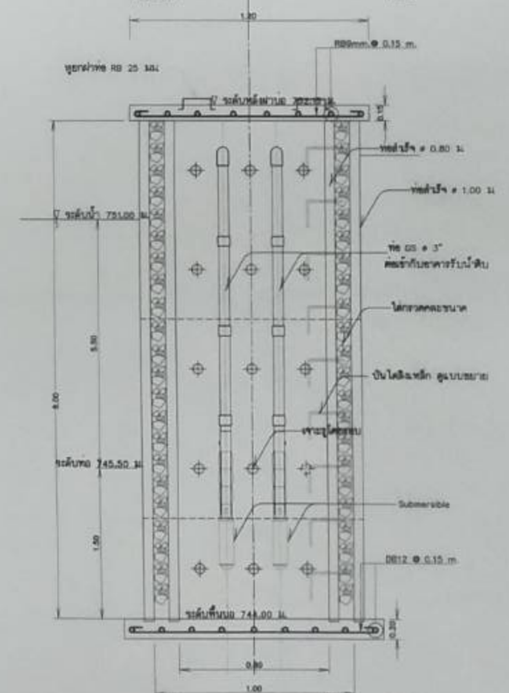
แปดนอาคารบอกรองน้ำดิบ คสล
