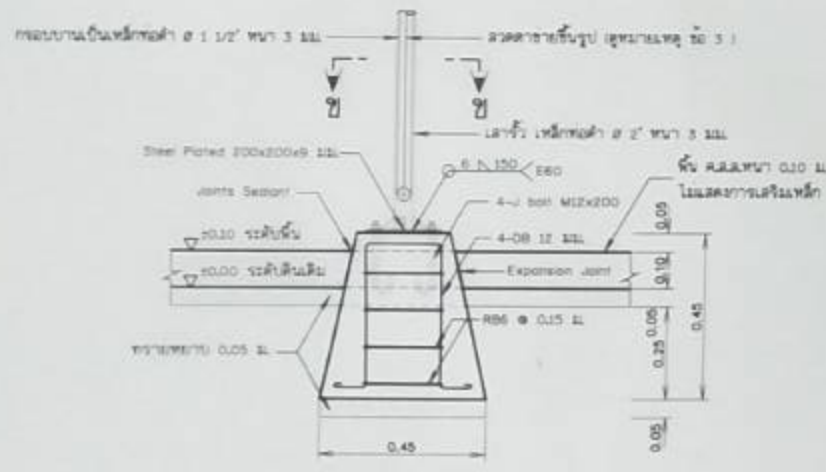
รูปขยายฐานรากโครงสร้างรับแผง F1 (ตาม ค.ส.พ. หรือสำหรับรูปหล่อเหล็ก) โมเดลมาตรฐาน
