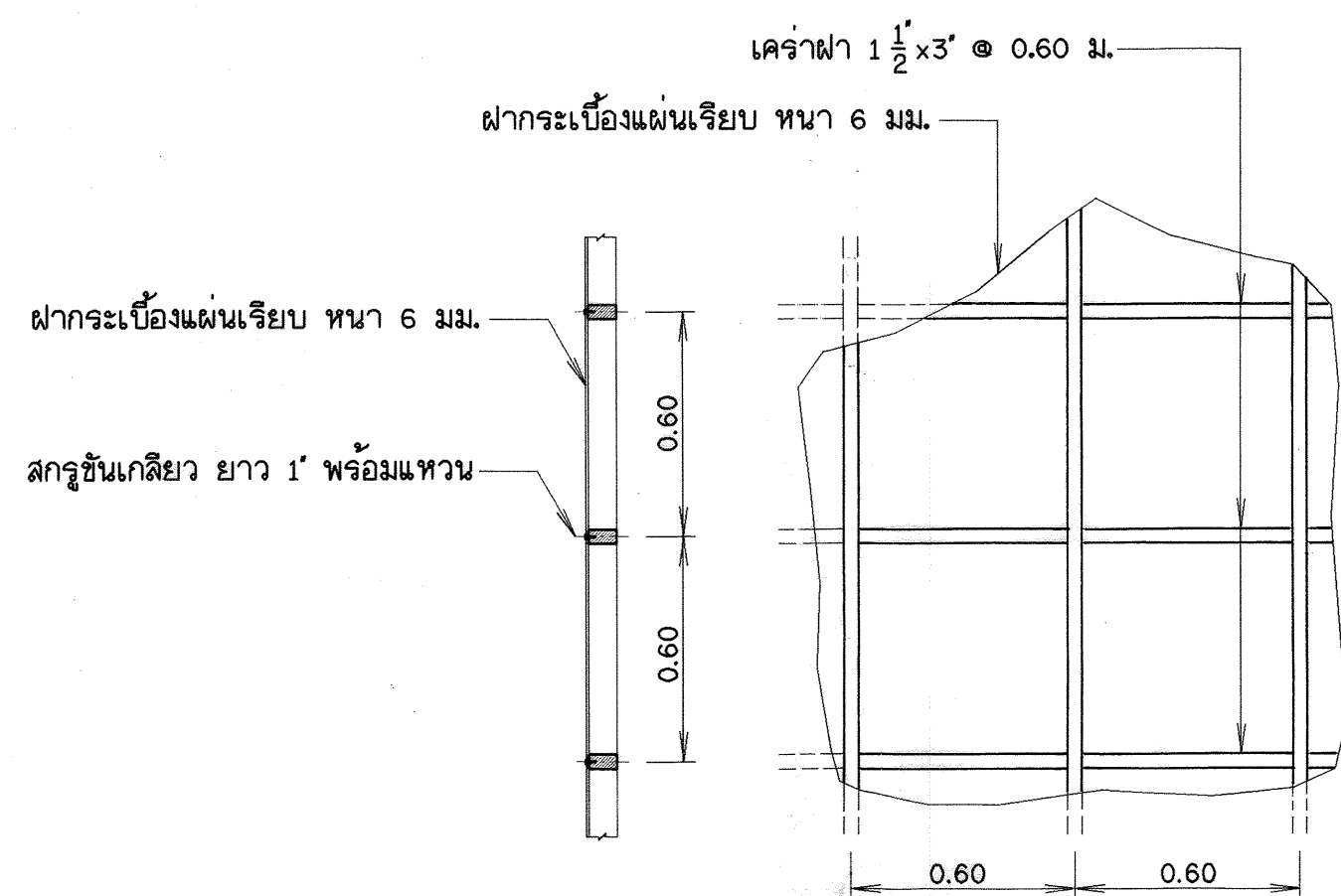
รูปชยายแคร่ , ฝา มาตราส่วน 1:20
