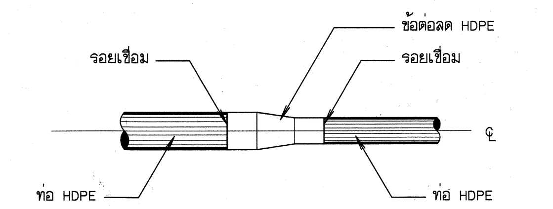
การบรรจุท่อ HDPE กับข้อต่อท่อ HDPE
