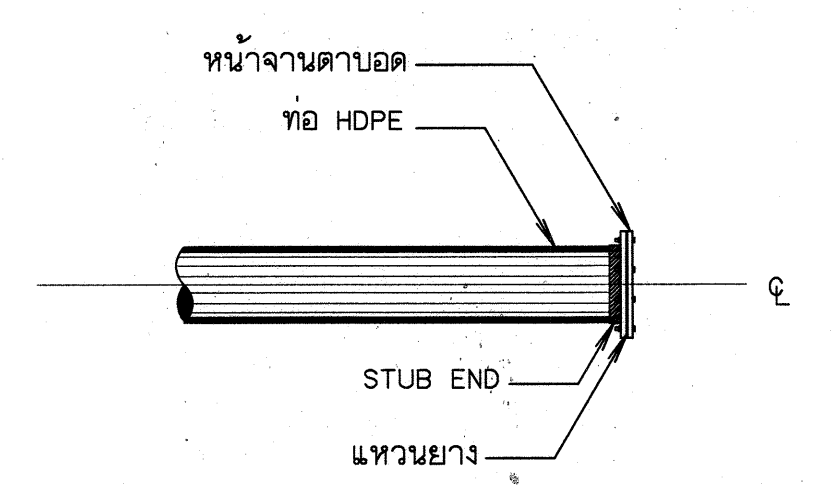
การปิดปลายท่อ
