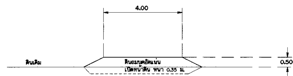
รูปตัดทางลำลอง
