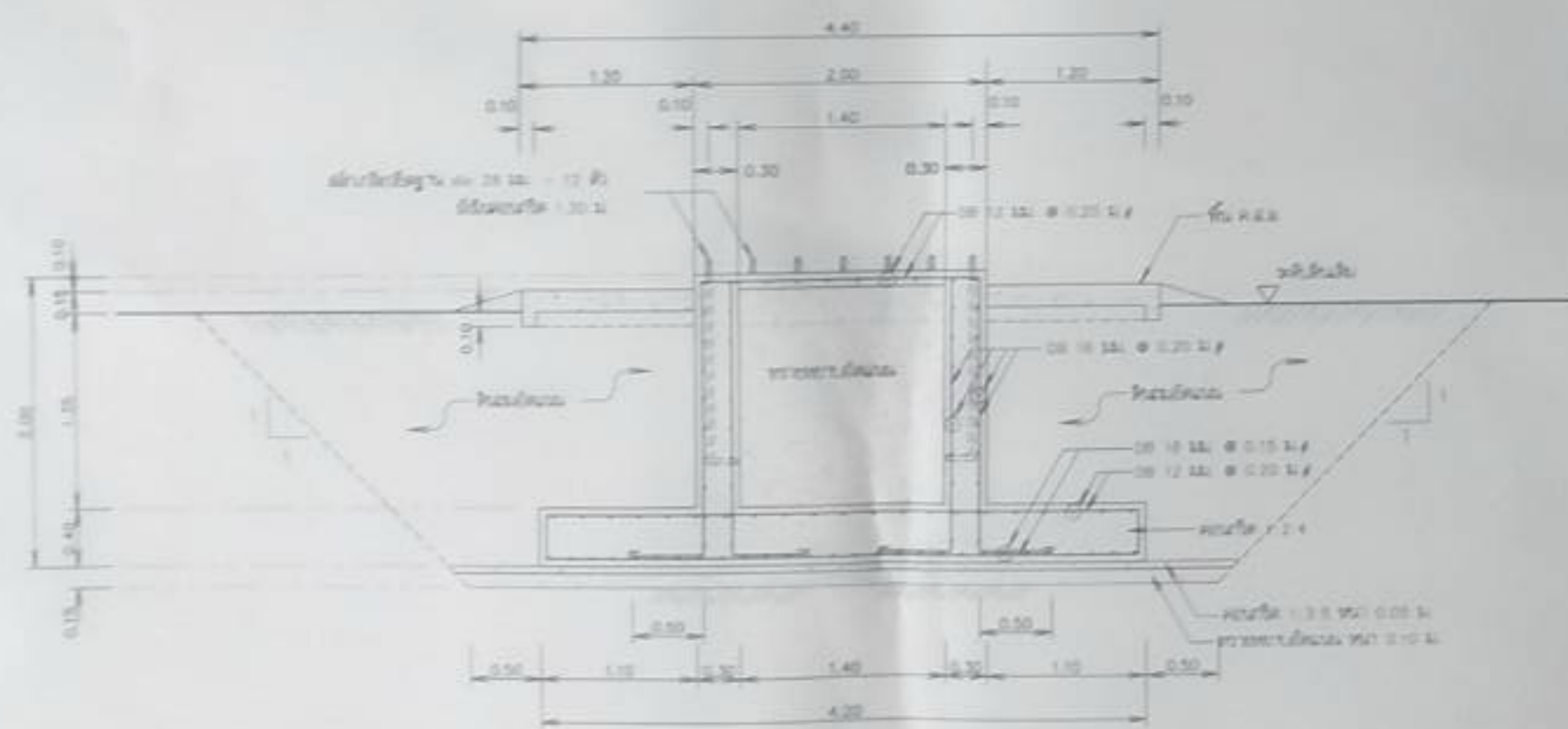
รูปตัด ก-ก
