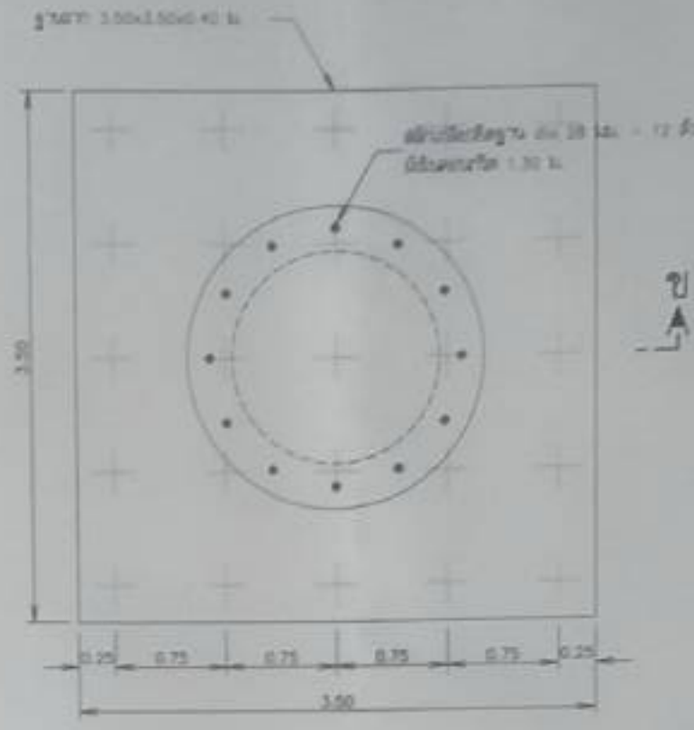
แปลน ฐานรากหอดังสูง (แบบเสาเข็ม)
