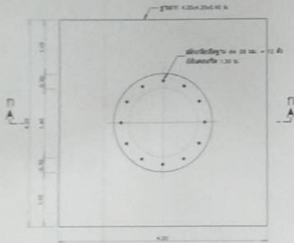
ฐานรากหอดึงสูง (แบบฐานแฉก)
