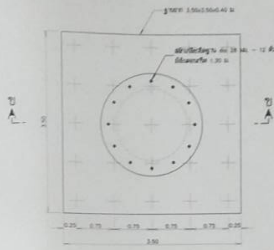
ฐานรากหอดึงสูง (แบบเสาเข็ม)
