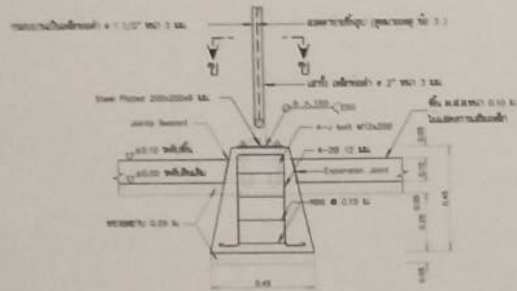
รูปขยายฐานรากโครงสร้างรับแรง F1
