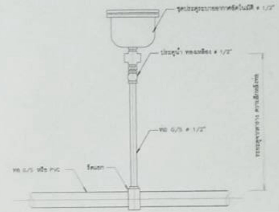
12. การติดตั้งประตูระบายอากาศอัตโนมัติ
