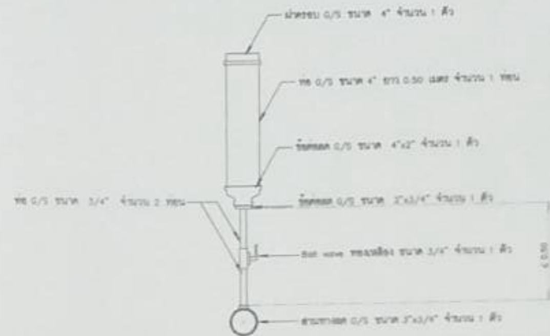
11. ช่องเติมน้ำ Inlet Water
