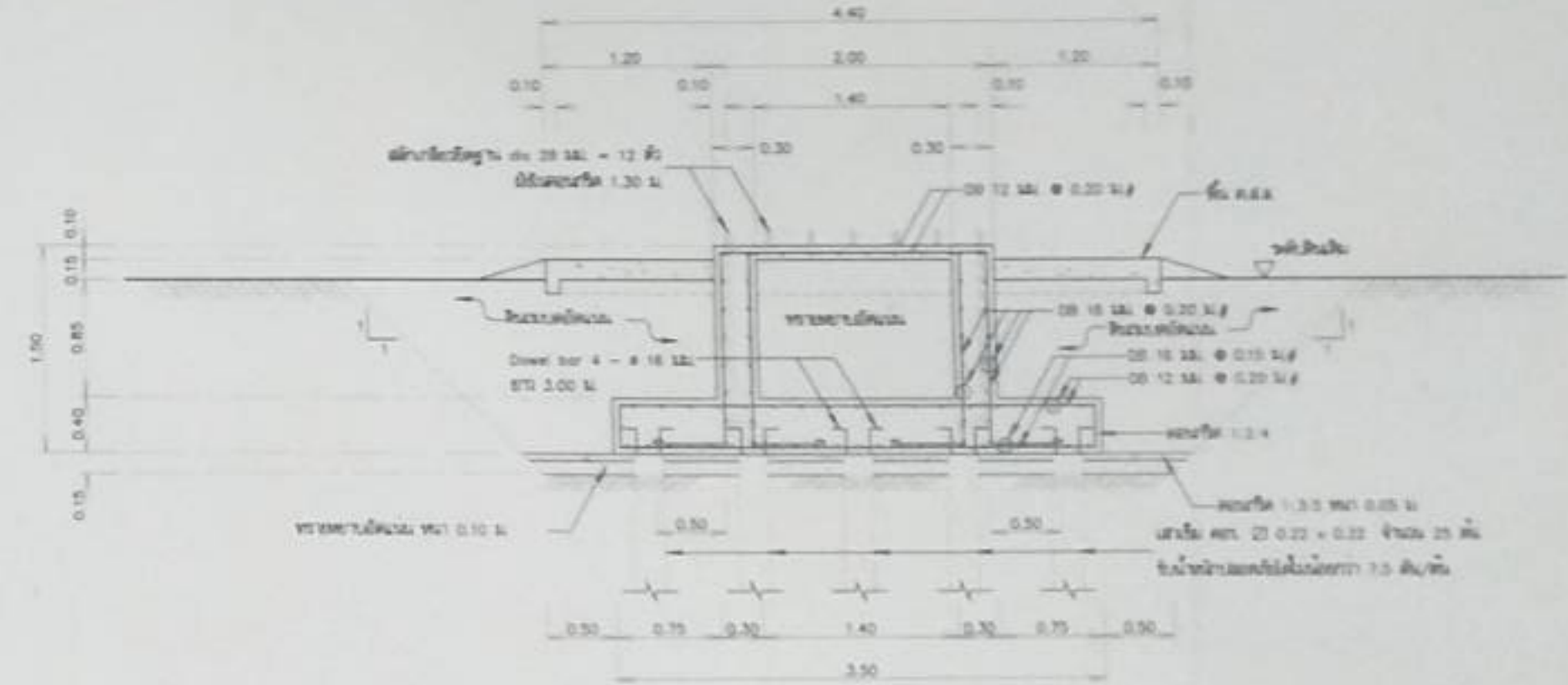
รูปตัด ข-ข
