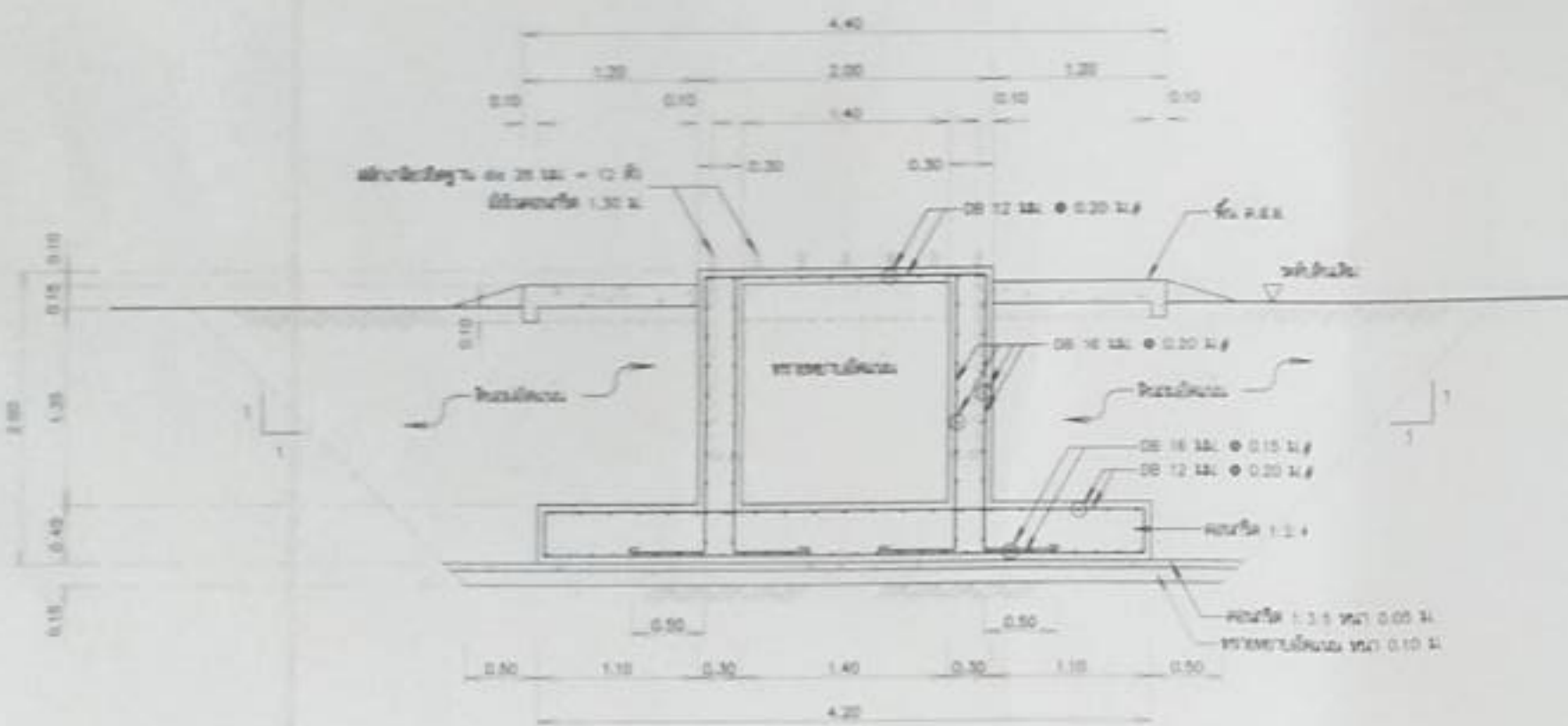
รูปตัด ก-ก
