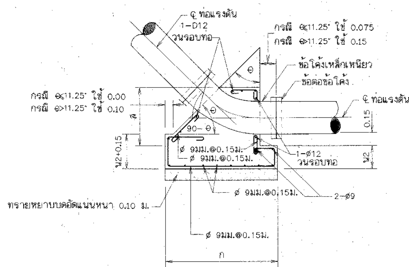
รูปตัด ๓-๓
