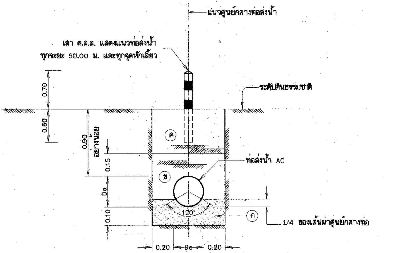
รูปตัดขวางการฝังท่อซีเมนต์ใยหิน (ท่อAC) ไม่แสดงมาตราส่วน
