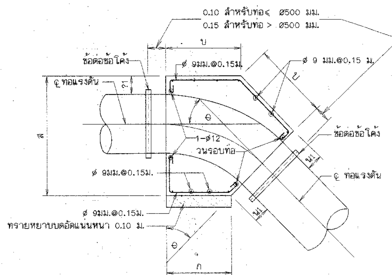
รูปตัด ๓-๓
