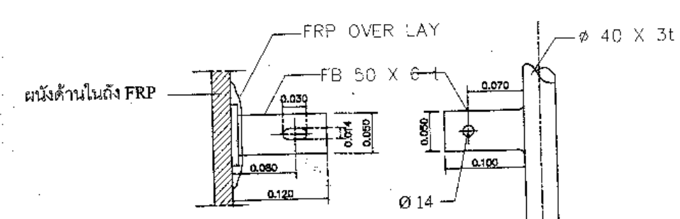
DETAIL A (ขี้คั่นใบโค)
