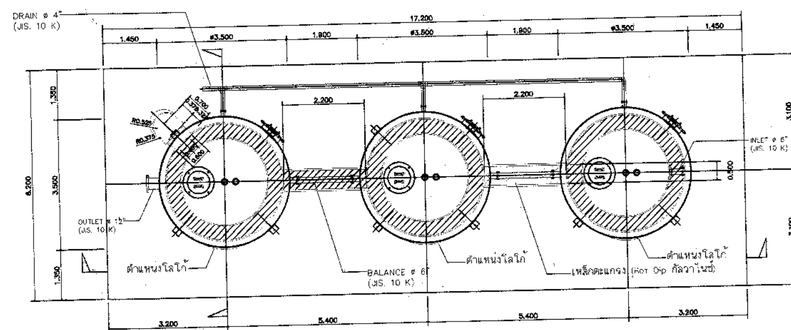
PLAN SCALE: 1/20
