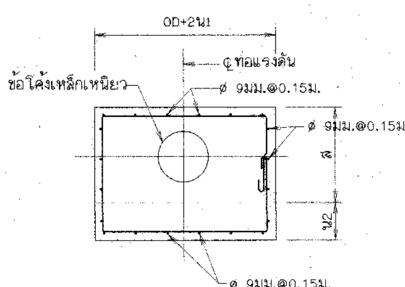
รูปตัด ๓-๓
