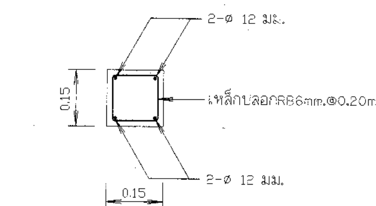
รูปตัด ก - ก มาตรฐาน 1:10
