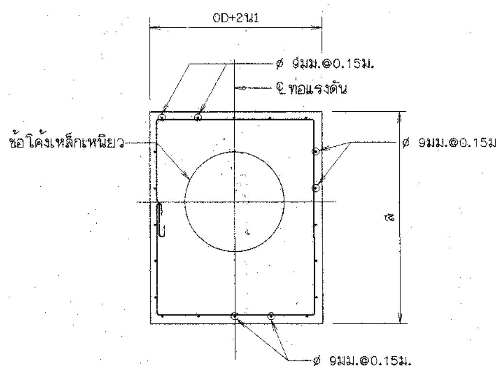
รูปตัด ๓-๓
