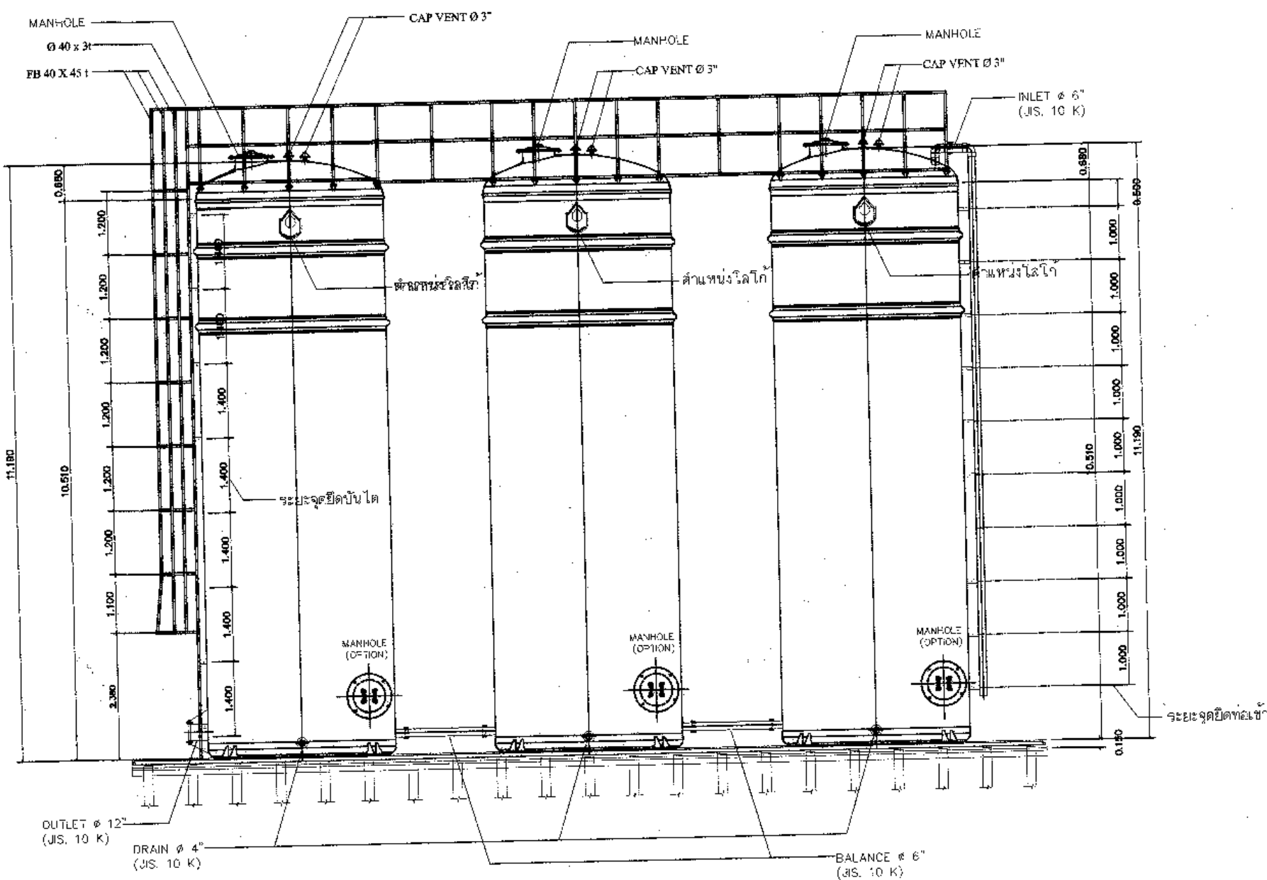
SECTION SCALE: 1/10
