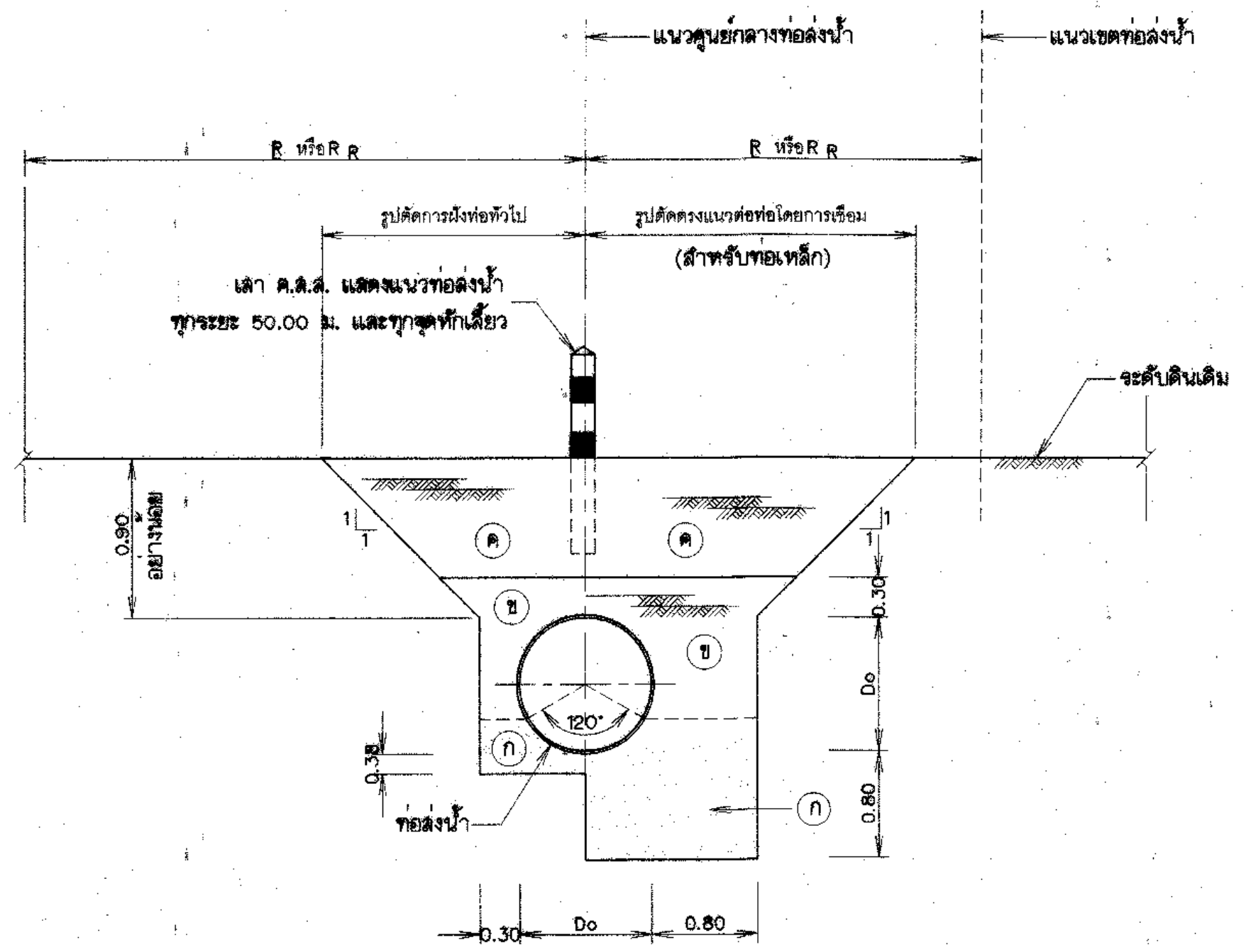
รูปตัดขวางการฝังท่อเหล็กเหนียว (SP) ไม่แสดงมาตราส่วน
