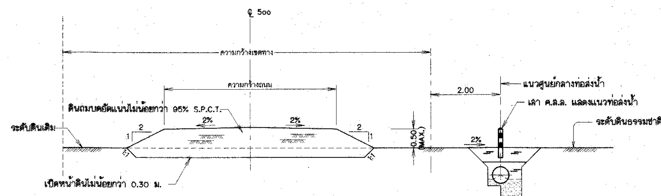
รูปตัดแสดงการวางท่อใต้ดินข้างถนน (กรณีดินถม)
