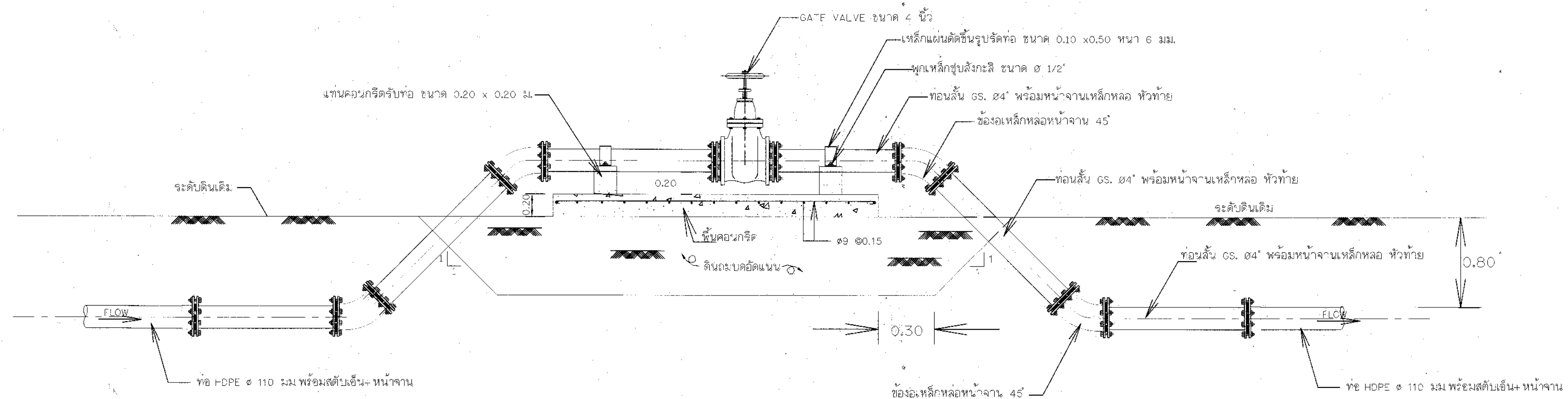
รูปตัดของระบบกระจายน้ำท่อ HDPE ขนาด 110 มม. ก-ก
