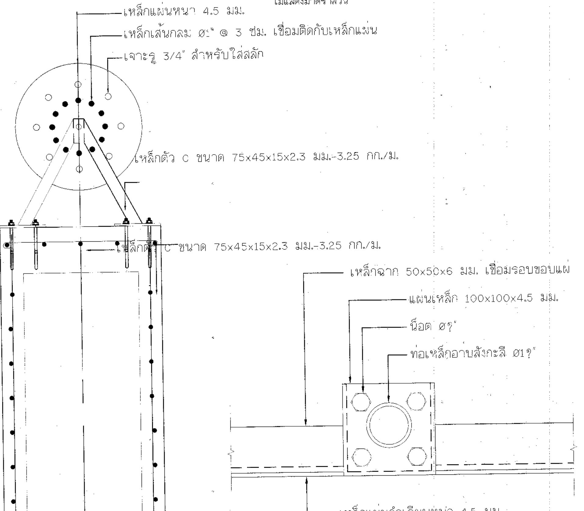
รูปตัด 1-1
