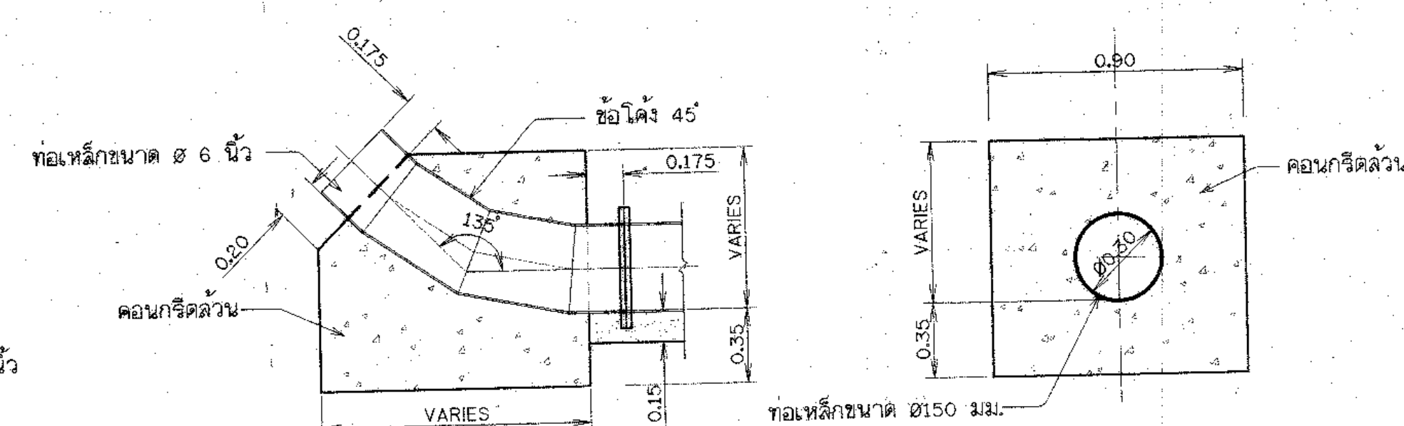
รูปตัด ข1 - ข1 ไม่แสดงมาตราส่วน
