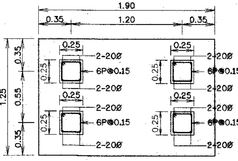
รูปตัด จ-จ
