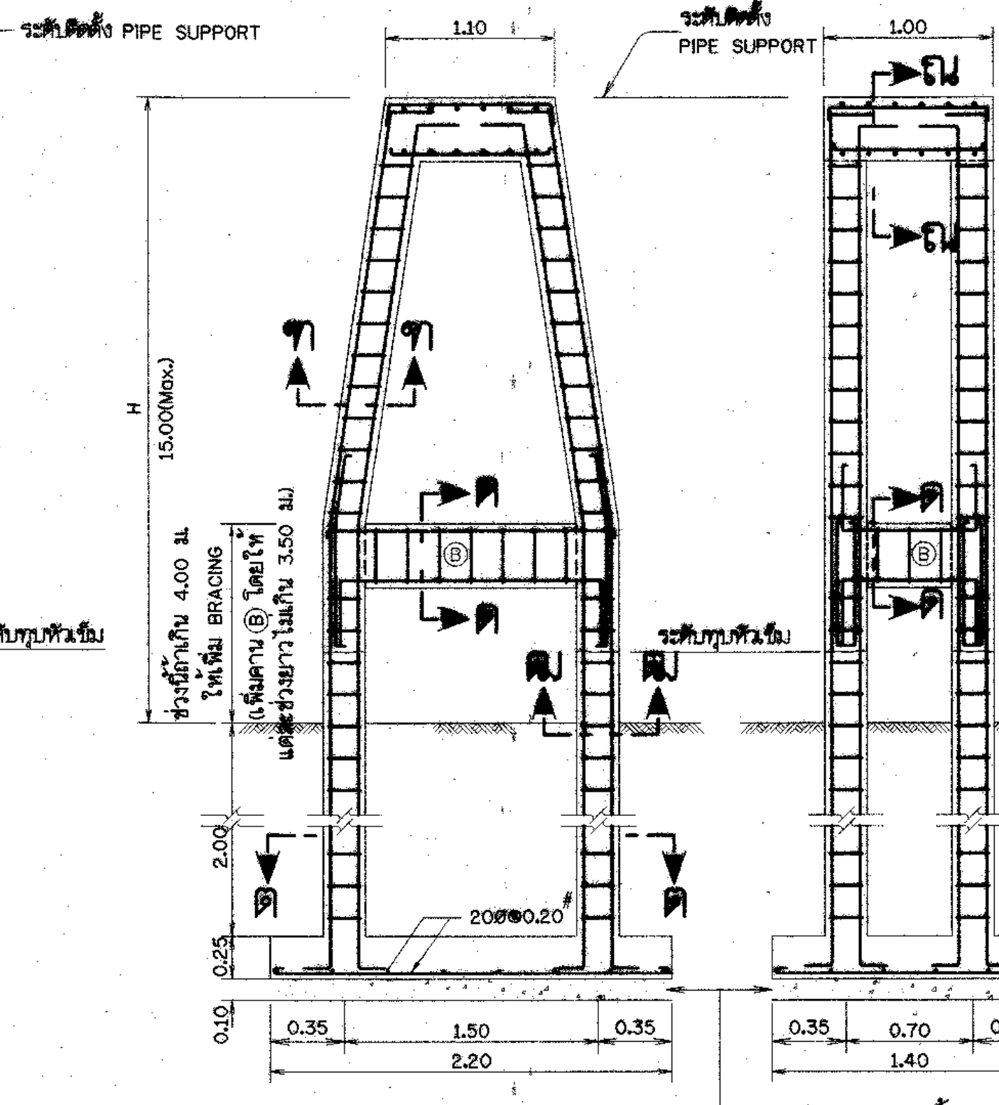
รูปตัดตามขวาง
