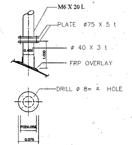
DETAIL B (ขี้ดรวก้นคก)
