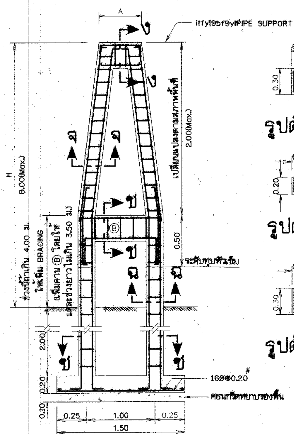
การเสริมเหล็ก คอมม่อแบบที่ 2
