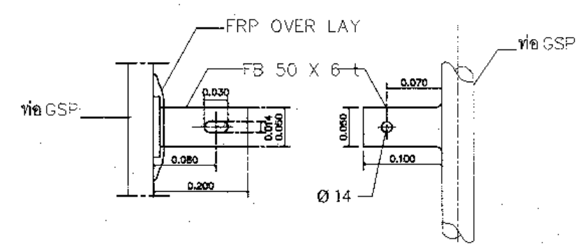
DETAIL C (ขี้ดท่อ)
