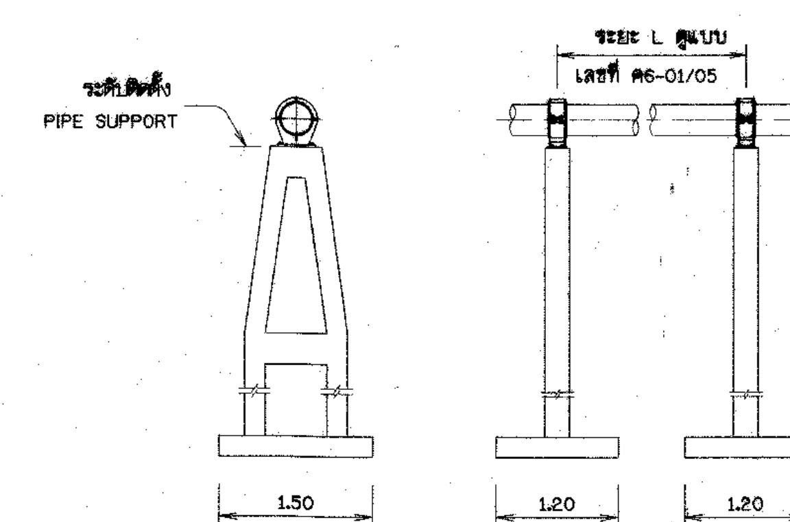
รูปด้านหน้า
