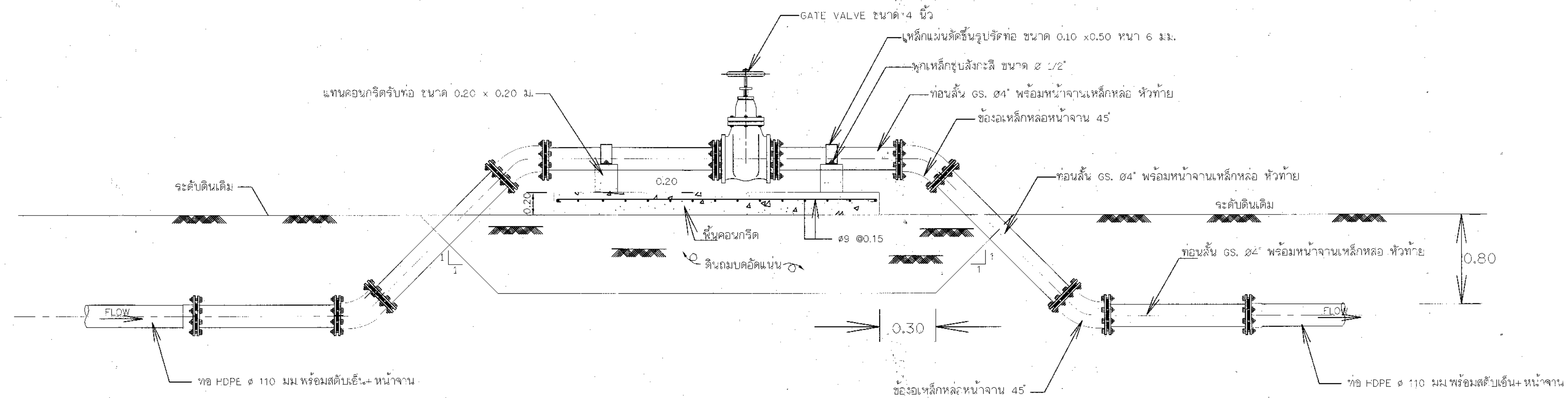
รูปตัดขยายประตุน้ำคุมท่อจ่ายน้ำ ท่อ DPL ขนาด 110 มม ก-ก
