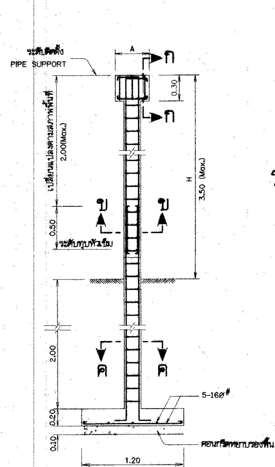
การเสริมเหล็ก คอมม่อแบบที่ 1
