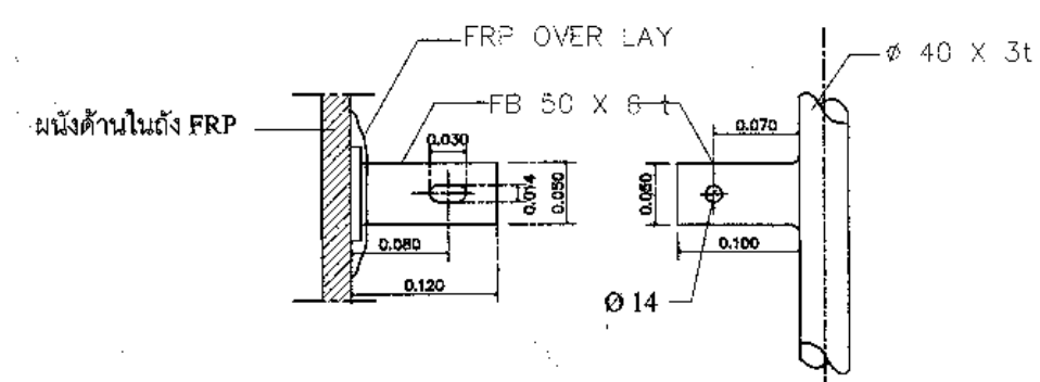
DETAIL A (ขี้ดบ้นโด)
