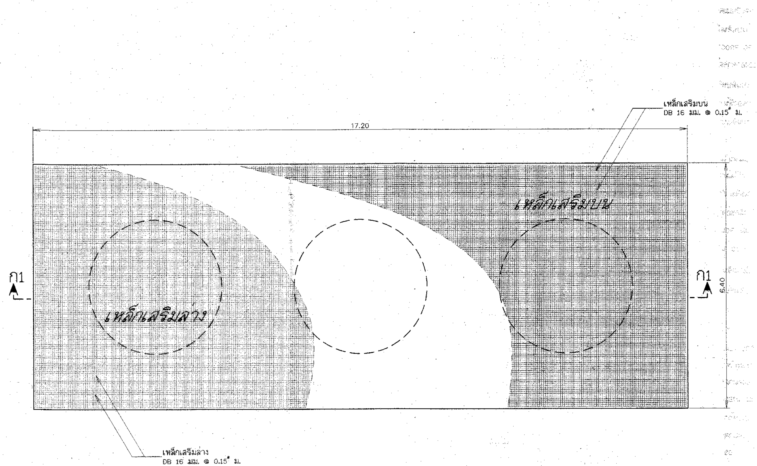
แปลนเสริมเหล็กพื้น มาตราส่วน 1:50
