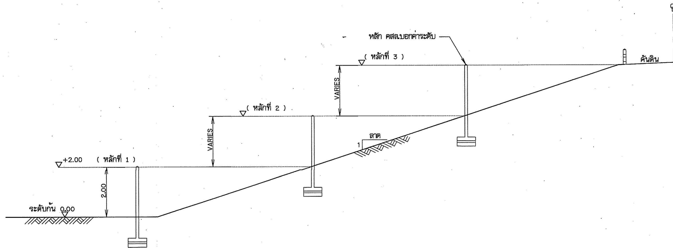
รูปตัดทั่วไปแสดงตำแหน่งหลักบ่อค่าระดับน้ำ
