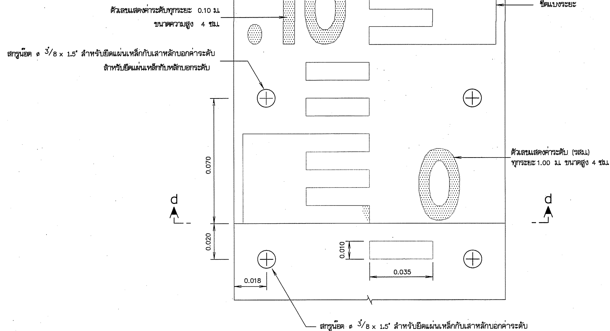
ขยายแผ่นหลักบ่อค่าระดับ
