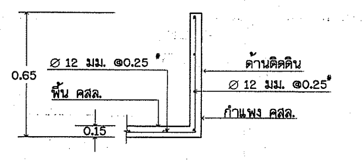
รูปตัด ๑-๑ (ความหนาหิน 0.15 ม.) ไม่แสดงมาตราส่วน
