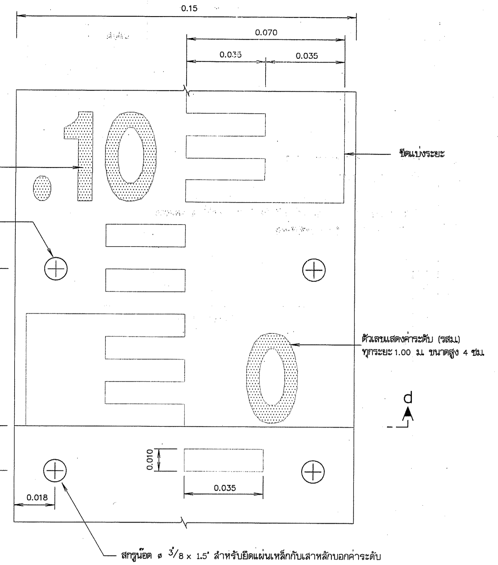
ขยายแผ่นเหล็กบอกค่าระดับ
