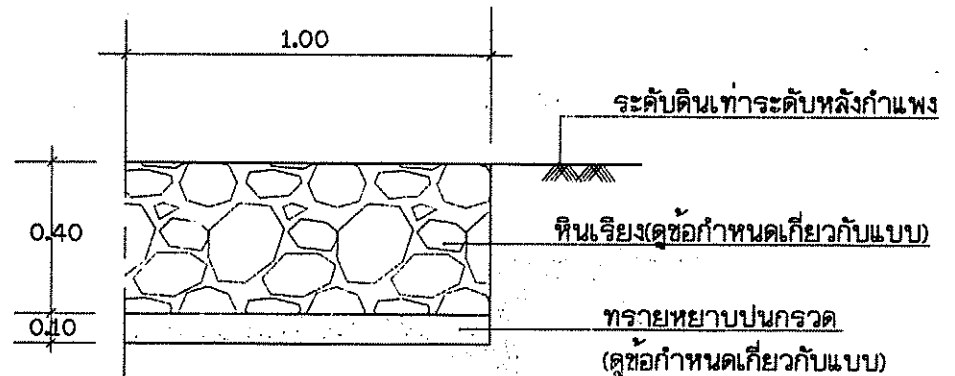
ขยายหินเรียง 2 ไม่แสดงมาตราส่วน
