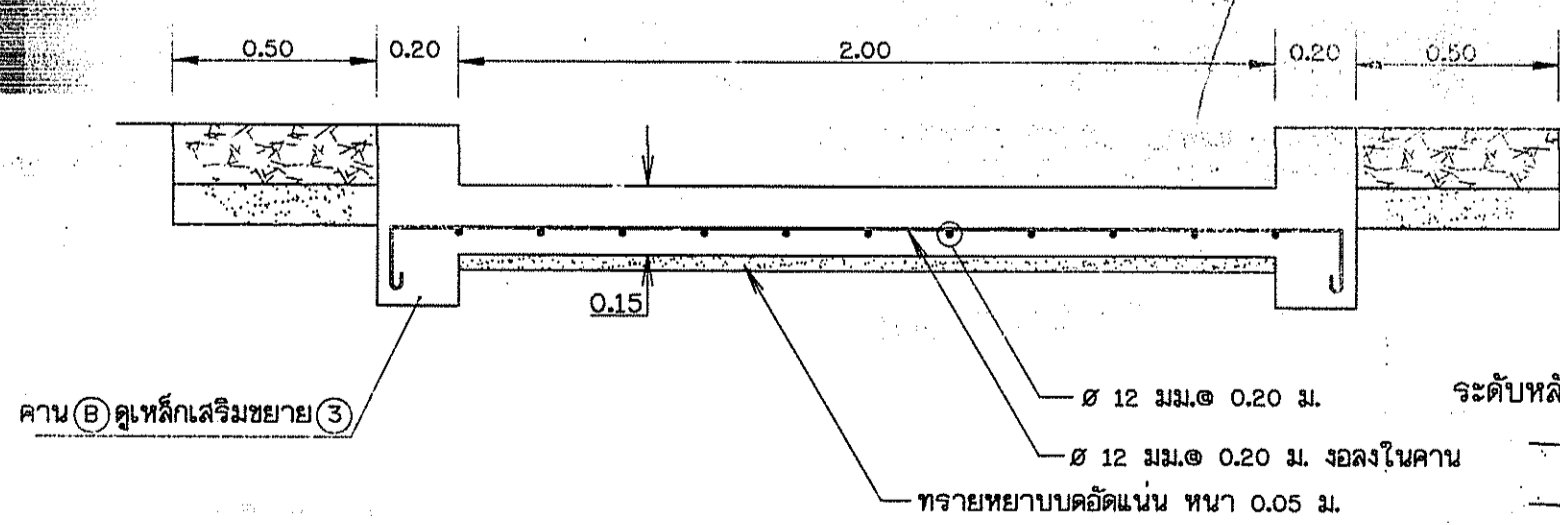
รูปตัด ค - ค
