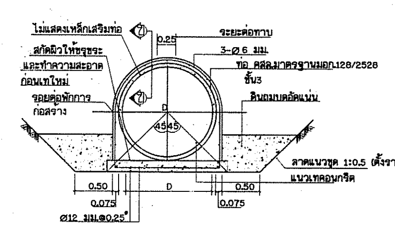
รูปตัดการวางท่อ คสล. ไม่แสดงมาตราส่วน
