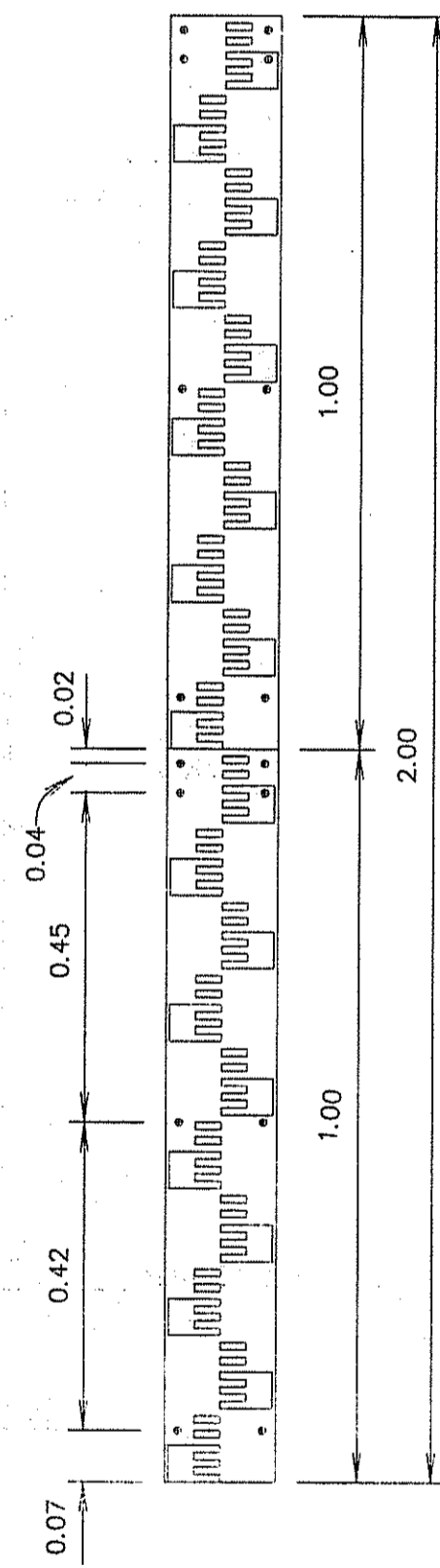
ขยายแผ่นเหล็กบอกค่าระดับ
