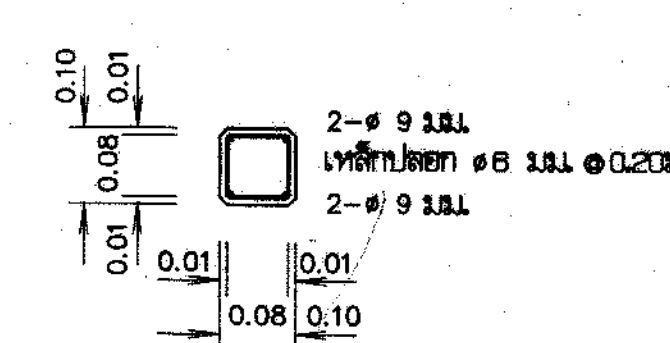
รูปตัด ข-ข มาตรฐาน 1:10
