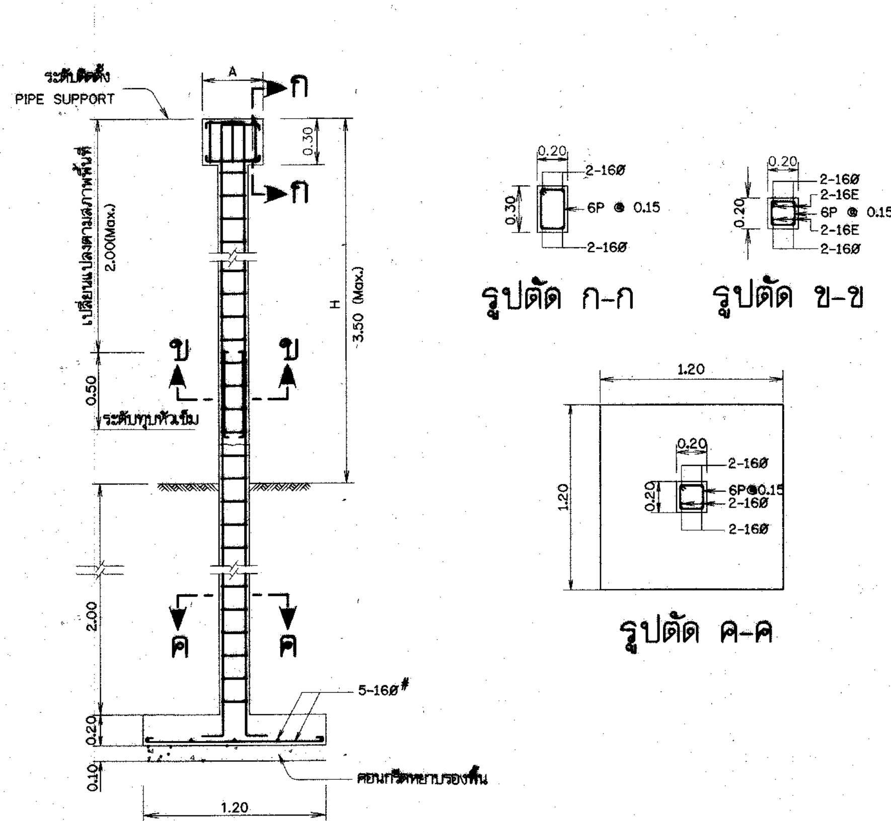
การเสริมเหล็ก แบบที่ 1
