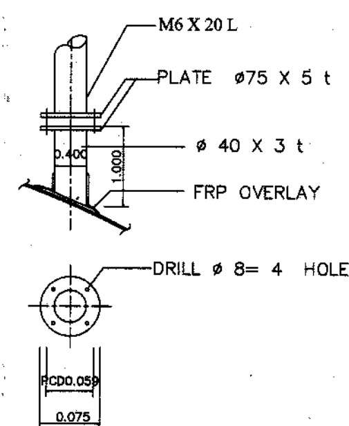
DETAIL B (ขี้ดราวกั้นคก)
