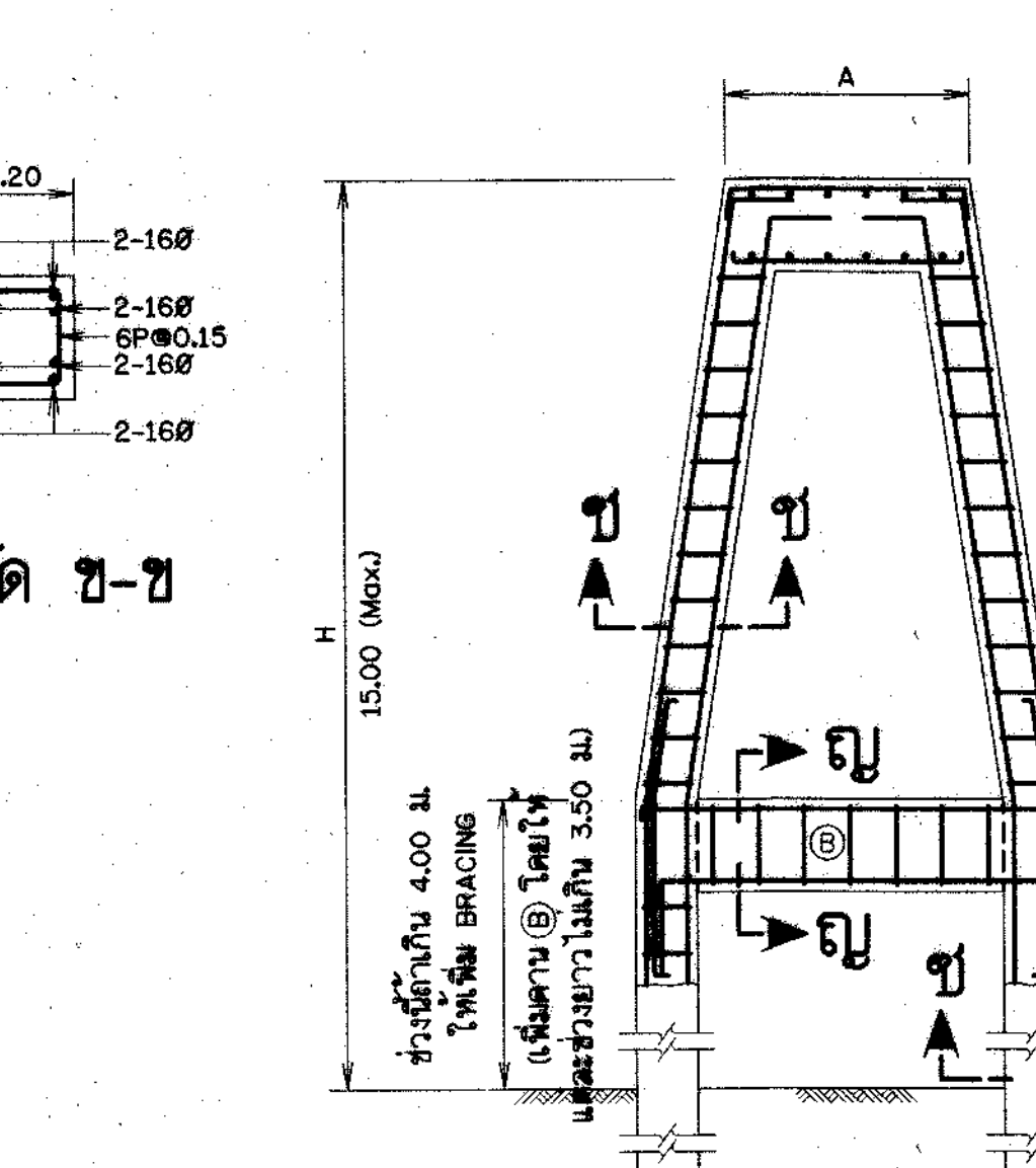
การเสริมเหล็ก ตอม่อแบบที่ 2
