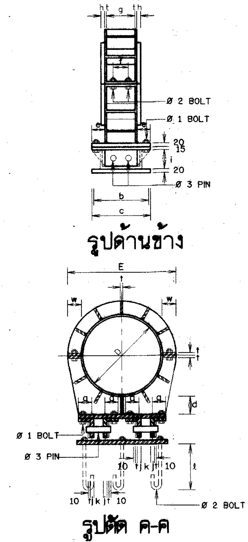
PIPE SUPPORT สำหรับท่อเหล็กขนาด \varnothing 400 มม. - \varnothing 800 มม. มาตราส่วน
