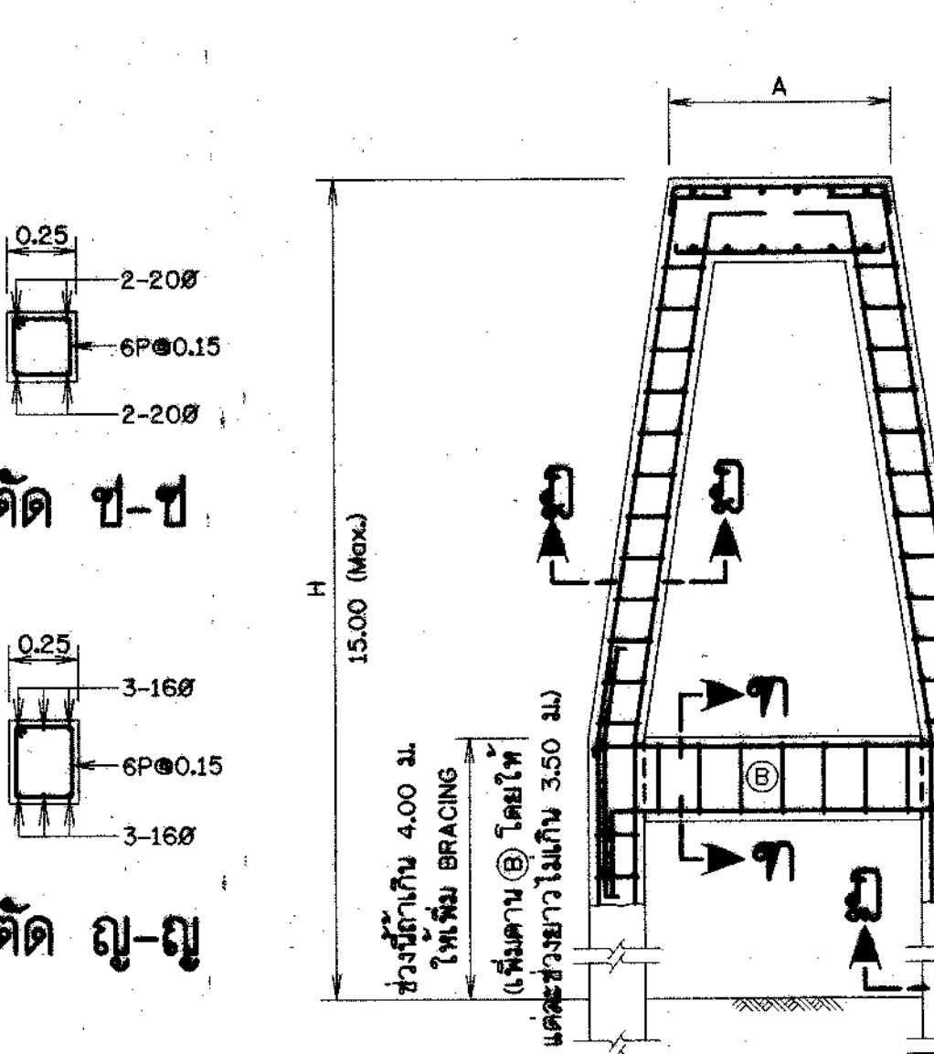
การเสริมเหล็ก ตอม่อแบบที่ 3,4
