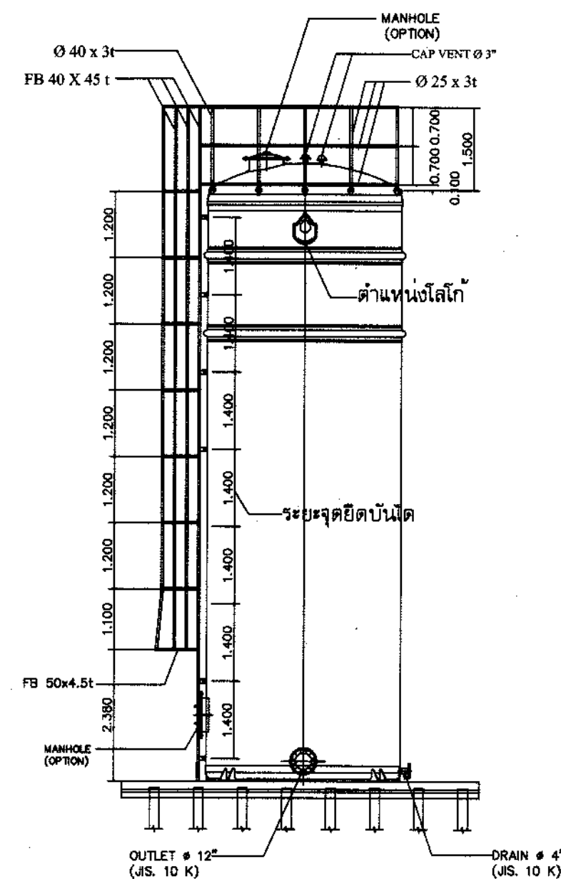
SECTION SCALE: 1:100
