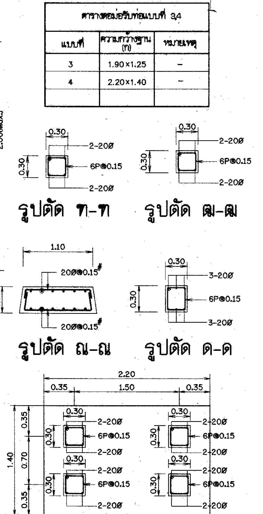
รูปตัด ก-ก
