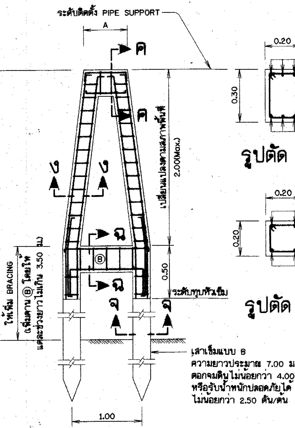
การเสริมเหล็ก ตอม่อแบบที่ 1
