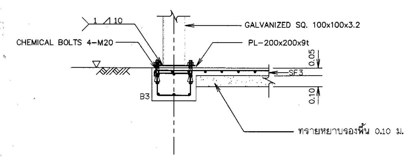
รูปตัด ก1 - ก1
