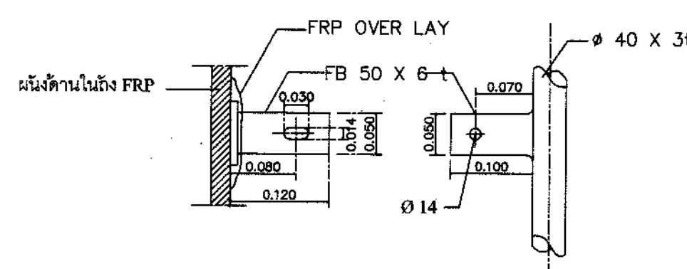
DETAIL A (ขี้ดบันได)
