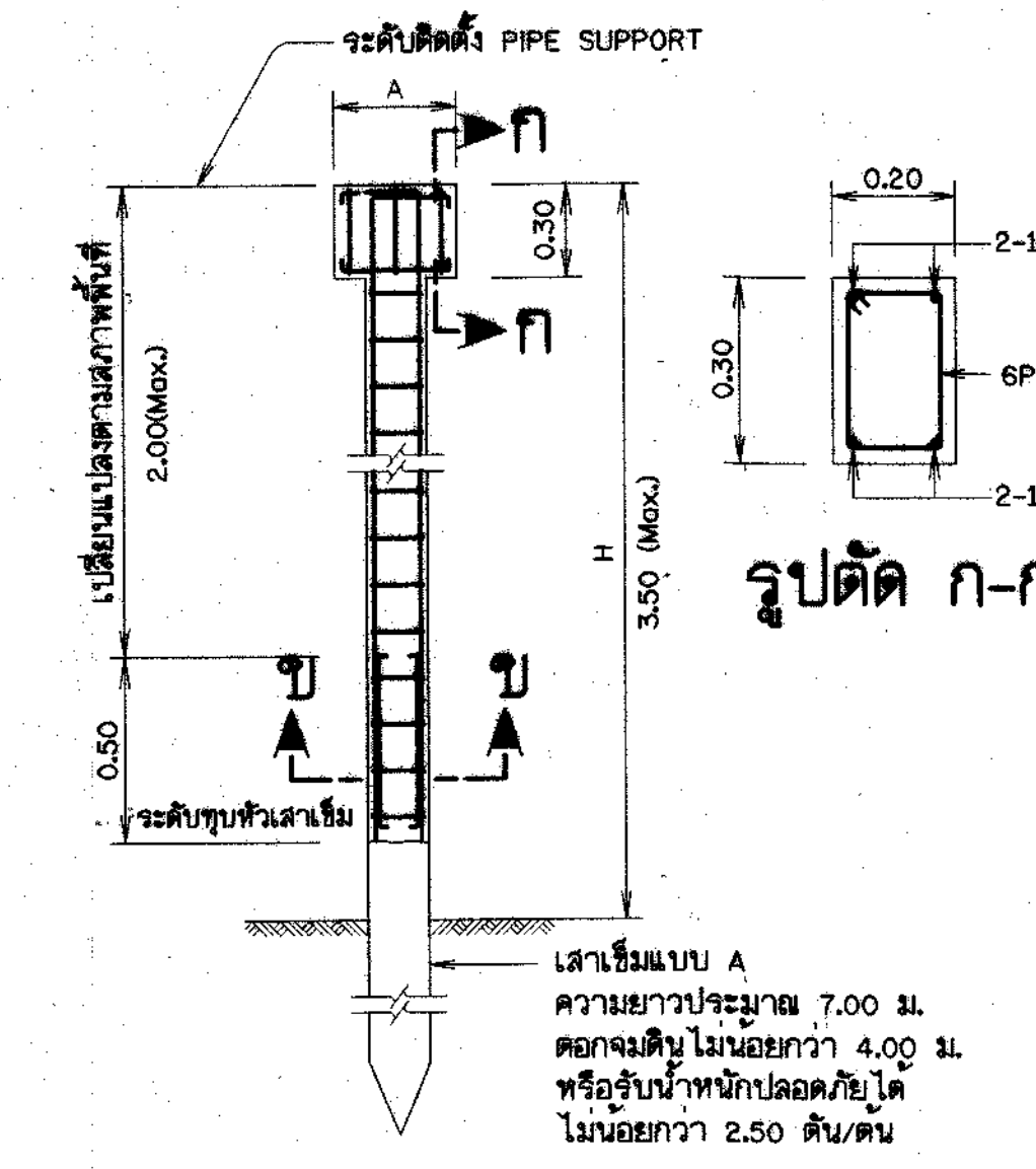
การเสริมเหล็ก ตอม่อแบบที่ 1
