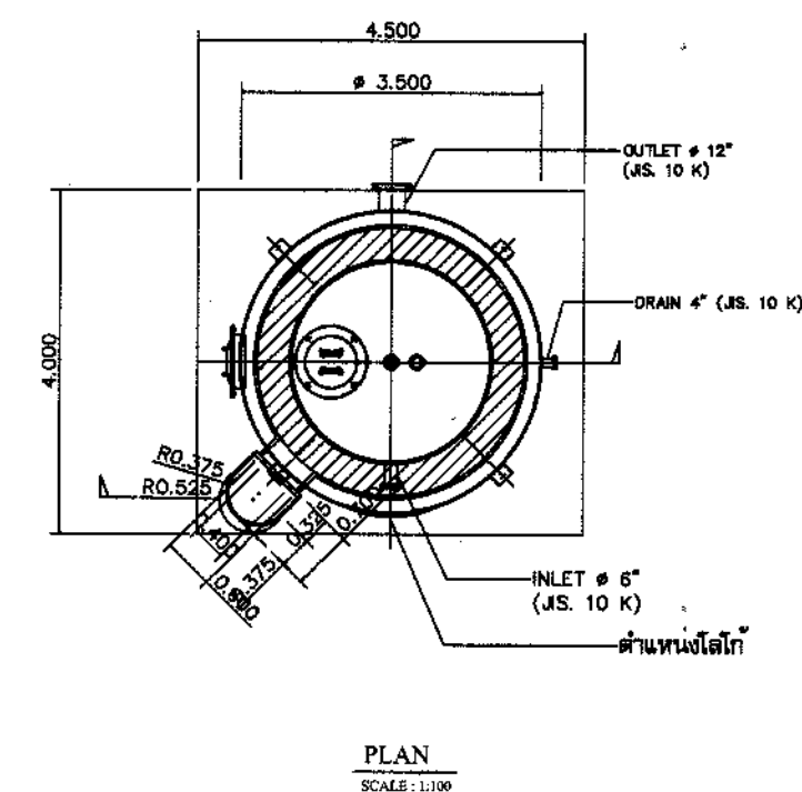
PLAN SCALE: 1:100
