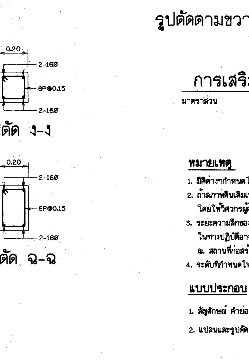
การเสริมเหล็ก ตอม่อแบบที่ 2
