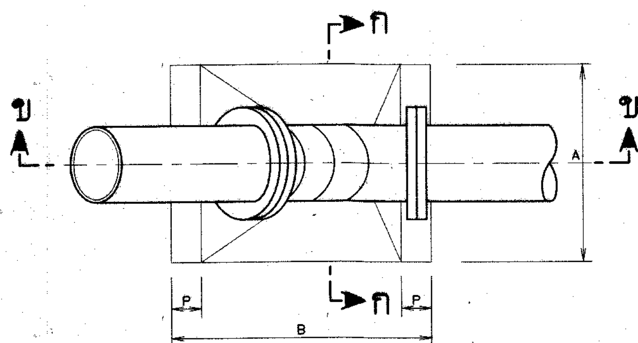
แปลน THRUST BLOCK รับข้อต่อโค้งแนวตั้ง มาตราส่วน (สำหรับท่อเหล็ก)
