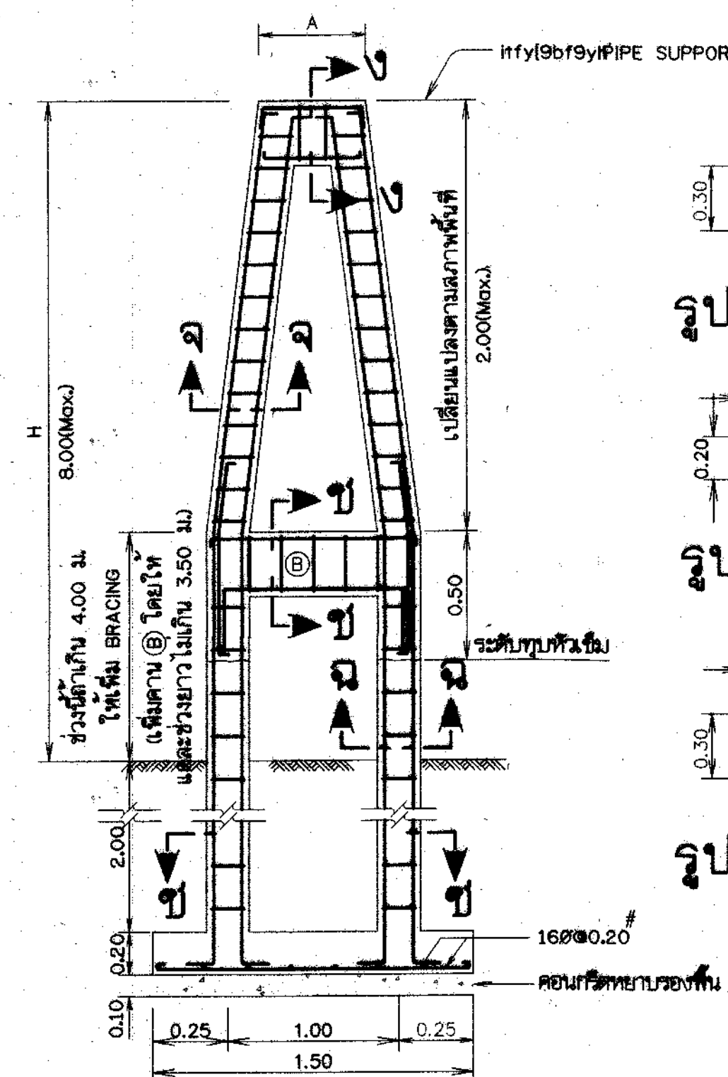
การเสริมเหล็ก แบบที่ 2
