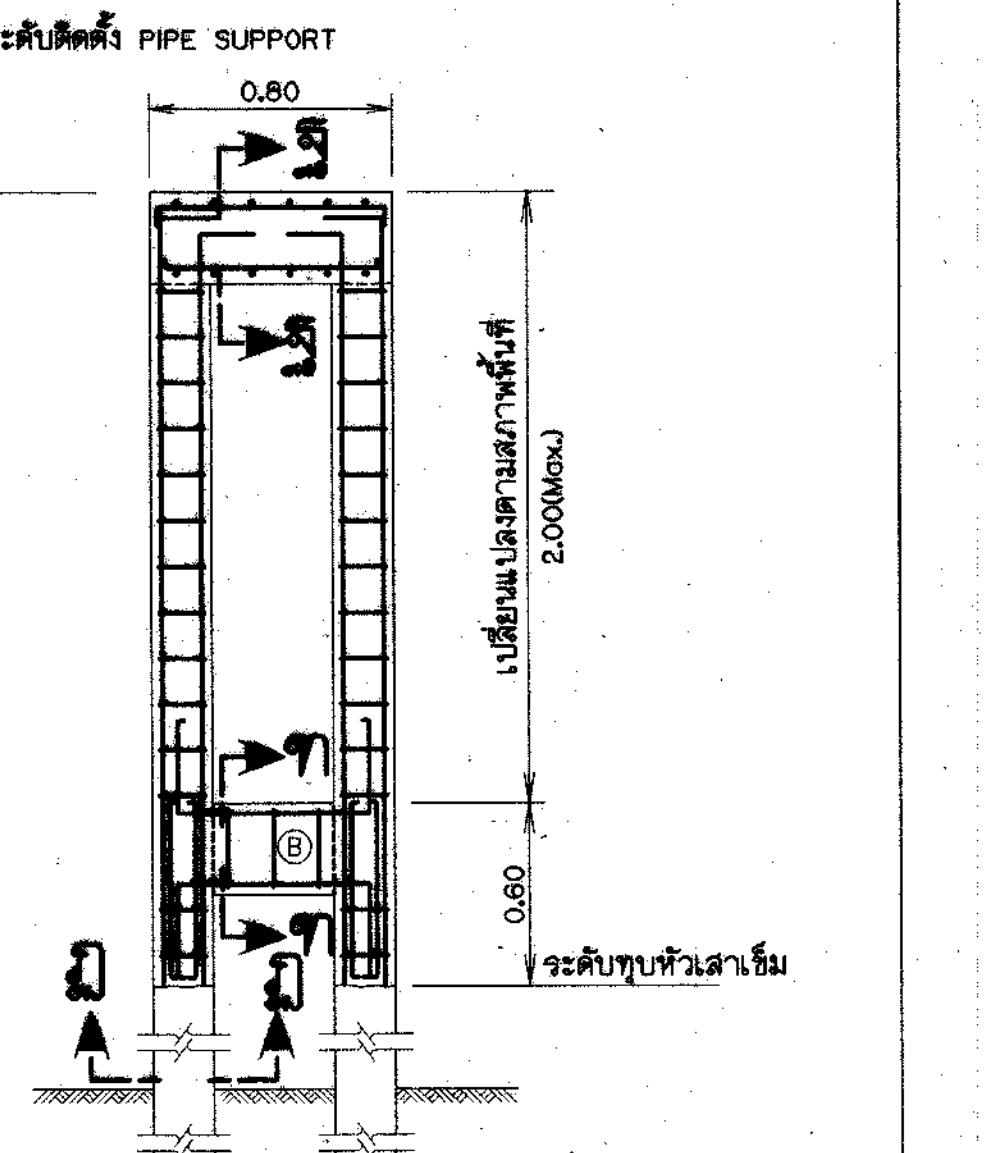
การเสริมเหล็ก ตอม่อแบบที่ 3,4
