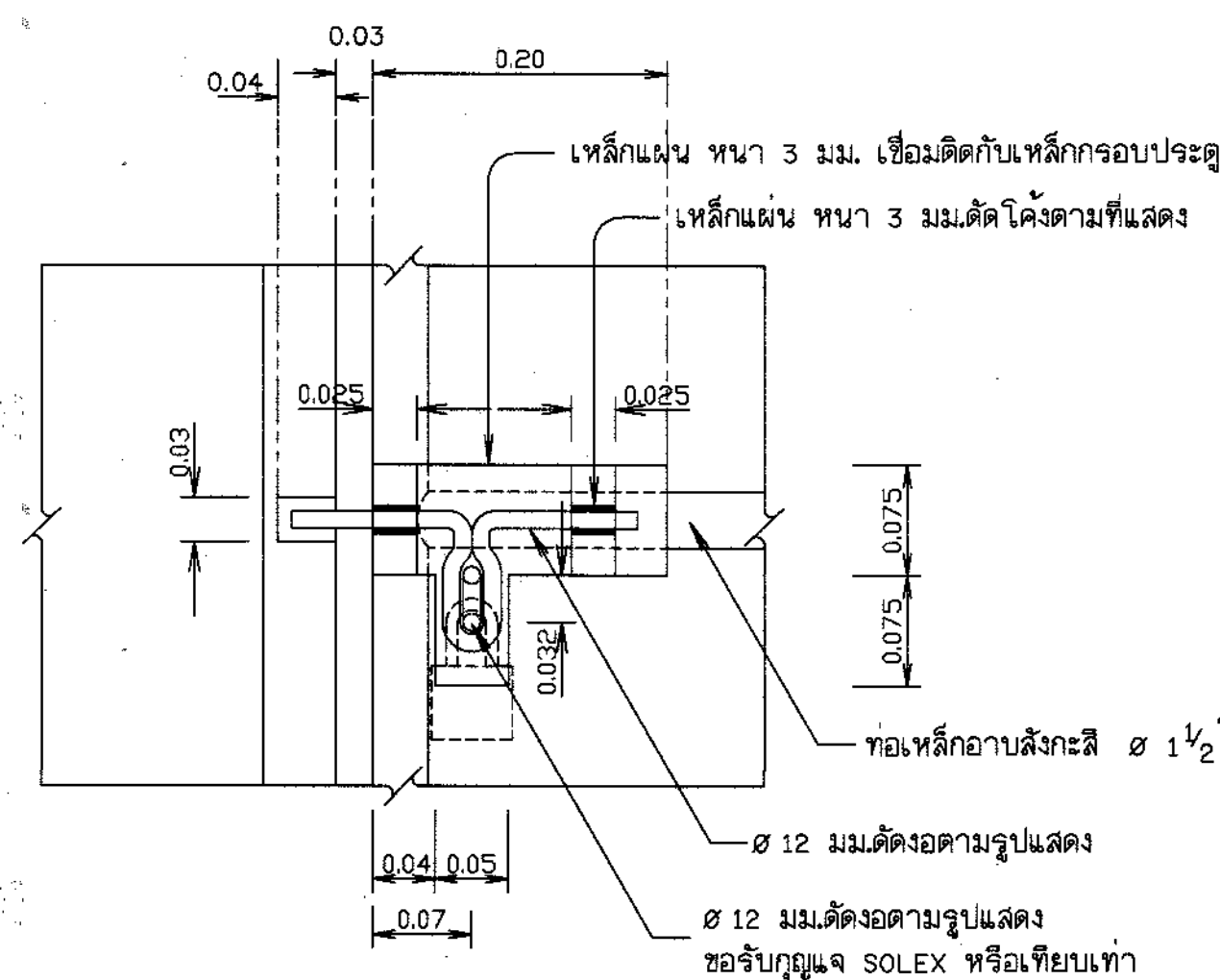
แบบขยาย 1 มาตราส่วน 1:5
