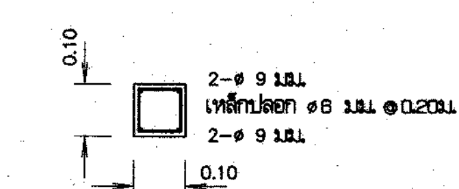
รูปตัด ก-ก มาตรฐาน 1:10
