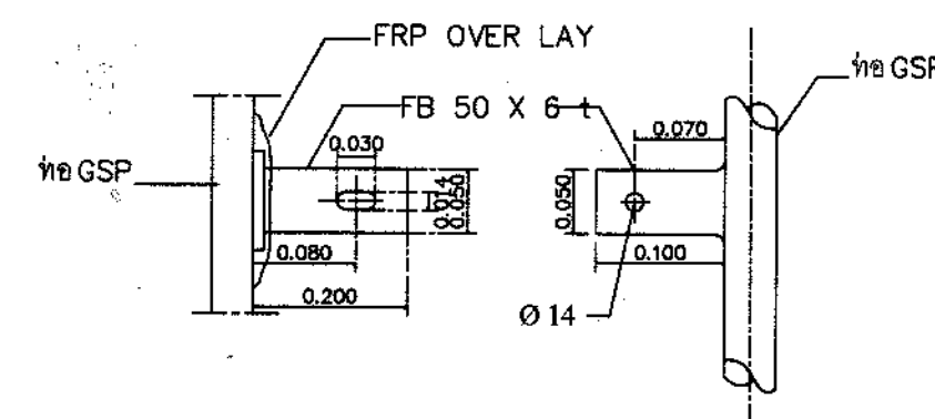
DETAIL C (ขี้ดท่อ)
