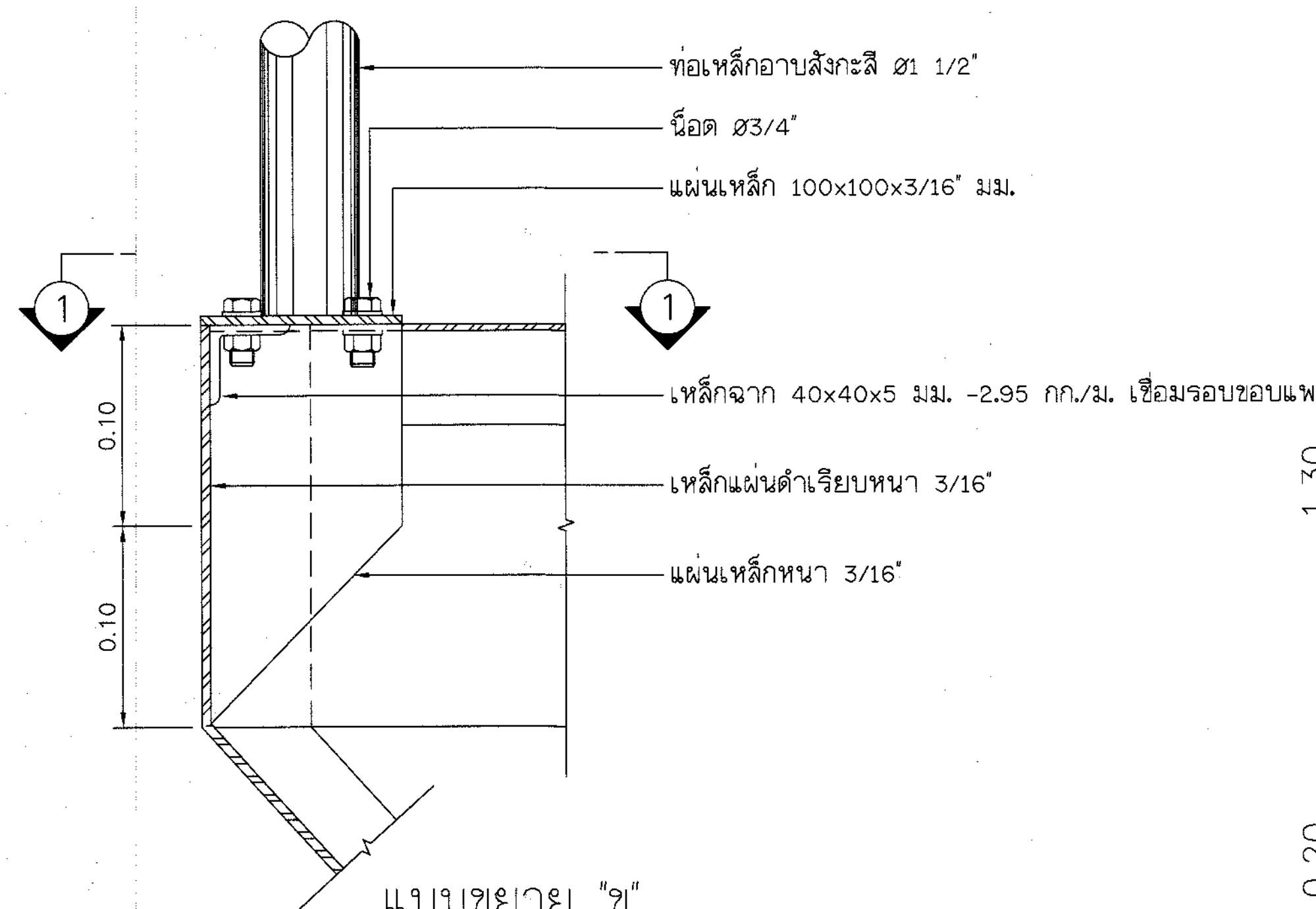
แบบขยาย "ข" ไม่แสดงมาตราส่วน
