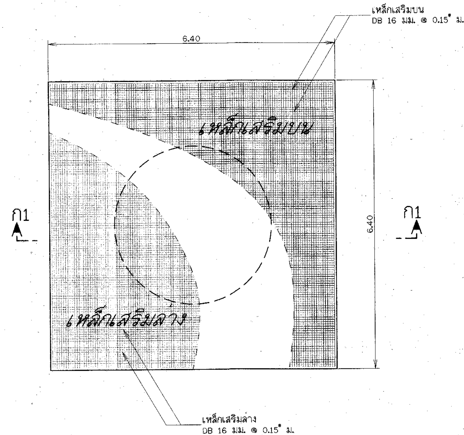
แปลนเสริมเหล็กพื้น มาตราส่วน 1:50
