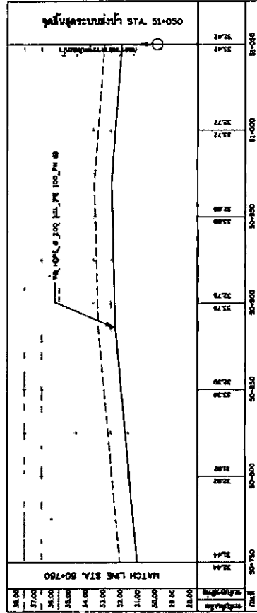
แปลระบลงน้ำ STA.50+750-51+050
