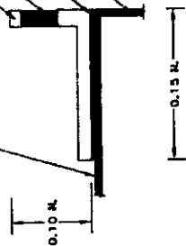
รูปตัดเหล็กยึดถึง 1:5
