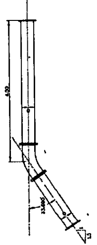
รายละเอียดท่อรับน้ำฝน ลาด 1:1.5 ขนาดหน้า 1:1 40
