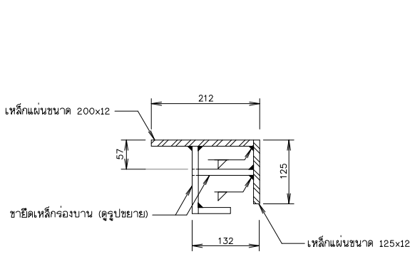
รูปตัดเหล็กกรอบบาน มาตราส่วน 1:10
