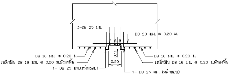
รูปขยาย 2 ไม่แสดงมาตราส่วน
