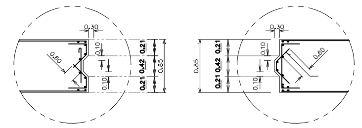
รูปขยาย 1 มาตราส่วน 1:10
