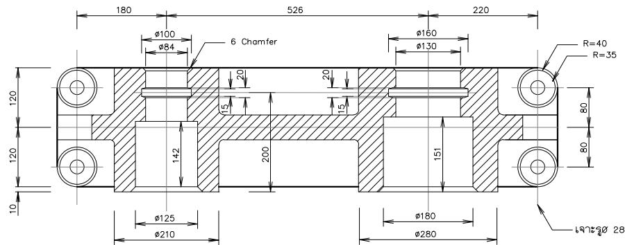
รูปตัด ฅ - ฅ มาตราส่วน 1:5
