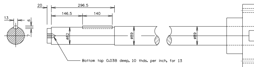
เพลาลม มาตราส่วน 1:5
