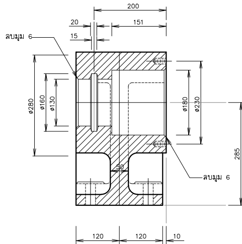
รูปตัด ท - ท มาตราส่วน 1:5
