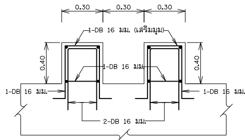
รูปตัด ๒ - ๒ ไม่แสดงมาตราส่วน
