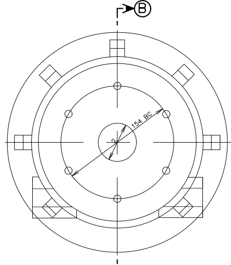
CLUTCH BOX มาตราส่วน (STEEL JIS G5101 SC 42) 1:1.5
