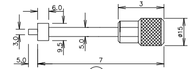
KNOB มาตราส่วน (STEEL JIS G4051 S 50 C) 1:1
