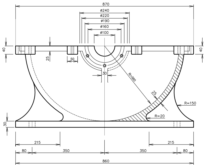
① โครงยึดเฟืองฐาน (เหล็กหล่อ) มาตราส่วน 1:5
