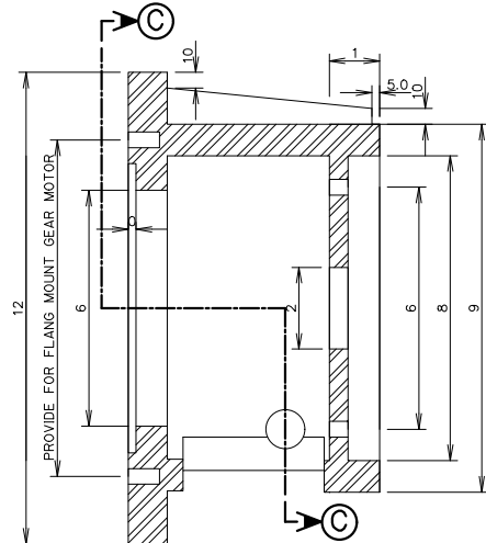
SECTION B-B มาตราส่วน 1:2.5
