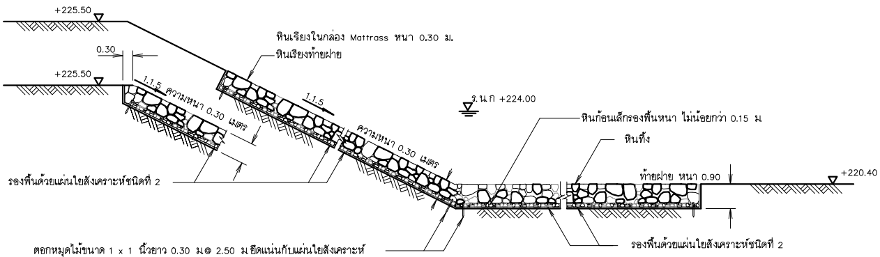
รูปตัดทั่วไปแสดงการเรียงหิน (ท้ายฝาย) ไม่แสดงมาตราส่วน
