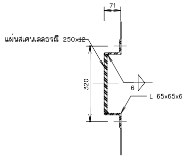
รูปตัด จ-จ
