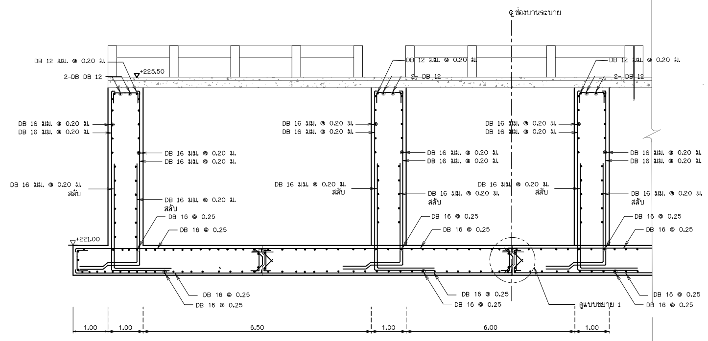
รูปตัด แสดงการเสริมเหล็ก จ - จ มาตราส่วน 1:50
