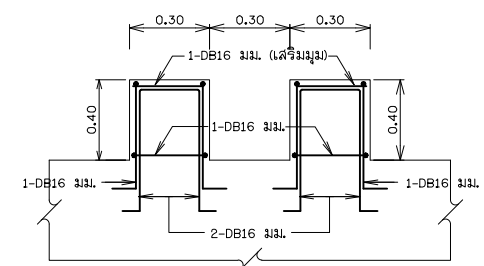
รูปตัด ข - ข
