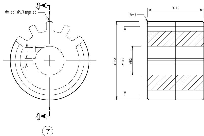
เฟืองทด มาตราส่วน 1:2.5
