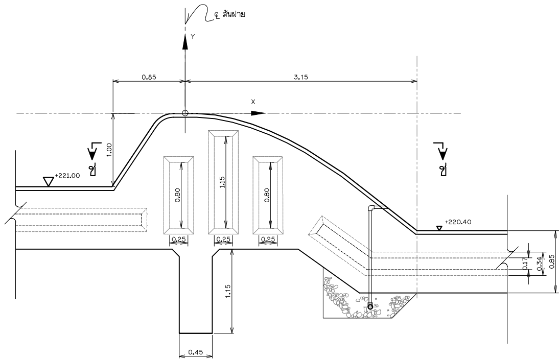
รูปขยายรอยต่อที่สันฝายฯ 1.00 ม.
