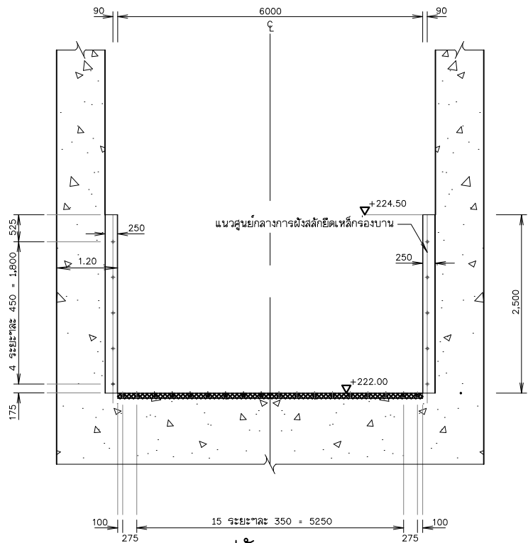
รูปตัด ง-ง
