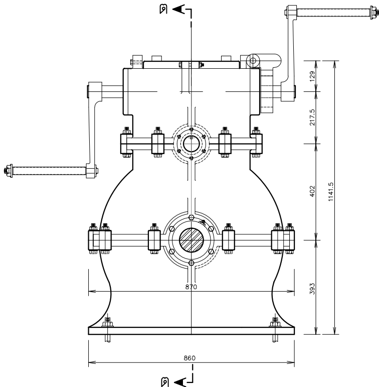
รูปด้านหน้า มาตราส่วน 1:7.5
