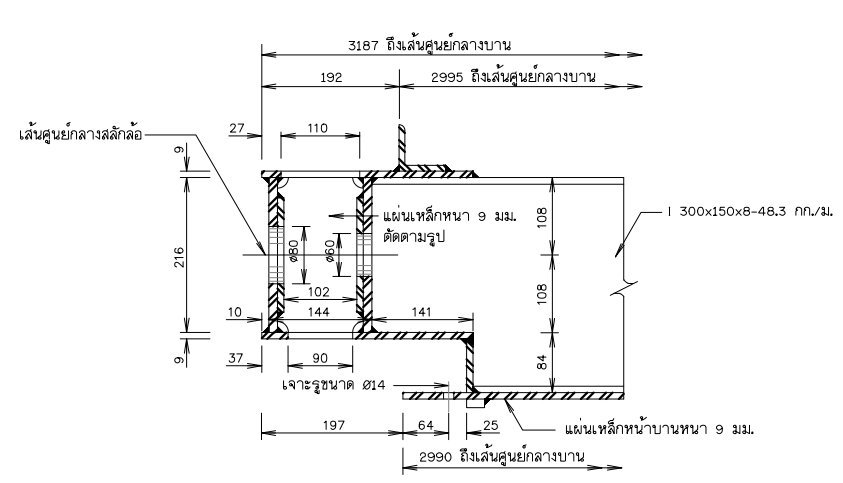
รูปตัด ค-ค มาตราส่วน 1:5
