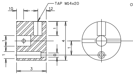
HANDLE BLOCK มาตราส่วน (STEEL JIS G 4051 S 50 C) 1:1.5
