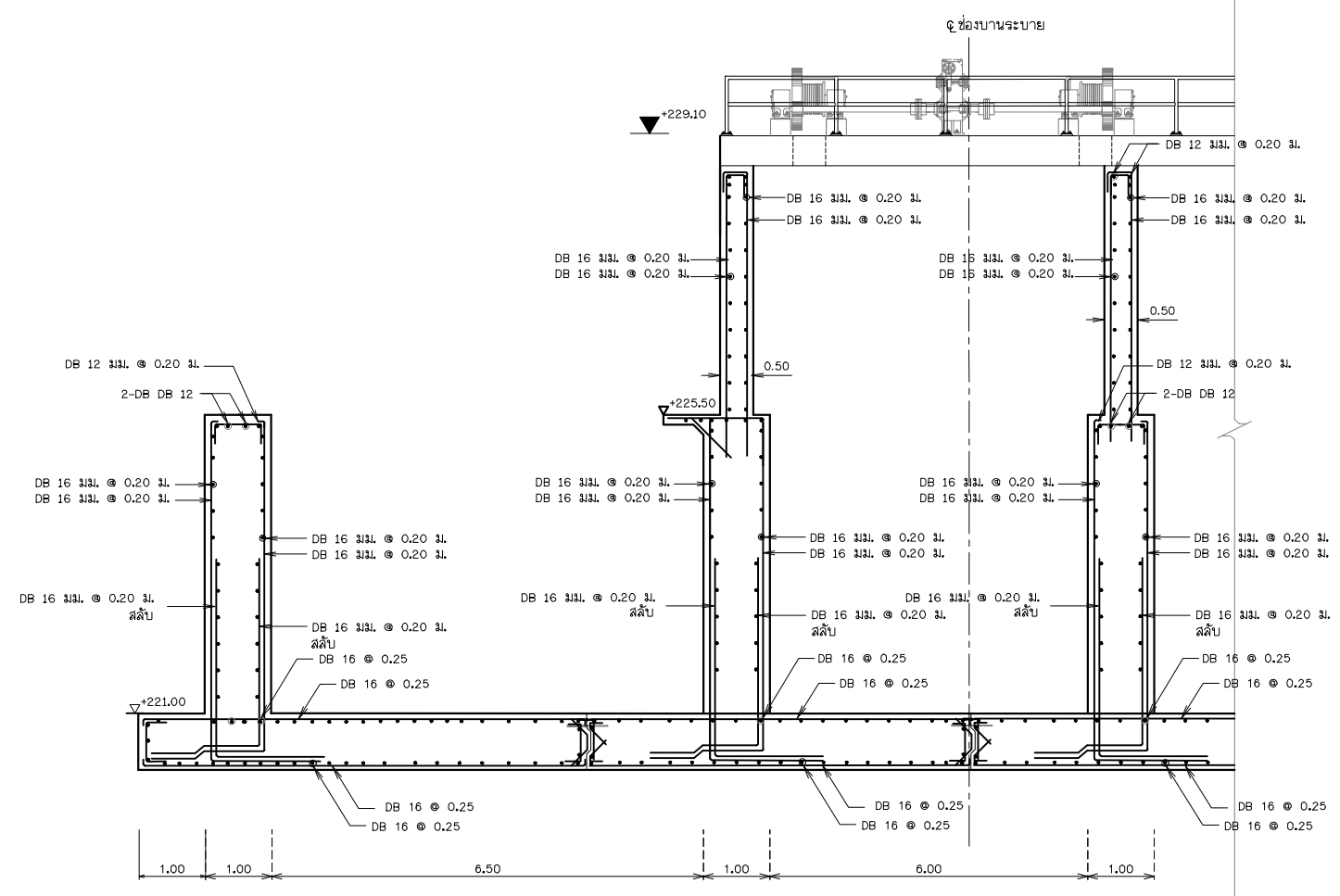
รูปตัด แสดงการเสริมเหล็ก จ - จ มาตราส่วน 1:50
