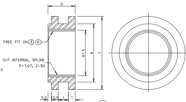
SPLINE HUB มาตราส่วน STEEL JIS G4051 S 50 C 1:1.5
