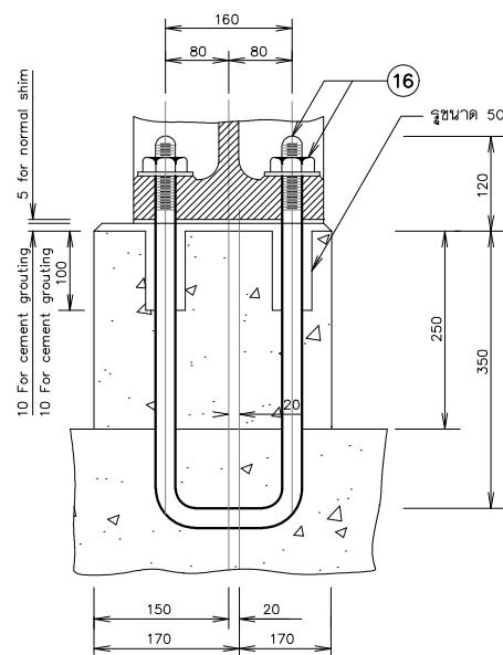
รูปตัด ฉ - ฉ มาตราส่วน 1:5
