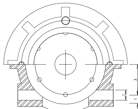
SECTION C-C มาตราส่วน 1:2.5
