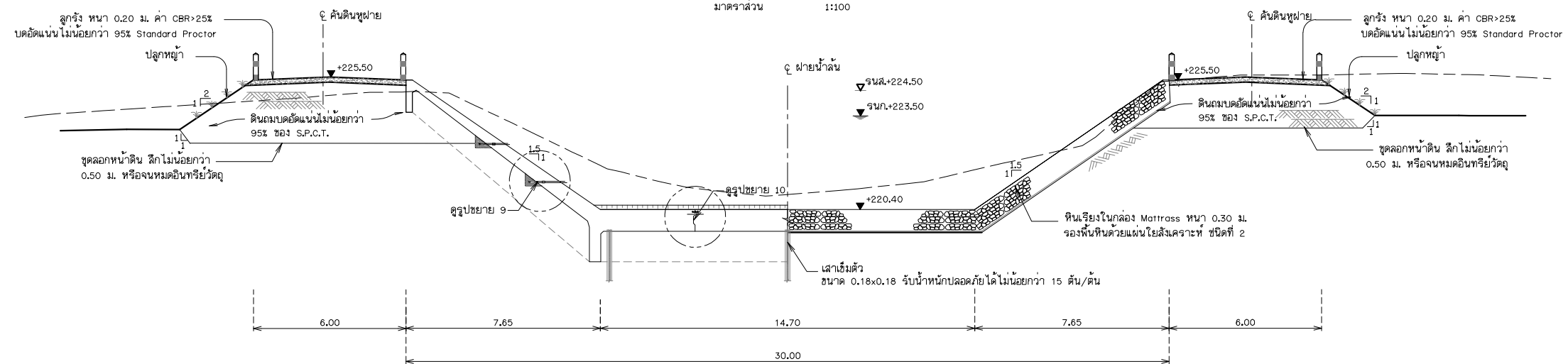
รูปตัด ง - ง มาตราส่วน 1:100
