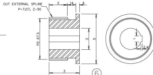
EXTERNAL SPLINE มาตราส่วน (STEEL JIS G 4051 S 50 C) 1:1.5
