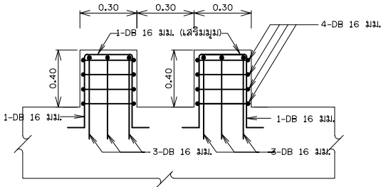
รูปตัด ๕ - ๕ ไม่แสดงมาตราส่วน
