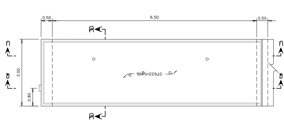
แปลนการเสริมเหล็ก มาตราส่วน 1:50
