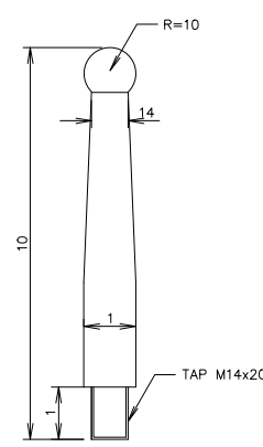
CLUTCH HANDLE มาตราส่วน (STEEL JIS G4051 S 30 C) 1:1.5
