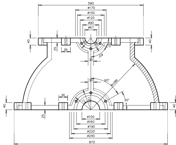
② โครงยึดเฟืองกลาง (เหล็กหล่อ) มาตราส่วน 1:5
