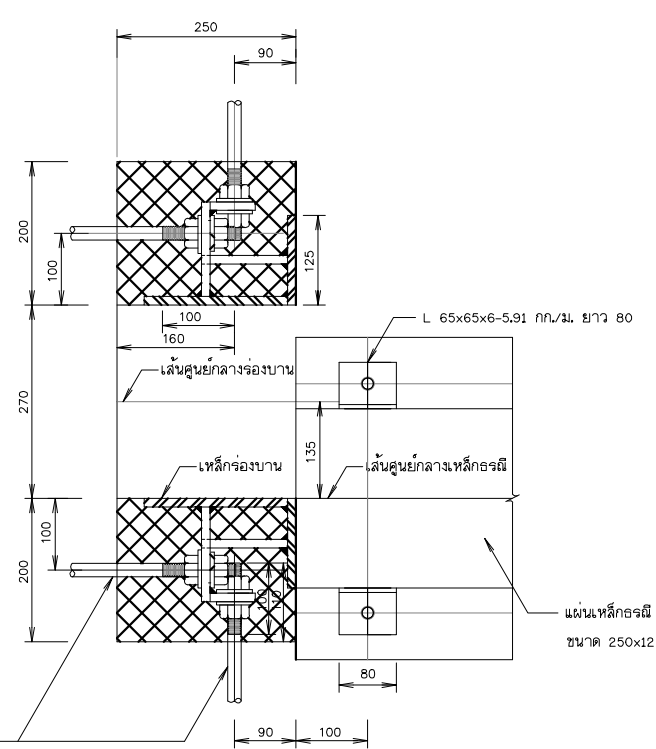
รูปขยาย " 6 " มาตราส่วน 1:5
