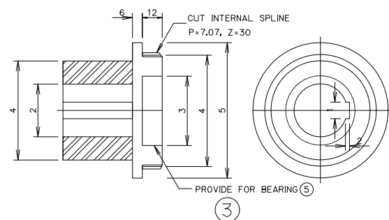
EXTERNAL SPLINE มาตราส่วน (STEEL JIS G 4051 S 50 C) 1:1.5
