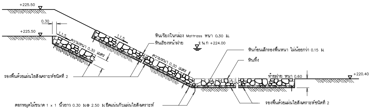
รูปตัดทั่วไปแสดงการเรียงหิน (หน้าฝาย) ไม่แสดงมาตราส่วน
