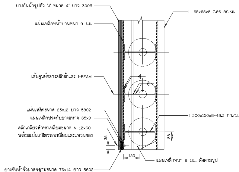
รูปขยาย " 2 " มาตราส่วน 1:10
