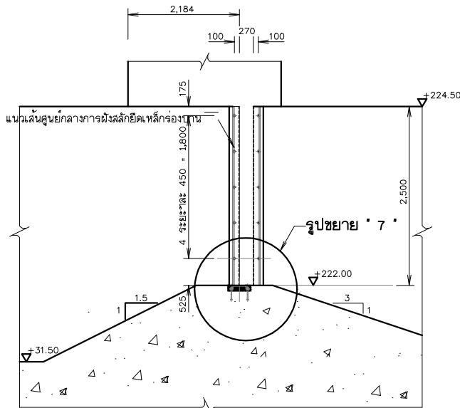
รูปตัด จ-จ
