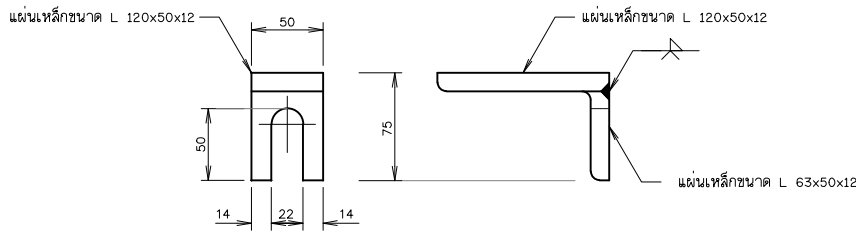
ขายึดเหล็กกรอบบาน มาตราส่วน 1:2.5
