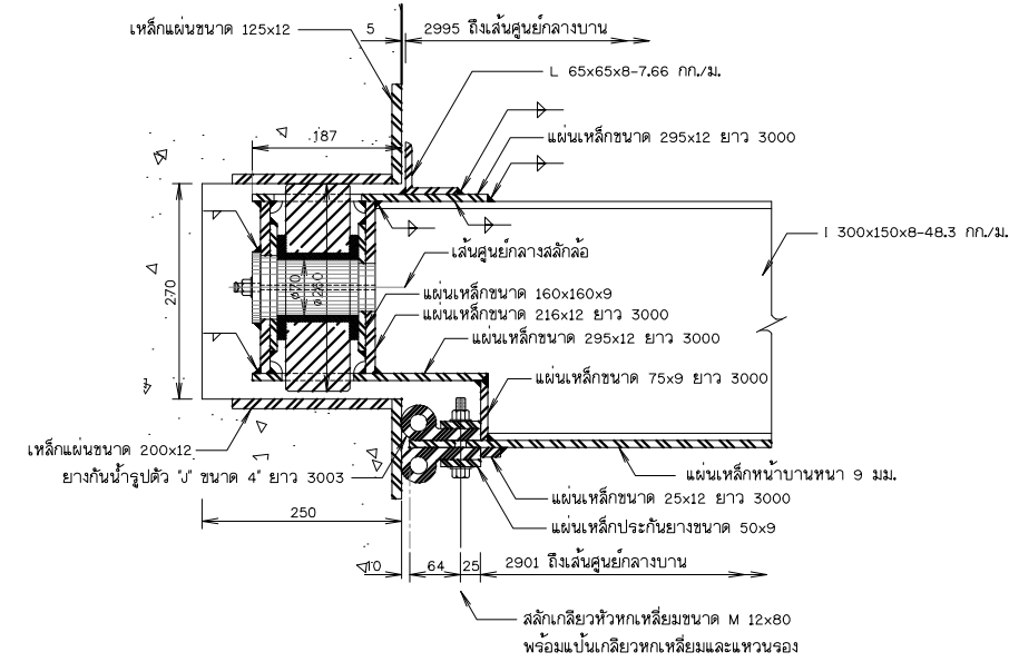
การประกอบ มาตราส่วน 1:5
