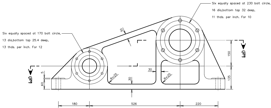
ฐานดานนอก มาตราส่วน 1:5
