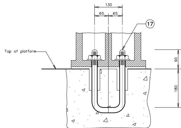
รูปตัด ยุ - ยุ มาตราส่วน 1:5
