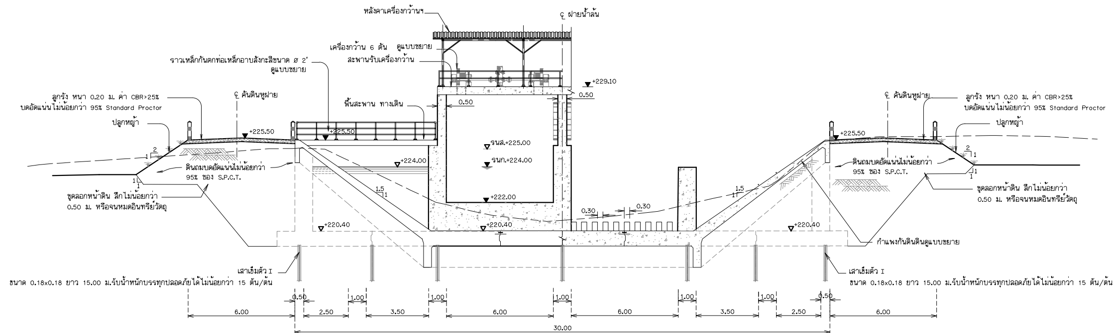
รูปตัด ง - ง มาตราส่วน 1:100
