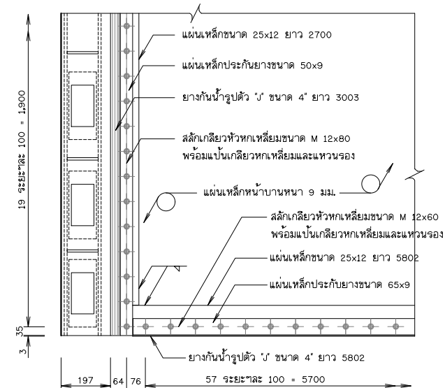
รูปขยาย " 3 " มาตราส่วน 1:10
