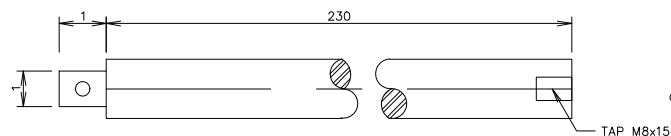
SHAFT มาตราส่วน (STEEL JIS G4051 S 50 C) 1:1.5
