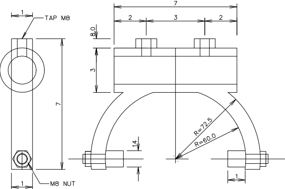
YOKE มาตราส่วน (STEEL JIS G5101 SC 42) 1:1.5
