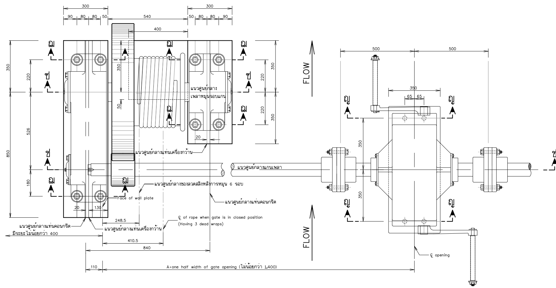
แปลนเครื่องกั้น มาตราส่วน 1:7.5
