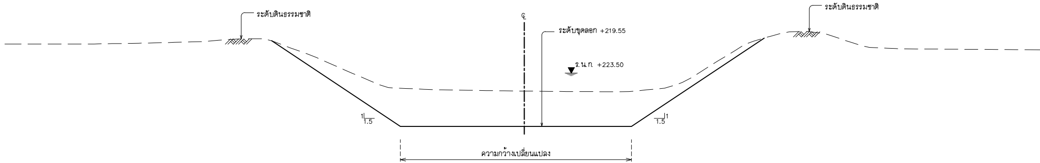
รูปตัดทั่วไปงานปรับเกลียลาดข้างและท้องคลอง ไม่แสดงขนาดราล่วน
