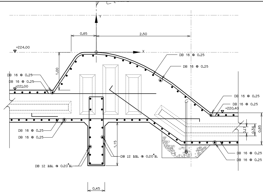
รูปแสดงการเสริมเหล็กสันฝายฯ 1.00 ม.
