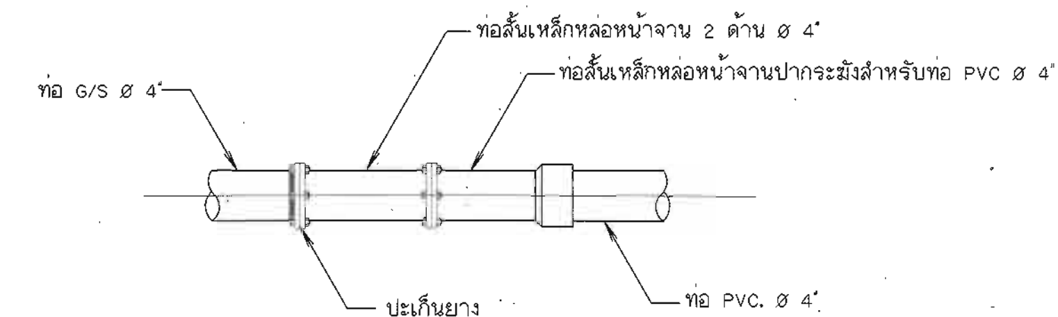
8. การบรรจุท่อเหล็กกล้าปลั่งกะสี G/S กับท่อ PVC. ไม่แสดงมาตราส่วน
