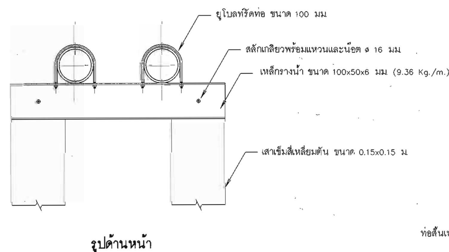
13. เสาตอม่อรับท่อชุด และแบบขยายอุปกรณ์รัดท่อ ไม่แสดงมาตราส่วน
