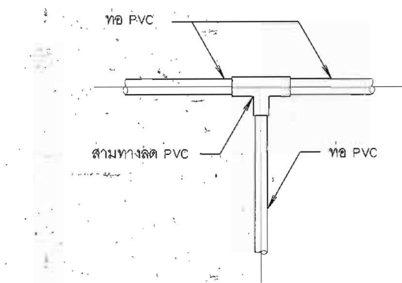
9. แบบการต่อสามทางลด PVC ไม่แสดงมาตราส่วน
