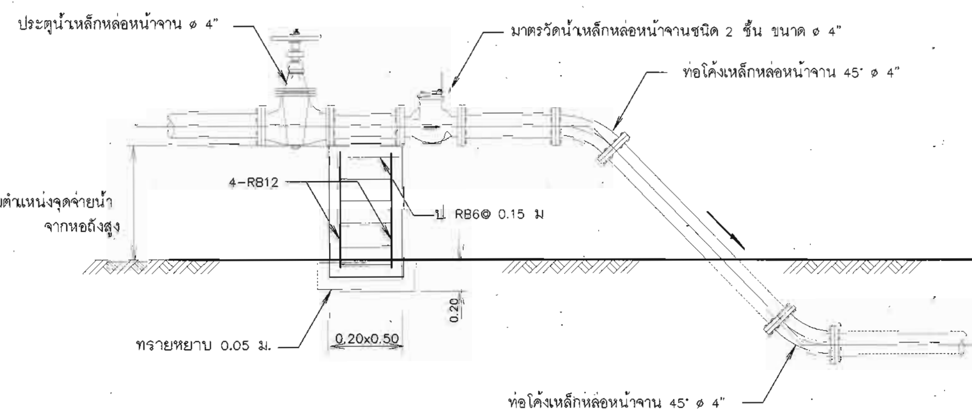
14. การติดตั้งมาตรวัดน้ำบนพื้นดิน 1/2" ไม่แสดงมาตราส่วน
