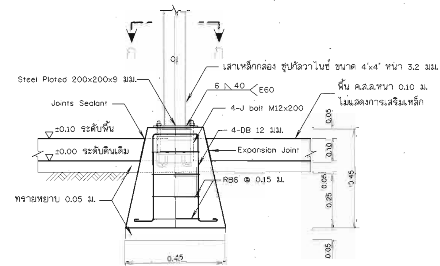
รูปขยายฐานรากโครงสร้างรับแผง F1
