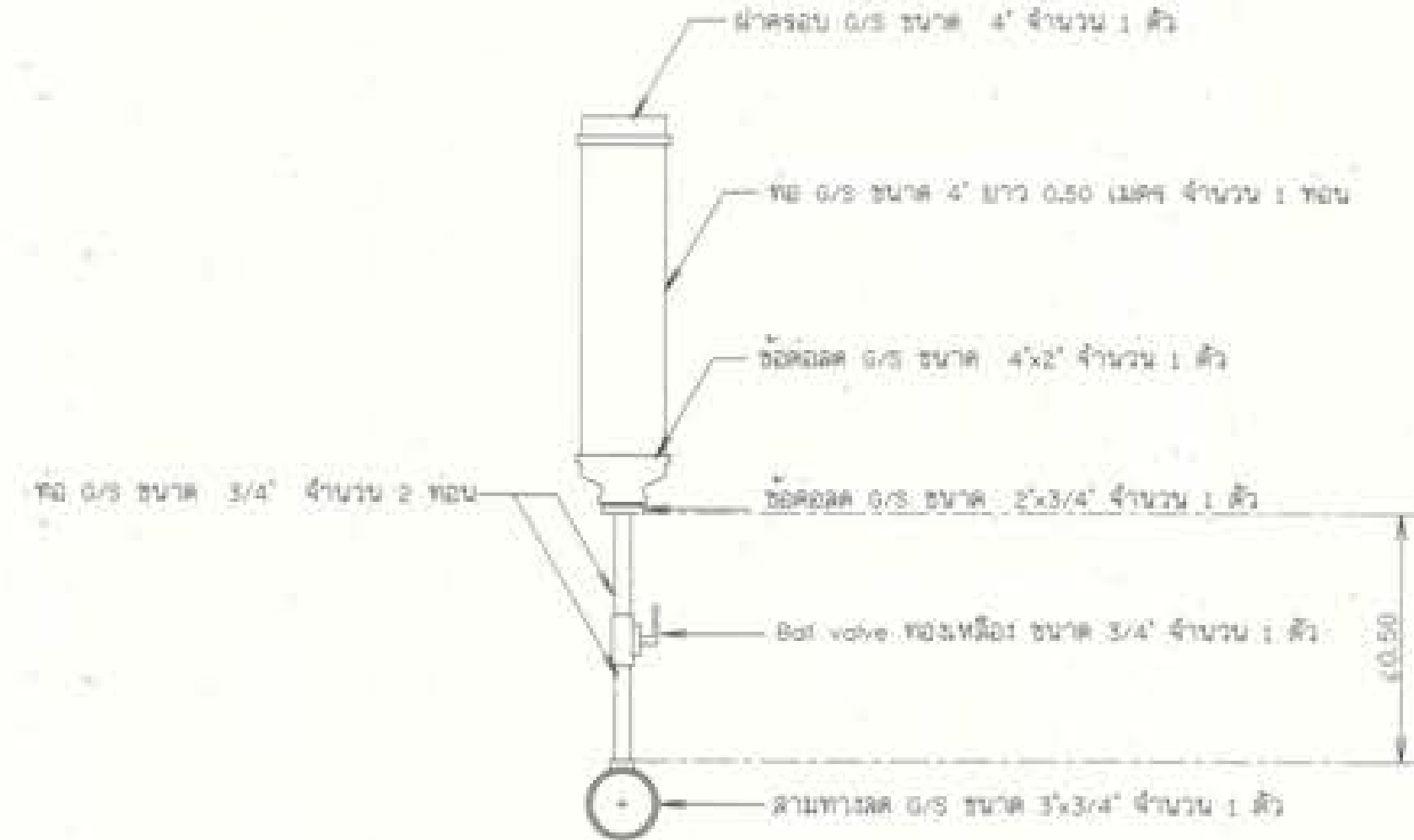
11. ช่องเติมน้ำ โมเดลมาตรฐาน
