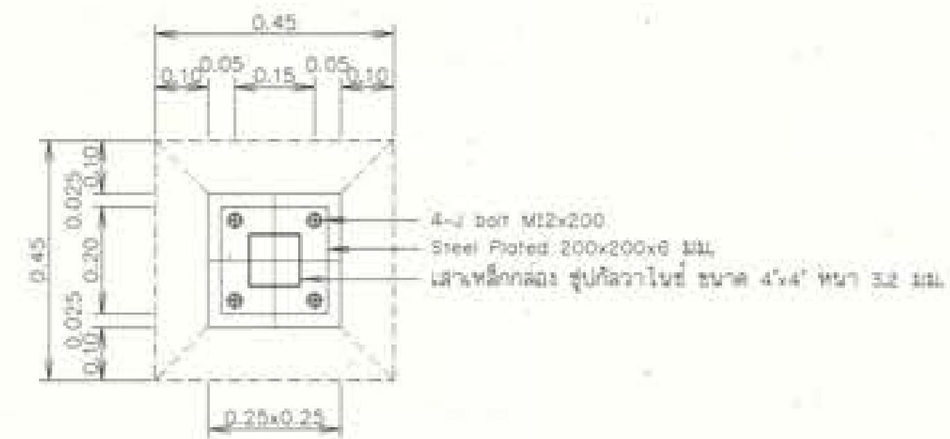
รูปตัด ก-ก ไม่แสดงขนาดราส่วน
