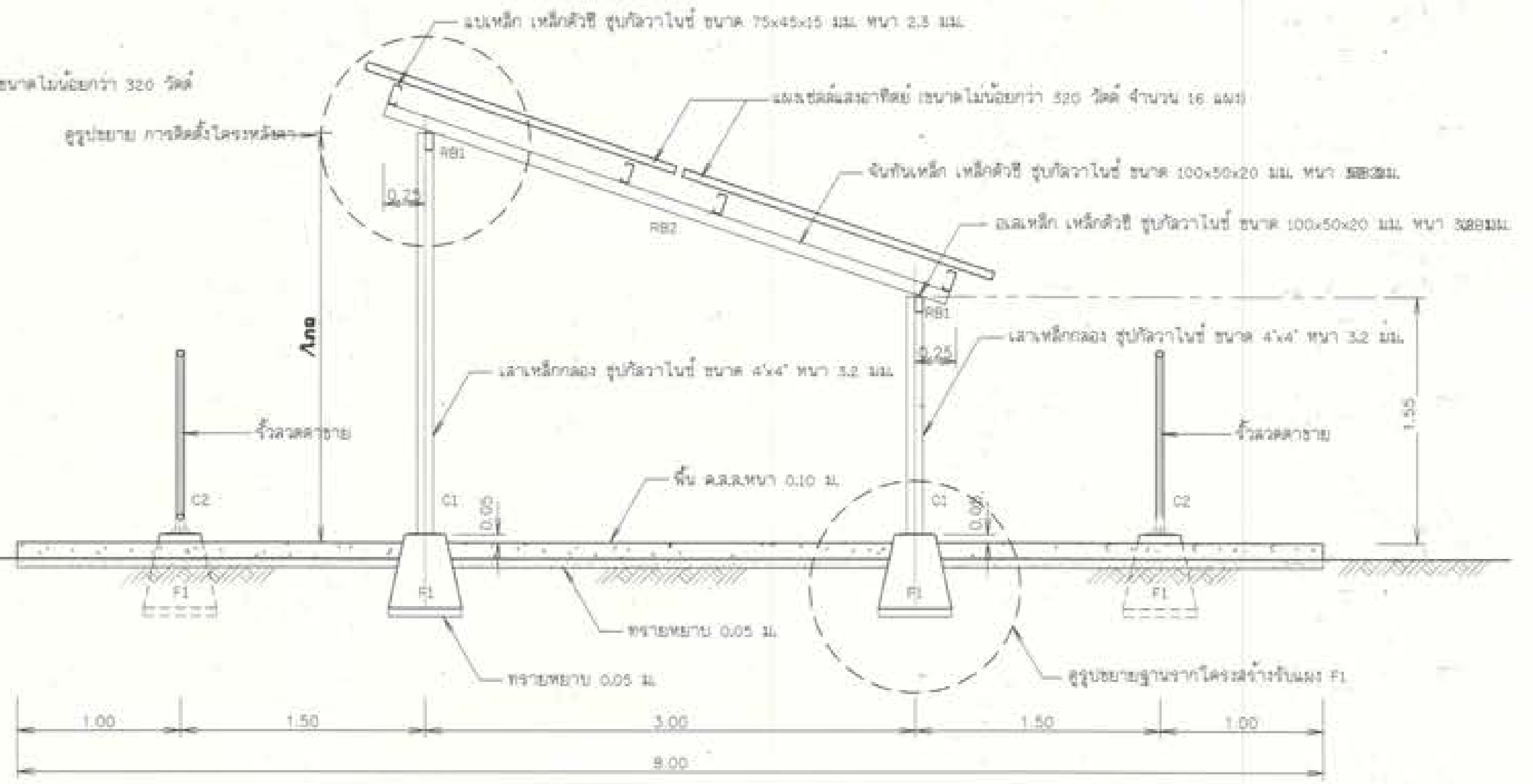
รูปด้านข้าง ไม่แสดงขนาดราส่วน
