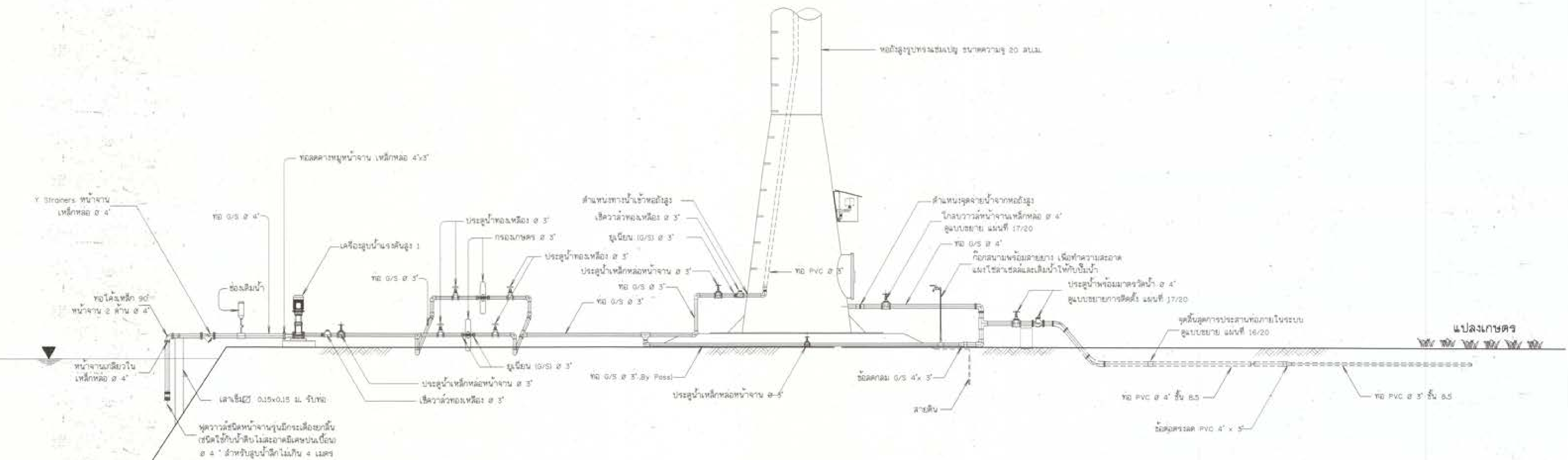
รูปแสดงรายละเอียดท่อและอุปกรณ์ระบบส่งน้ำพลังงานแสงอาทิตย์
