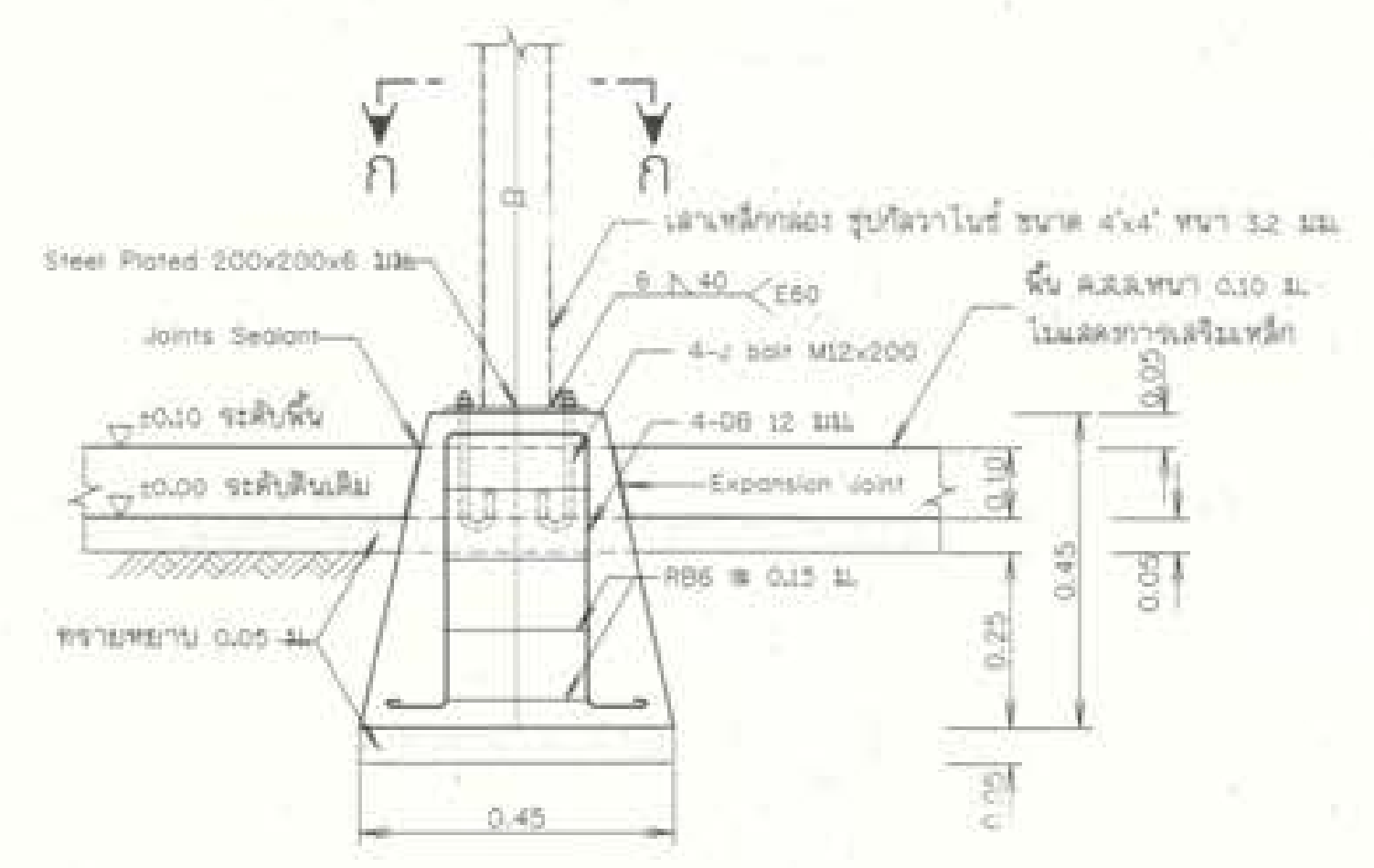
รูปขยายฐานรากโครงสร้างรับแผง F1 0.05m คม, ท่อสำหรับรูพ่นน้ำ ไม่แสดงขนาดราส่วน
