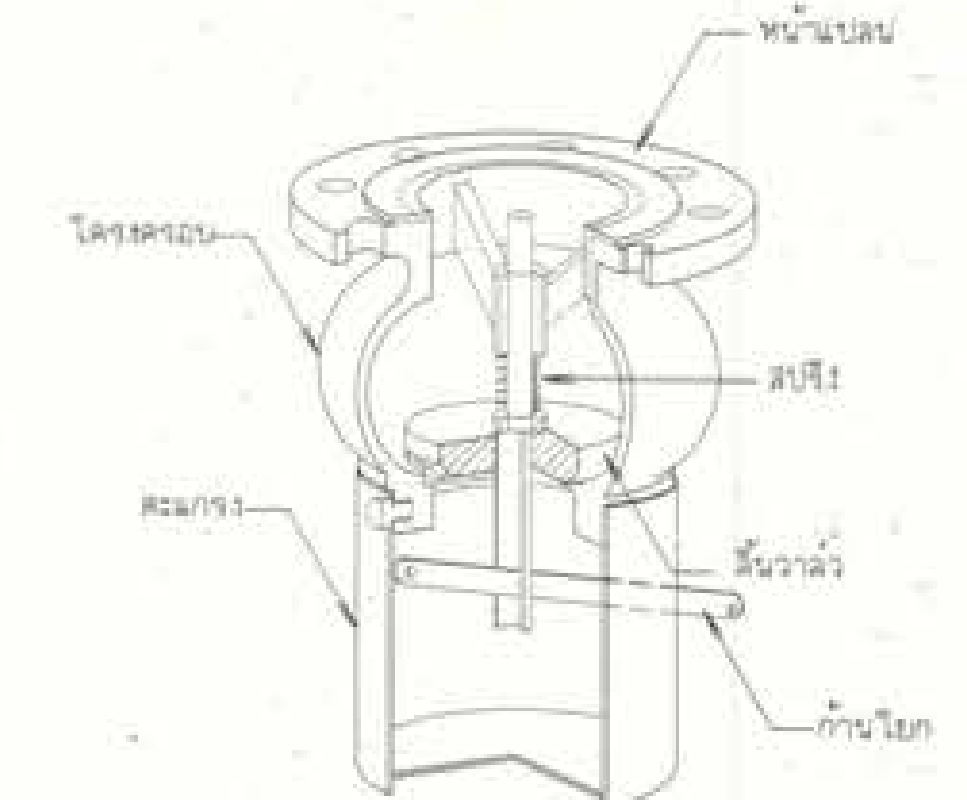
ฟุตวาล์ว แบบก้านโยก โมเดลมาตรฐาน
