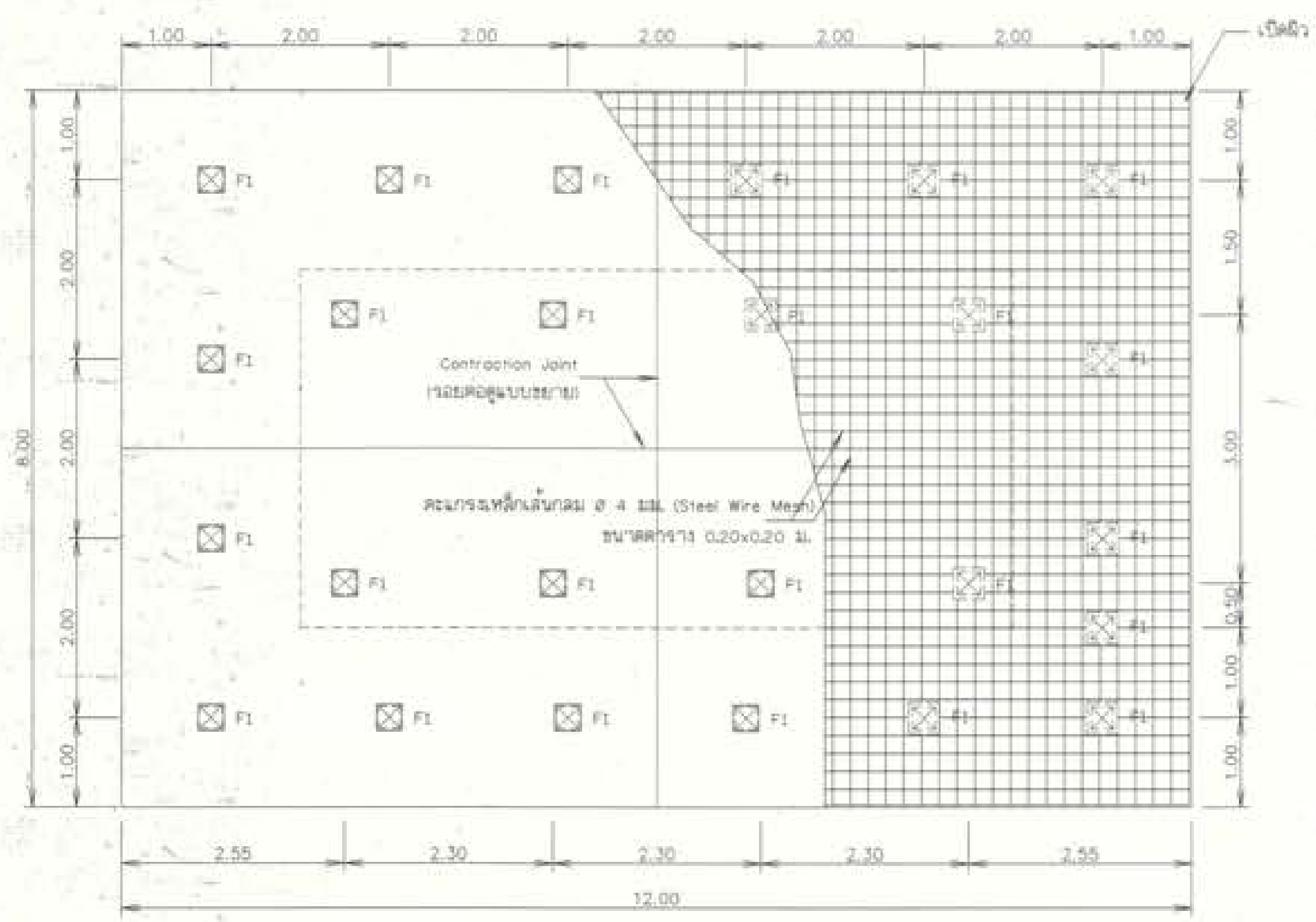
รูปขยายพื้นคอนกรีต ไม่แสดงขนาดราส่วน
