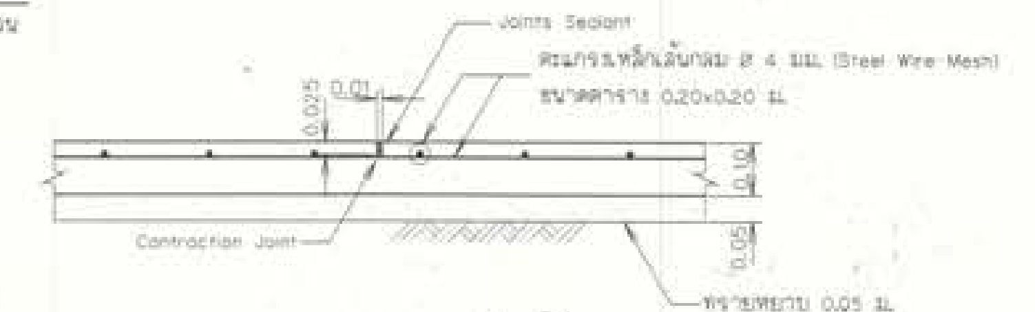
แบบขยายรอยต่อพื้น ไม่แสดงขนาดราส่วน
