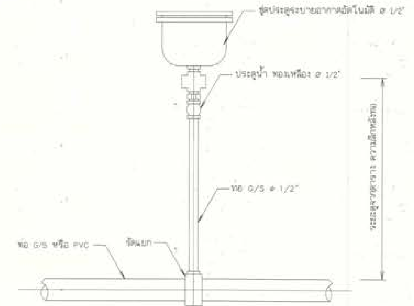
12. การติดตั้งประจุระบายอากาศอัตโนมัติ โมเดลมาตรฐาน
