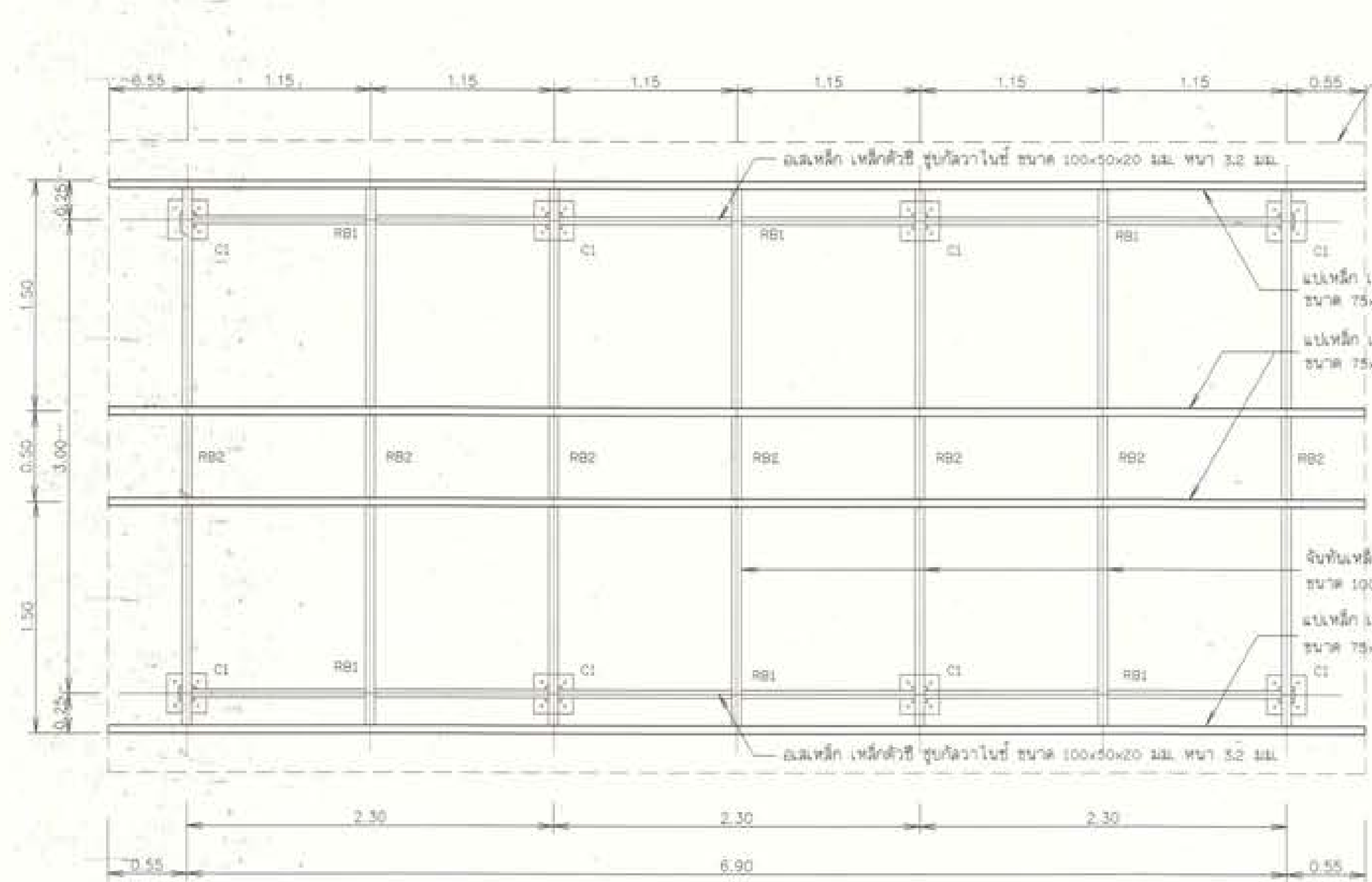
แปลนฐานรากและโครงหลังคา ไม่แสดงขนาดราส่วน
