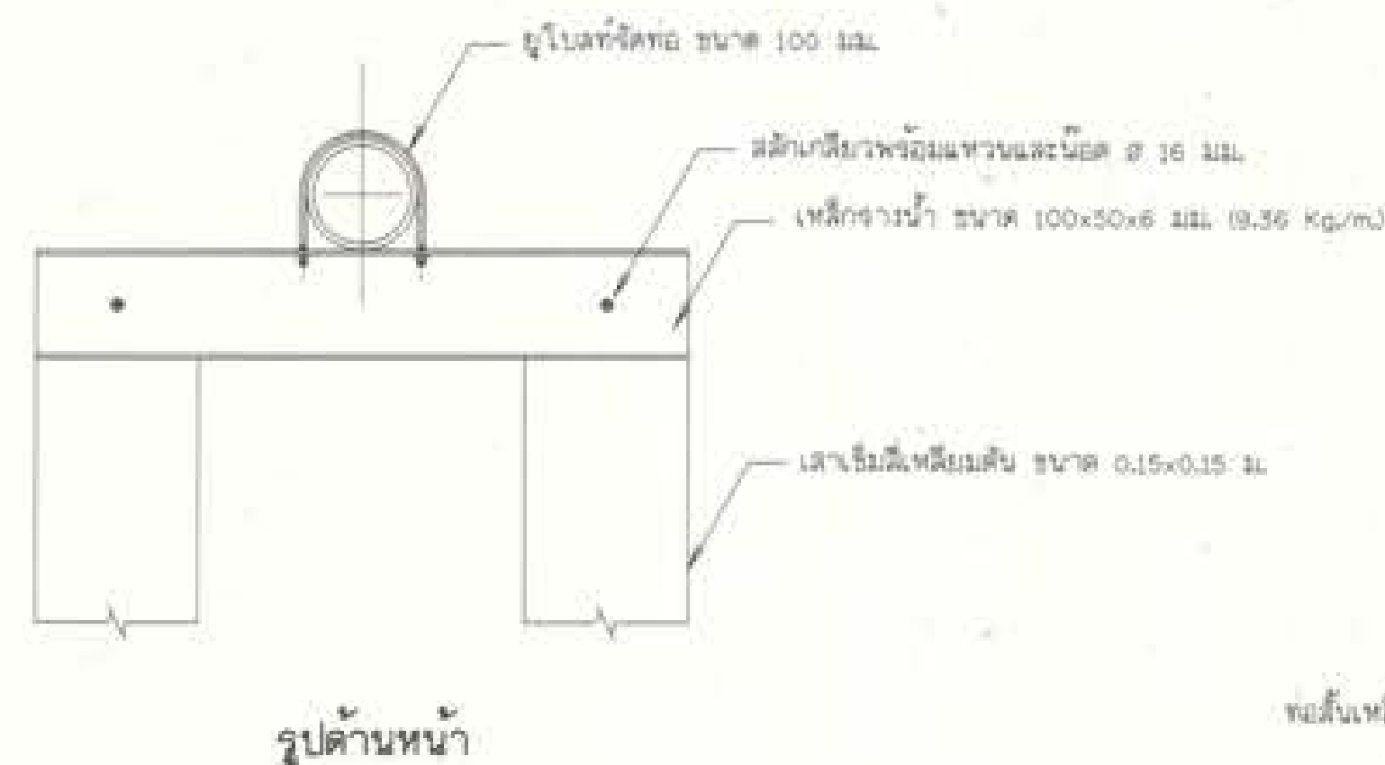
13. เสาคอนกรีตรับท่อดูด และแบบขยายอุปกรณ์รั่วท่อ โมเดลมาตรฐาน
