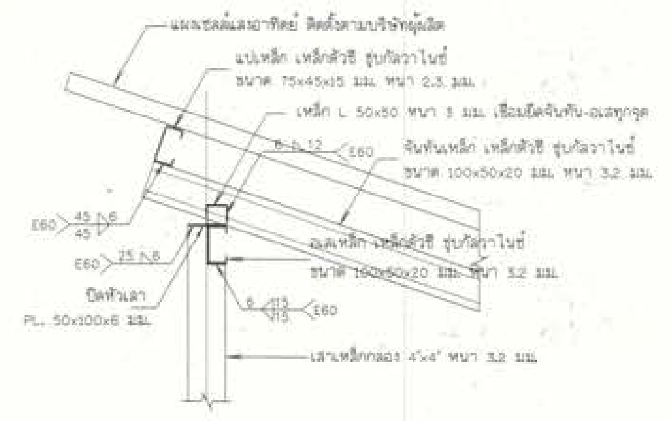
รูปขยาย การติดตั้งโครงหลังคา ไม่แสดงขนาดราส่วน
