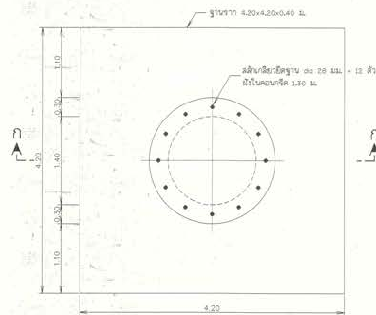
แปลน ฐานรากห่อถังสูง (แบบฐานแผ่)
