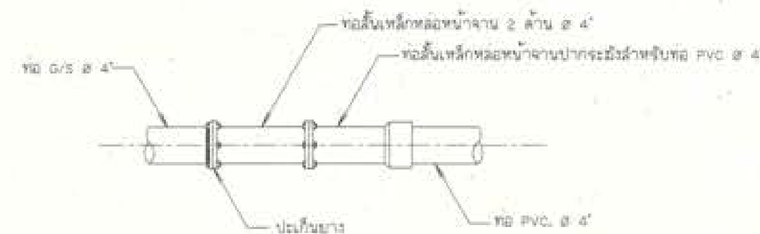
8. การบรรจุท่อเหล็กอาบสังกะสี G/S กับท่อ PVC. ไม่แสดงมาตรฐาน
