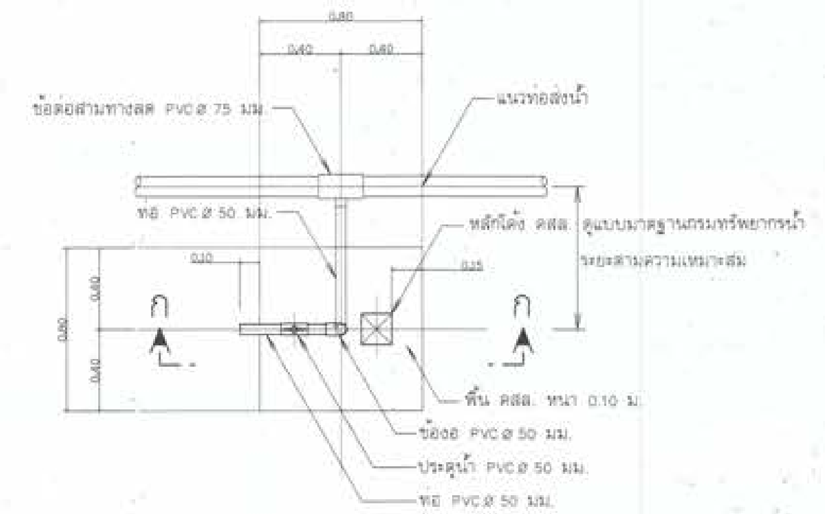
แปลงอาคารจุดปล่อยน้ำ
