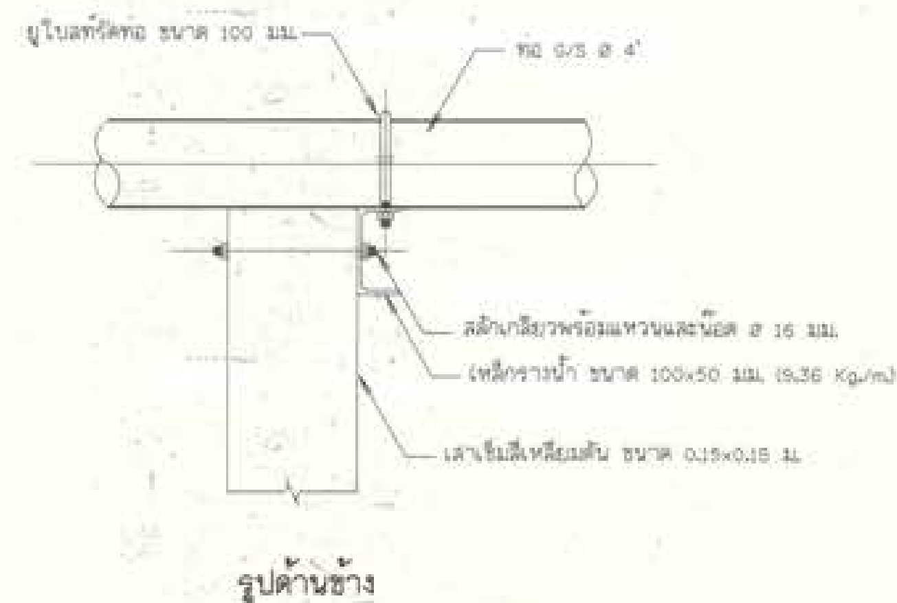
13. เสาคอนกรีตรับท่อดูด และแบบขยายอุปกรณ์รั่วท่อ โมเดลมาตรฐาน
