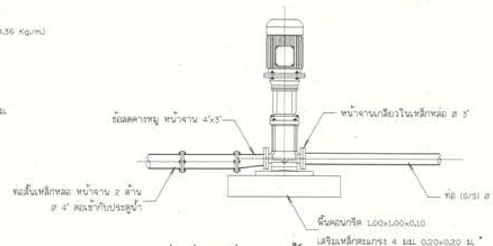
15. การต่อท่อเครื่องสูบน้ำ โมเดลมาตรฐาน
