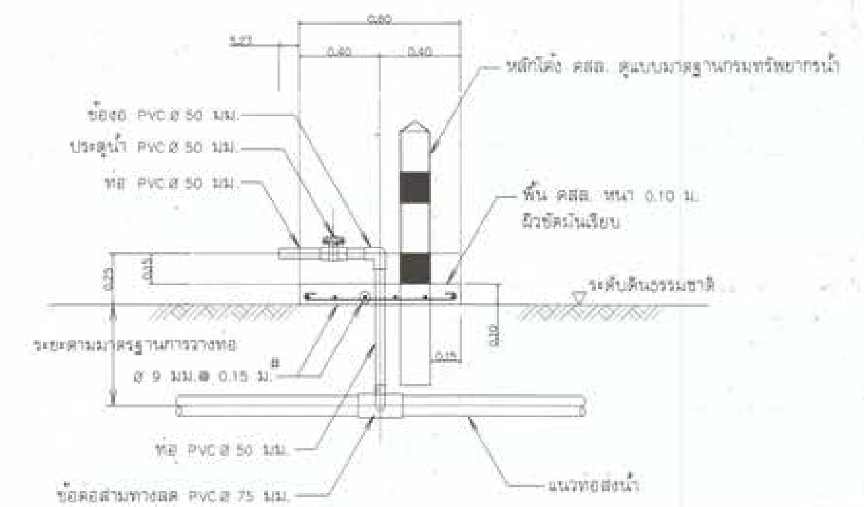
รูปตัด ก - ก แสดงการติดตั้งประตูจุดปล่อยน้ำ
