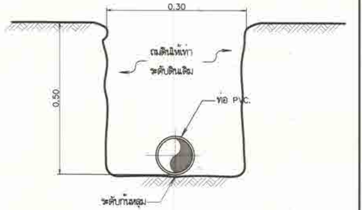
รูปตัดแสดงการวางท่อส่งน้ำ
