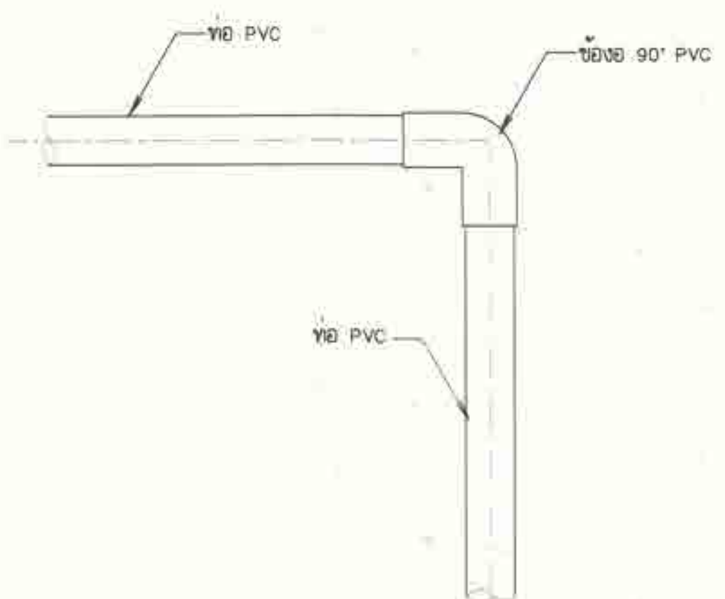
7. แบบการต่อข้อโค้ง 90° PVC ไม่แสดงมาตรฐาน
