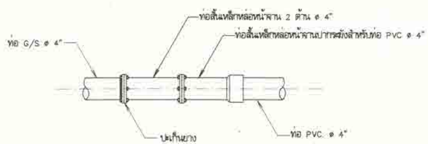
8. การบรรจบท่อเหล็กอบสังกะสี G/S กับท่อ PVC. ไม่แสดงมาตรฐาน
