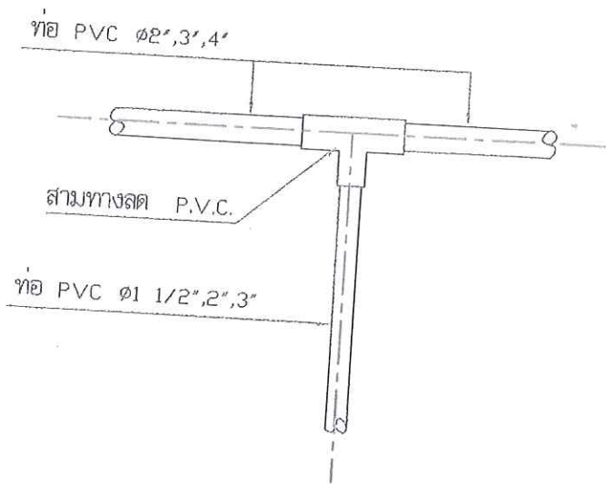
8. แบบการต่อสามทางลด PVC
