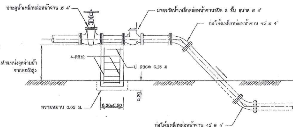
14. การติดตั้งมาตรวัดน้ำบนพื้นดิน ๕ 4" ไม่แสดงขนาดจาล้วน
