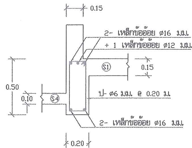
รูปตัด จ - จ 1:20
