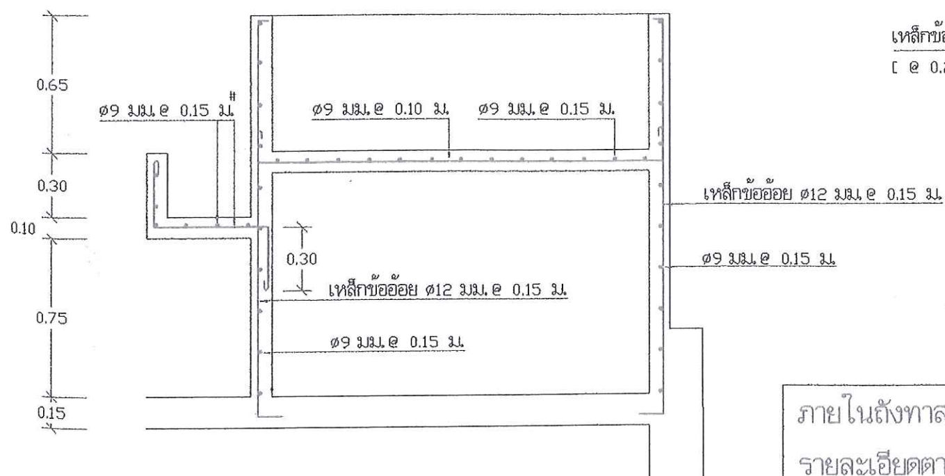
รูปตัด ๑ - ๑ 1:25
