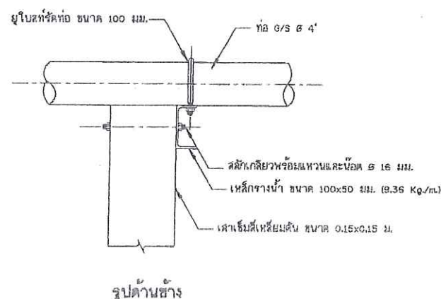
13. เสาคอมม่อนรับท่อชุด และแบบขยายอุปกรณ์รีดท่อ ไม่แสดงขนาดจาล้วน
