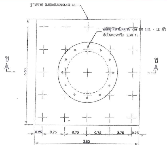
แปลน ฐานรากหอลังสูง (แบบเสาเข็ม)
