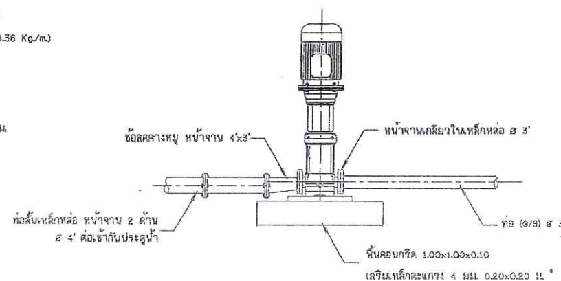
18. การต่อท่อเครื่องสูบน้ำ ไม่แสดงขนาดจาล้วน
