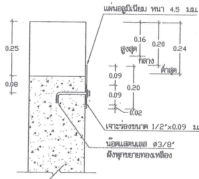
รูปตัด ญ - ญ 1 : 10
