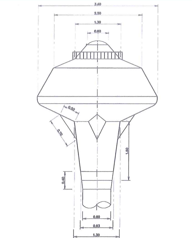
แบบขยายแมนโฮลบนท่อถึงสูง ไม่แสดงมาตราส่วน
