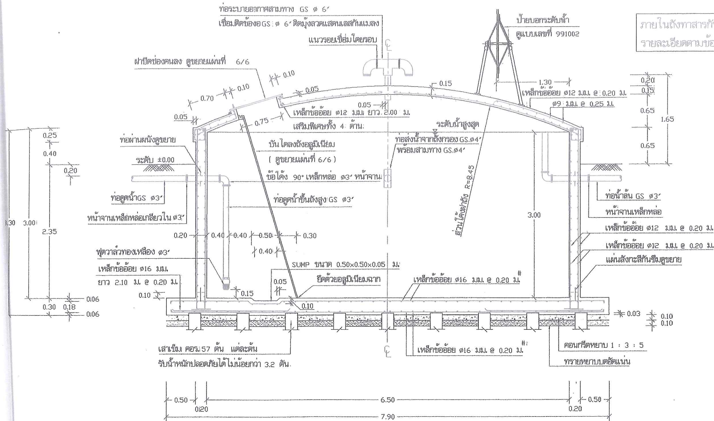
รูปตัด ก - ก 1 : 40
