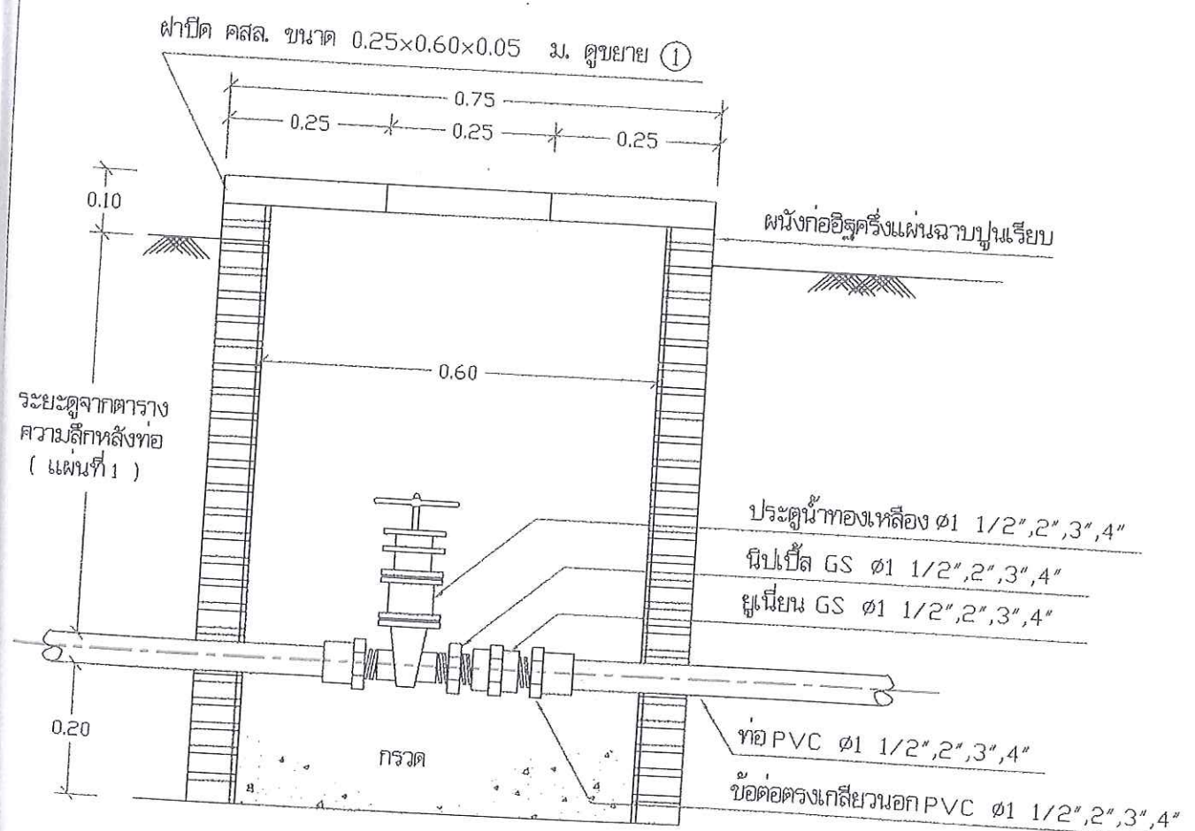
10. แบบการติดตั้งประตุน้ำทองเหลือง \phi 1 1/2', 2', 3', 4'' 1:10
