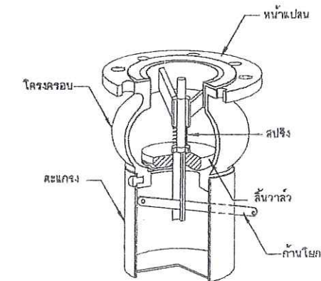
15. ฟุตวาล์ว แบบก้านโยก ไม่แสดงขนาดจาล้วน
