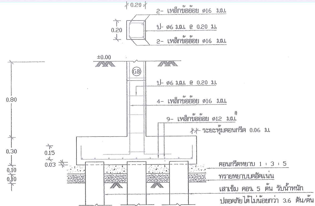
รูปตัด ฉ - ฉ 1:20
