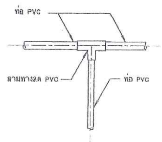
9. แบบการต่อสามทางลด PVC ไม่แสดงขนาดจาล้วน
