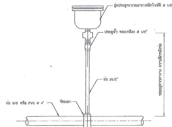
12. การติดตั้งประตูละบายอากาศอัตโนมัติ ไม่แสดงขนาดจาล้วน
