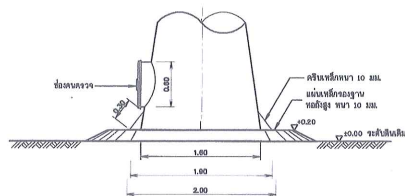
แบบขยายแมนไฮล์ล่างหอดึงสูง ไม่แสดงมาตราส่วน
