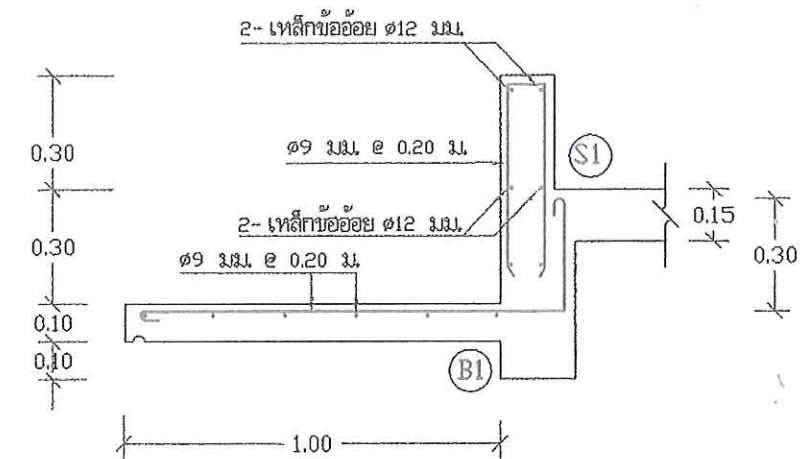
แบบแสดงการเสริมเหล็กพื้นกันสาด (จ) 1 : 20
