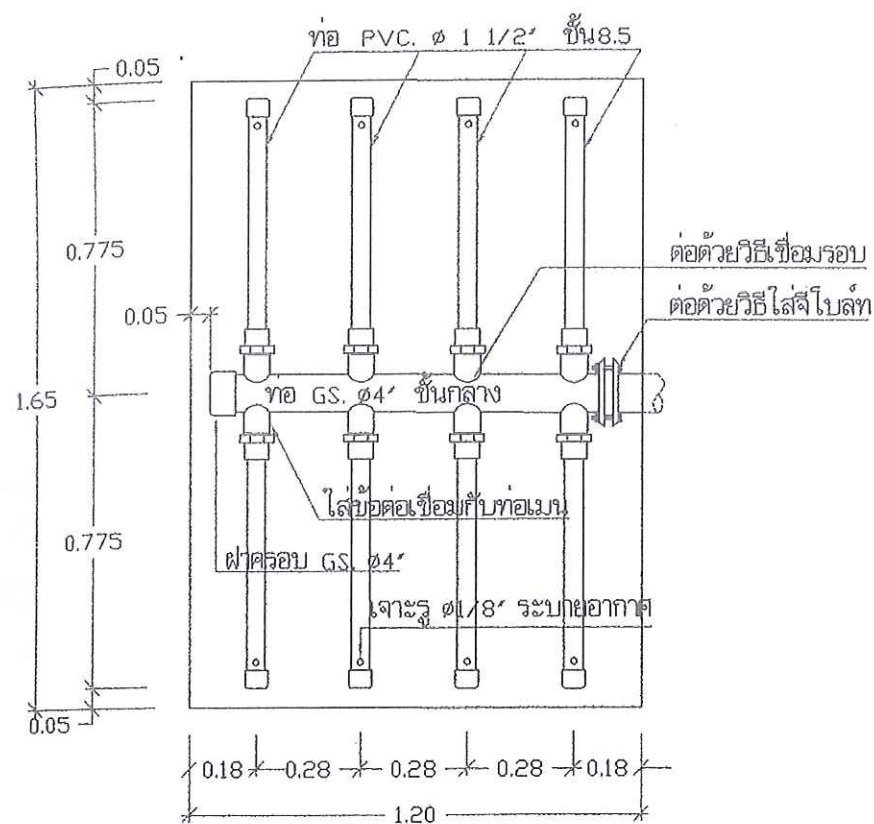
แบบขยายท่อทางปลา 1:20
