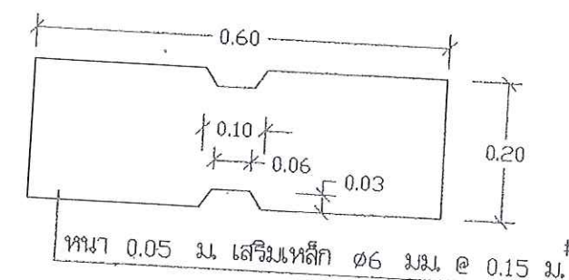
รูปขยาย ② 1:10
