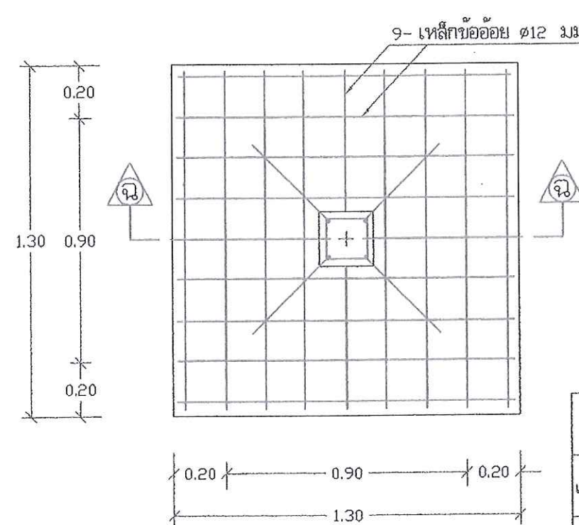
แบบขยายฐานราก F 2 (แบบดอกเข็ม) 1:20
