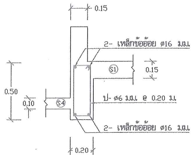
รูปตัด จ - จ 1:20
