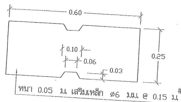
รูปขยาย ① 1:10
