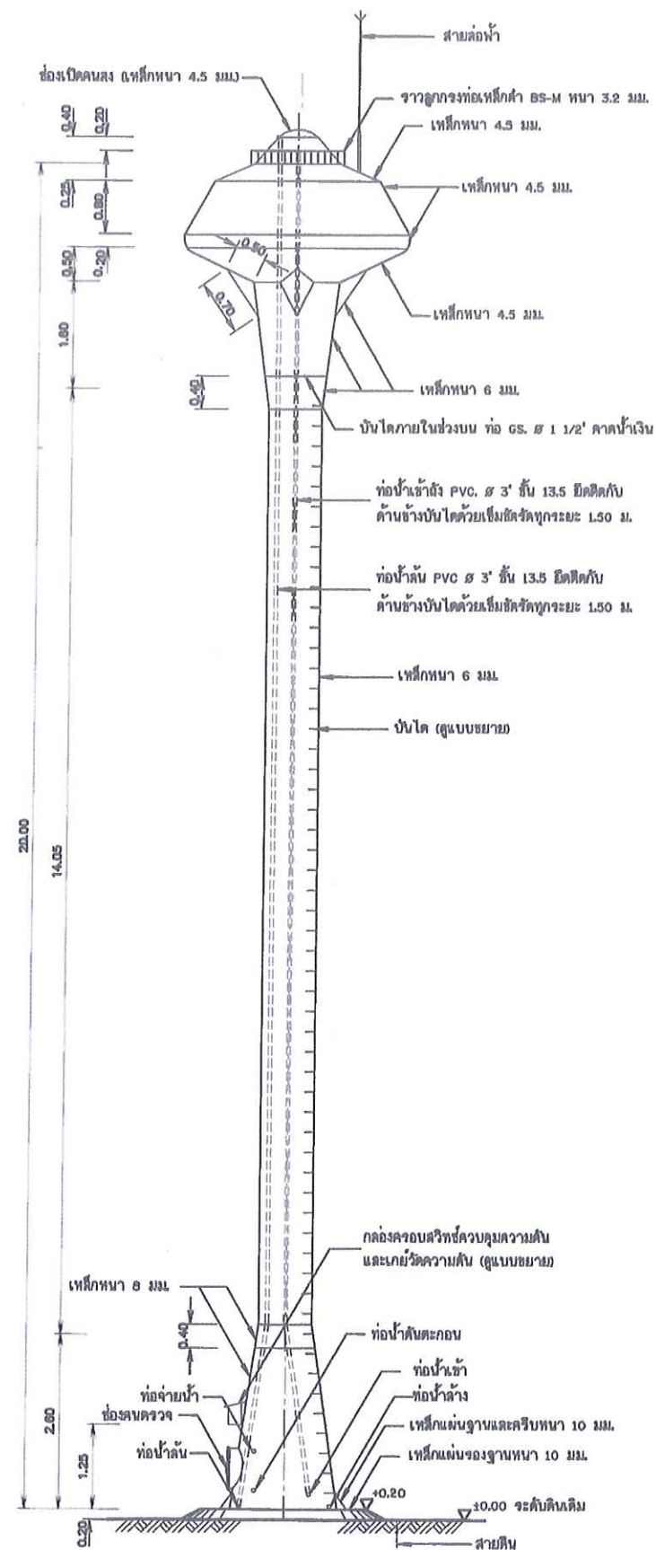
รูปด้านข้างทอดถึงสูง แบบถึงเหล็กรูปทรงแฉมแปญ ไมแสดงนตราส่วน
