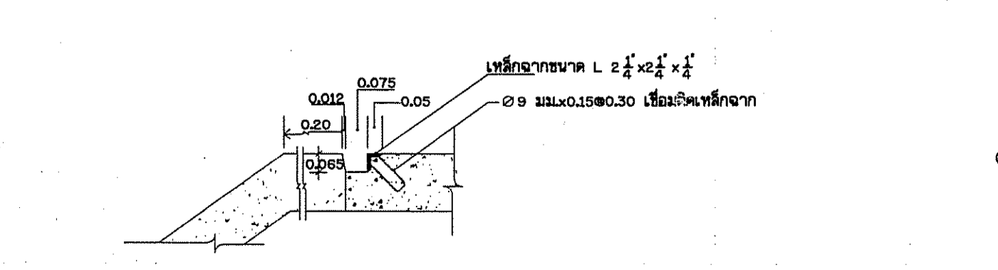
ขยายร่องใส่บานประตูไม้ ไม่แสดงมาตราส่วน
