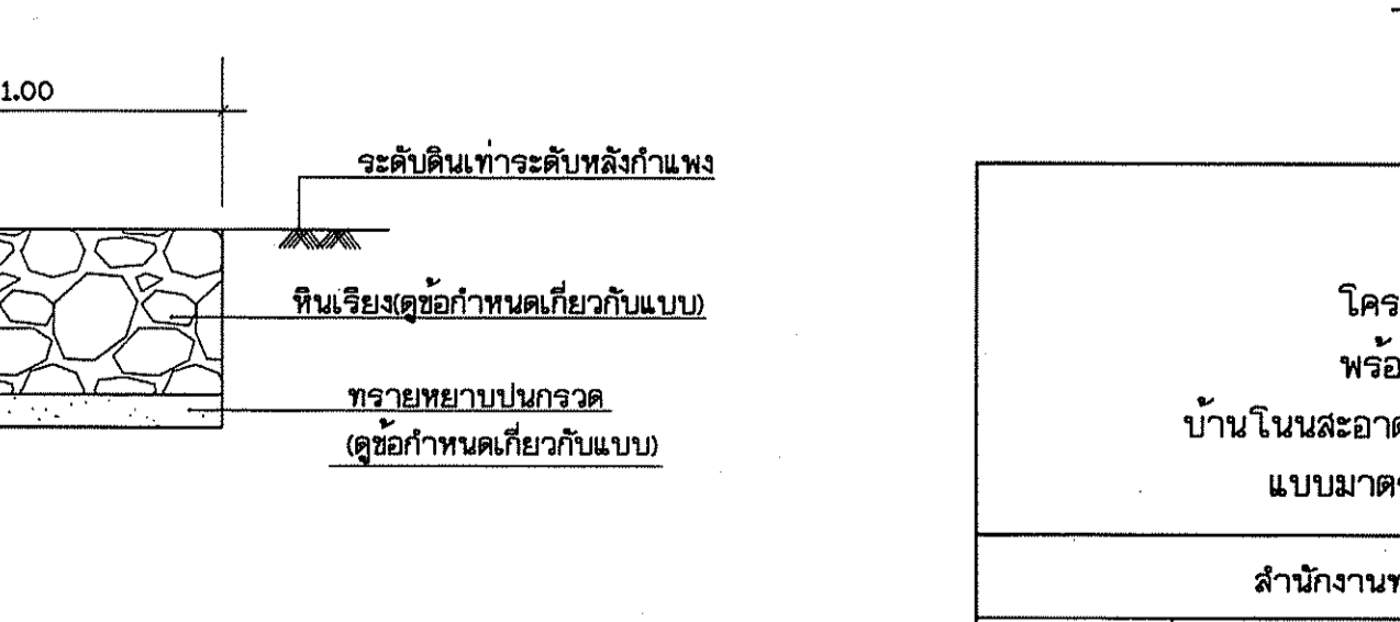
ขยายหินเรียง 2 ไม่แสดงมาตราส่วน
