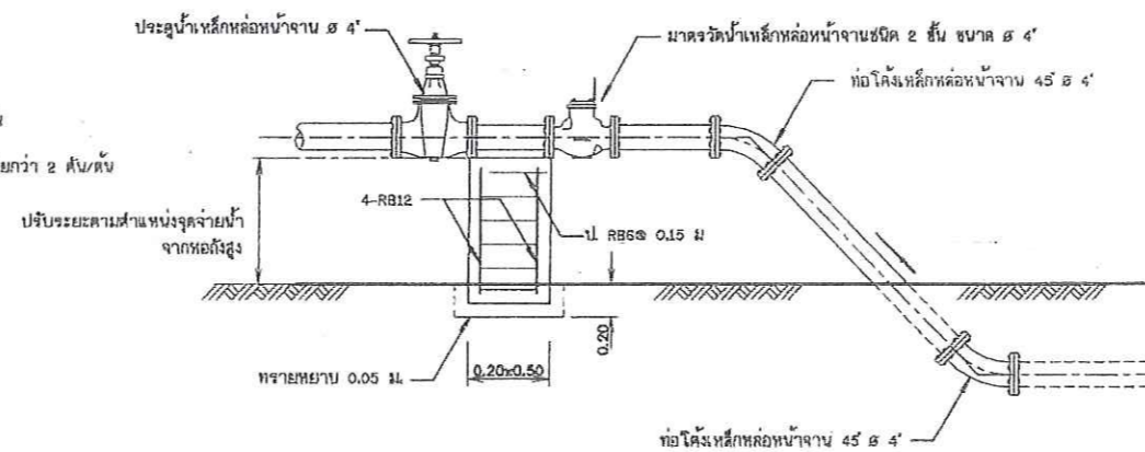
14. การติดตั้งมาตรวัดน้ำบนพื้นดิน 1/2\"/>
