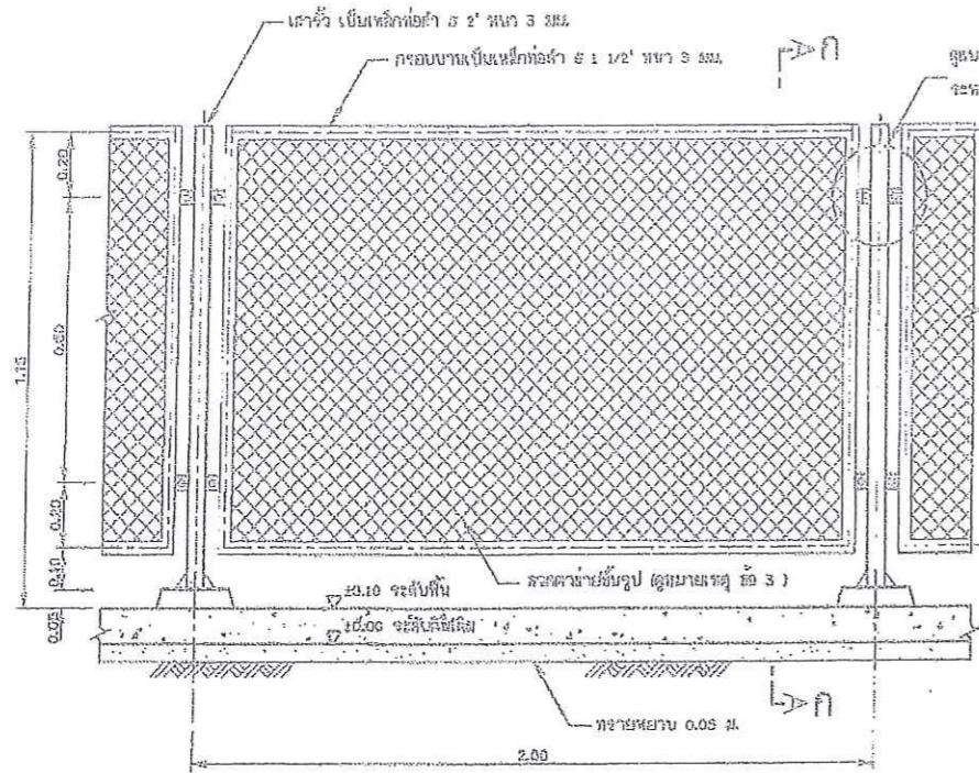
แบบขยายรั้วลวดตาข่าย ไม่แสดงขนาดจั่ว
