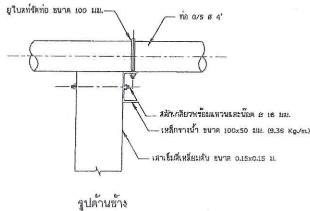
13. เสาต่อมอรับท่อวัด และแบบขยายอุปกรณ์วัดท่อ ไม่แสดงมาตราส่วน
