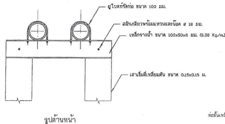
13. เสาต่อมอรับท่อวัด และแบบขยายอุปกรณ์วัดท่อ ไม่แสดงมาตราส่วน
