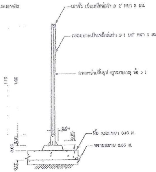
รูปตัด ก-ก ไม่แสดงขนาดจั่ว
