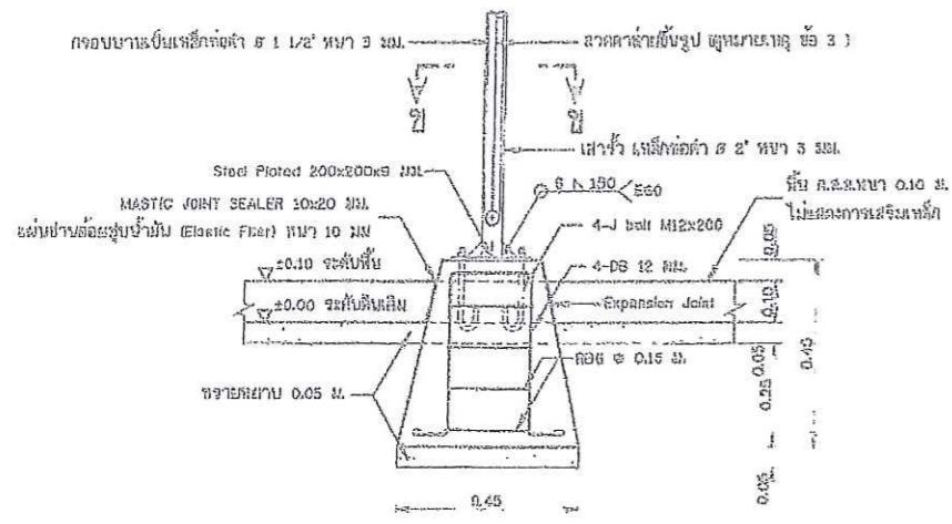
รูปขยายฐานจากโครงสร้างรับแผง F1 ถอมัด ศสส. หรือสำหรับจุดรับน้ำหนักอื่น ไม่แสดงขนาดจั่ว
