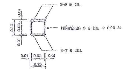
รูปตัด ข-ข ไม้ระแนงพลาสติก
