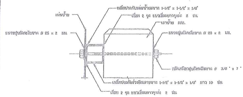
รูปตัดขยายการยึดแผ่นป้ายและเสา ไม้ระแนงพลาสติก
