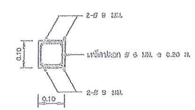
รูปตัด ก-ก ไม้ระแนงพลาสติก
