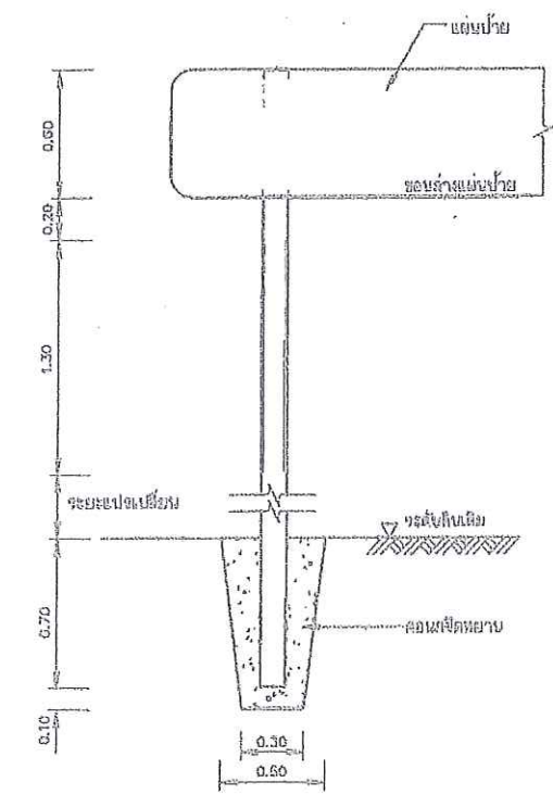
รายละเอียดการติดตั้งเสาป้าย ไม้ระแนงพลาสติก
