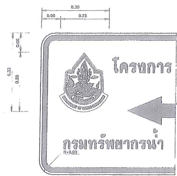
ป้ายแนะนำโครงการ ไม้ระแนงพลาสติก
