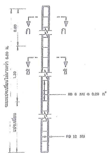
รายละเอียดเสาป้าย คสล. ไม้ระแนงพลาสติก
