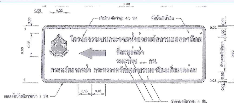
ป้ายแนะนำโครงการ ไม้ระแนงพลาสติก
