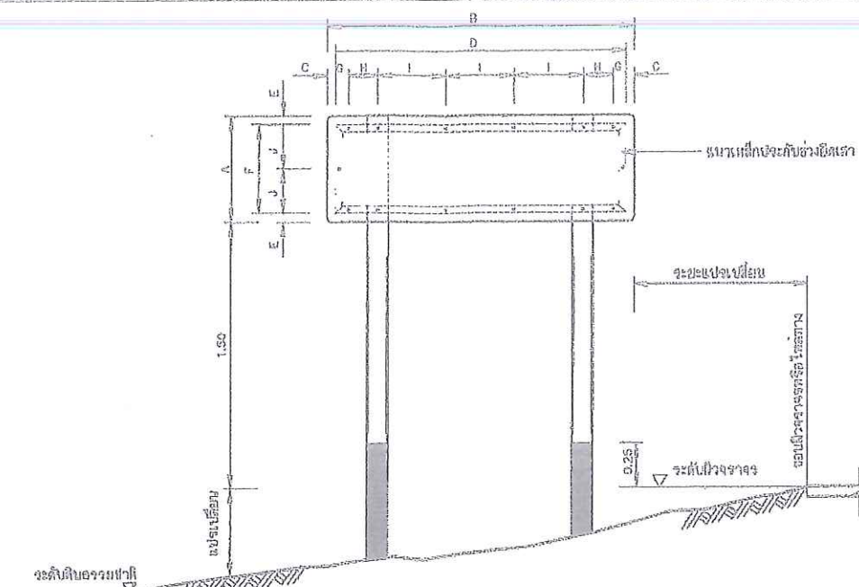
รูปแสดงการประกอบแผ่นป้าย ไม้ระแนงพลาสติก
