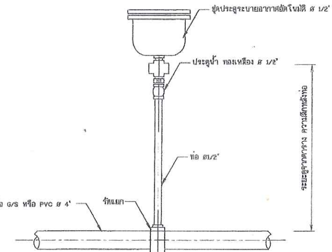
12. การติดตั้งประตูละบายอากาศอัตโนมัติ ไม่แสดงขนาดบางส่วน
