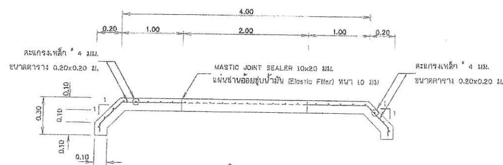
รูปตัด ค-ค ไม่แสดงขนาดจาลัว
