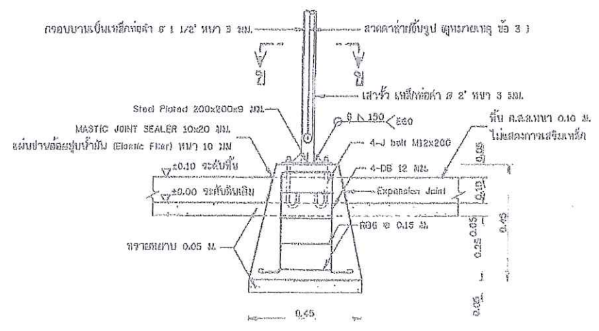
รูปขยายฐานรากโครงสร้างรับแผง F1 คอนกรีต คสล. หรือสำหรับรูปหล่อค้ำตั้ง ไม่แสดงขนาดส่วน
