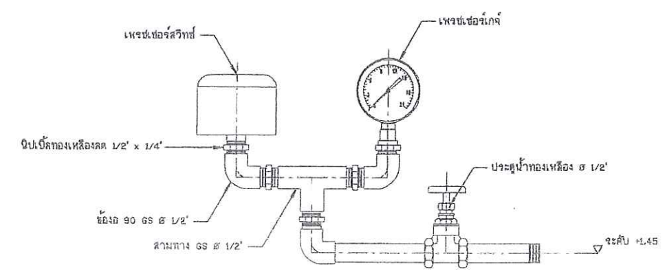
แบบขยายสวิตช์ควบคุมและเกจวัดความดัน ไม่แสดงมาตราส่วน
