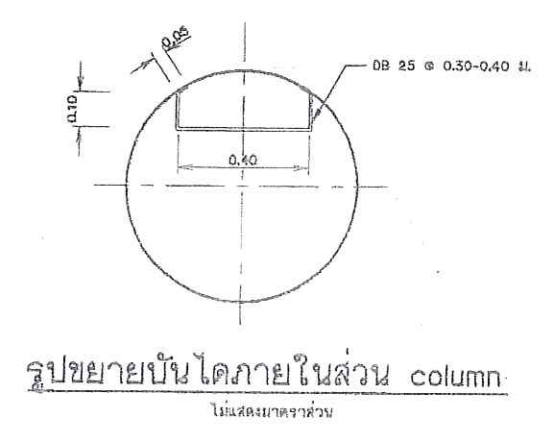
แบบขยายบันได ภายในหอถังสูง ไม่แสดงมาตราส่วน
