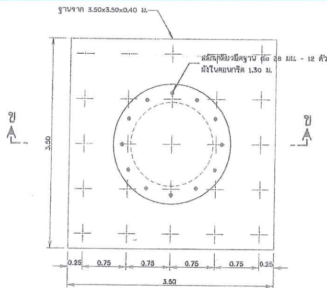
แปลน ฐานรากห่อถังสูง (แบบเสาเข็ม) ไม่แสดงขนาดจาลัว
