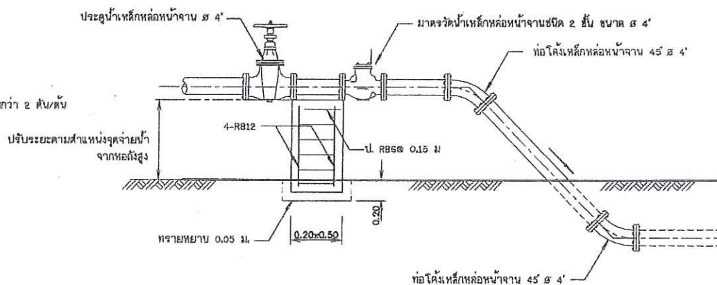
14. การติดตั้งมาตรวัดน้ำบนพื้นดิน ๕ 4" ไม่แสดงขนาดบางส่วน
