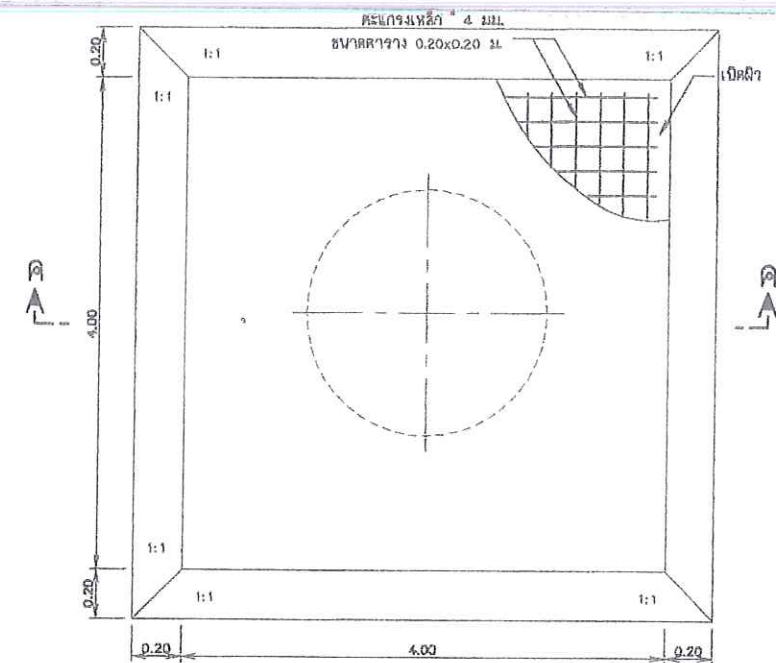
แปลนพื้นคอนกรีตเสริมเหล็ก ไม่แสดงขนาดจาลัว
