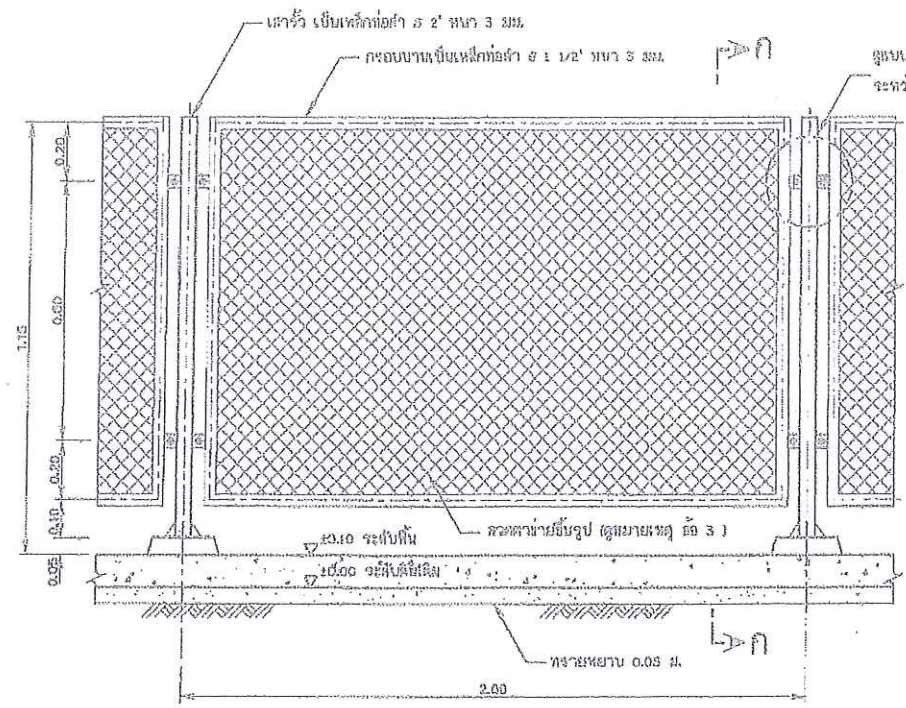
แบบขยายรั้วลดตาข่าย ไม่แสดงขนาดส่วน
