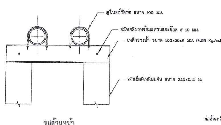
13. เสาต่อม่อรับท่อชุด และแบบขยายอุปกรณ์รัดท่อ ไม่แสดงขนาดบางส่วน
