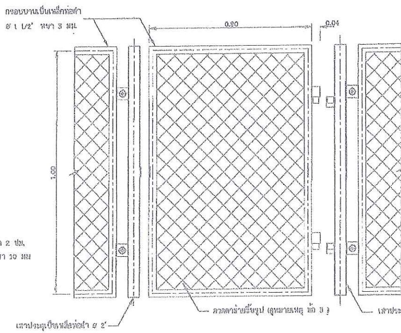
แบบขยายรายละเอียดประตู ไม่แสดงขนาดส่วน
