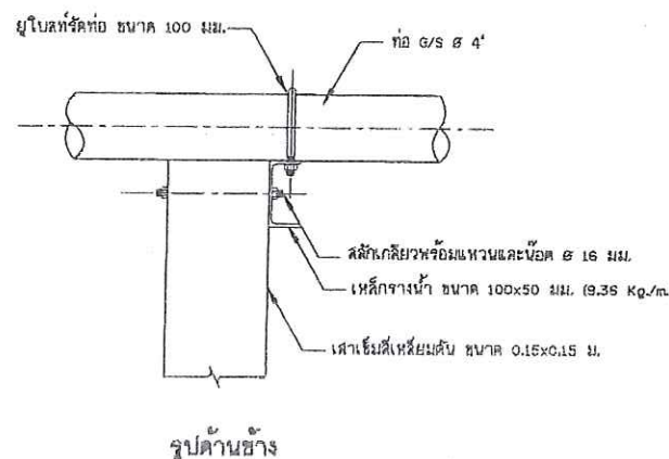
13. เสาต่อม่อรับท่อชุด และแบบขยายอุปกรณ์รัดท่อ ไม่แสดงขนาดบางส่วน
