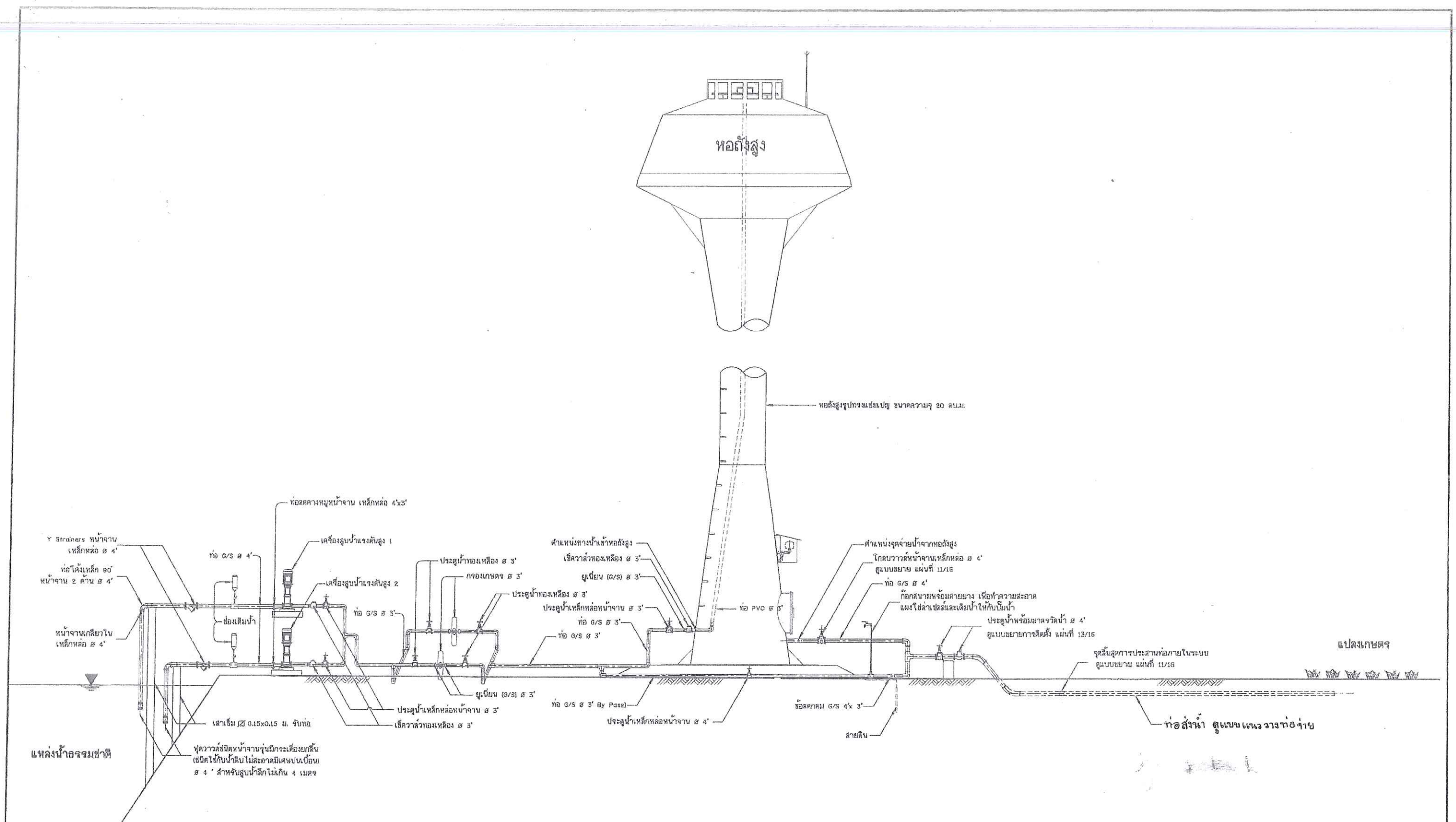
รูปแสดงรายละเอียดท่อและอุปกรณ์ระบบส่งจ่ายน้ำพลังงานแสงอาทิตย์ ไม่แสดงมาตราส่วน
