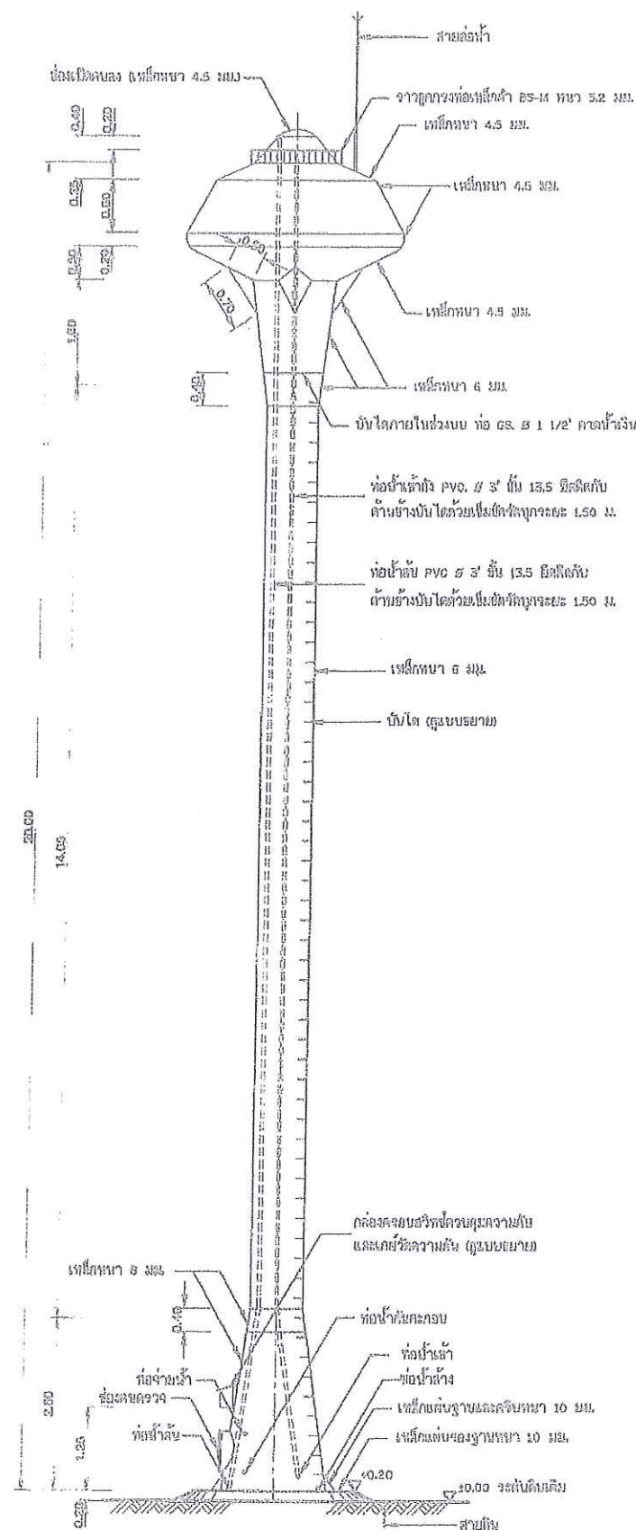
รูปด้านข้างพอดีสูง แบบต้นหลักรูปทรงแฝงอยู่
