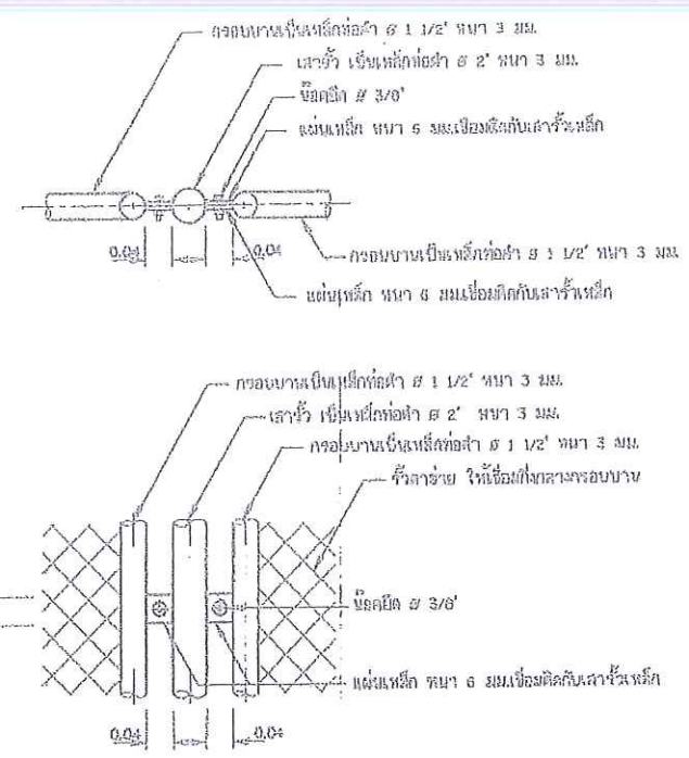
แบบขยายรายละเอียดแสดงการยึดระหว่างรั้วกับเสา ไม่แสดงขนาดส่วน
