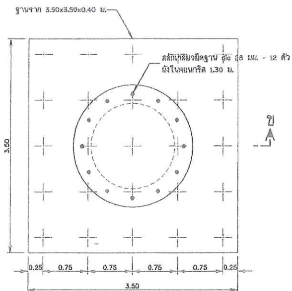
แปลน ฐานรากหอลังสูง (แบบเสาเข็ม)
