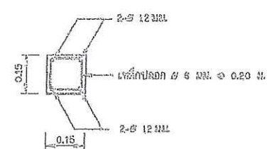
รูปตัด ก-ก โหนดและจุดรวม
