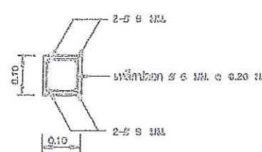
รูปตัด ก-ก ไม้แสดงมาตรฐาน
