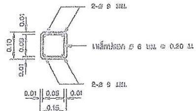
รูปตัด ข-ข ไม้แสดงมาตรฐาน
