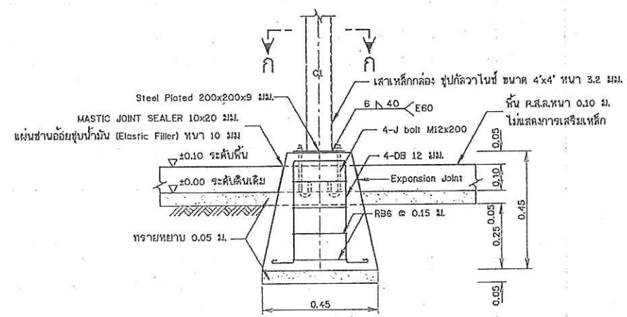
รูปขยายฐานรากโคจรลงรับแรงแผ่ F1 (ขณะเปิด คลส. หลังสำเร็จรูปพร้อมติดตั้ง) ไม่แสดงมาตราส่วน
