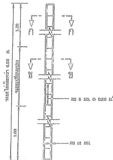
รายละเอียดภายใน คลัง
