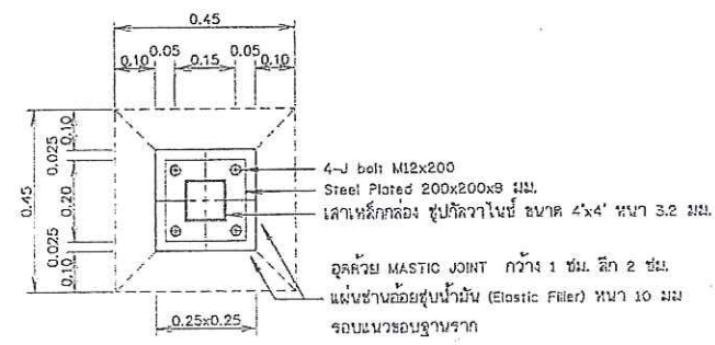
รูปตัด ก-ก โรงเรียนบดินทรเดชา
