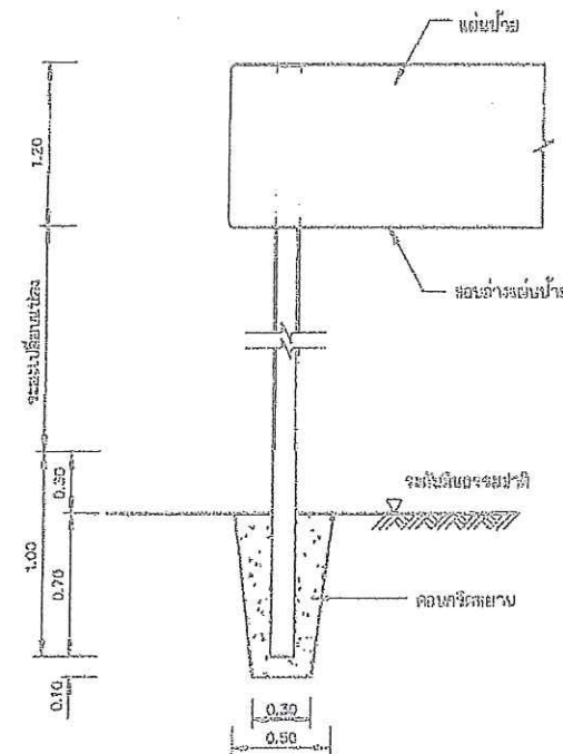
รายละเอียดการติดตั้งเสาน้ำยา โมเดลเบรจด์
