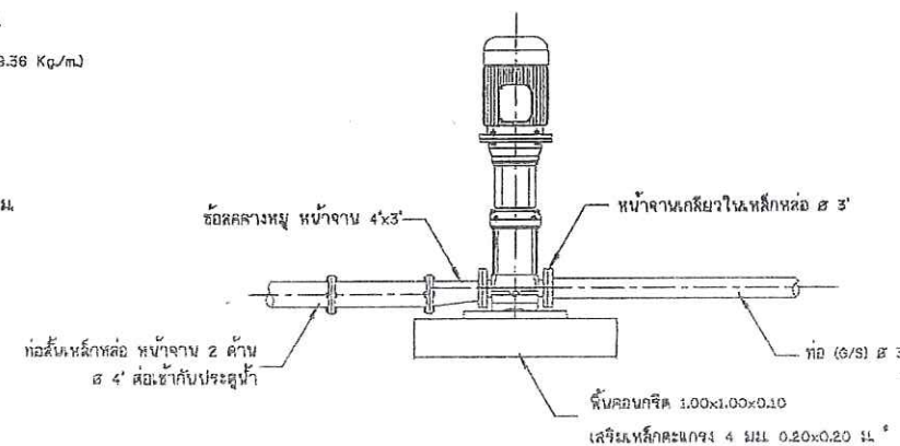
15. การต่อท่อเครื่องสูบน้ำ ไม่แสดงขนาดบางส่วน
