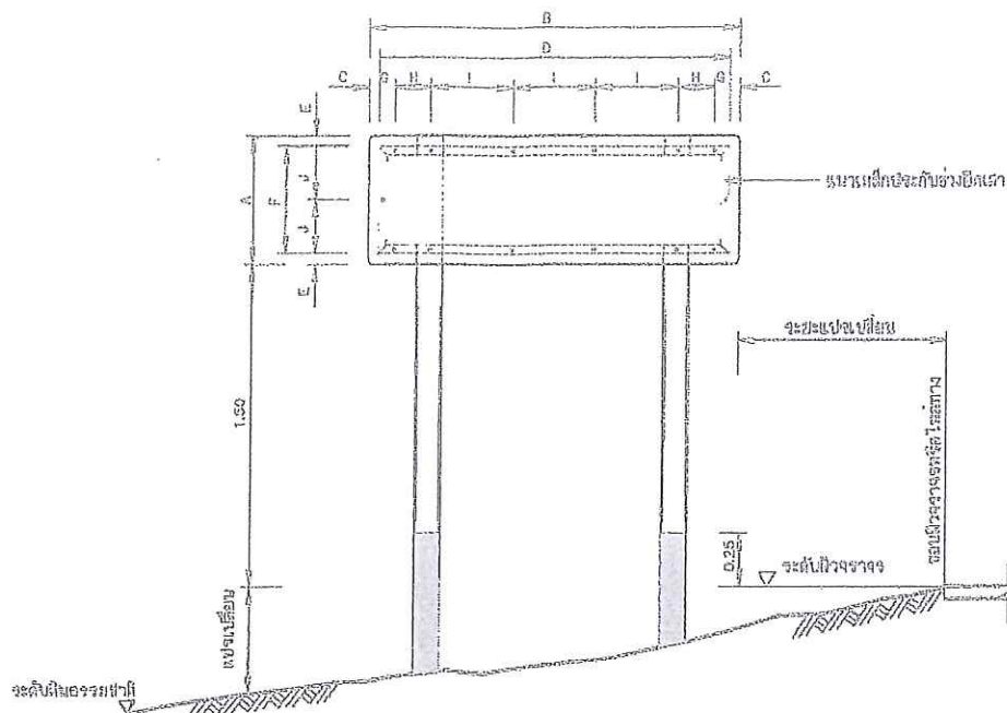
รูปแสดงการประกอบแผ่นป้าย ไม้แสดงมาตรฐาน
