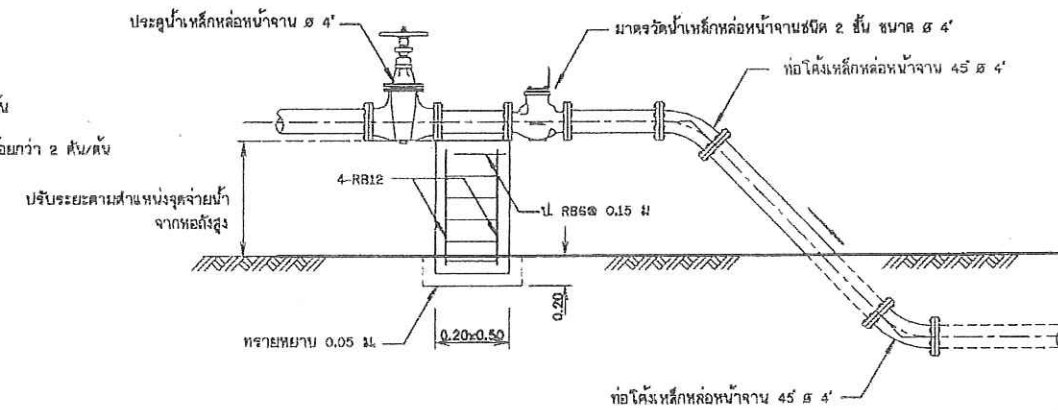
14. การติดตั้งมาตรวัดน้ำบนพื้นดิน ๕ 4" ไม่แสดงขนาดบางส่วน
