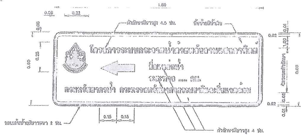
ป้ายแนะนำโครงการ ไม้แสดงมาตรฐาน
