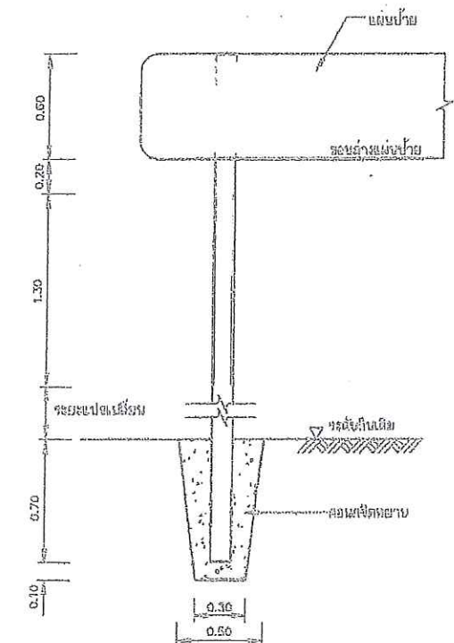
รายละเอียดการติดตั้งเสาป้าย ไม้แสดงมาตรฐาน
