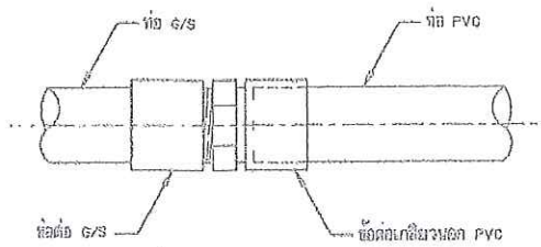
2. แบบการต่อท่อ G/S กับท่อ PVC ไม่แสดงขนาดจากรายงาน
