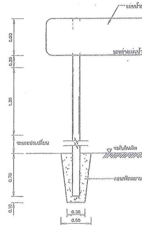
รายละเอียดการติดตั้งเสาป้าย ไม้แป้นขนาดจั่วส่วน
