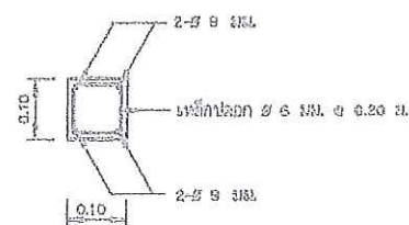
รูปตัด ก-ก ไม้แป้นขนาดจั่วส่วน
