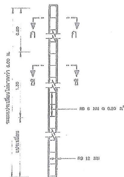
รายละเอียดเสาป้าย คสล. ไม้แป้นขนาดจั่วส่วน
