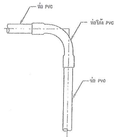
6. แบบการต่อท่อโค้ง 90° PVC ไม่แสดงขนาดจากรายงาน
