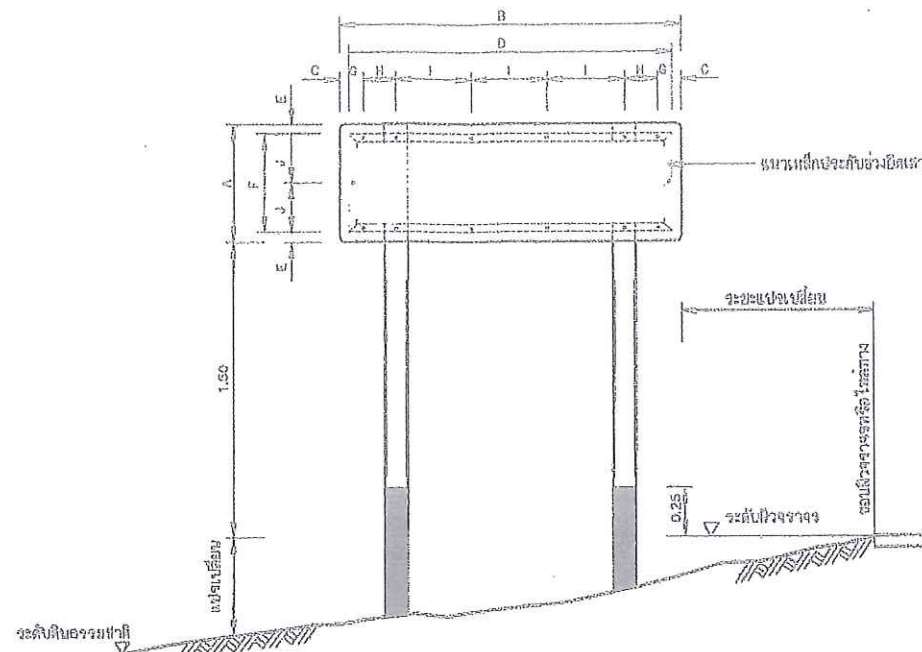
รูปแสดงการประกอบแผ่นป้าย ไม้แป้นขนาดจั่วส่วน
