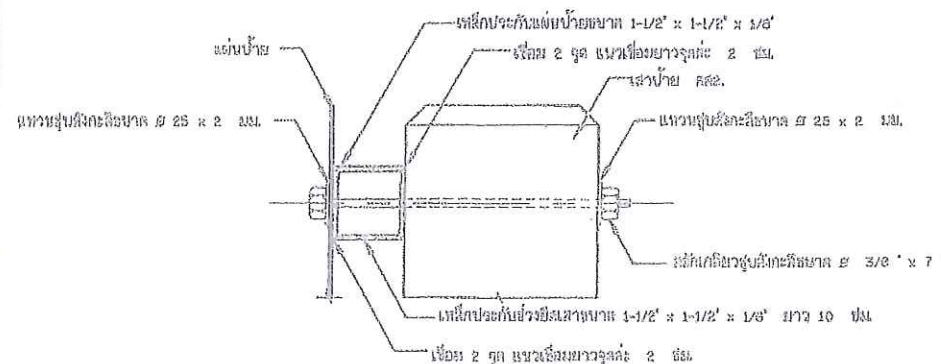
รูปตัดขยายการยึดแผ่นป้ายและเสา ไม้แป้นขนาดจั่วส่วน
