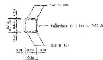
รูปตัด ข-ข ไม้แป้นขนาดจั่วส่วน
