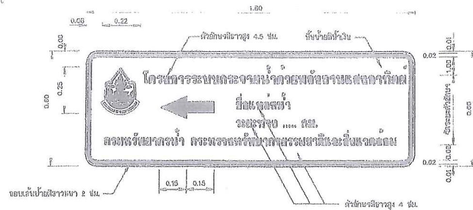
ป้ายแนะนำโครงการ ไม้แป้นขนาดจั่วส่วน
