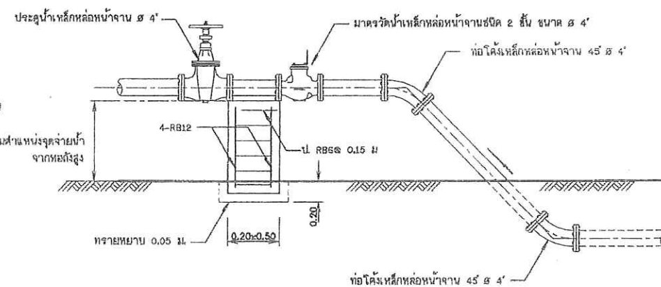
14. การติดตั้งมาตรวัดน้ำบนพื้นดิน 2' 4" ไม่แสดงมาตราส่วน
