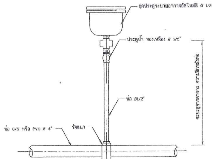
12. การติดตั้งประจุระบายอากาศอินโด ไม่แสดงมาตราส่วน
