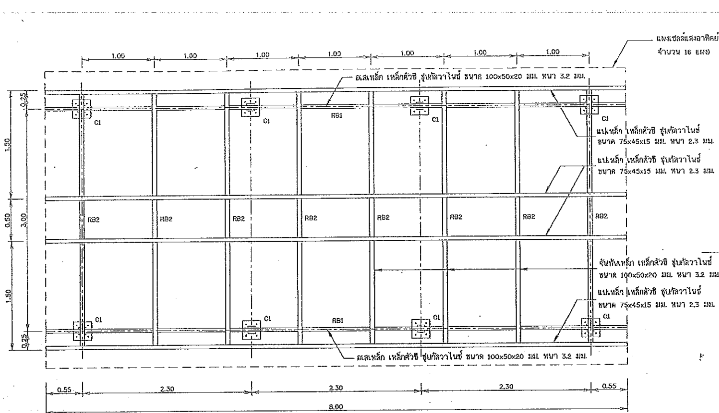
แปลนฐานจากและโครงหลังคา ไม่แสดงขนาดราตัว
