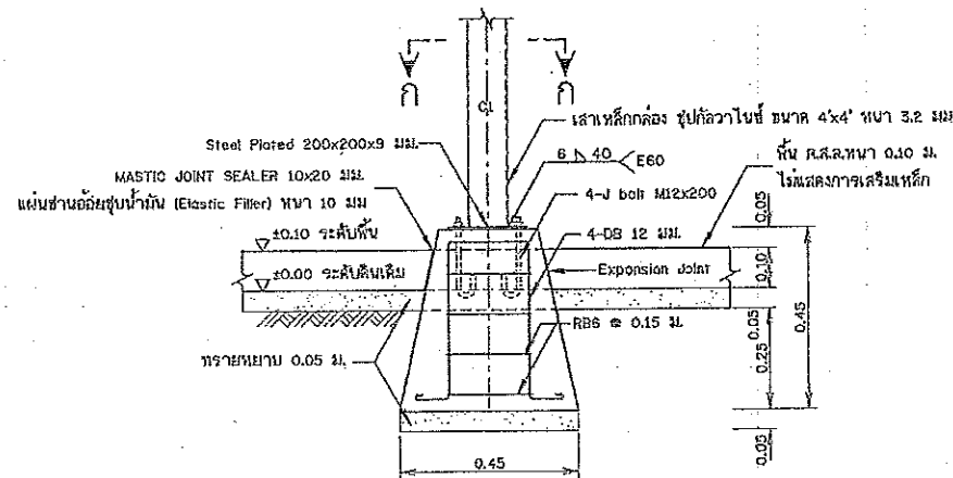
รูปขยายฐานจากโครงหลังคา F1 (ค้ำยัน ค้ำยัน หลังคาหลังคาหลังคาหลังคา) ไม่แสดงขนาดราตัว
