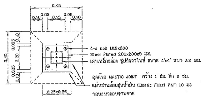
รูปตัด ก-ก ไม่แสดงขนาดราตัว
