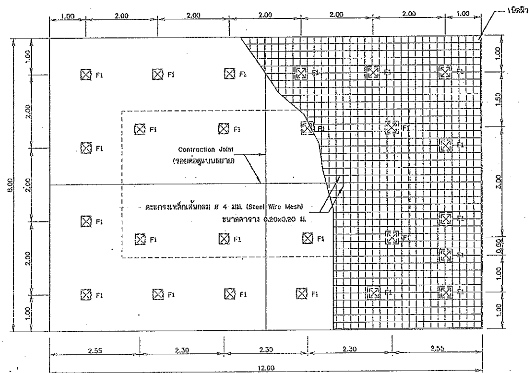
รูปขยายพื้นคอนกรีต ไม่แสดงขนาดราตัว
