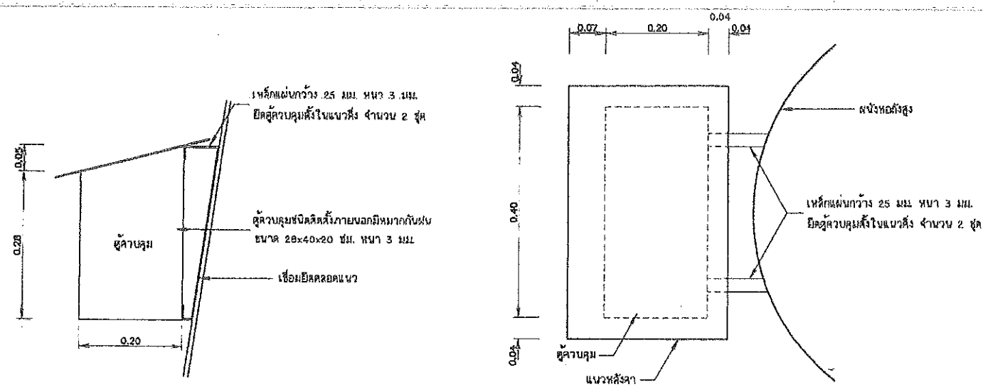
แบบขยายตัวควบคุม ไม่แสดงมาตราส่วน
