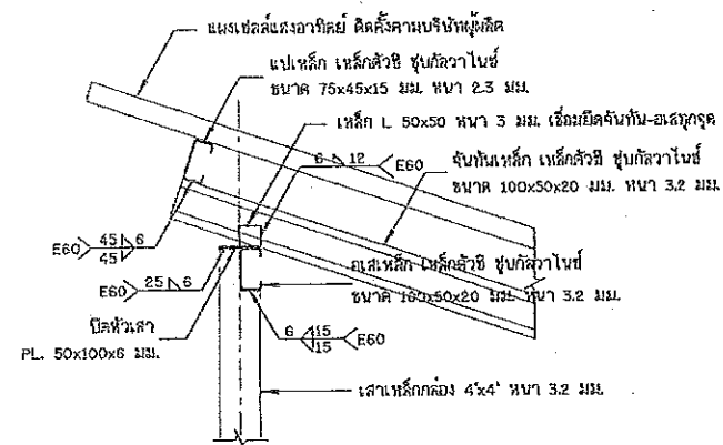
รูปขยาย การติดตั้งโครงหลังคา ไม่แสดงขนาดราตัว
