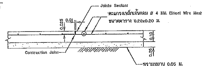
แบบขยายรอยต่อพื้น (Contraction Joint) ไม่แสดงขนาดราตัว
