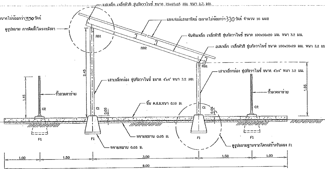
รูปด้านข้าง ไม่แสดงขนาดราตัว
