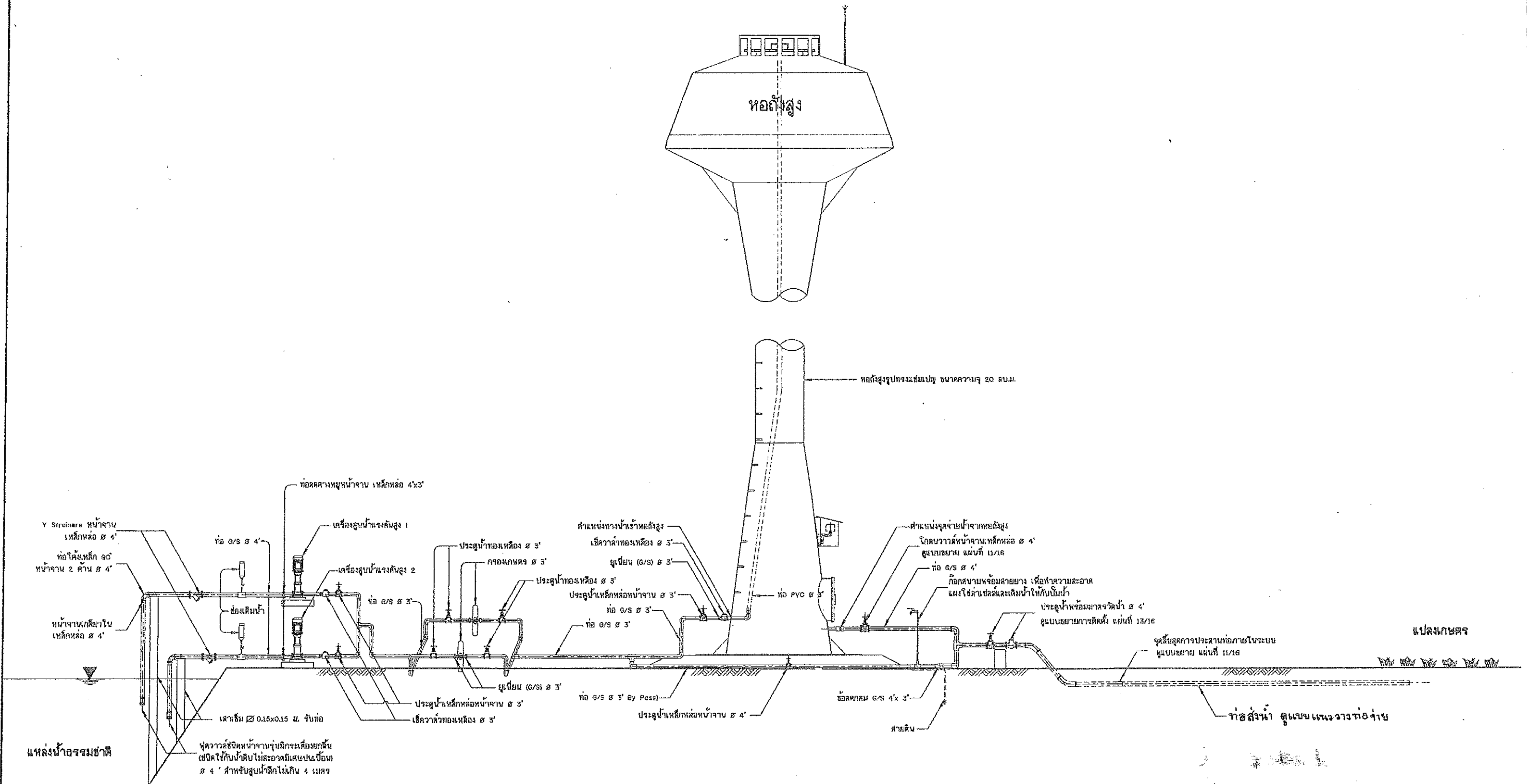
รูปแสดงรายละเอียดท่อและอุปกรณ์ระบบส่งน้ำพลังงานแสงอาทิตย์ โมเดลขนาดจริง
