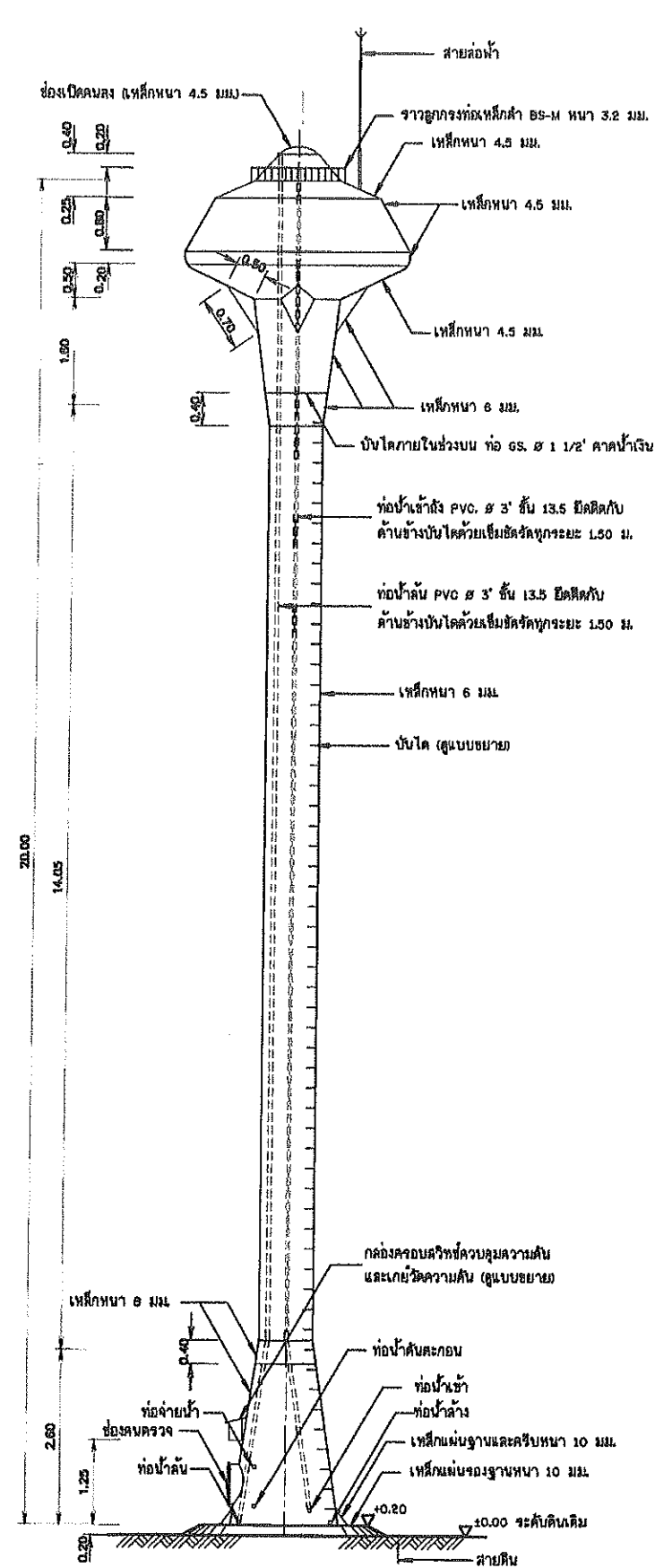
รูปด้านข้างทอดึงสูง แบบถึงเหล็กรูปทรงแฉมเปญ ไมศดงมดงส่ว
