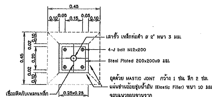
รูปตัด ข-ข ไม้ส่งมาตรวจแล้ว
