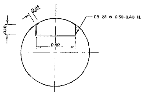
รูปขยายบันไดภายในส่วน column ไม่แสดงขนาดจริง
