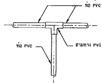
10. แบบการต่อสามทาง PVC ไม่แสดงขนาดจำนวน
