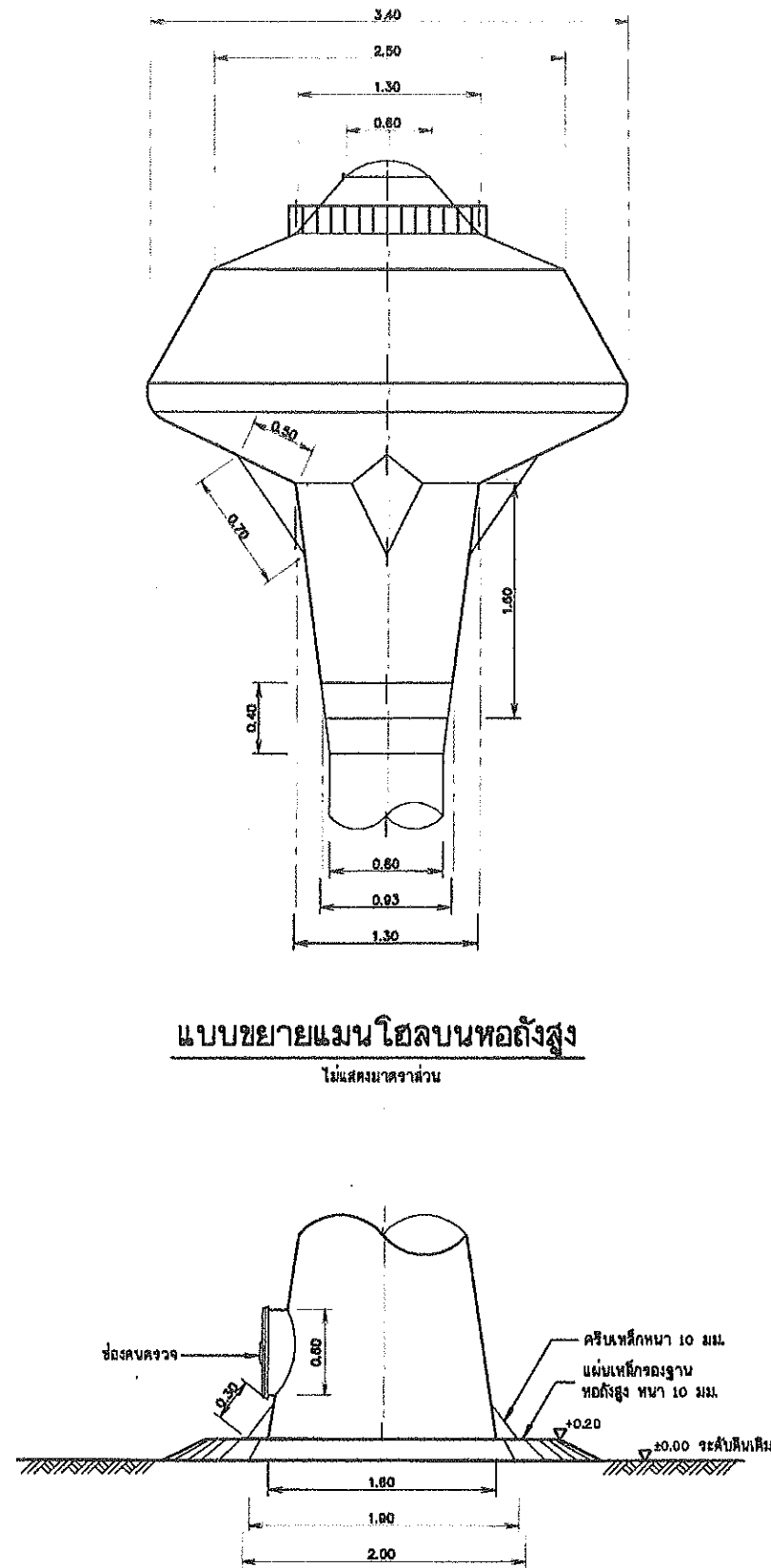
แบบขยายแมนโฮลล่างท้องถิ่นสูง ไมแสดงมาตราส่วน
