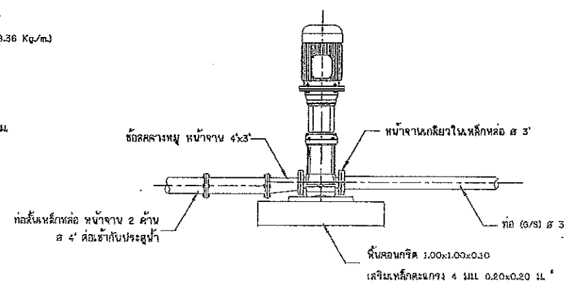
18. การต่อท่อเครื่องสูบน้ำ ไม่แสดงขนาดจำนวน
