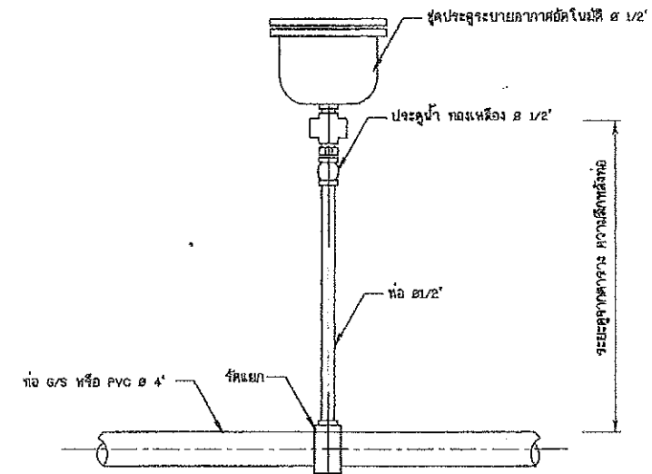
12. การติดตั้งประตูละบายอากาศอัตโนมัติ ไม่แสดงขนาดจำนวน
