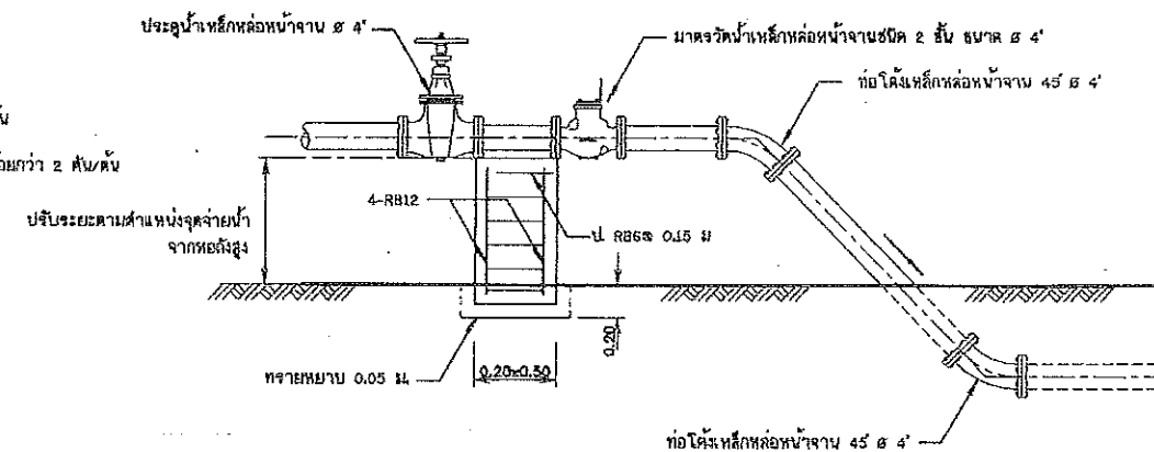
14. การติดตั้งมาตรวัดน้ำบนพื้นดิน ๕ 4' ไม่แสดงขนาดจำนวน
