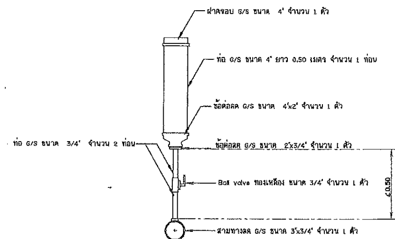
11. ช่องเติมน้ำ ไม่แสดงขนาดจำนวน
