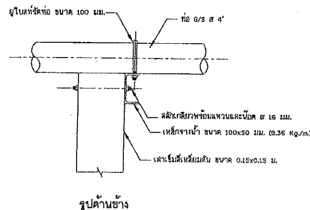
13. เสาคอมม่อนรับท่อชุด และแบบขยายอุปกรณ์รัดท่อ ไม่แสดงขนาดจำนวน
