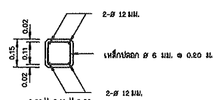
รายละเอียดการติดตั้งเสาป้าย ไม่แสดงมาตราส่วน
