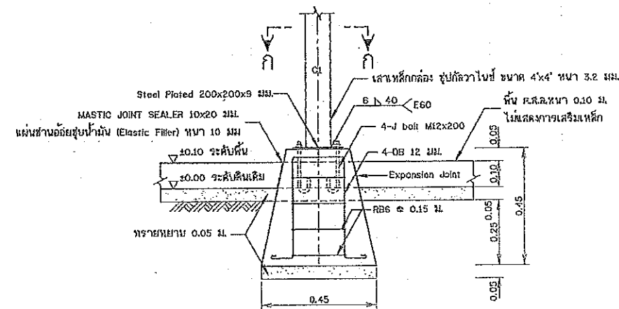
รูปขยายฐานรากโครงสร้างรับแผง F1 (คาน้ำมอ คสล. หล่อสำเร็จรูปพร้อมติดตั้ง) ไม่แสดงขนาดจั่วส่วน
