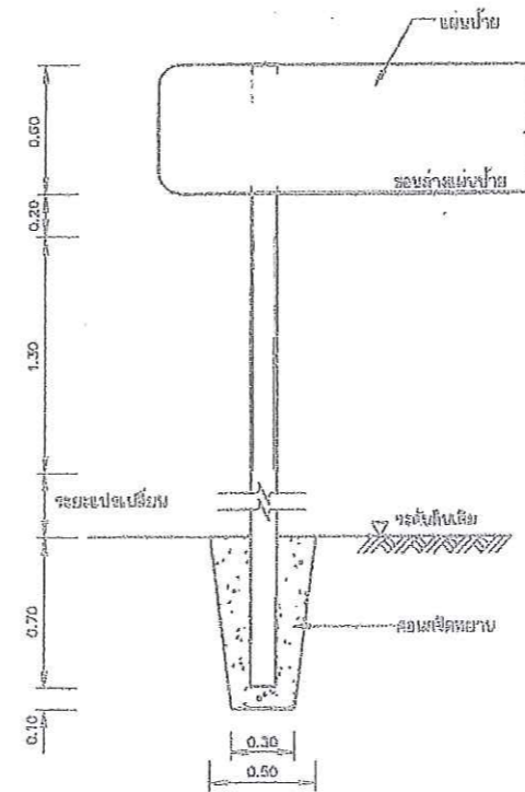
รายละเอียดการติดตั้งเสาป้าย ไม่แสดงอาคารส่วน
