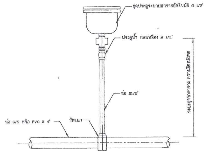
12. การติดตั้งประตูประบายอากาศอัตโนมัติ ไม่แสดงขนาดจากรายละเอียด
