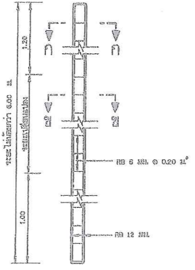
รายละเอียดเสาป้าย คสล. ไม้สนขนาดจาวสวน
