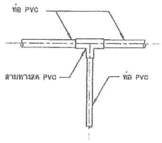
9. แบบการต่อสามทางลด PVC ไม่แสดงขนาดจากรายละเอียด
