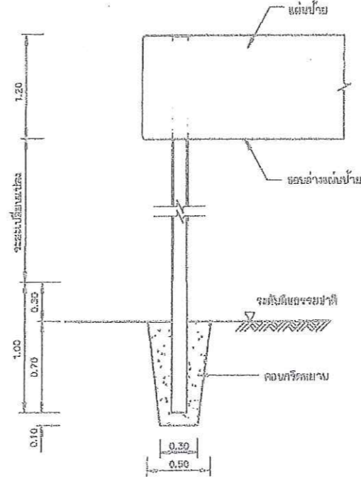
รายละเอียดการติดตั้งเสาป้าย ไม้สนขนาดจาวสวน
