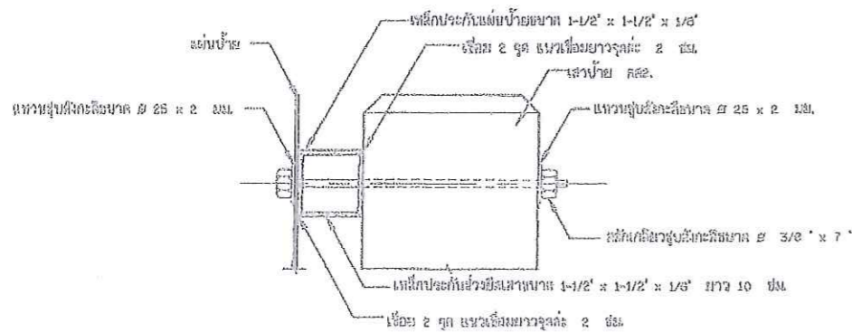
รูปตัดขยายการยึดแผ่นป้ายและเสา ไม่แสดงอาคารส่วน
