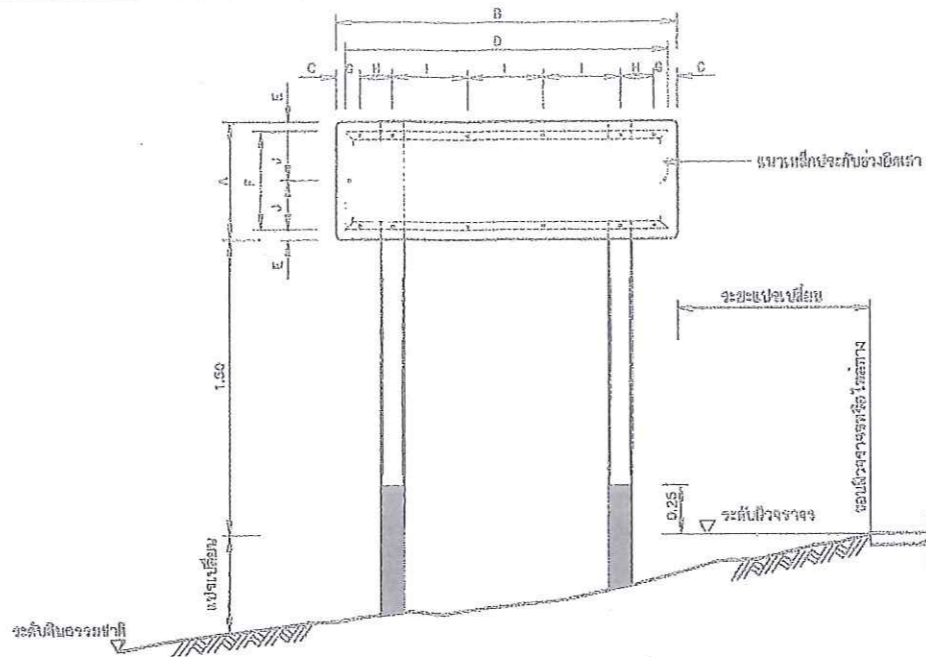
รูปแสดงการประกอบแผ่นป้าย ไม่แสดงอาคารส่วน
