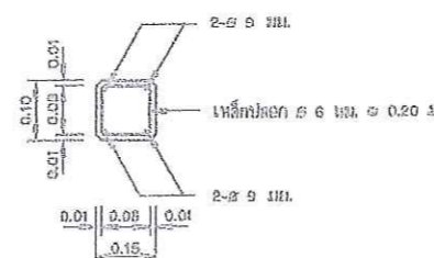
รายละเอียดการติดตั้งเสาป้าย ไม่แสดงอาคารส่วน
