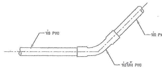
5. แบบการต่อข้อโค้ง 22 1/2, 45° PVC ไม่แสดงขนาดจาวง
