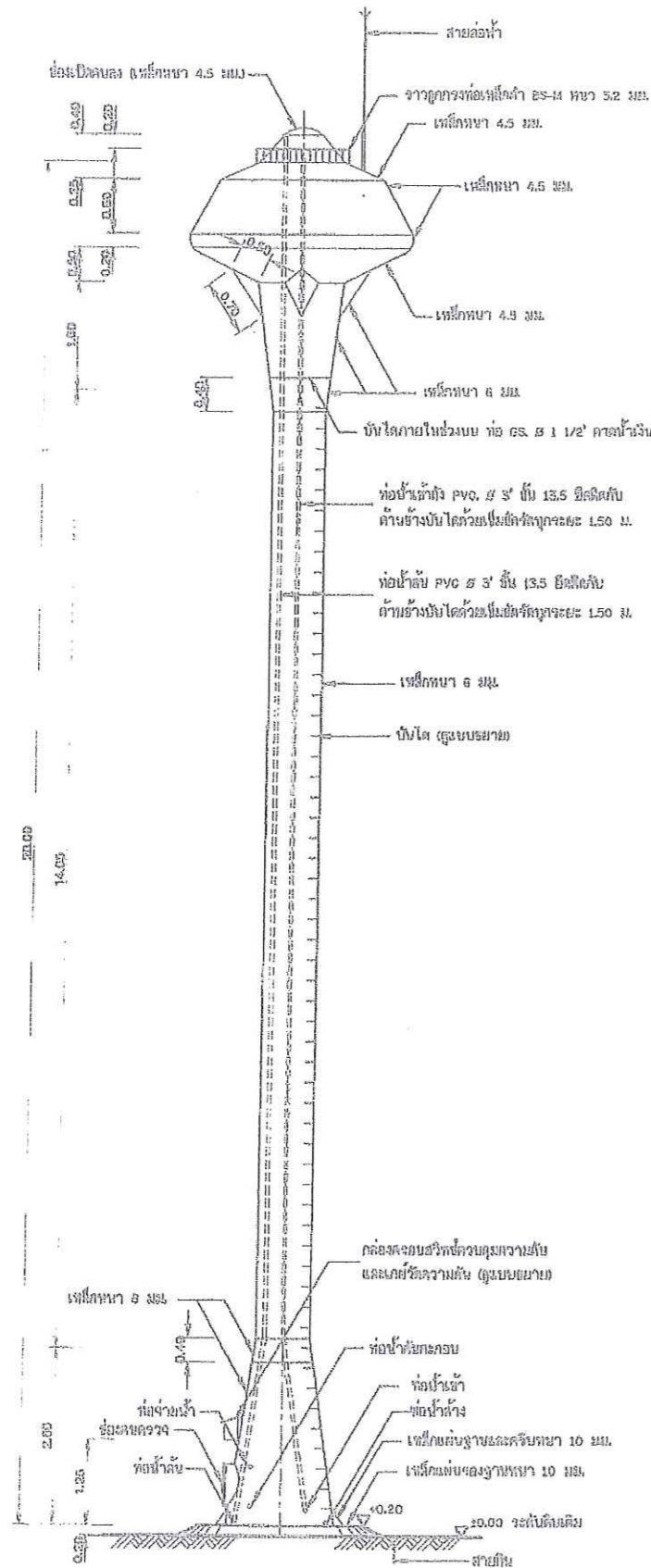
รูปตัดข้างท่อส่งสูง แบบตั้งเหล็กรูปทรงแปดเหลี่ยม ไม่แสดงมาตราส่วน
