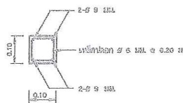
รูปตัด ก-ก ไม่แสดงอาคารส่วน
