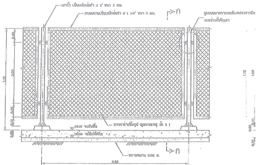
แบบขยายรั้วลดตาข่าย ไม่แสดงขนาดส่วน
