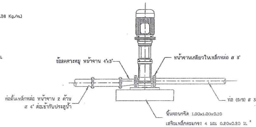
17. การต่อท่อเครื่องสูบน้ำ ไม่แสดงขนาดจากรายละเอียด
