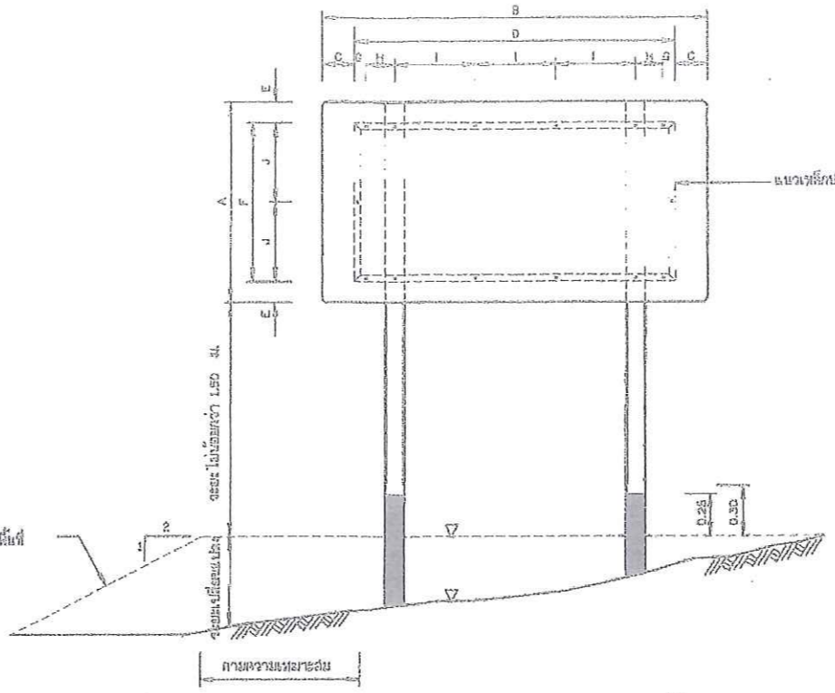
รูปแสดงการประกอบแผ่นป้าย ไม้สนขนาดจาวสวน
