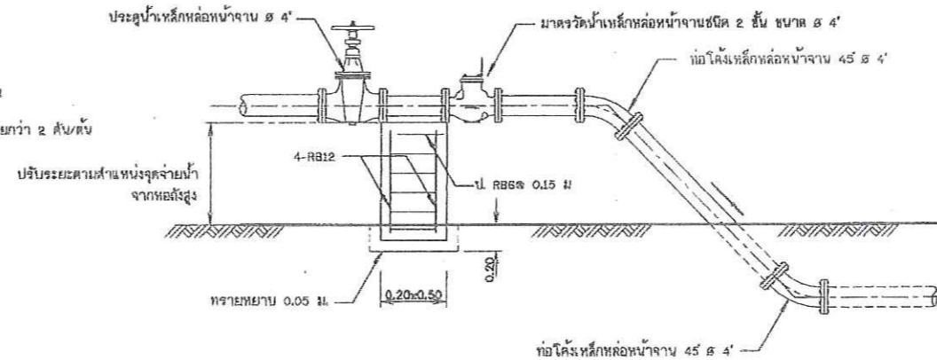
14. การติดตั้งมาตรวัดน้ำบนพื้นดิน Ø 4" ไม่แสดงขนาดจากรายละเอียด
