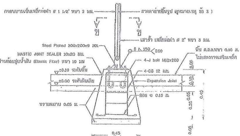
รูปขยายฐานรากโครงสร้างรับแผง F1 ตามข้อ ๗.๕. มอดูลสำเร็จรูปพร้อมติดตั้ง ไม่แสดงขนาดส่วน
