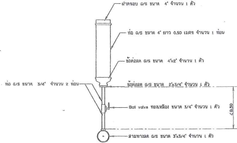
11. ช่องเติมน้ำ ไม่แสดงขนาดจากรายละเอียด
