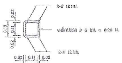
รูปตัด ข-ข ไม้สนขนาดจาวสวน
