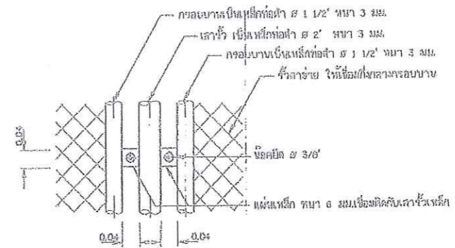
แบบขยายรายละเอียดแสดงการยึดระหว่างรั้วกับเสา ไม่แสดงขนาดส่วน
