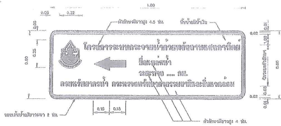
ป้ายแนะนำโครงการ ไม่แสดงอาคารส่วน
