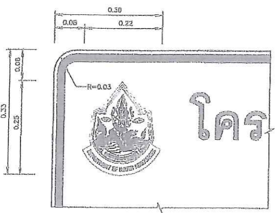
ป้ายโครงการ ไม้สนขนาดจาวสวน
