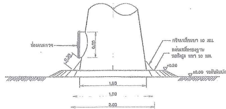
แบบขยายแมนโฮลล่างท่อส่งสูง ไม่แสดงมาตราส่วน
