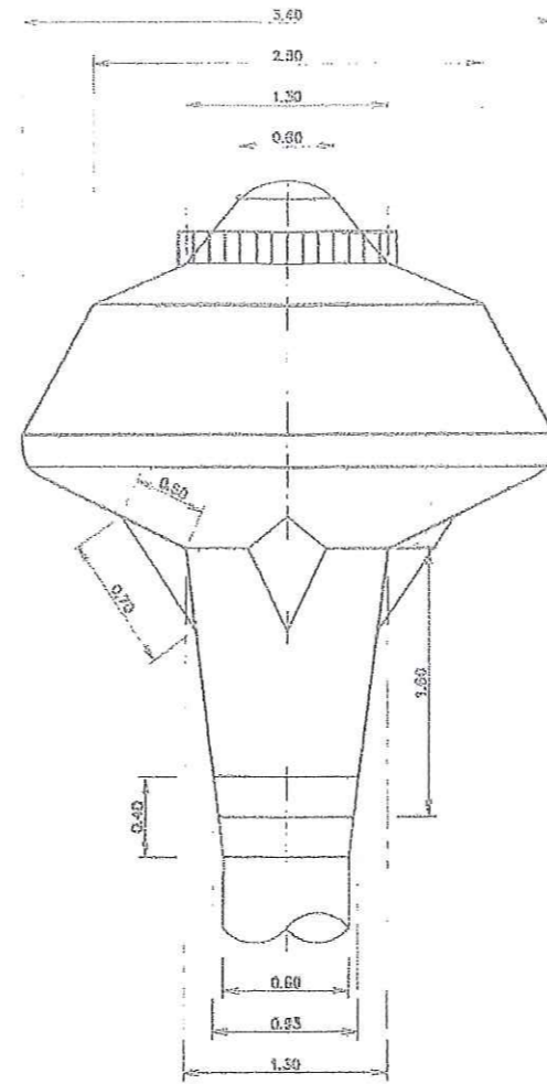
แบบขยายแมนโฮลบนท่อส่งสูง ไม่แสดงมาตราส่วน
