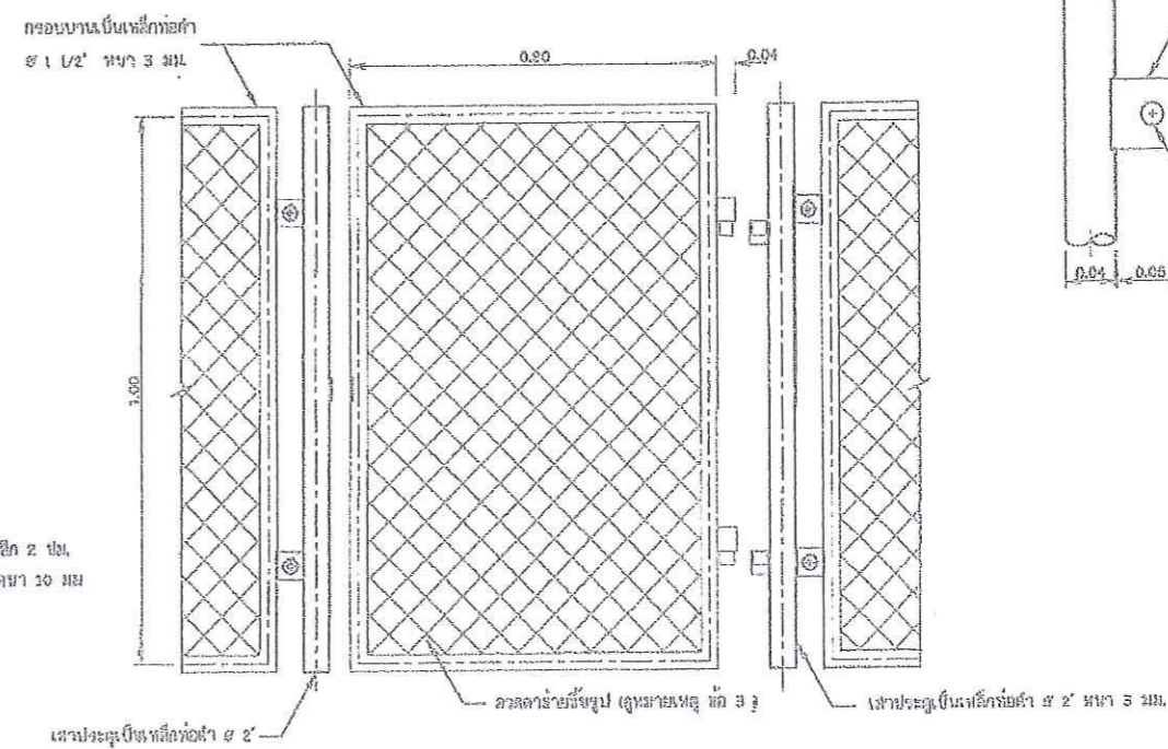
แบบขยายสายลึง ไม่แสดงขนาดส่วน
