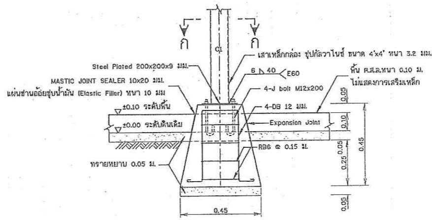
รูปขยายฐานรากโครงสร้างรับแผง F1 (กรณี คสล. ท่อส่งน้ำหรือท่อประปาฝัง) ไม่แสดงขนาดจั่วส่วน
