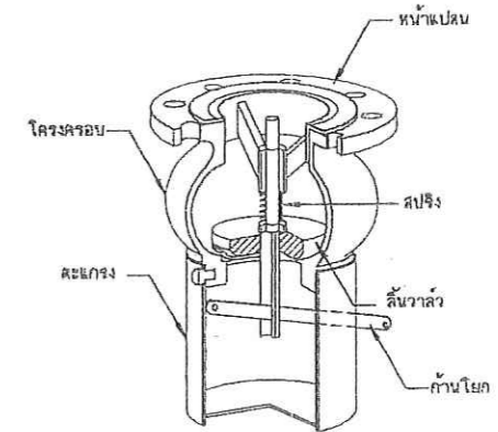
15. ชุดวาล์ว แบบก้านโยก ไม่แสดงขนาดจากรายละเอียด
