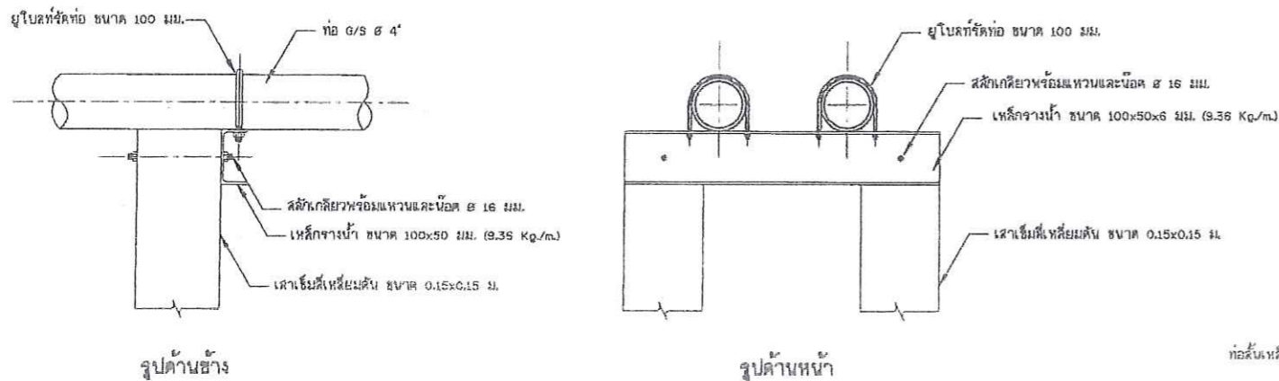
13. เสาคอดม่อรับท่อลอด และแบบขยายอุปกรณ์รัดท่อ ไม่แสดงขนาดจากรายละเอียด
