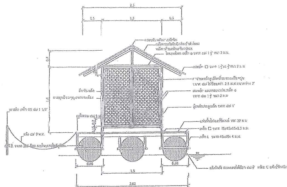
รูปด้านหน้า 1:25
