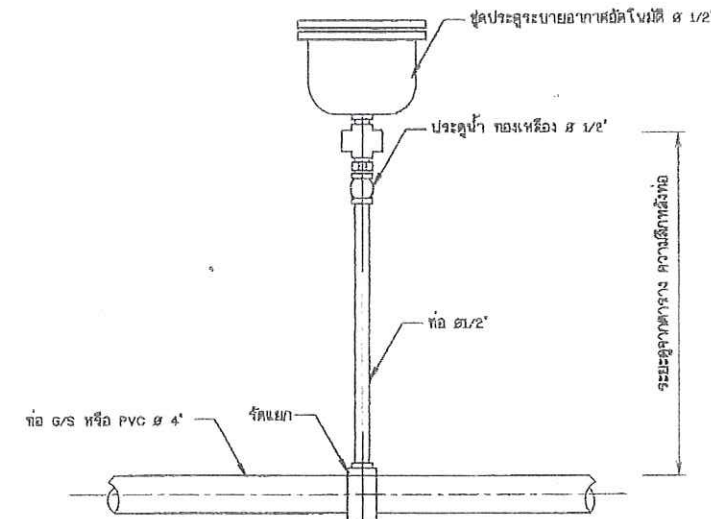
12. การติดตั้งประตูละบายอากาศอัด โนมิติ ไม่แสดงขนาดบางส่วน
