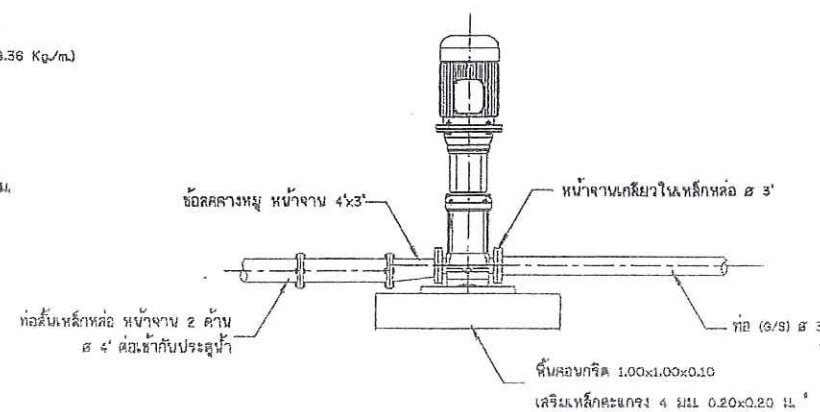
18. การต่อท่อเครื่องสูบน้ำ ไม่แสดงขนาดบางส่วน
