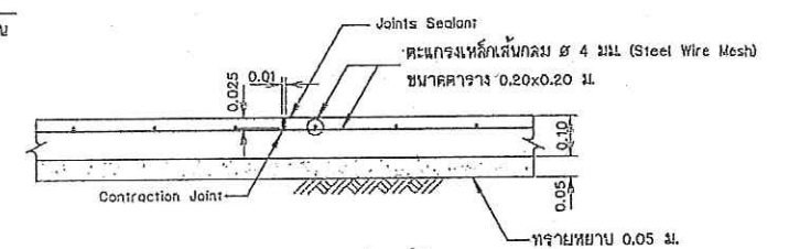
แบบขยายรอยต่อพื้ (Contraction Joint) ไม่แสดงมาตราส่วน
