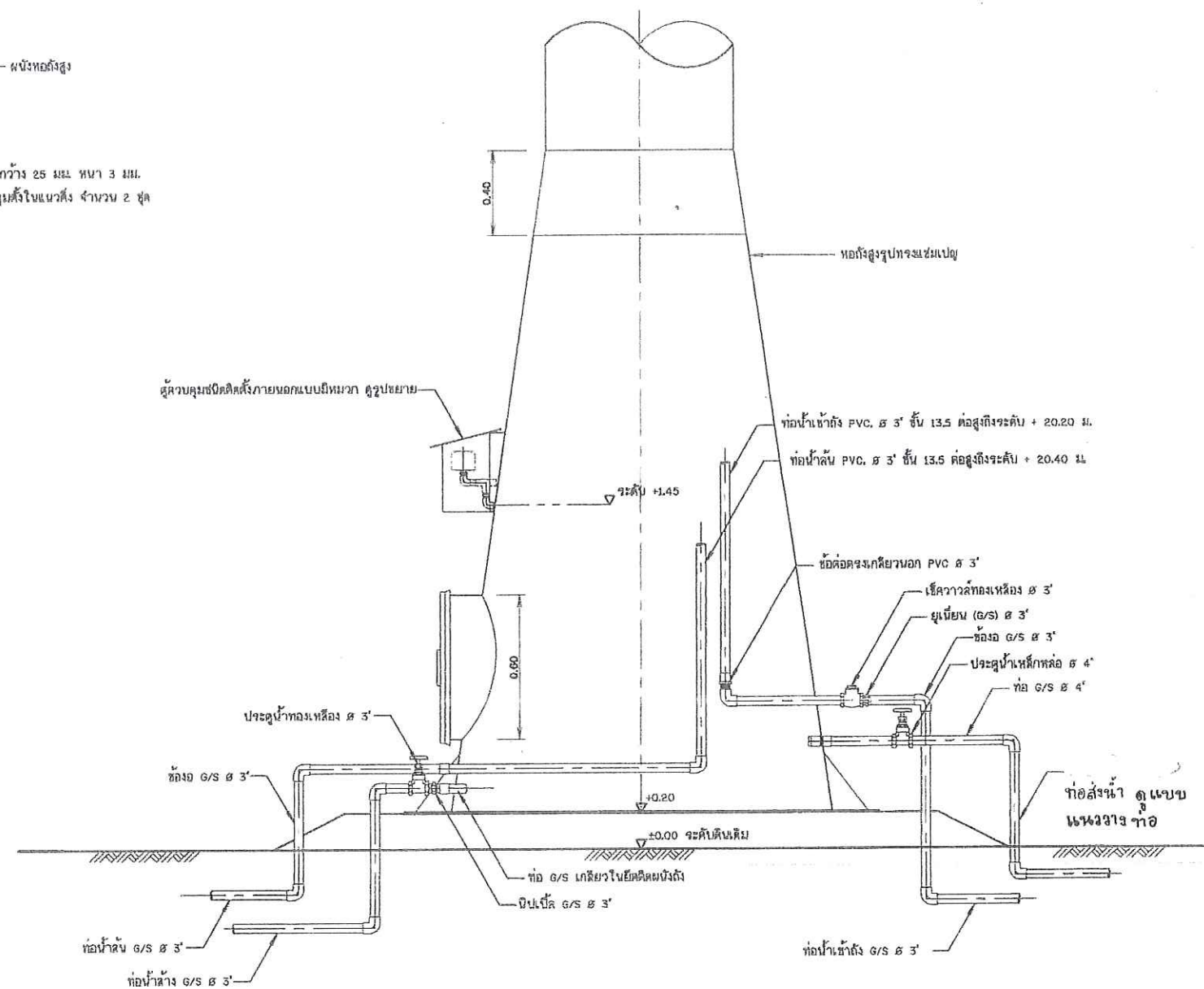
แบบแสดงการเดินท่อในท่อถึงสูง
