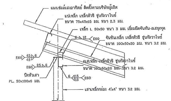
รูปขยาย การติดตั้งโครงหลังคา ไม่แสดงมาดราส่วน
