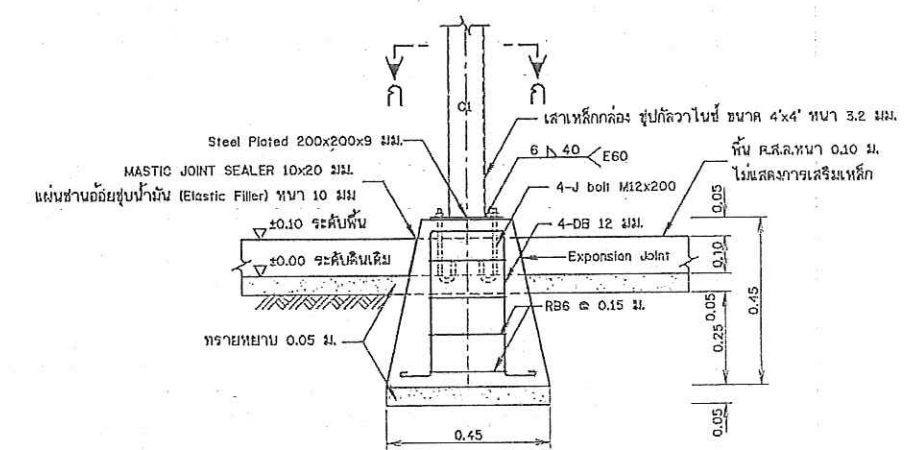
รูปขยายจากโครงสร้างรับแรง F1 (คณณ ศสส. หล่อสำรูปพร้อมเค็ดคัง) ไม่แสดงมาตราส่วน
