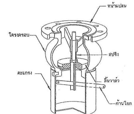
15. ฟุตวาล์ว แบบก้านโยก ไม่แสดงขนาดบางส่วน
