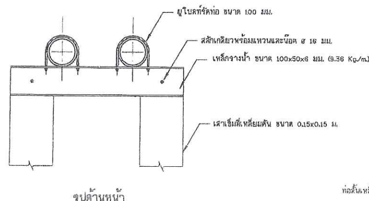
13. เสาคอมม่อนรับท่อชุด และแบบขยายอุปกรณ์รัดท่อ ไม่แสดงขนาดบางส่วน
