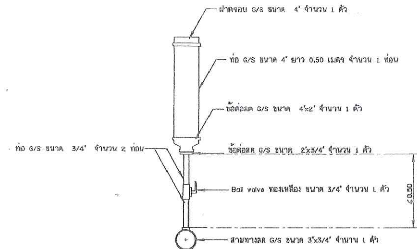
11. ช่องเติมน้ำ ไม่แสดงขนาดบางส่วน
