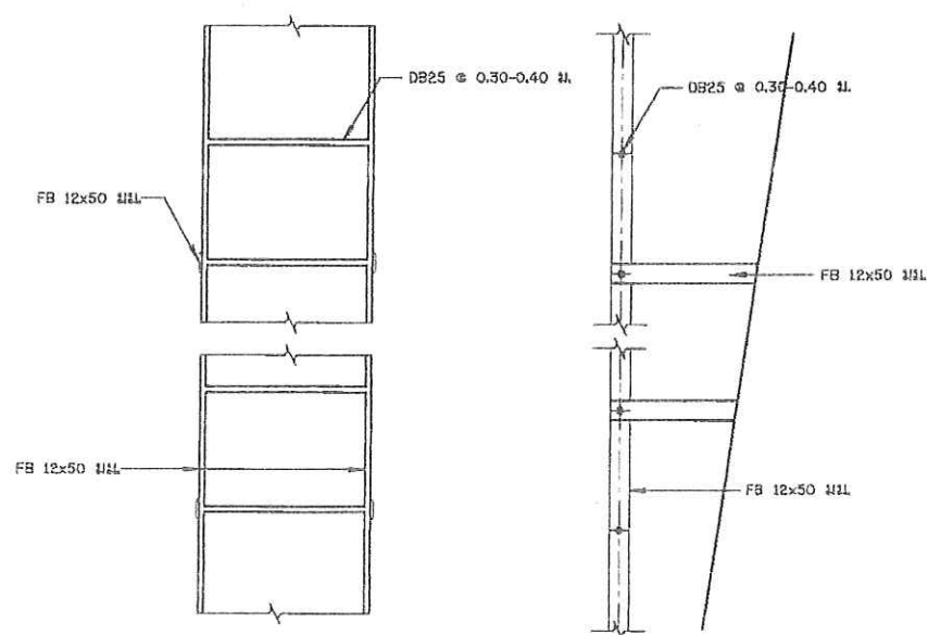
แบบขยายบันได ภายในท่อถึงสูง
