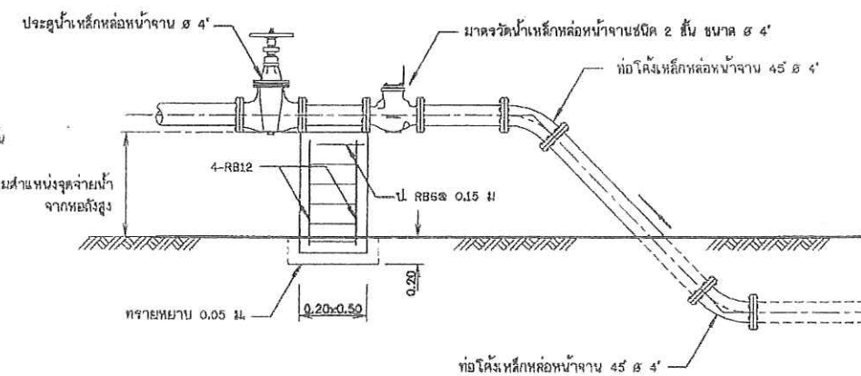
14. การติดตั้งมาตรวัดน้ำบนพื้นดิน Ø 4" ไม่แสดงขนาดบางส่วน
