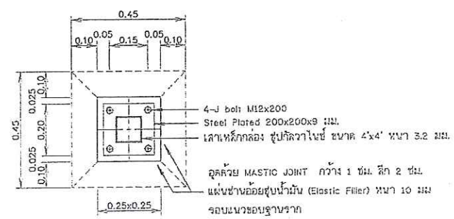
รูปตัด ก-ก ไม่แสดงขนาดจริง
