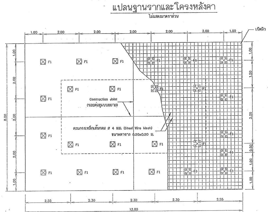
รูปขยายพื้นคอนกรีต ไม่แสดงขนาดจั่วบน
