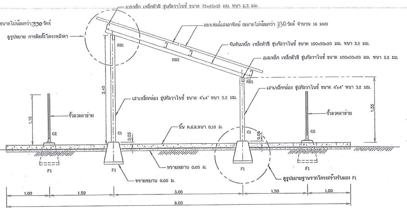
รูปด้านข้าง ไม่แสดงมาตราส่วน
