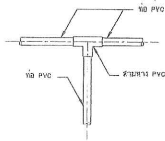
10. แบบการต่อสามทาง PVC ไม่แสดงขนาดบางส่วน
