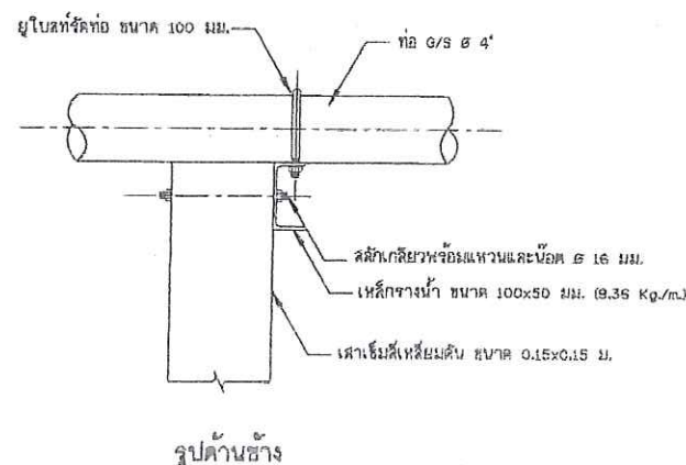
13. เสาคอมม่อนรับท่อชุด และแบบขยายอุปกรณ์รัดท่อ ไม่แสดงขนาดบางส่วน
