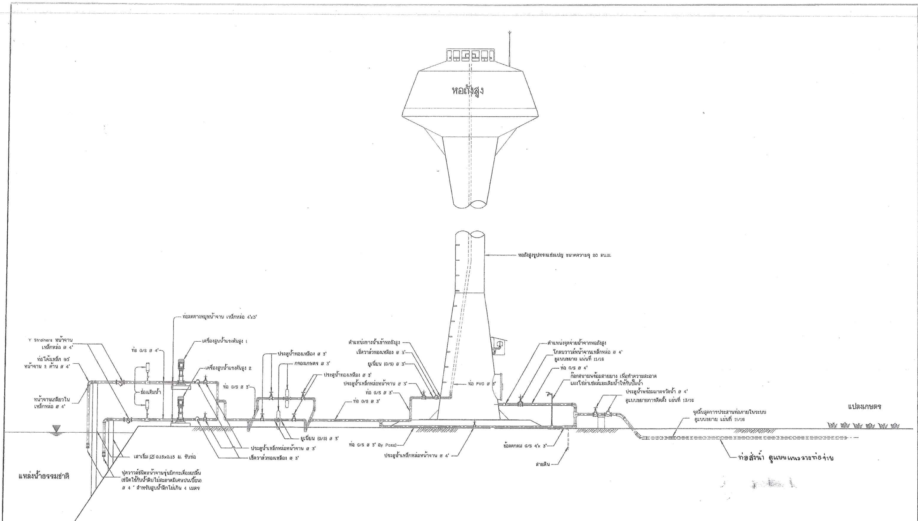
รูปแสดงรายละเอียดท่อและอุปกรณ์ระบบส่งน้ำพลังงานแสงอาทิตย์ ไม่แสดงมาตราส่วน
