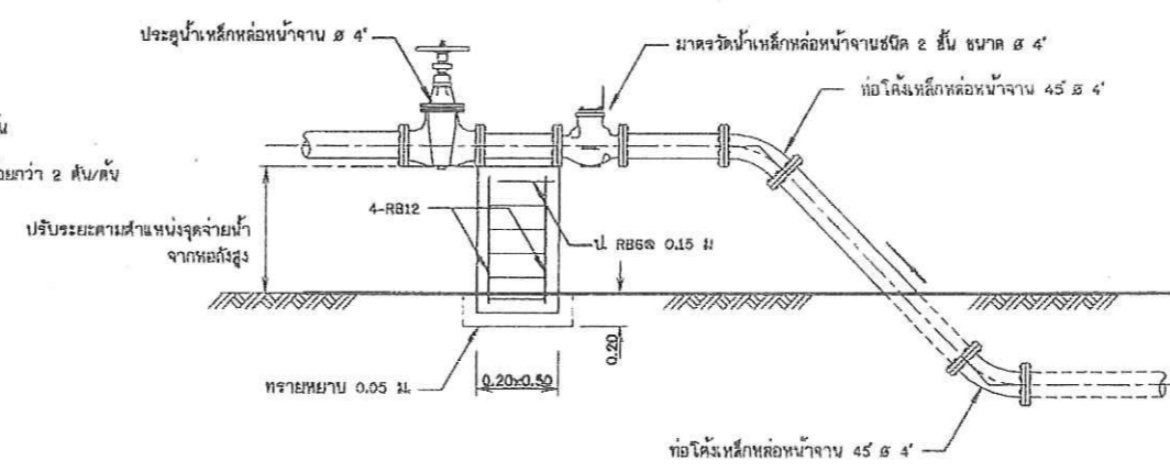
14. การติดตั้งมาตรวัดน้ำบนพื้นดิน ๕ 4" ไม่แสดงมาตราส่วน
