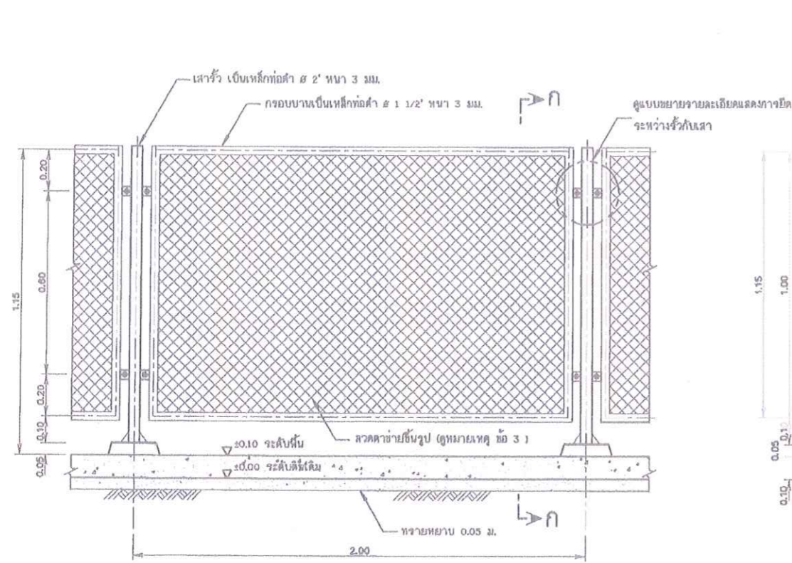
แบบขยายรั้วลวดตาข่าย ไม่แสดงมาตราส่วน
