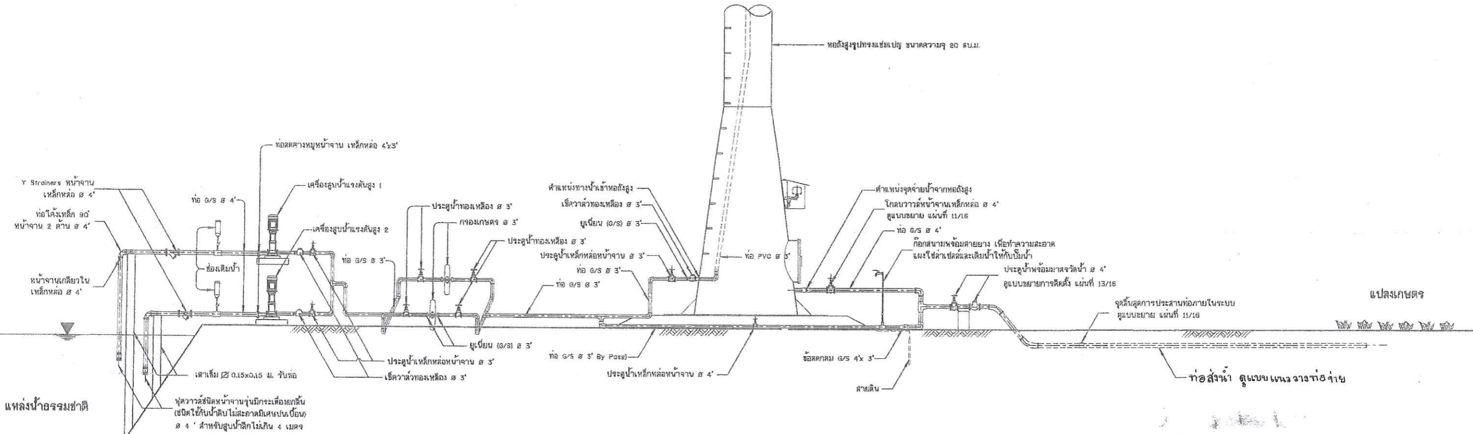
รูปแสดงรายละเอียดท่อและอุปกรณ์ระบบส่งน้ำพลังงานแสงอาทิตย์
