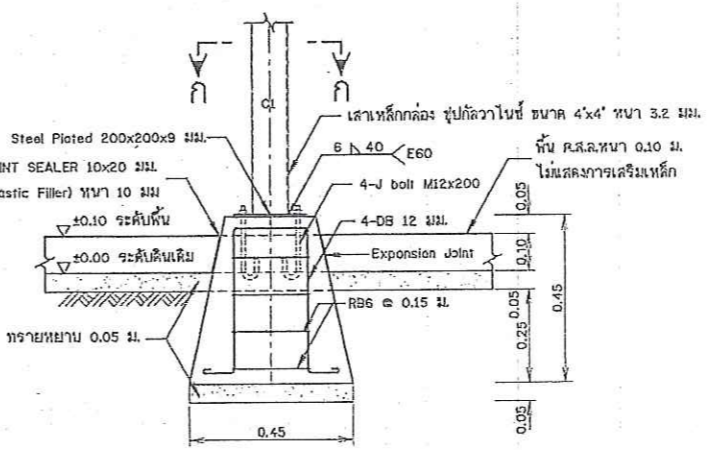
รูปขยายฐานรากโครงสร้างรับแผง F1 (คอดม คสล. หลอดน้ำรูปทรงกลมติดตั้ง) ไม่แสดงขนาดจั่วส่วน
