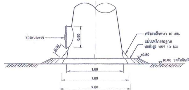
แบบขยายแมนไฮลล่างท่อน้ำสูง ไม่แสดงมาตราส่วน
