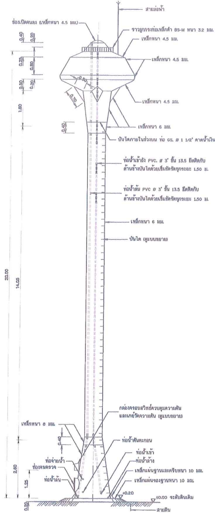
รูปดำนข้างท่อน้ำสูง แบบถึงเหล็กรูปทรงแปมเปญ ไม่แสดงมาตราส่วน
