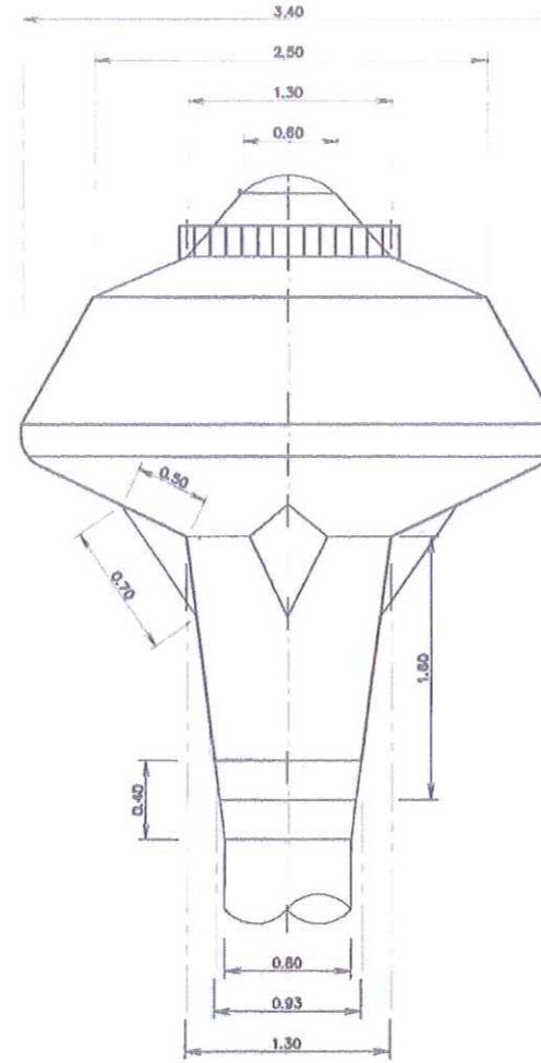
แบบขยายแมนไฮลบนท่อน้ำสูง ไม่แสดงมาตราส่วน
