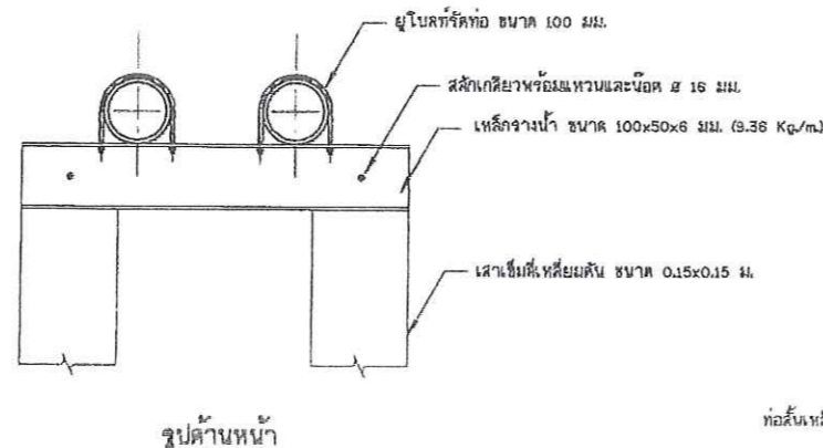
13. เสาคอมม่อรับท่อจุด และแบบขยายอุปกรณ์รีดท่อ ไม่แสดงมาตราส่วน
