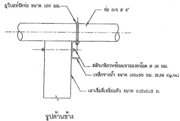
13. เสาคอมม่อรับท่อจุด และแบบขยายอุปกรณ์รีดท่อ ไม่แสดงมาตราส่วน
