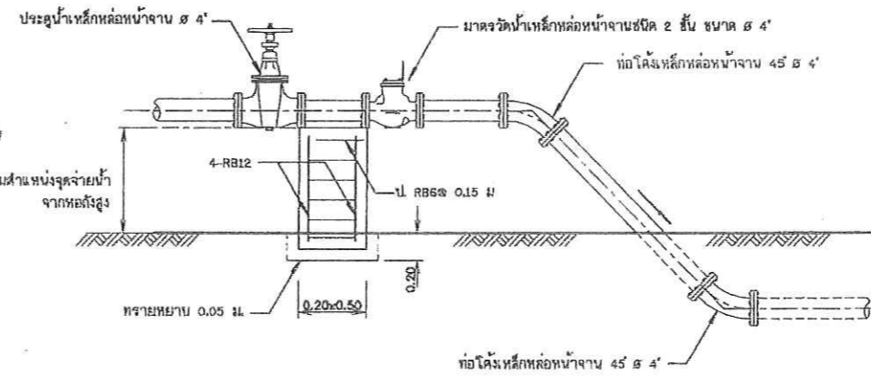
14. การติดตั้งมาตรวัดน้ำบนพื้นดิน ๕ 4" ไม่แสดงมาตราส่วน
