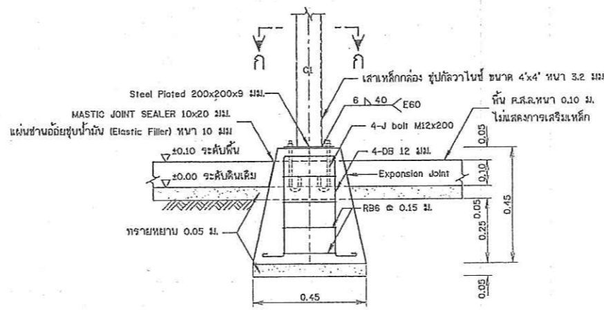
รูปขยายฐานรากโครงสร้างรับแผง F1 (ต่อหน้า คสล. หลังค้ำรับพร้อมติดตั้ง) ไม่แสดงขนาดจั่ว
