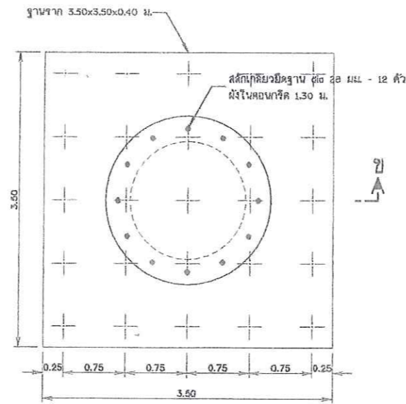
แปลน ฐานรากหล่อถึงสูง (แบบเสาเข็ม)
