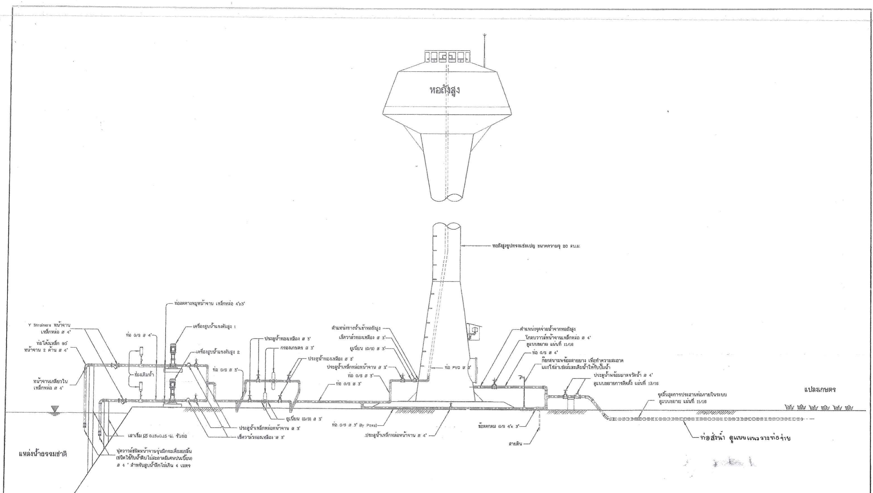
รูปแสดงรายละเอียดท่อและอุปกรณ์ระบบสูบน้ำพลังงานแสงอาทิตย์ ไม่แสดงมาตราส่วน
