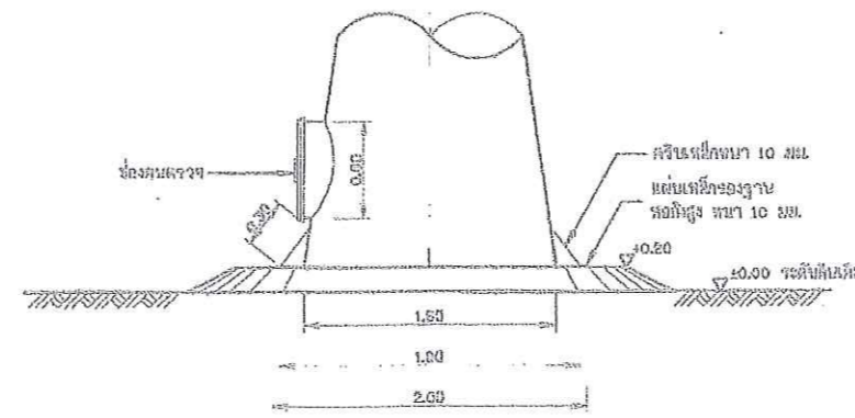
แบบขยายแผนสี่เหลี่ยมท่อตั้งสูง ไม้แสดงขนาดกลาง
