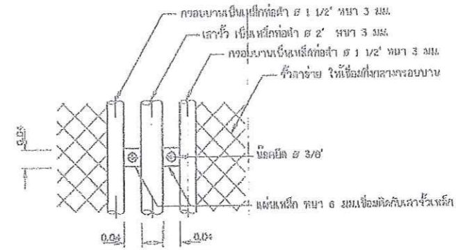
แบบขยายรายละเอียดแสดงการยึดระหว่างหัวกับเสา ไม่แสดงขนาดส่วน
