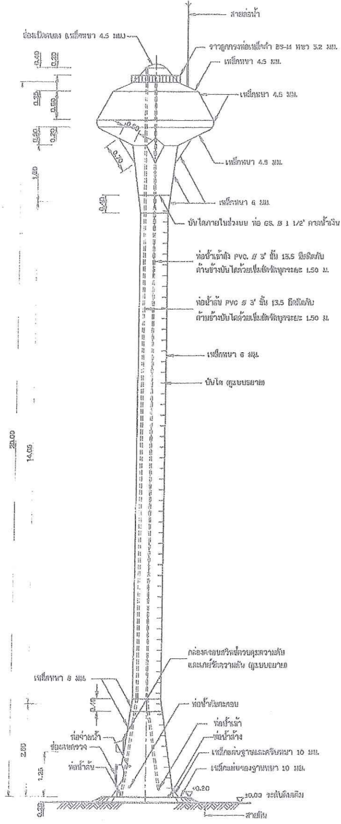
รูปด้านข้างท่อตั้งสูง แบบตั้งเหล็กรูปทรงแปดเหลี่ยม ไม้แสดงขนาดกลาง
