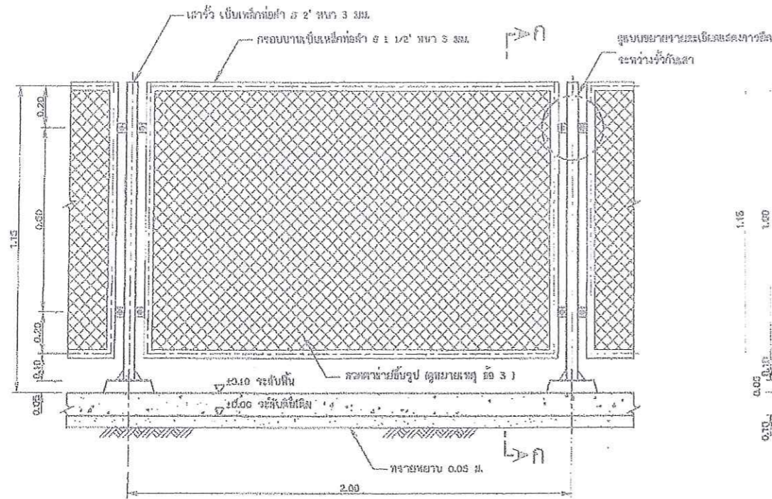
แบบขยายหัวลวดตาข่าย ไม่แสดงขนาดส่วน
