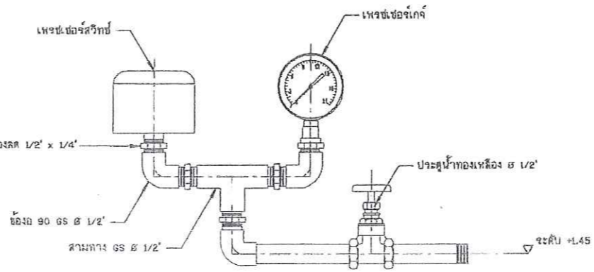
แบบขยายสวิตช์ควบคุมและเกจวัดความดัน ไม่แสดงมาตราส่วน
