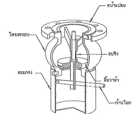
15. การต่อท่อเครื่องสูบน้ำ ไม่แสดงขนาดส่วน
