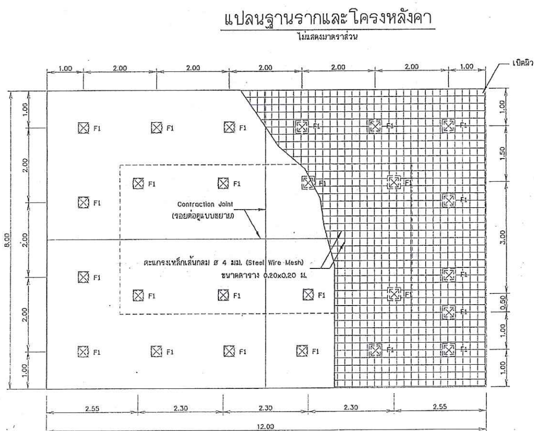
รูปขยายพื้นคอนกรีต ไม่แสดงขนาดจั่ว
