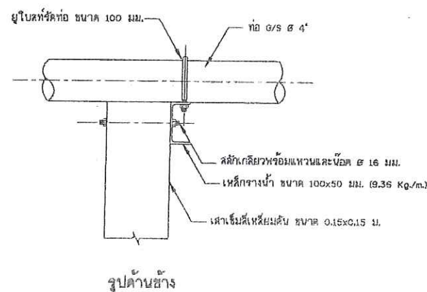
13. เสาคอมม่อนรับท่อชุด และแบบขยายอุปกรณ์รัดท่อ ไม่แสดงขนาดส่วน
