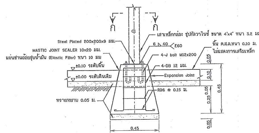
รูปขยายฐานรากโครงสร้างรับแผง F1 (คอนกรีต, เหล็กเสริม) ไม่แสดงขนาดจั่ว
