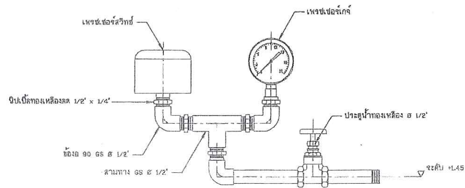
แบบขยายสวิตช์ควบคุมและแก้วัดความดัน ไม่แสดงขนาดส่วน
