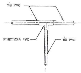
9. แบบการต่อสามทางลด PVC ไม่แสดงขนาดส่วน
