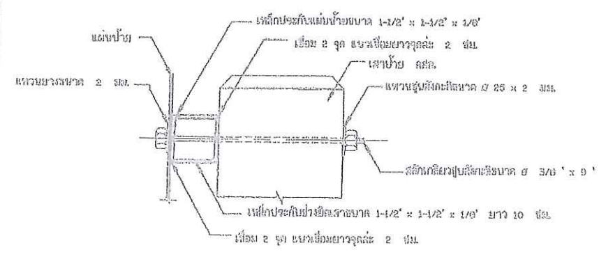
รูปตัดขยายการยึดแผ่นป้ายและเสา ไม่แสดงขนาดส่วน
