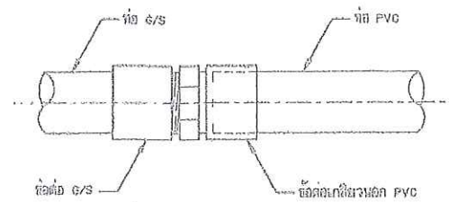
2. แบบการต่อท่อ G/S กับท่อ PVC ไม่แสดงขนาดส่วน
