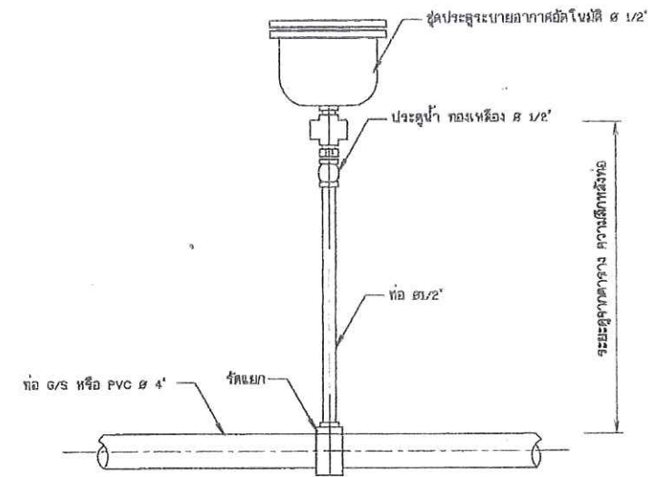
12. การติดตั้งประตูละบายอากาศอัด โนมิตี ไม่แสดงขนาดส่วน
