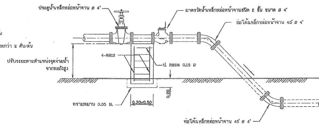
14. การติดตั้งมาตรวัดน้ำบนพื้นดิน ๔ ๔" ไม่แสดงขนาดส่วน
