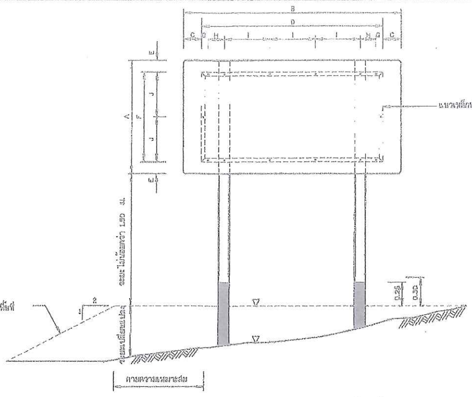
รูปแสดงการประกอบแผ่นป้าย ไม่แสดงขนาดส่วน
