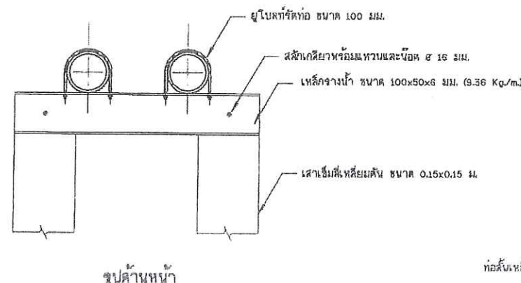
13. เสาคอมม่อนรับท่อชุด และแบบขยายอุปกรณ์รัดท่อ ไม่แสดงขนาดส่วน
