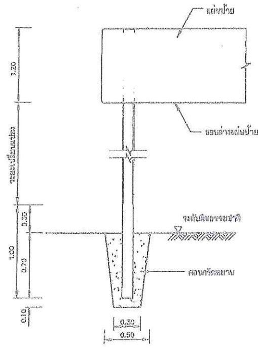
รายละเอียดการติดตั้งเสาป้าย ไม่แสดงขนาดส่วน
