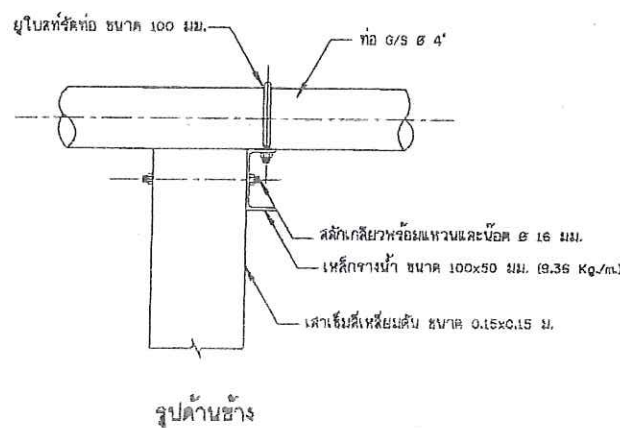
13. เสาคอมมิวติเตอร์ และแบบขยายอุปกรณ์วัดท่อ ไม่แสดงมาตราส่วน
