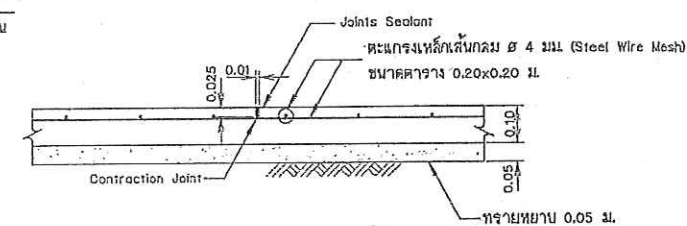
แบบขยายรอยต่อพื้น (Contraction Joint) ไม่แสดงขนาดจั่วส่วน
