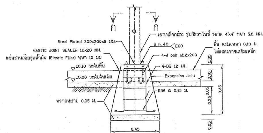
รูปขยายฐานรากโครงสร้างรับแผง F1 (ต่อม่อ คลสิ หล่อสำเร็จรูปหรือติดตั้ง) ไม่แสดงขนาดจั่วส่วน
