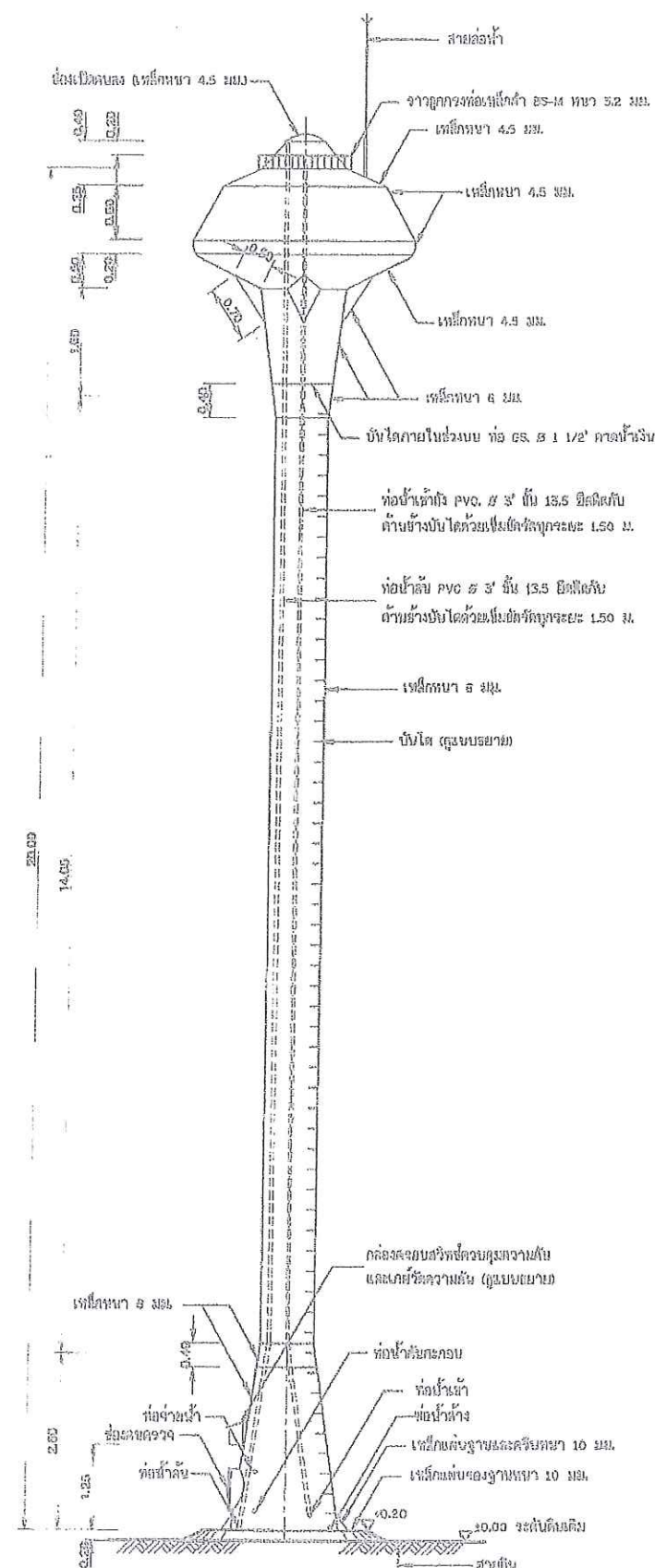
รูปด้านข้างพลัดสูง แบบตั้งเหล็กรูปทรงระฆังแปดเหลี่ยม
