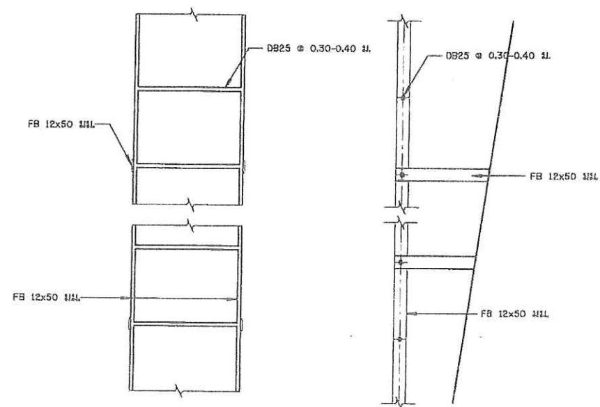
แบบขยายบันได ภายในหอถังสูง
