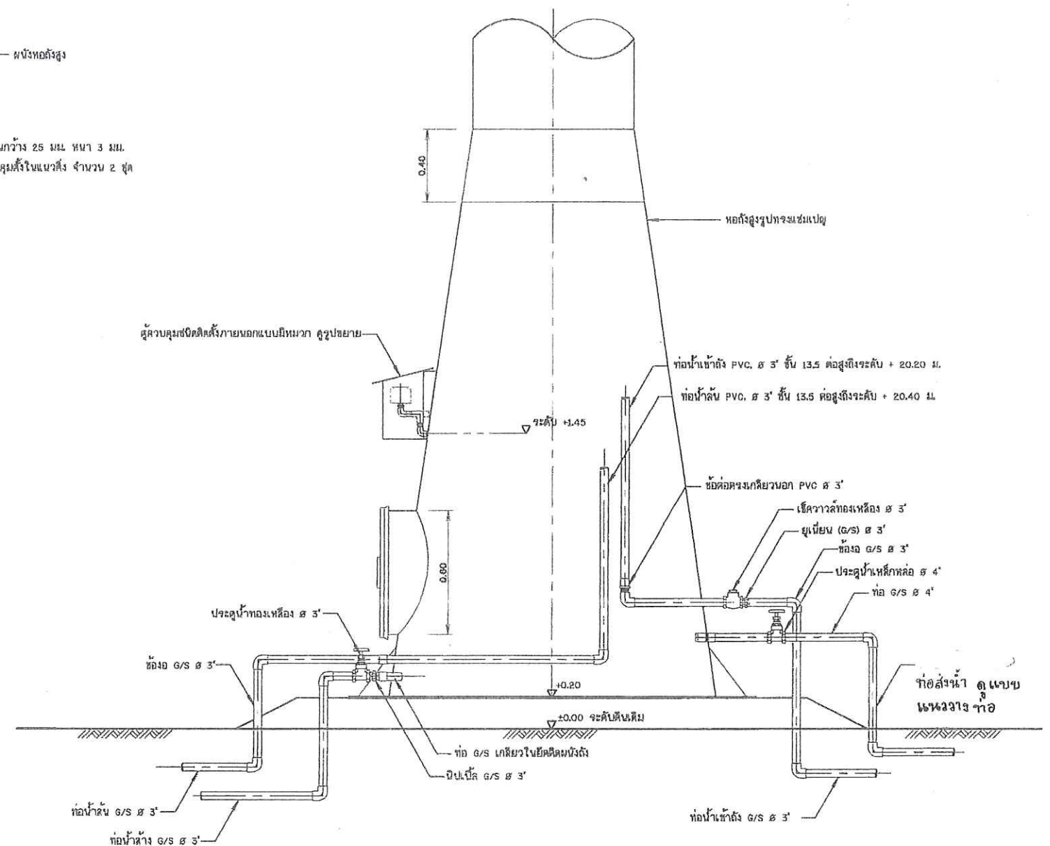
แบบแสดงการเดินท่อในหอถังสูง
