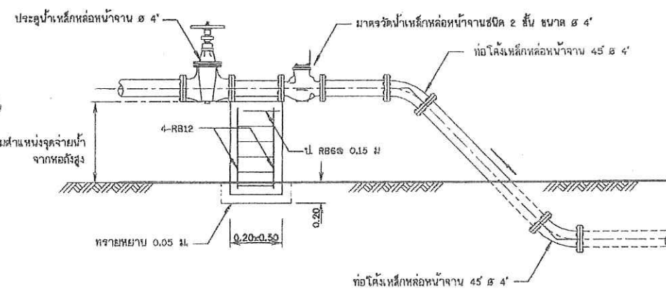
14. การติดตั้งมาตรวัดน้ำบนพื้นดิน Ø 4" ไม่แสดงมาตราส่วน
