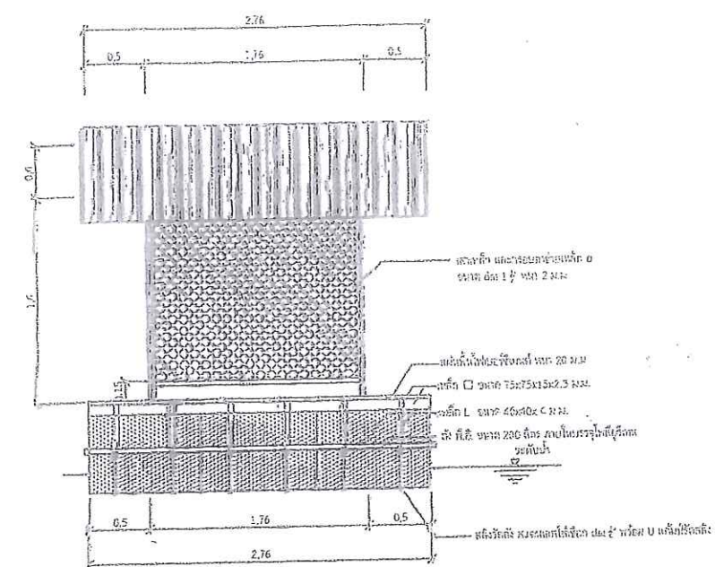
รูปด้านข้าง 1:25
