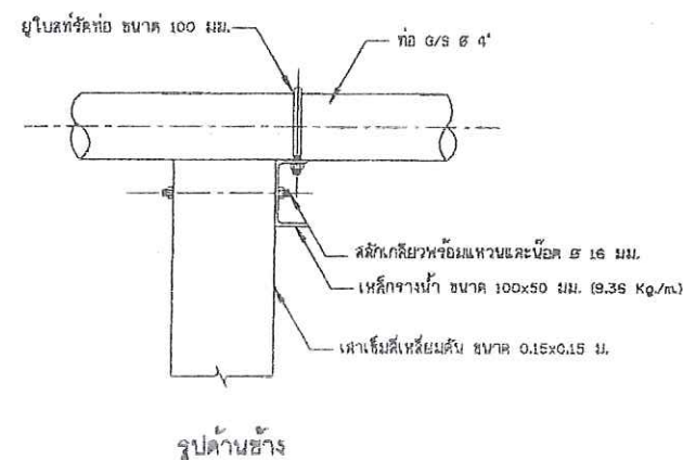
13. เสาดอม่อรับท่อชุด และแบบขยายอุปกรณ์รัดท่อ ไม่แสดงมาตราส่วน
