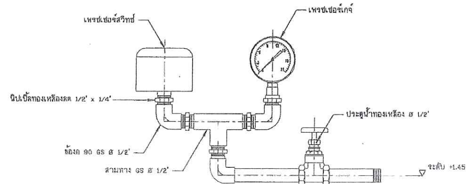
แบบขยายสวิตช์ควบคุมและเกจวัดความดัน
