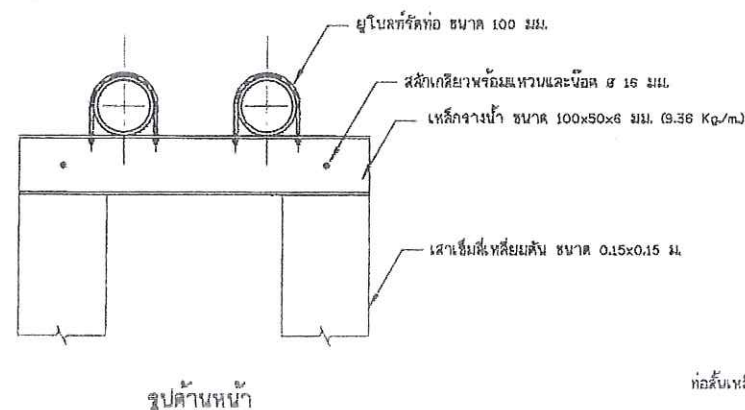
13. เสาดอม่อรับท่อชุด และแบบขยายอุปกรณ์รัดท่อ ไม่แสดงมาตราส่วน
