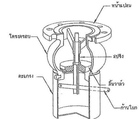
16. ฟุตวาล์ว แบบก้านโยก ไม่แสดงมาตราส่วน
