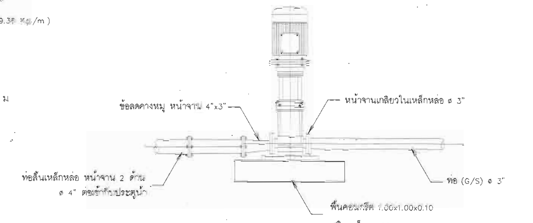
15. การต่อท่อเครื่องสูบน้ำ ไม่แสดงมาตราส่วน
