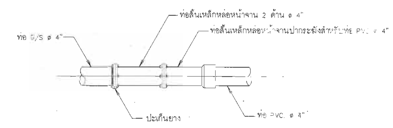
8. การบรรจบท่อเหล็กอาบสังกะสี G/S กับท่อ PVC. ไม่แสดงมาตราส่วน
