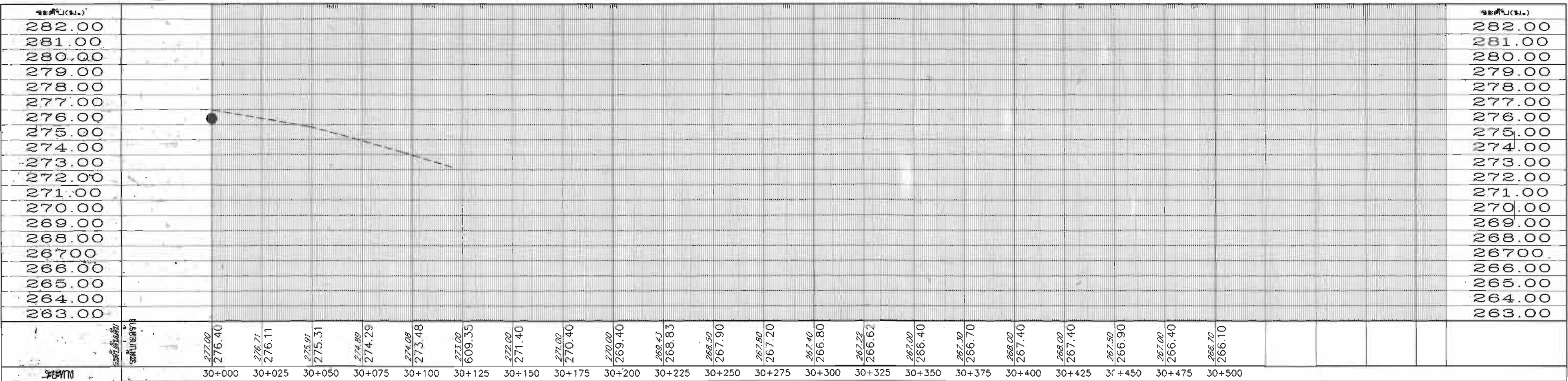
รูปตัดตามยาวแนววงทอ สาย MPR R1
