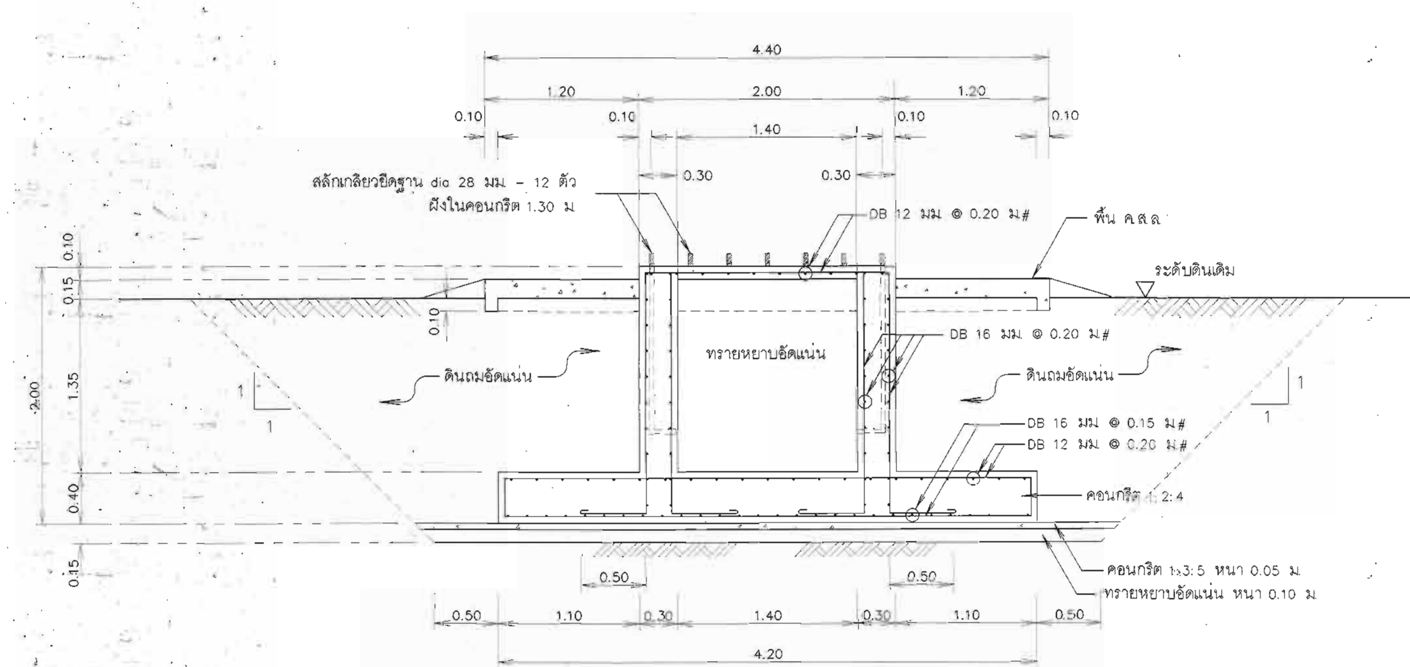
รูปตัด ก-ก
