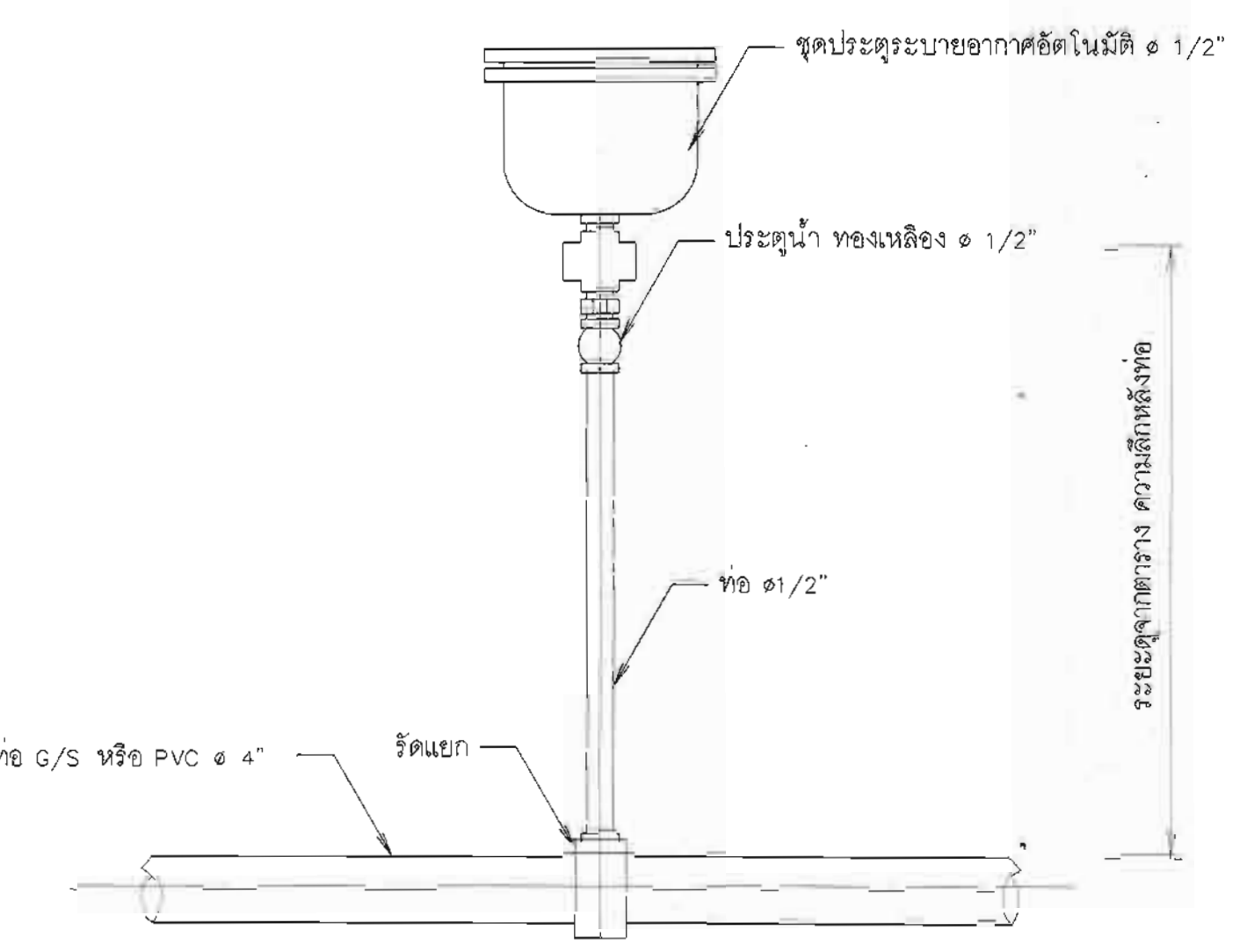
12. การติดตั้งประตูล็อกอากาศอัตโนมัติ ไม่แสดงมาตราส่วน
