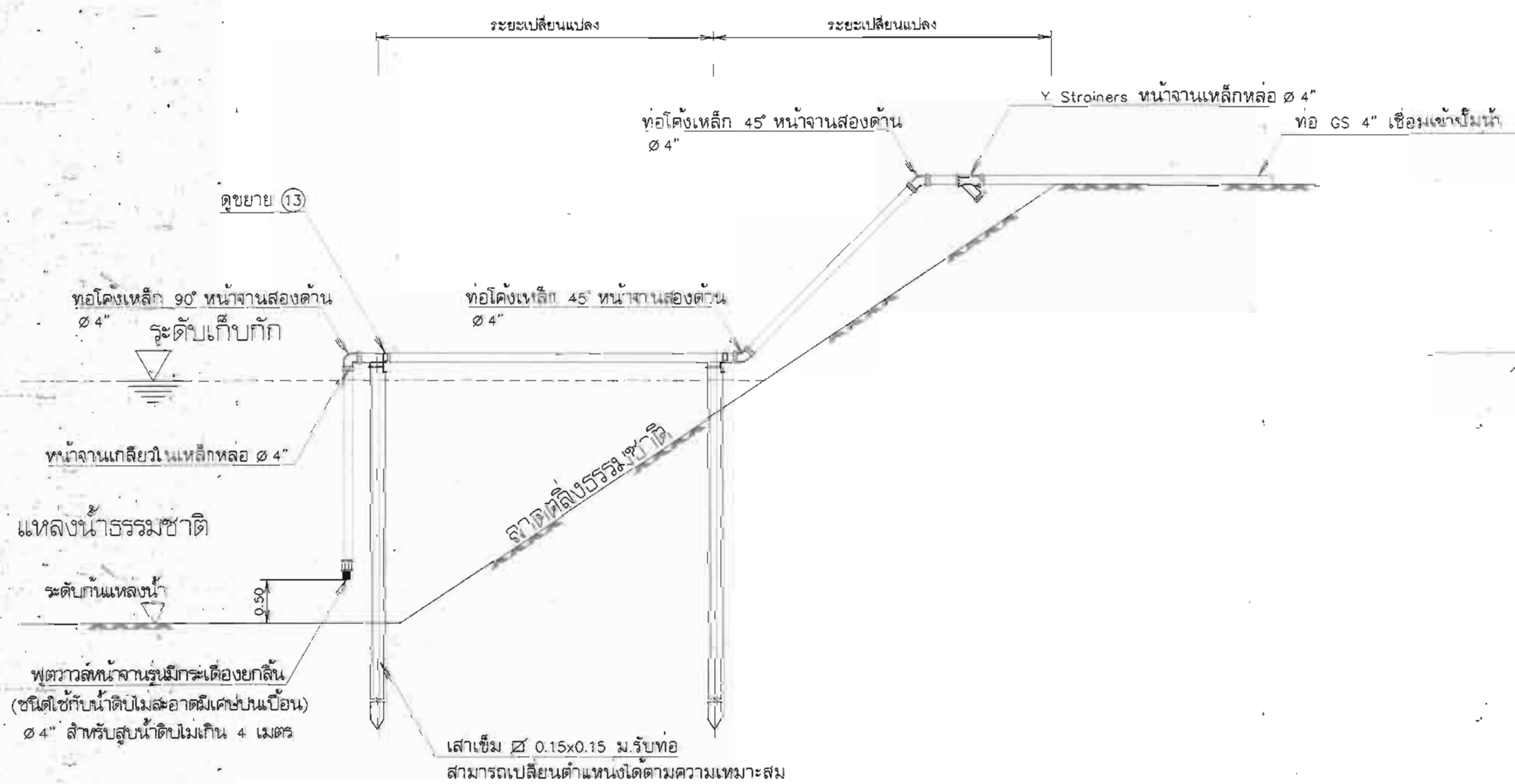
แบบขยายการเดินท่อน้ำจากแหล่งน้ำดิบ
