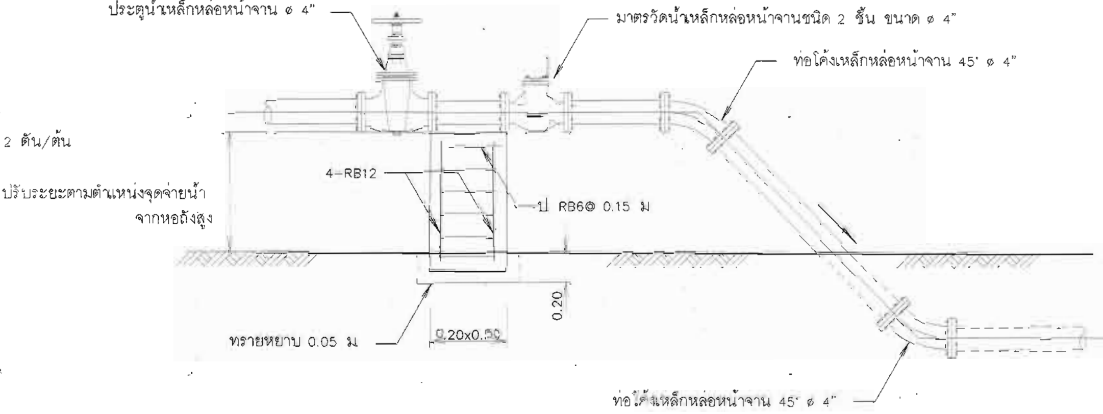
14. การติดตั้งมาตรวัดน้ำบนพื้นดิน ๑ 4" ไม่แสดงมาตราส่วน
