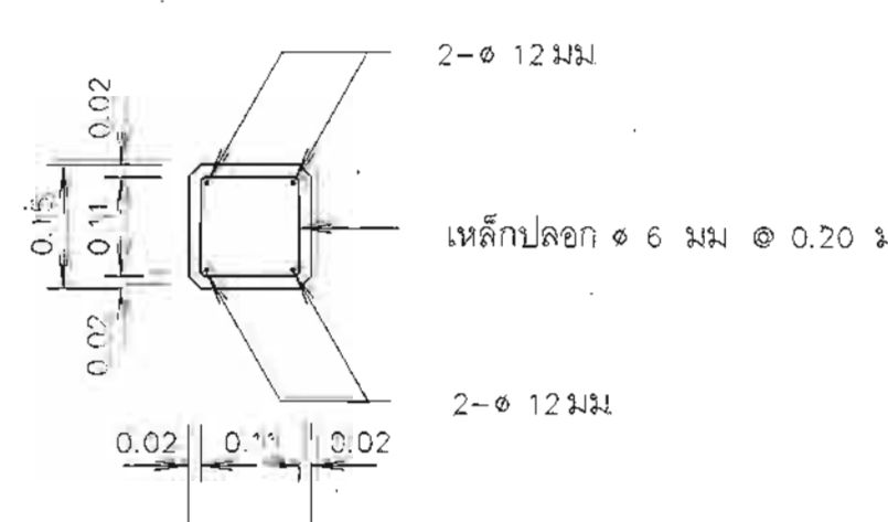
รูปตัด ข-ข
