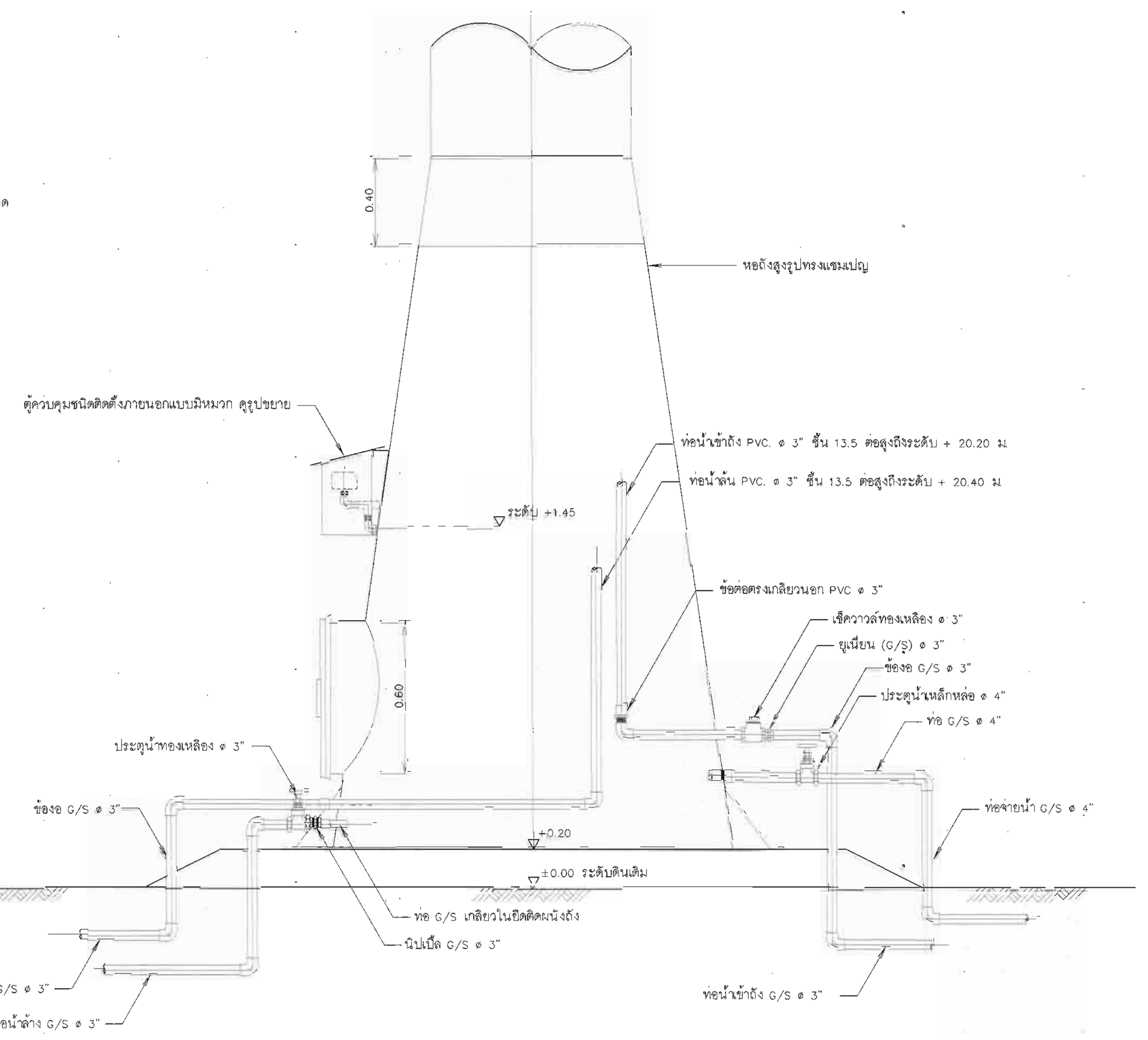
แบบแสดงการเดินท่อในห้องสูง ไม่แสดงมาตราส่วน
