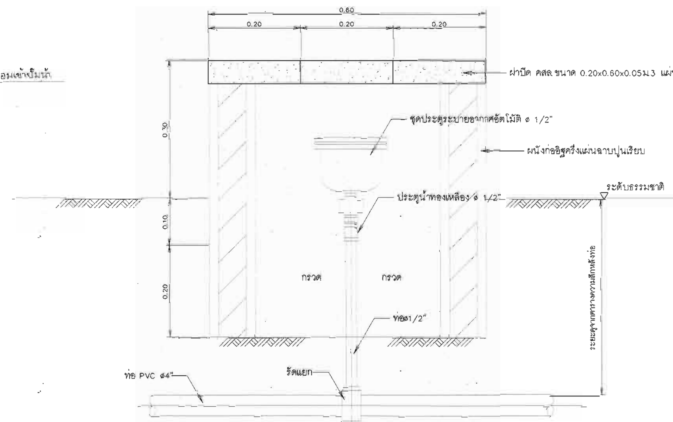
12 การติดตั้งประตูละบายอากาศอัตโนมัติ
