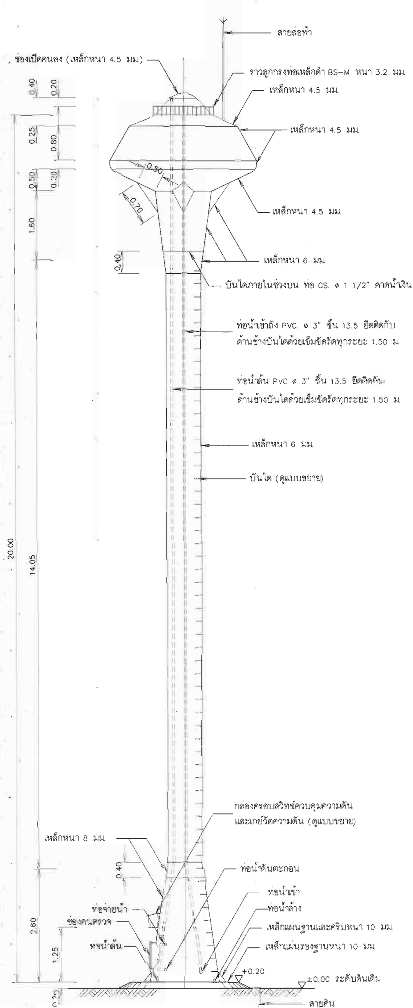
รูปด้านข้างท่อถึงสูง แบบถังเหล็กรูปทรงแฉมแปญ ไม่แสดงมาตราส่วน
