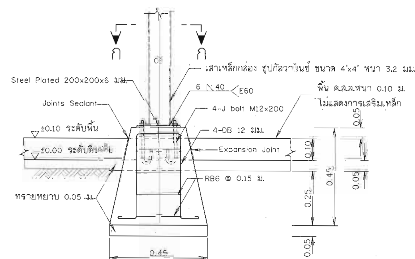
รูปขยายฐานรากโครงสร้างรับแผง F1
