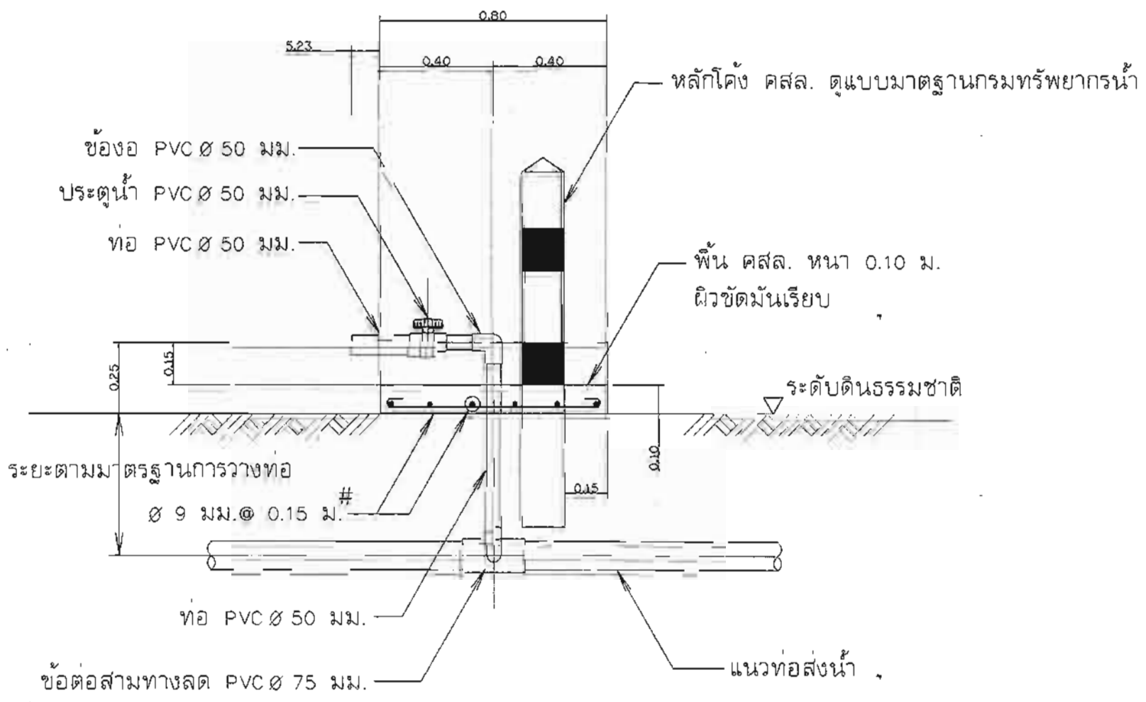
รูปตัด ก - ก แสดงการติดตั้งประตูดปล่อยน้ำ มาตราส่วน 1:20
