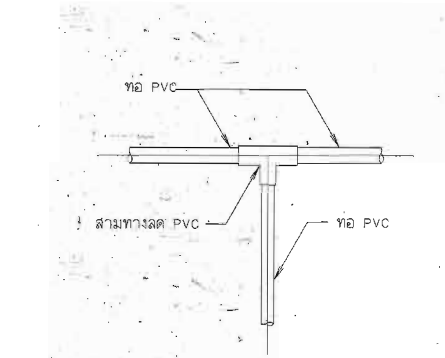
9. แบบการต่อสามทางลด PVC
