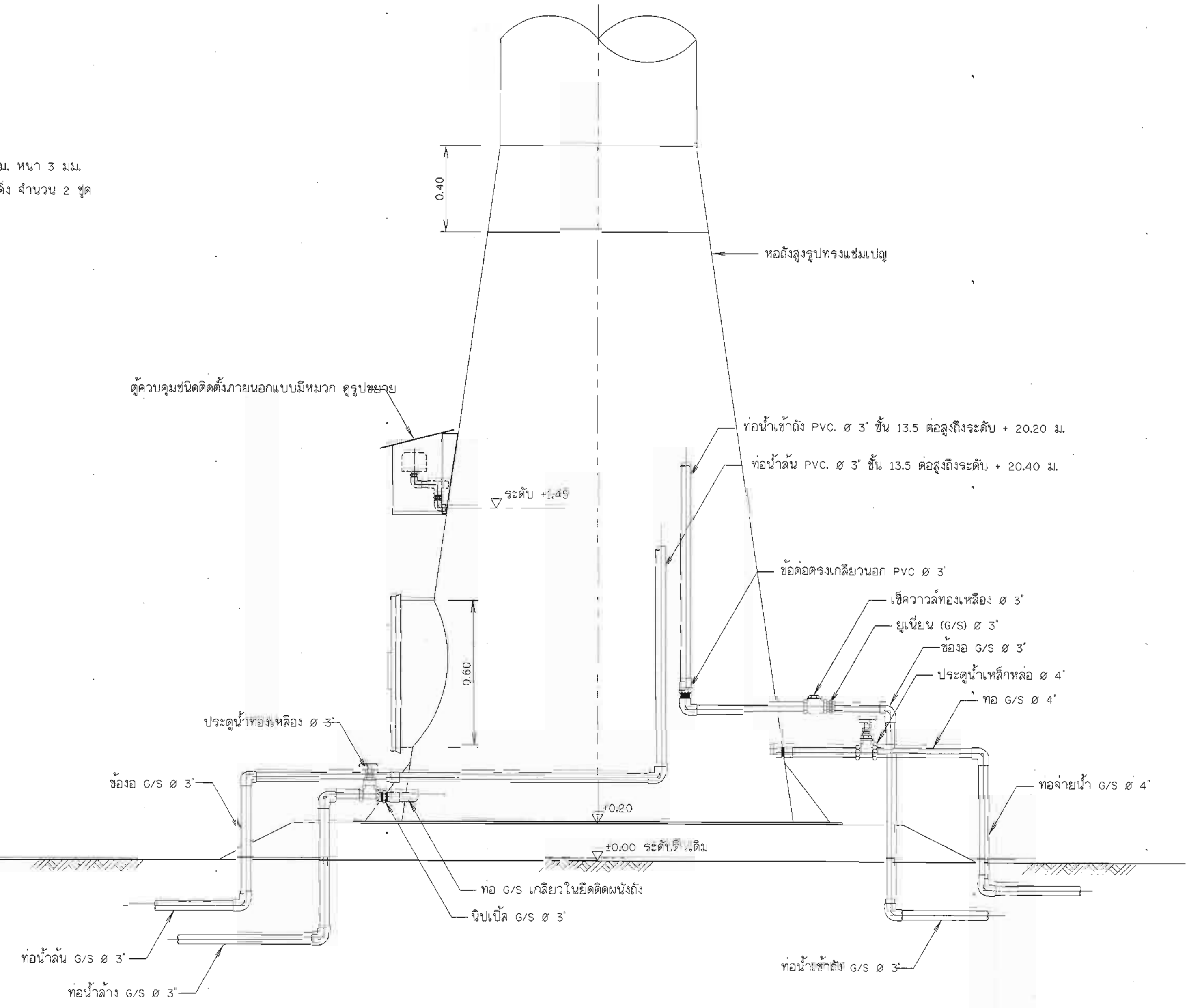
แบบแสดงการเดินท่อในห้องสูง
