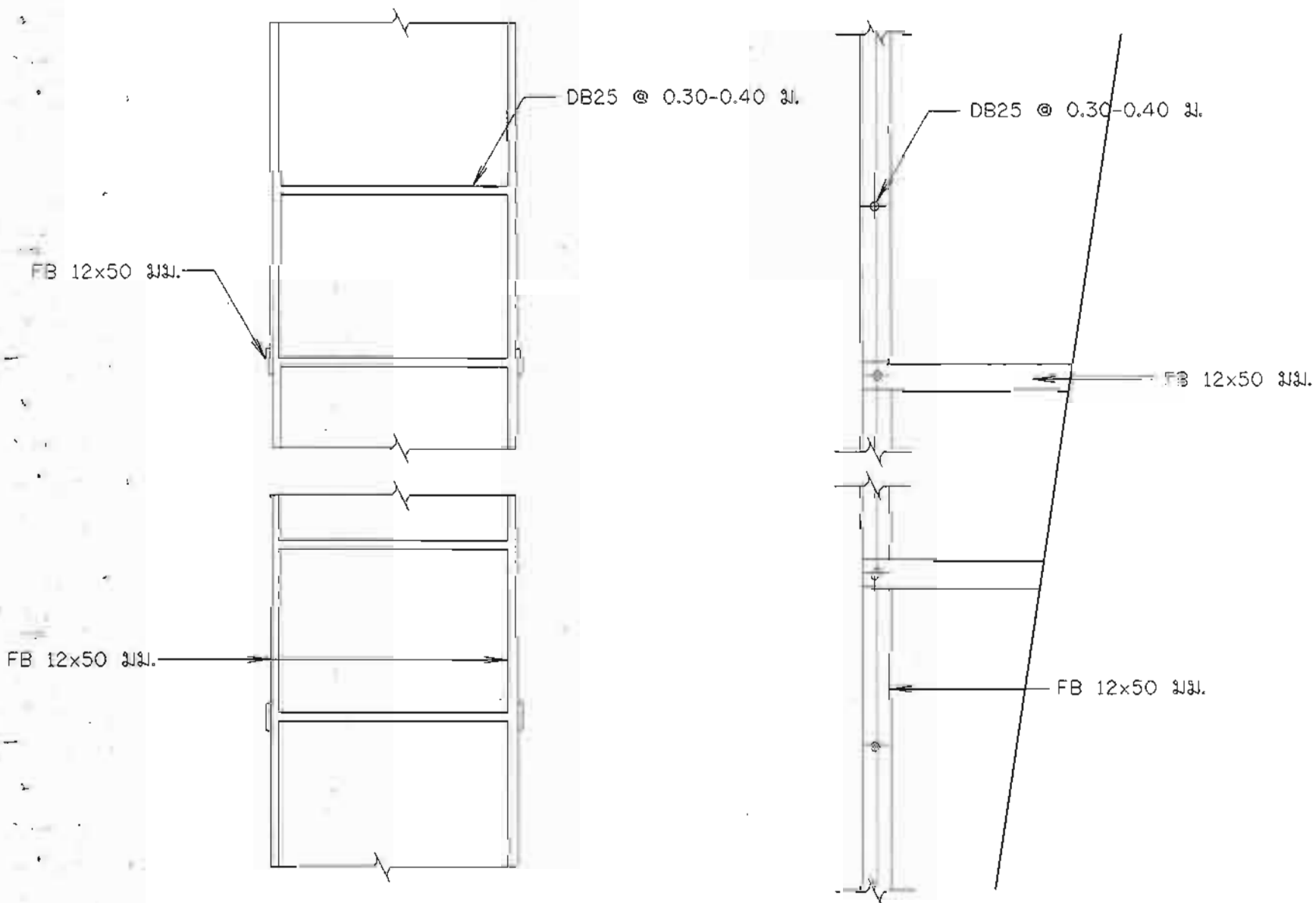
แบบขยายบันได ภายในห้องสูง
