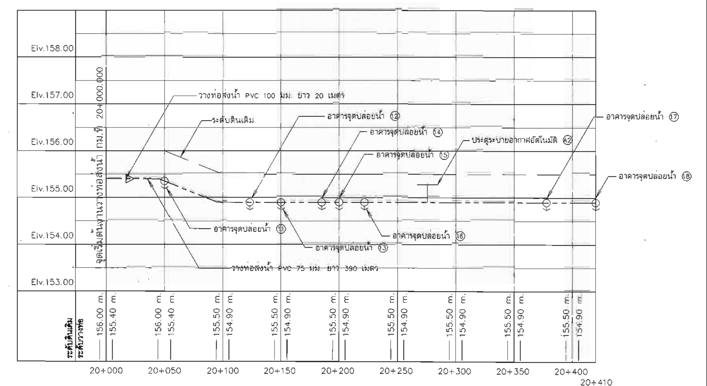
รูปตัดตามยาว PROFILE (B) ท่อส่งน้ำ PVC 75-100 มม. (STA.20+000 - STA.20+410)
