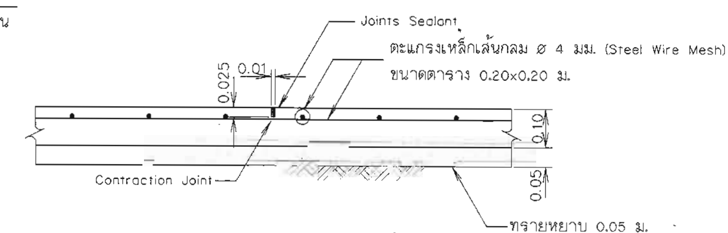
แบบขยายรอยต่อพื้น (Concrete Joint) ไม่แสดงมาตราส่วน
