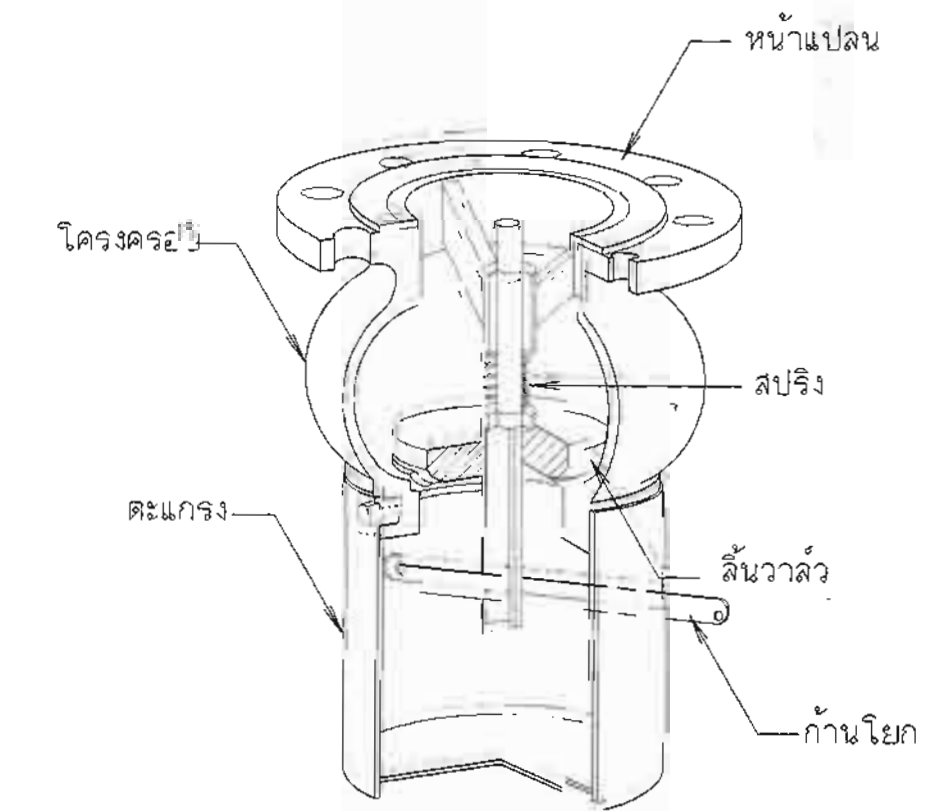
ฟุตวาล์ว แบบก้านโยก
