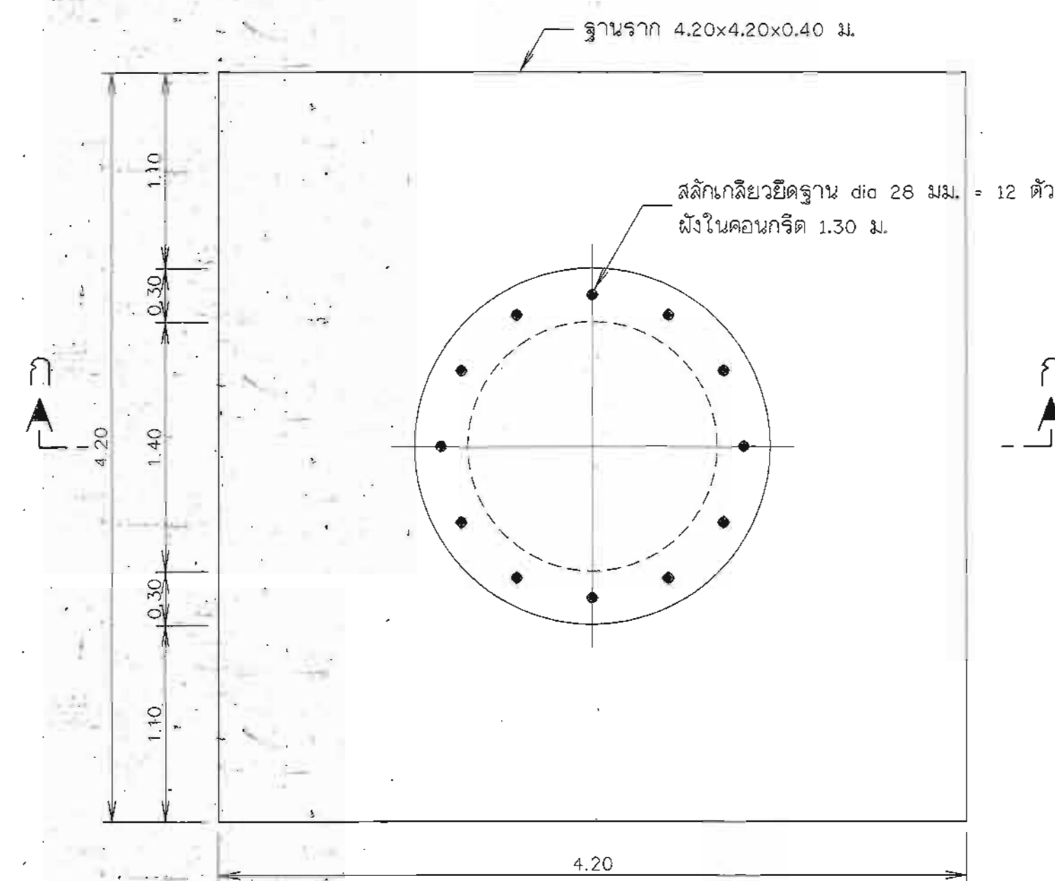
แปลน ฐานรากห่อถังสูง (แบบฐานแฉก)
