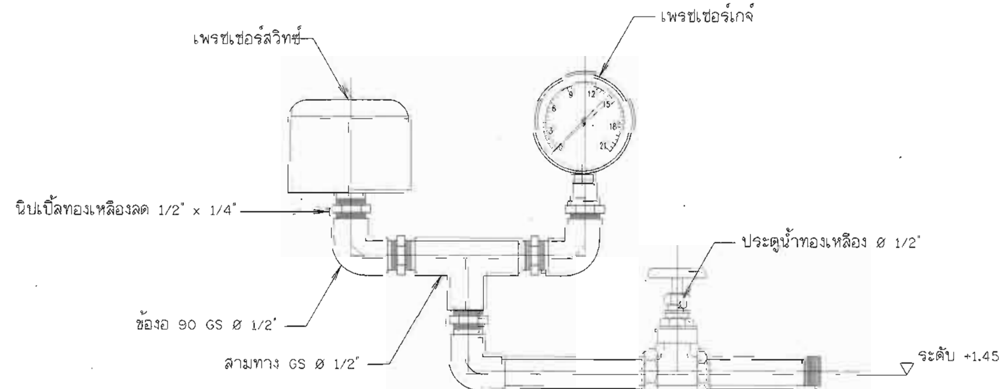
แบบขยายสวิตช์ควบคุมและเก้วัดความดัน
